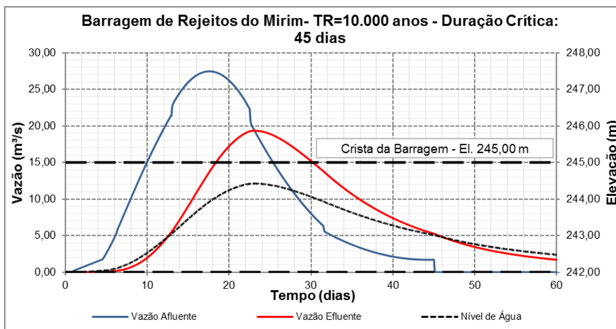
Figura 13 – Trânsito da cheia decamilenar com duração de 45 dias no reservatório da Barragem de Rejeitos do Mirim – El. 245,00 m
