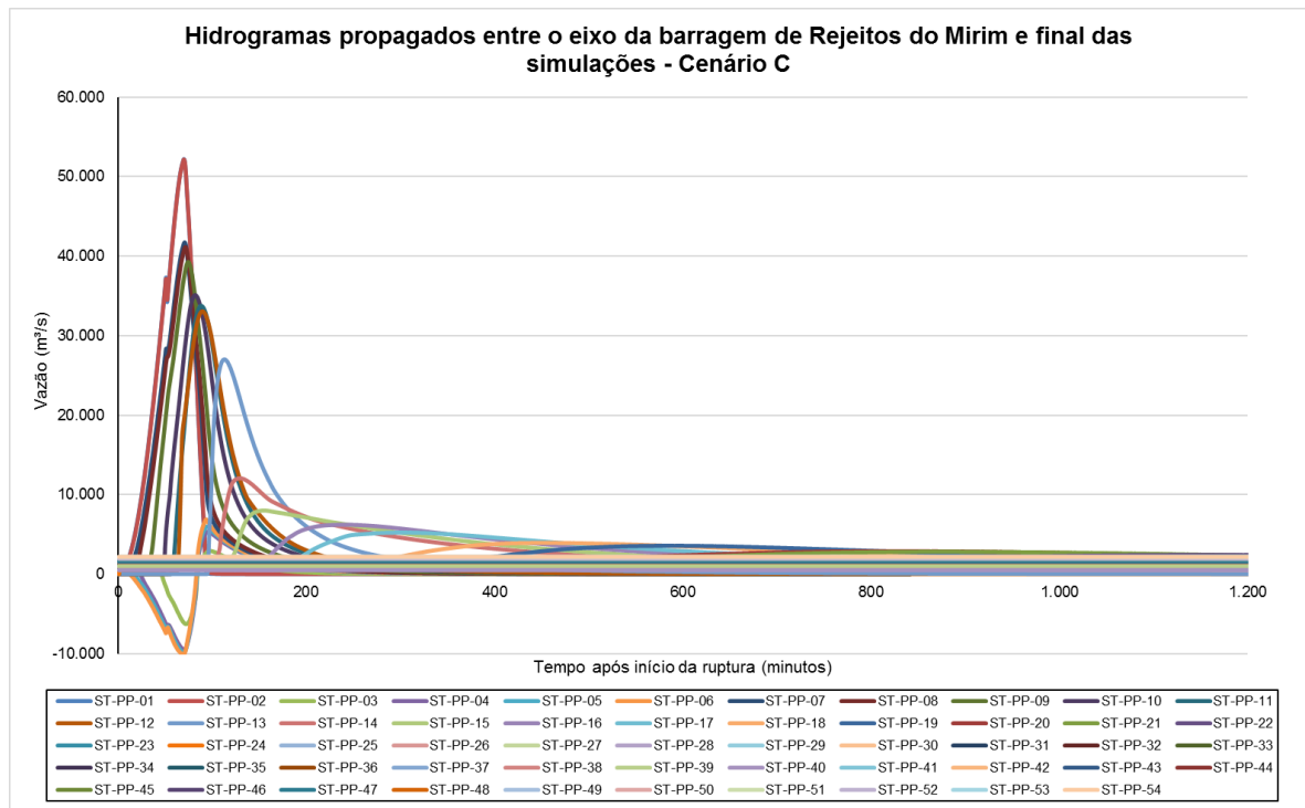
Figura 19 – Propagação do hidrograma de ruptura hipotética da barragem de Rejeitos do Mirim – Cenário C (Ruptura em dia seco)
