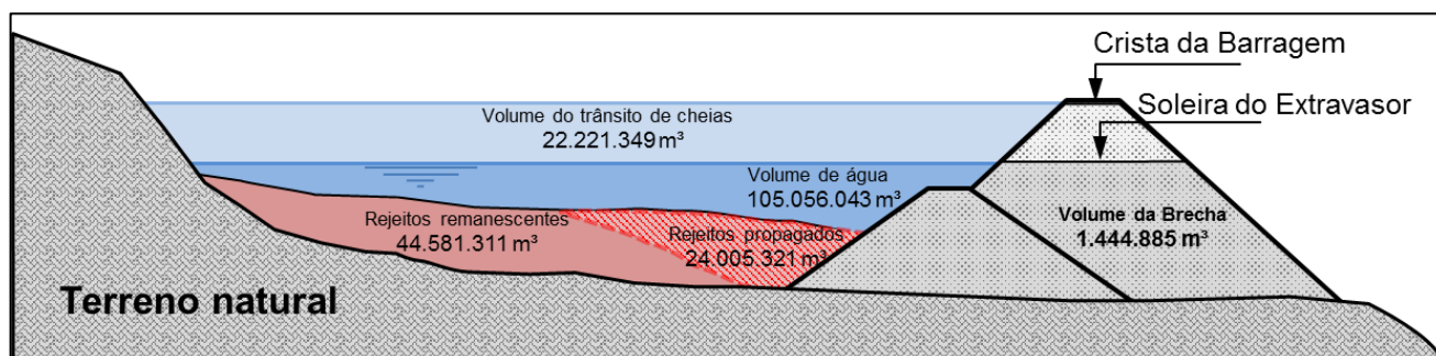
Figura 11 – Croqui esquemático da ocupação do reservatório da Barragem de Rejeitos do Mirim (sem escala).
