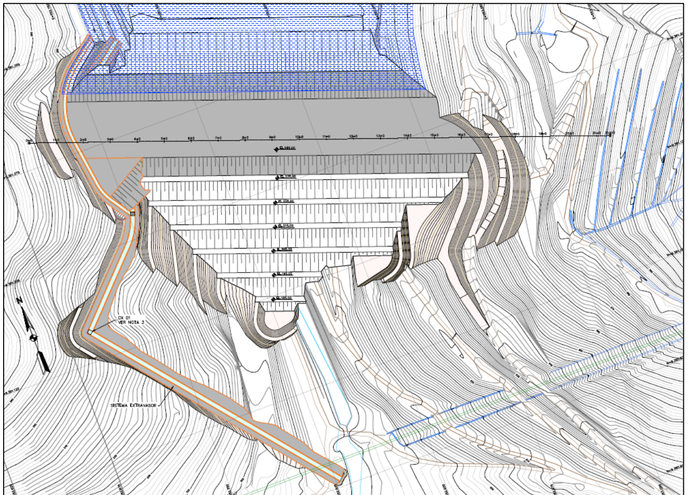
Figura 2 – Arranjo Geral da Barragem de Rejeitos do Mirim (El. 245,00 m) – Planta. Fonte: MC-9002SA-G-00001
