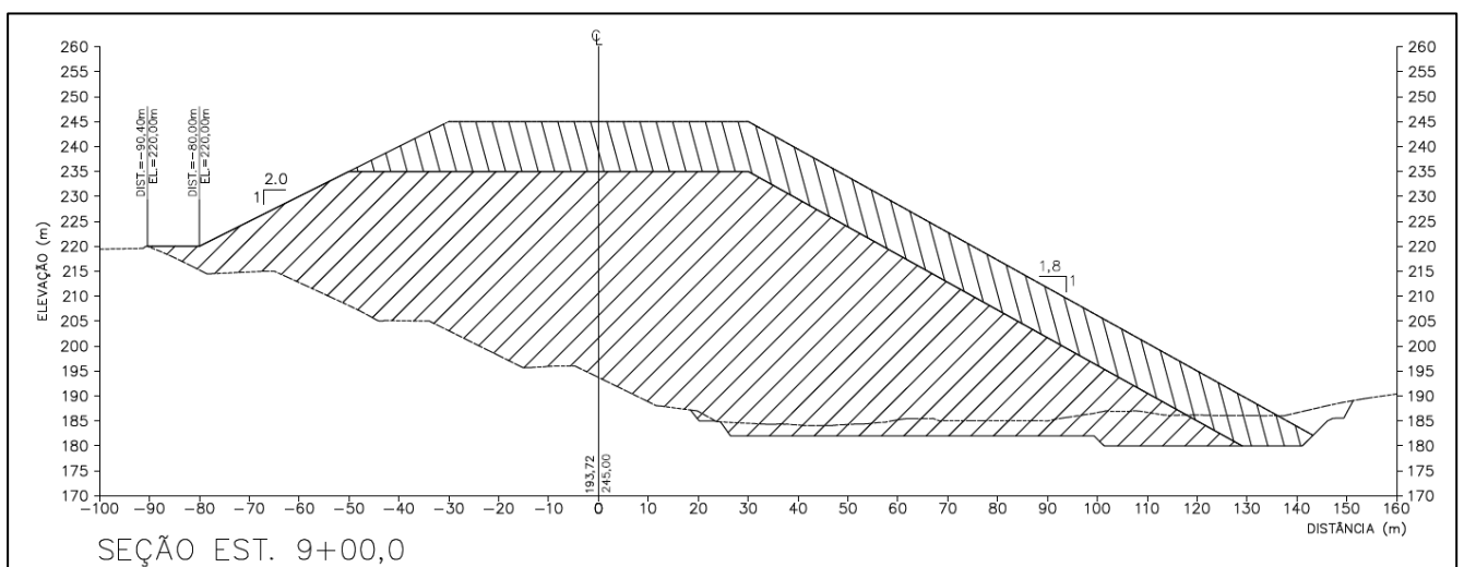
Figura 3 – Arranjo Geral da Barragem de Rejeitos do Mirim (El. 245,00 m) – Corte.
