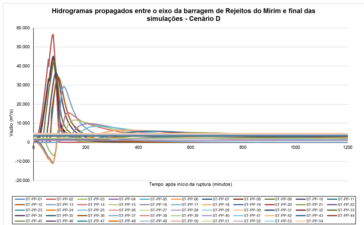
Figura 20 – Propagação do hidrograma de ruptura hipotética da barragem de Rejeitos do Mirim – Cenário D (Ruptura em dia chuvoso)
