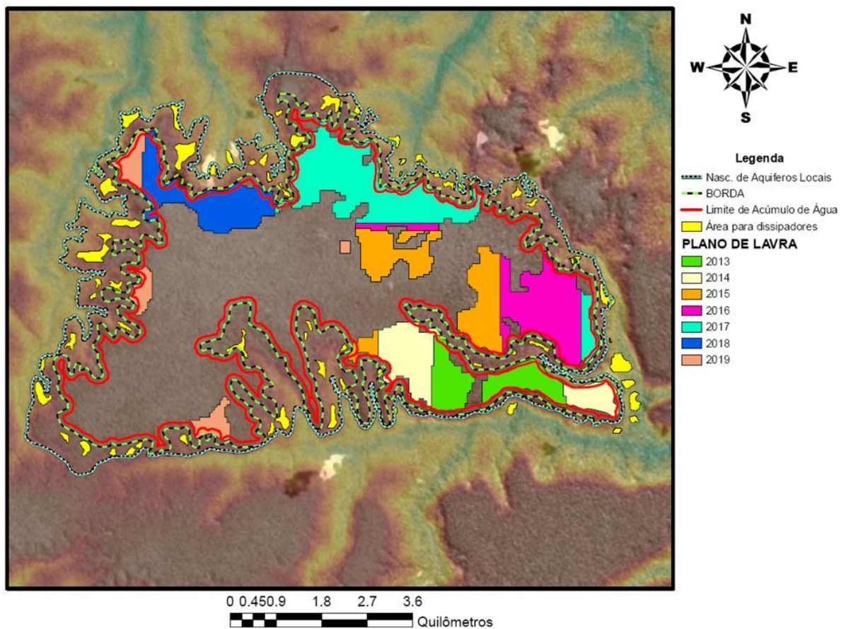
Figura 10 – Definição da área de contribuição a ser drenada (entre a borda e o limite de acúmulo de água – 100m) e áreas recomendadas para as caixas dissipadoras de energia (em amarelo).
