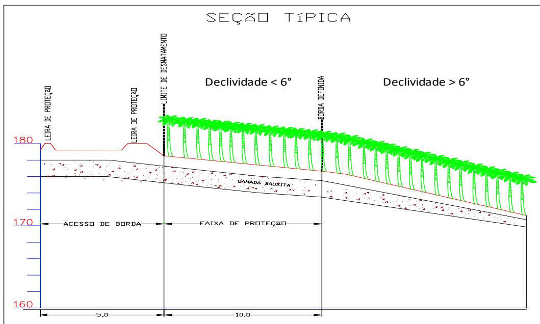
Figura 8 – Seção típica da borda de um platô.
