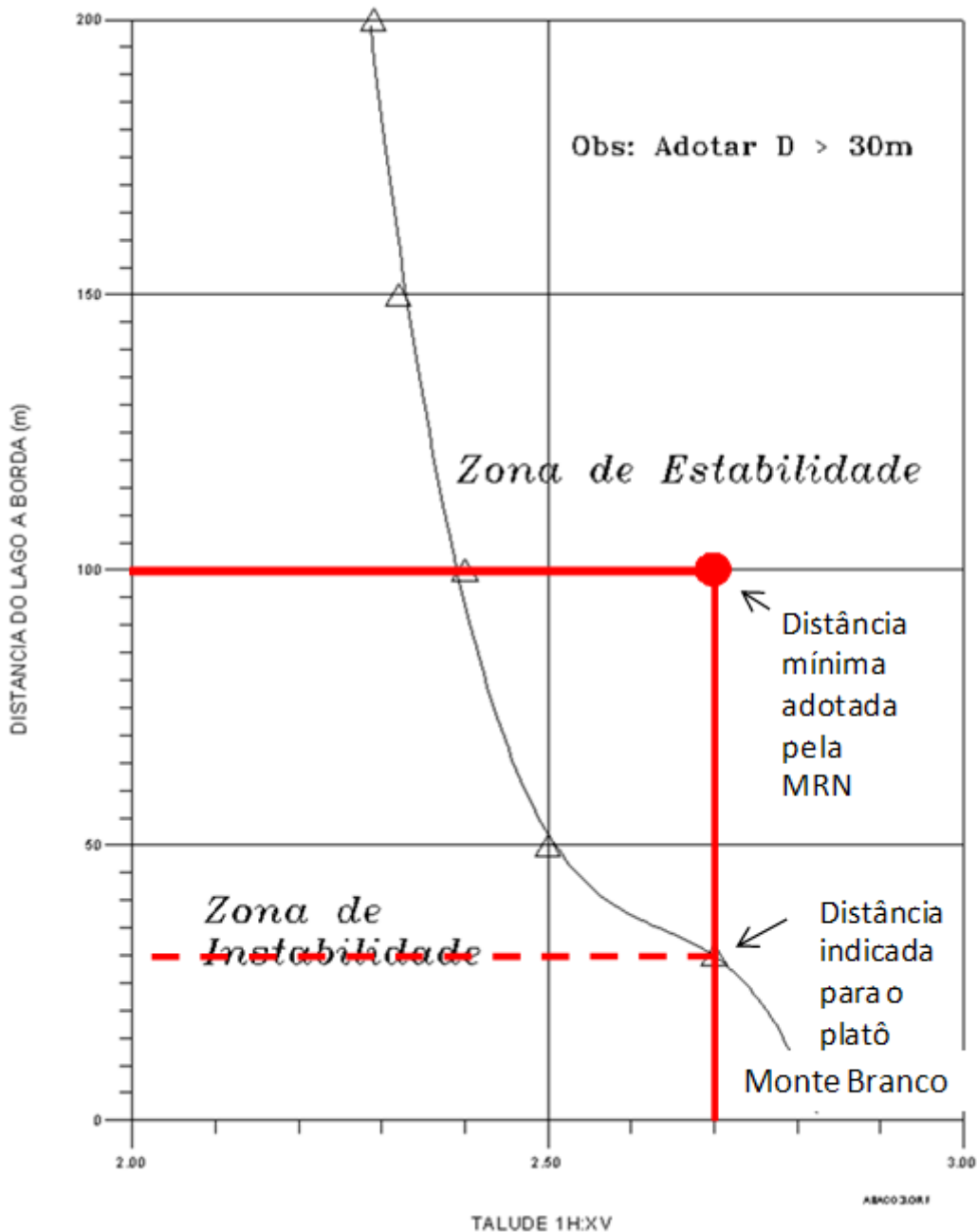
Figura 9 – Ábaco para determinação da distância mínima da borda para acumulação de água.
