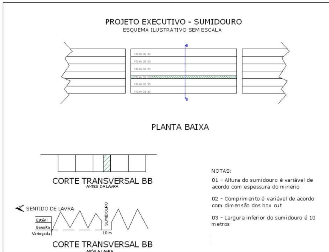
Figura 18 – Projeto executivo dos sumidouros
