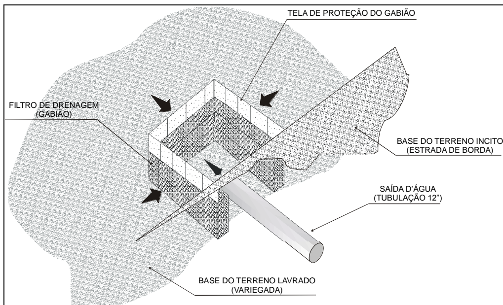
Figura 19 – Desenho esquemático de um filtro de gabião.
