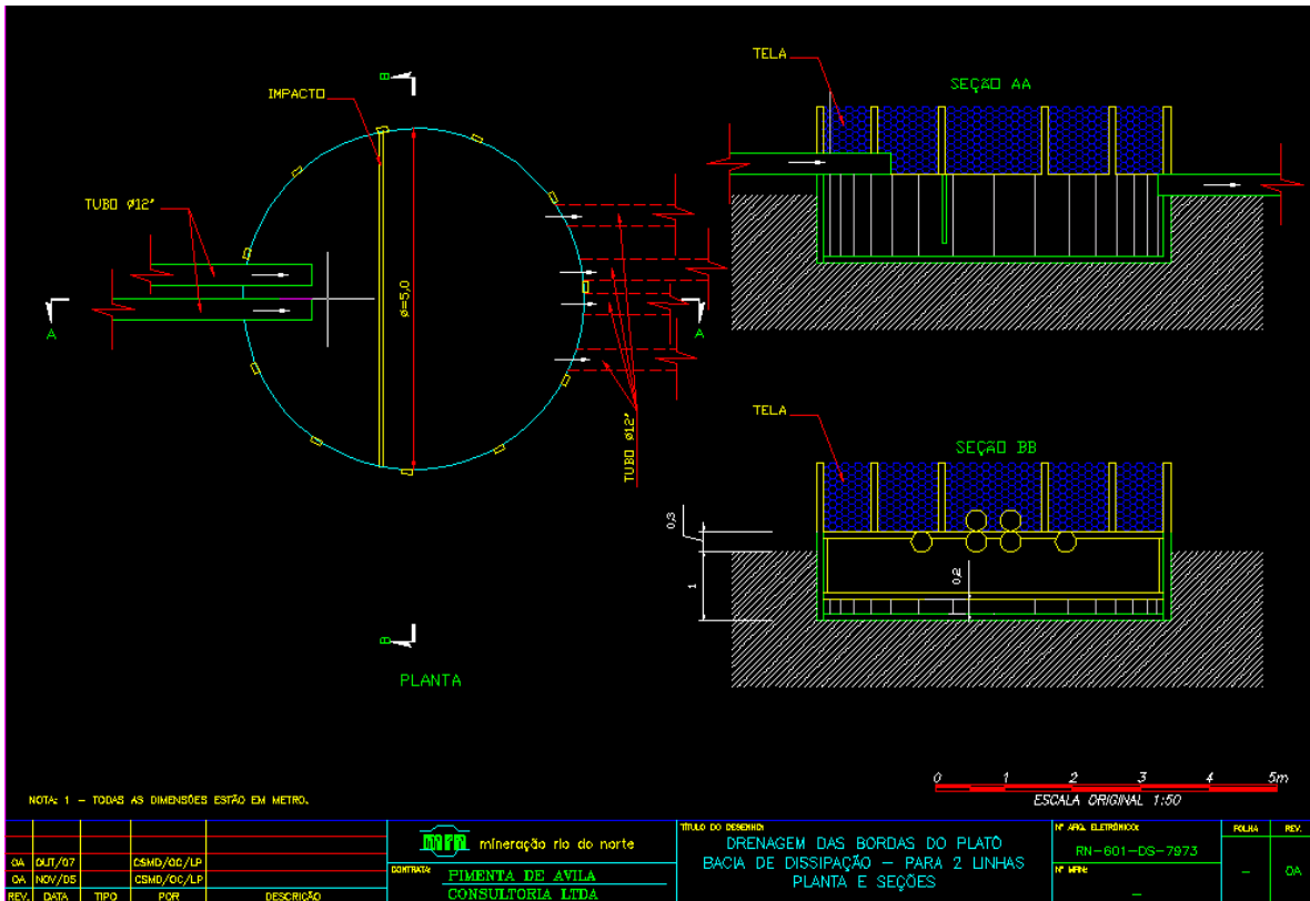
Figura 20 – Esquemas construtivos das caixas de dissipação de energia.
