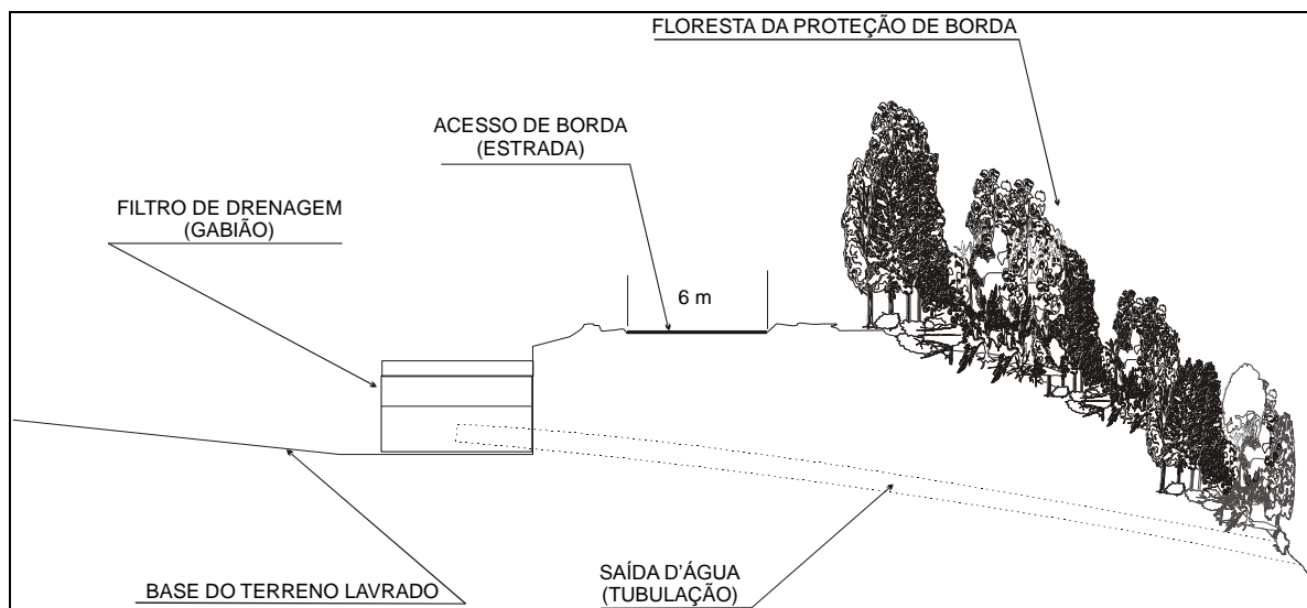
Figura 4 – Perfil esquemático do sistema de drenagem.
