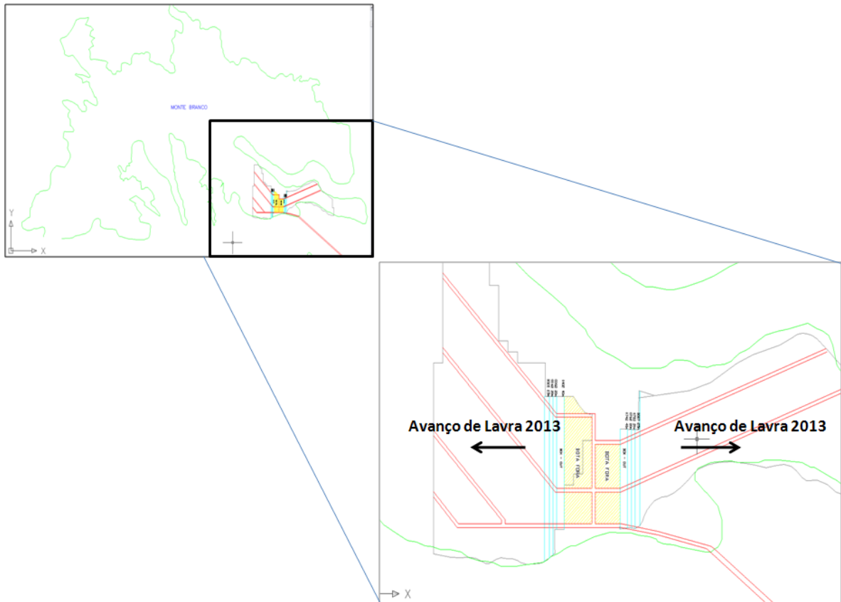
Figura 3 – Desenho esquemático para abertura do “box-cut” na mina do platô Monte Branco.
