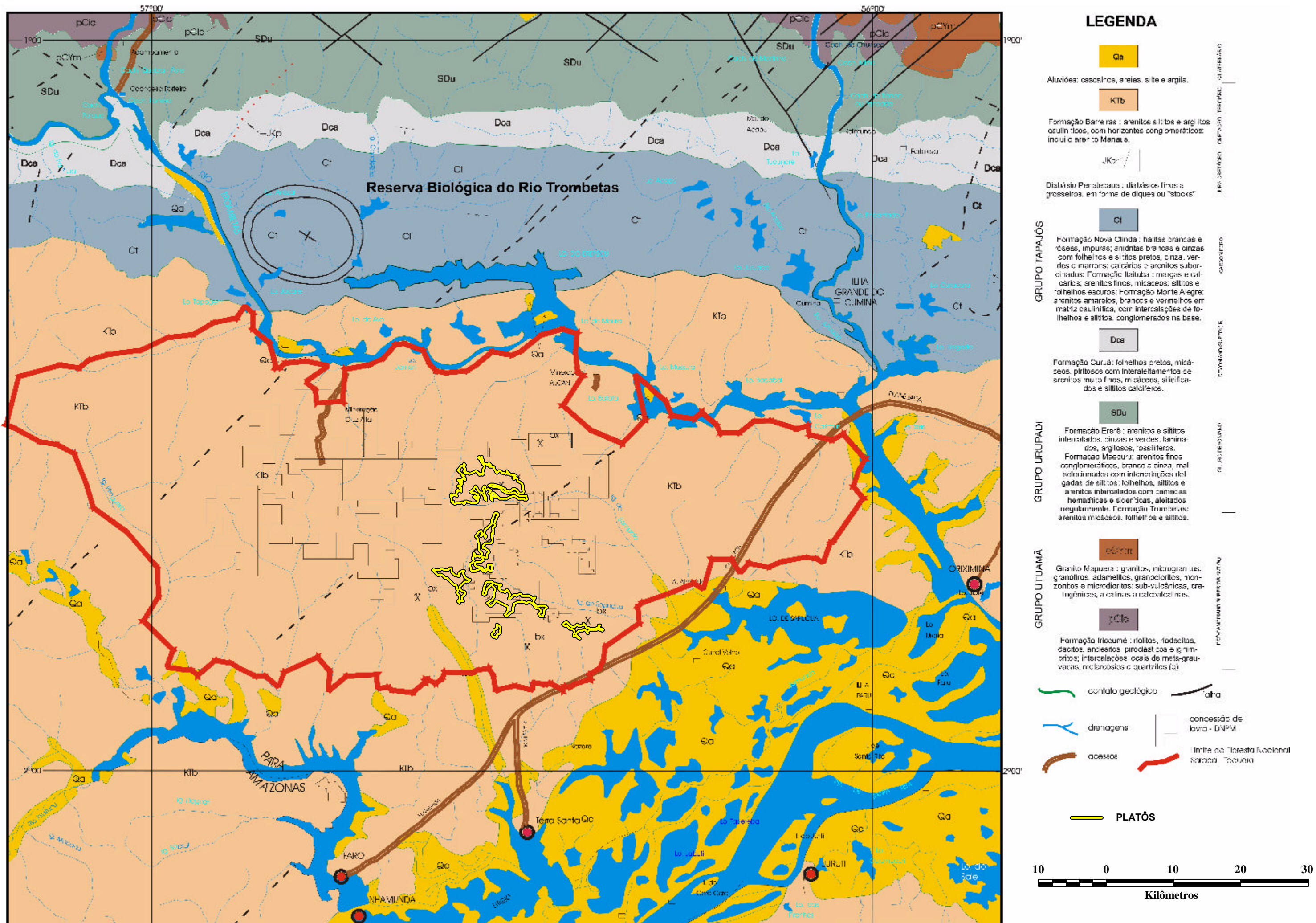
FIGURA 5.8 - Mapa da geologia regional
