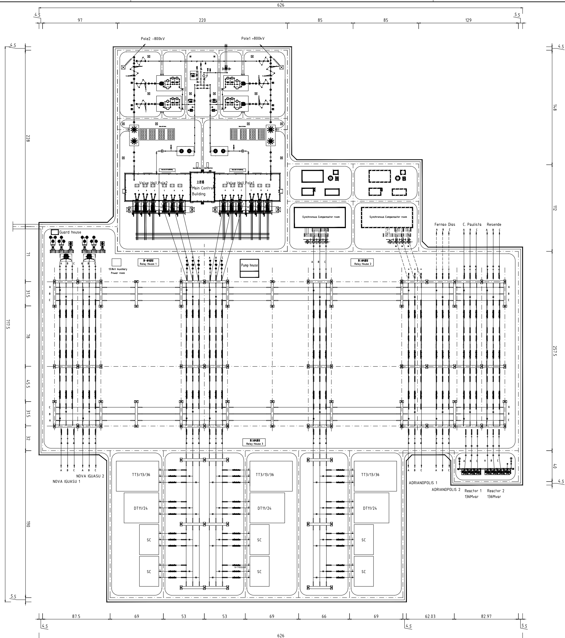
PLANTA
