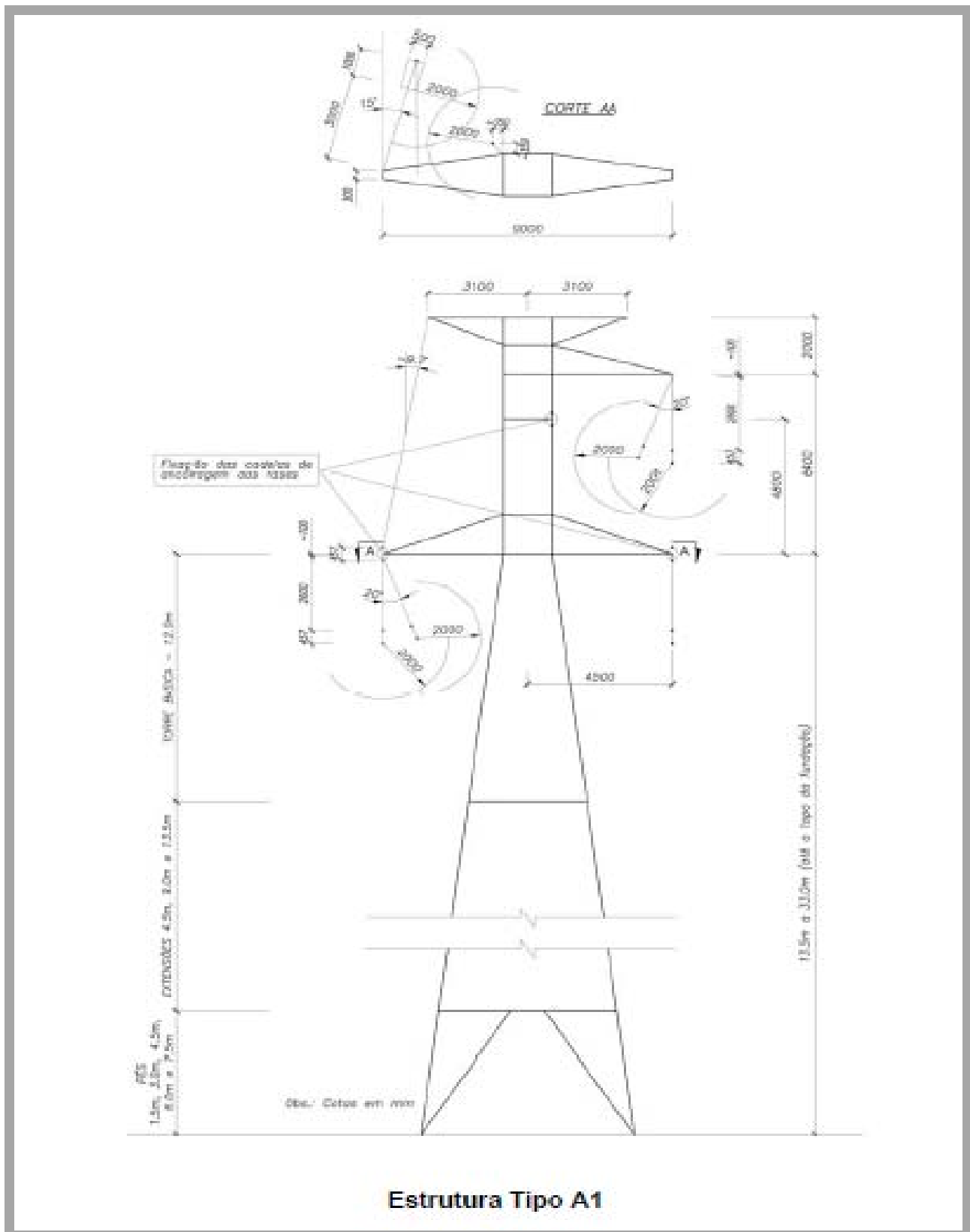
Figura 3.4.4.2-4: Torre de Ancoragem Média Autoportante.
