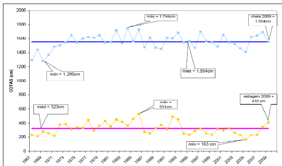
Figura 3.6.3.9.3-7: Variação das cotas máximas e mínimas na bacia do rio Madeira em Porto Velho-RO, no período de 1967 a 2010. (Fonte: ANA, 2009)
