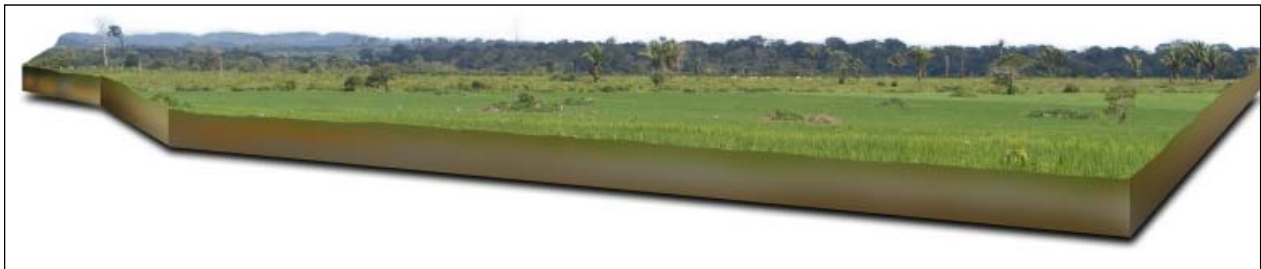
Figura 3.6.4.2-3: Vista geral do AMBIENTE 1 onde se percebem, em primeiro plano, os solos mais alagados e ao fundo pastagens de braquiária e a floresta.
