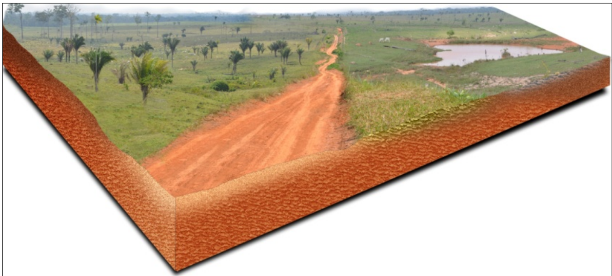
Figura 3.6.4.2-7: Presença de Latossolos Vermelhos na região de Acrelândia (Acre). Ocorrem com maior frequência nos topos da paisagem em relevo plano a suave ondulado.
