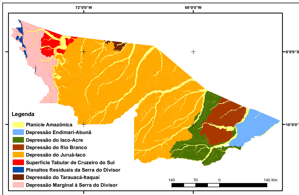
Figura 3.6.3.5.1-1: Distribuição das unidades geomorfológicas do estado do Acre. Fonte: Base de dados geográficos do ZEE/AC, Fase II, 2006.
