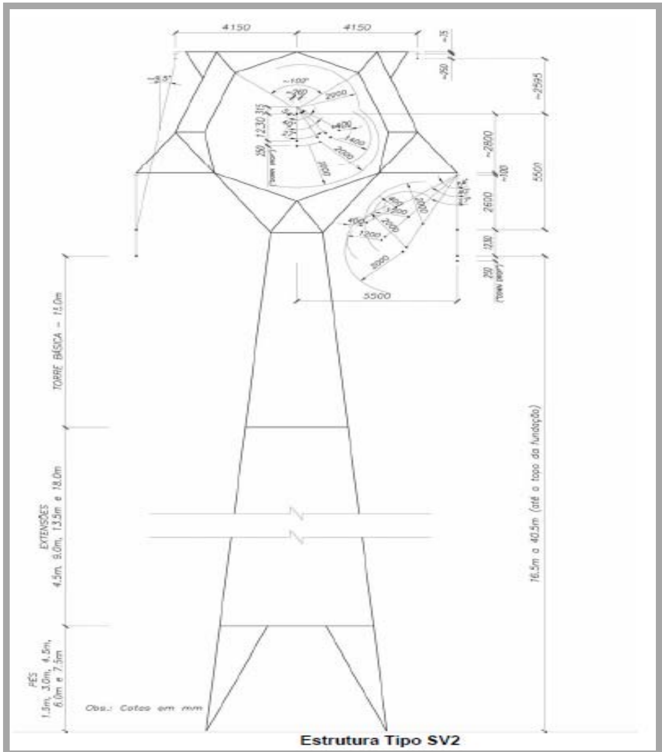
Figura 3.4.4.2-3: Torre de Suspensão Pesada Autoportante.
