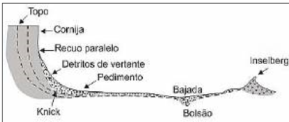
Figura 3.6.3.5.1-4: Modelo de Evolução de um Pediplano. Fonte: AMARAL (2008).
