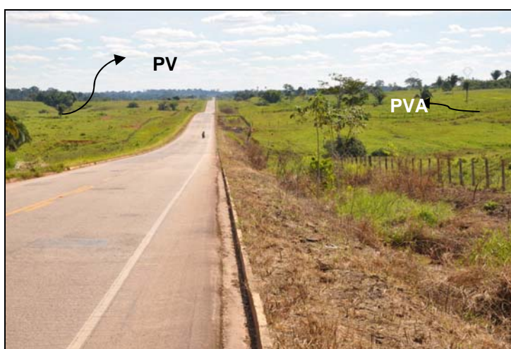
Figura 3.6.3.6.2-20: Pedaambiente com domínio de Argissolos Vermelhos e Vermelho-Amarelos (PV/PVA), no trecho 4 entre o rio Marmelo e a Divisa com o Estado do Acre. Fonte: NEPUT, 2010.
