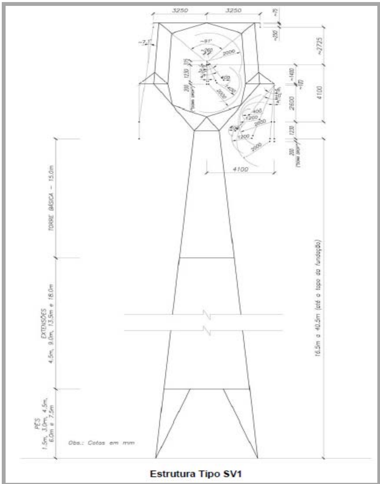
Figura 3.4.4.2-2: Torre de Suspensão Leve Autoportante.
