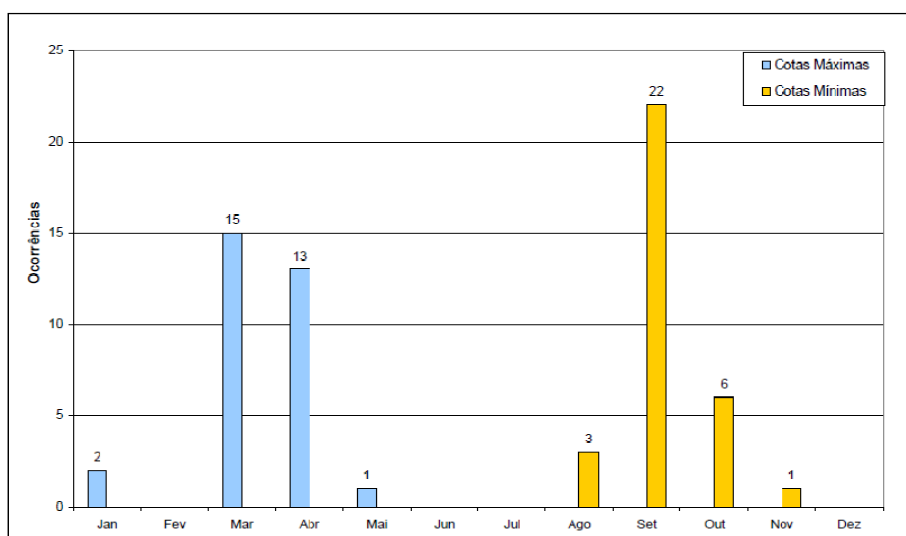
Figura 3.6.3.9.3-12: Variação das cotas máximas e mínimas do rio Abunã, afluente do rio Madeira, no período de 1976 a 2010. Distribuição mensal das ocorrências de cotas máximas e mínimas anuais. (Fonte: ANA, 2009).
