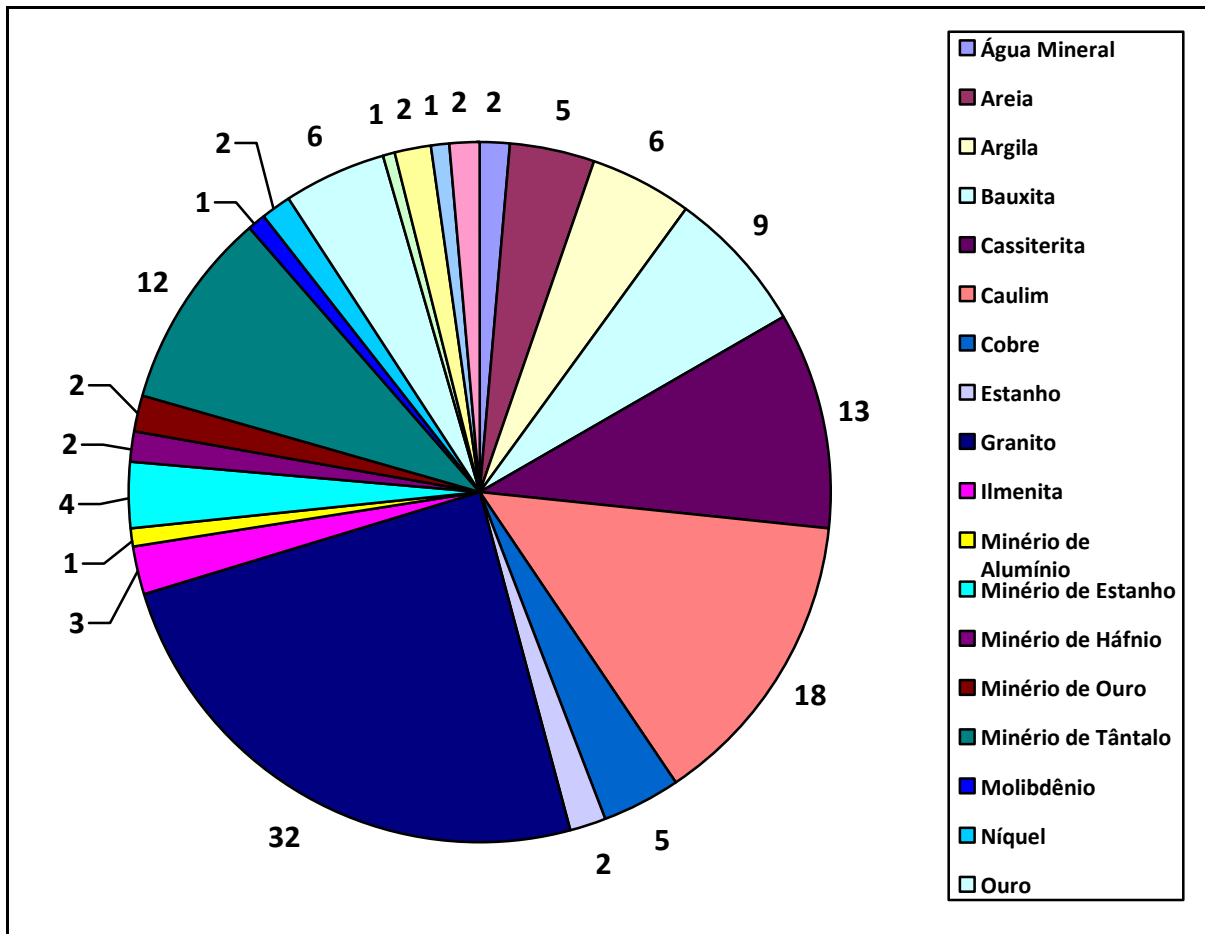
Figura 3.6.3.4-3 - Substâncias exploradas dos jazimentos minerais dentro da faixa de servidão.
