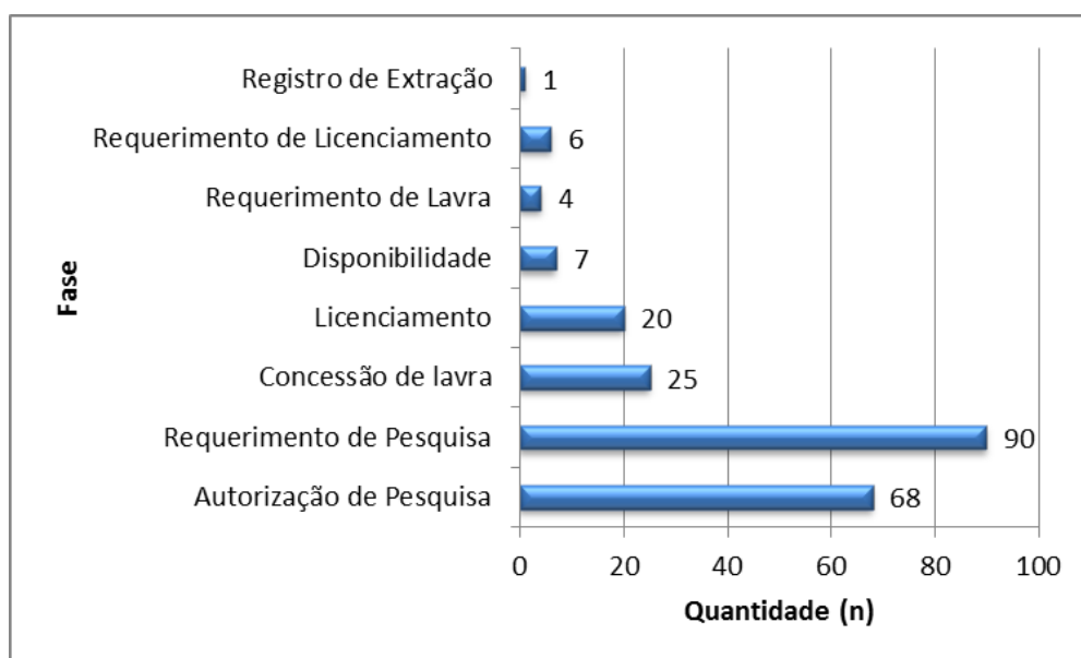
Figura 3.6.3.4-2 - Situação legal dos processos minerários junto ao DNPM, para a AID.
