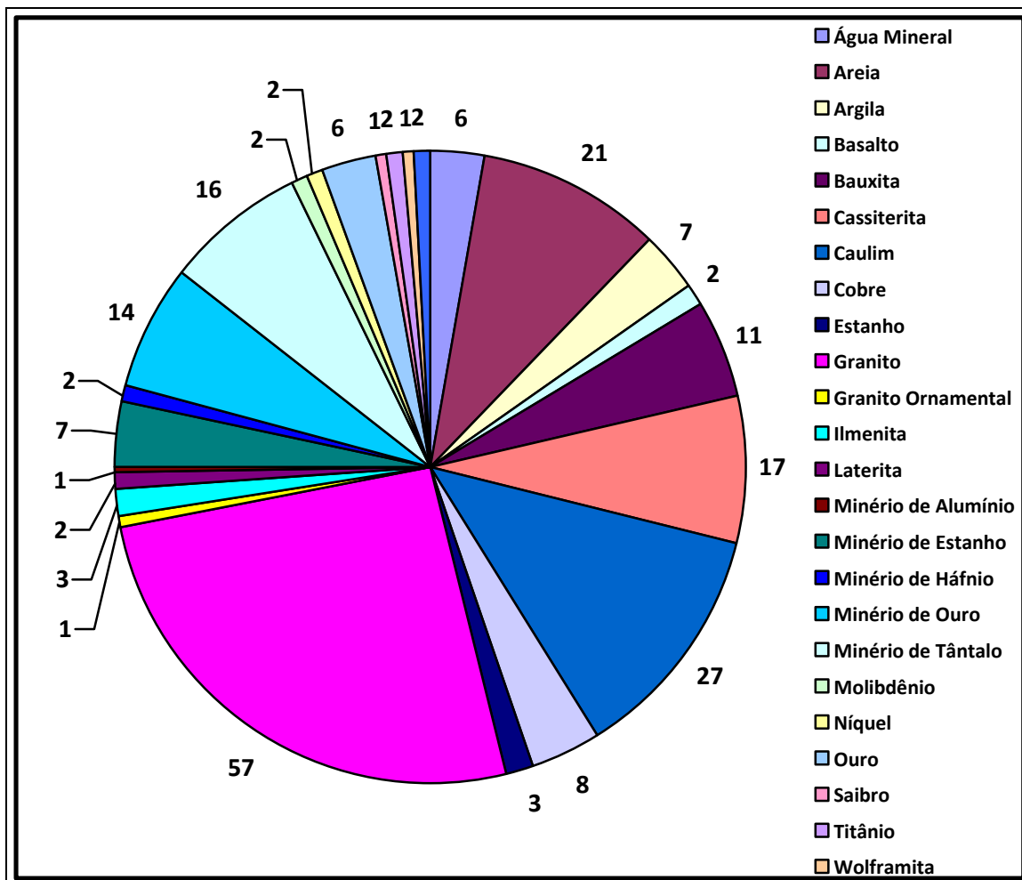
Figura 3.6.3.4-1 - Substâncias exploradas na AID da LT 500 kV Manaus - Boa Vista e Subestações Associadas
