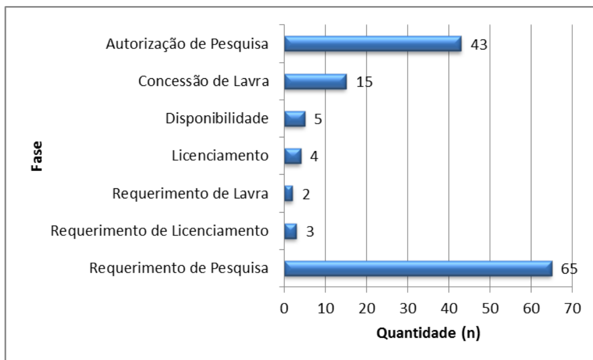
Figura 3.6.3.4-4 - Situação Legal dos processos minerários, junto ao DNPM, na faixa de servidão da LT.
