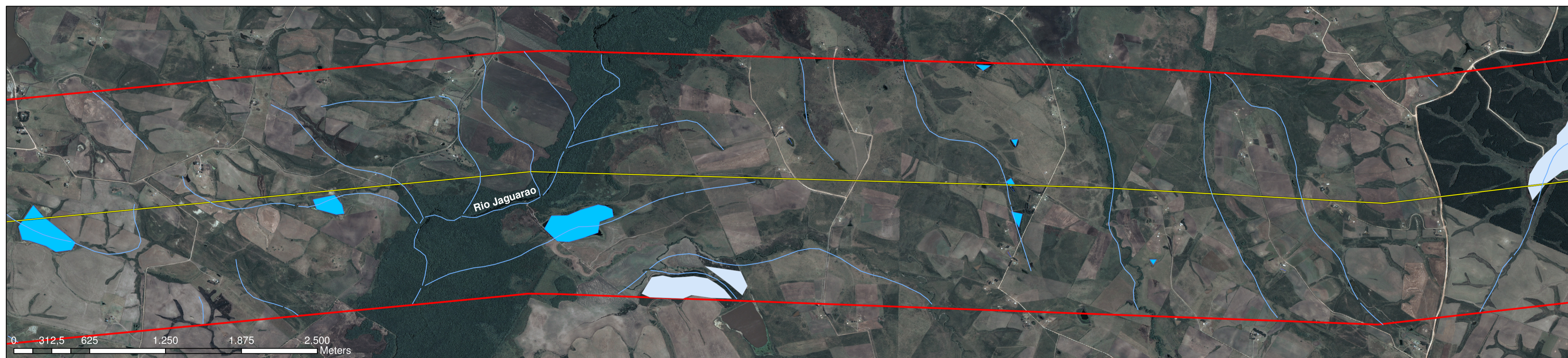
Imagem orbital do KM 4, da interligação energética Brasil - Uruguai
