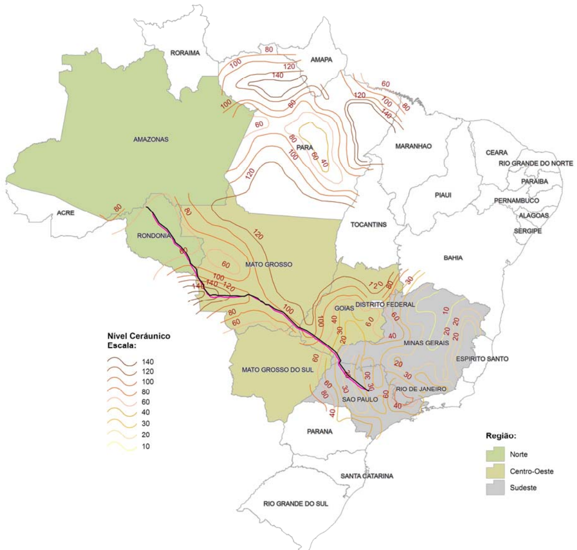
Figura 3.6.3.1-19 – Isoceraunicas distribuídas pelos estados atravessados pela LT
