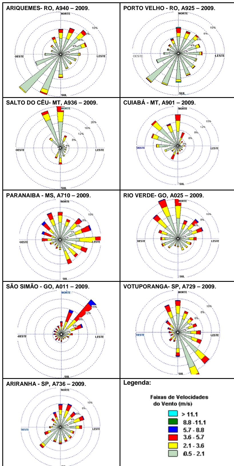
Figura 3.6.3.1-17 – Rosa dos Ventos anual de 2009, ao Longo da AII da Linha de Transmissão. Fonte: (INMET, 2009)
