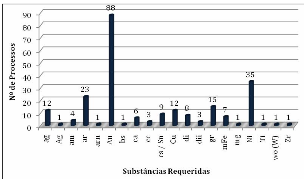
Figura 3.6.3.7-4 – Histogramas das Principais Substâncias Requeridas nos Processos DNPM na AID da LT.
