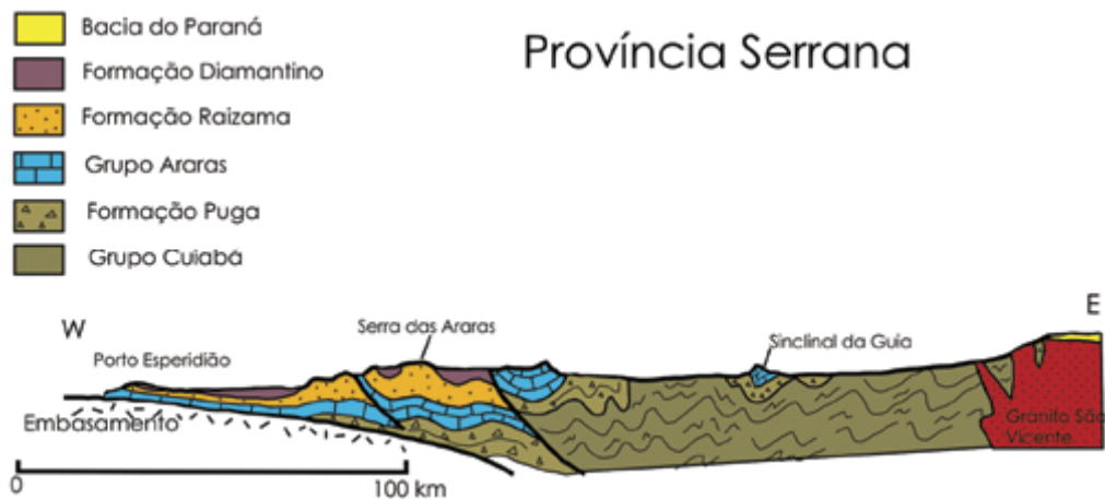
Figura 3.6.3.2-2 – Perfil esquemático transversal à estruturação da Faixa Paraguai na sua porção nordeste (Fonte: BOGGIANI & ALVARENGA, 2004).
