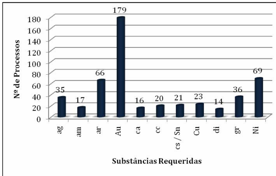
Figura 3.6.3.7-2 – Histogramas das Principais Substâncias Requeridas nos Processos DNPM na All da LT. Fonte: SIGMINE, DNPM (13/02/2010).
