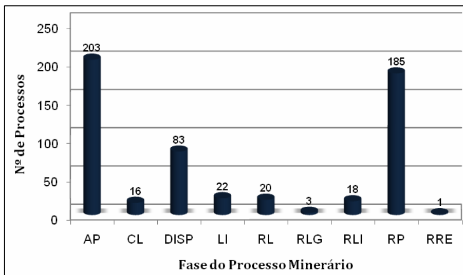
Figura 3.6.3.7-1 – Distribuição dos Processos de Direitos Minerários Requeridos na AII da LT, conforme a sua Fase de Tramitação no DNPM
