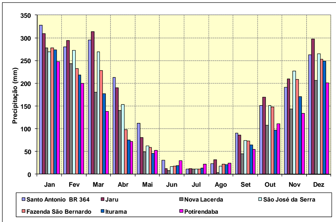
Figura 3.6.3.1-4 – Histograma Comparativo do Regime de Precipitações
