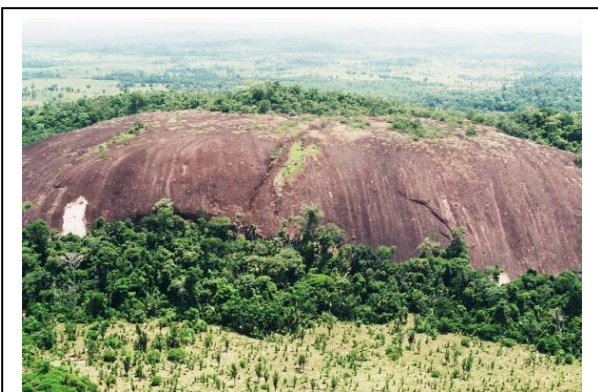
Foto 3.6.3.2-111 - Ponto 277: grande maciço rochoso Suíte Metamórfica Rio Crespo; do ponto 276 ao 277 são comuns afloramentos rochosos em terrenos rebaixados.
