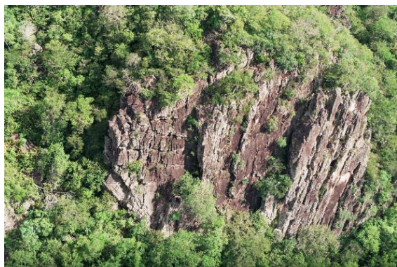
Foto 3.6.3.2-97 - Ponto 148: escarpas de rochas metassedimentares da Formação Raizama, na Serra das Araras.
