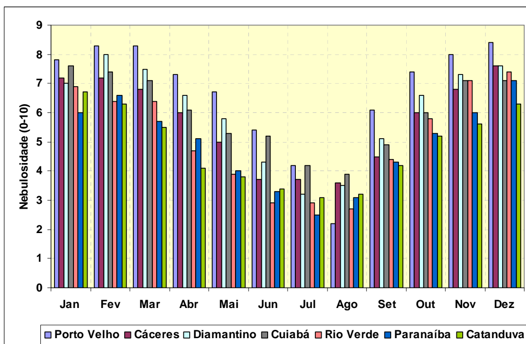
Figura 3.6.3.1-12 – Nebulosidade Média Mensal ao Longo da All da LT.
