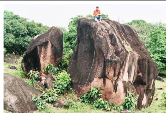
Foto 3.6.3.2-106 - Ponto 271: grandes matacões de granito equigranular rosa médio, com grãos de quartzo cinza-azulado estirados, imprimindo lineação N90° na rocha (matacões alinhados). MP1g_p Suíte Intrusiva Serra da Providência.
