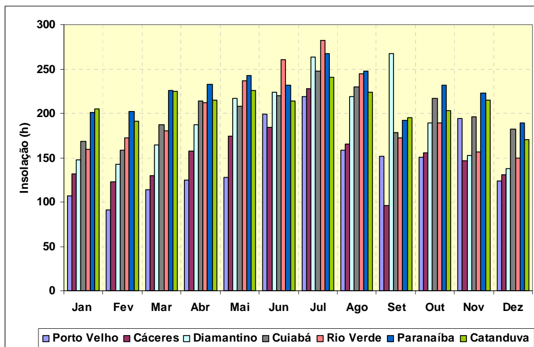
Figura 3.6.3.1-11 – Número de Horas de Insolação Média Mensal ao Longo da All da Linha de Transmissão. Fonte: INMET, 1992.
