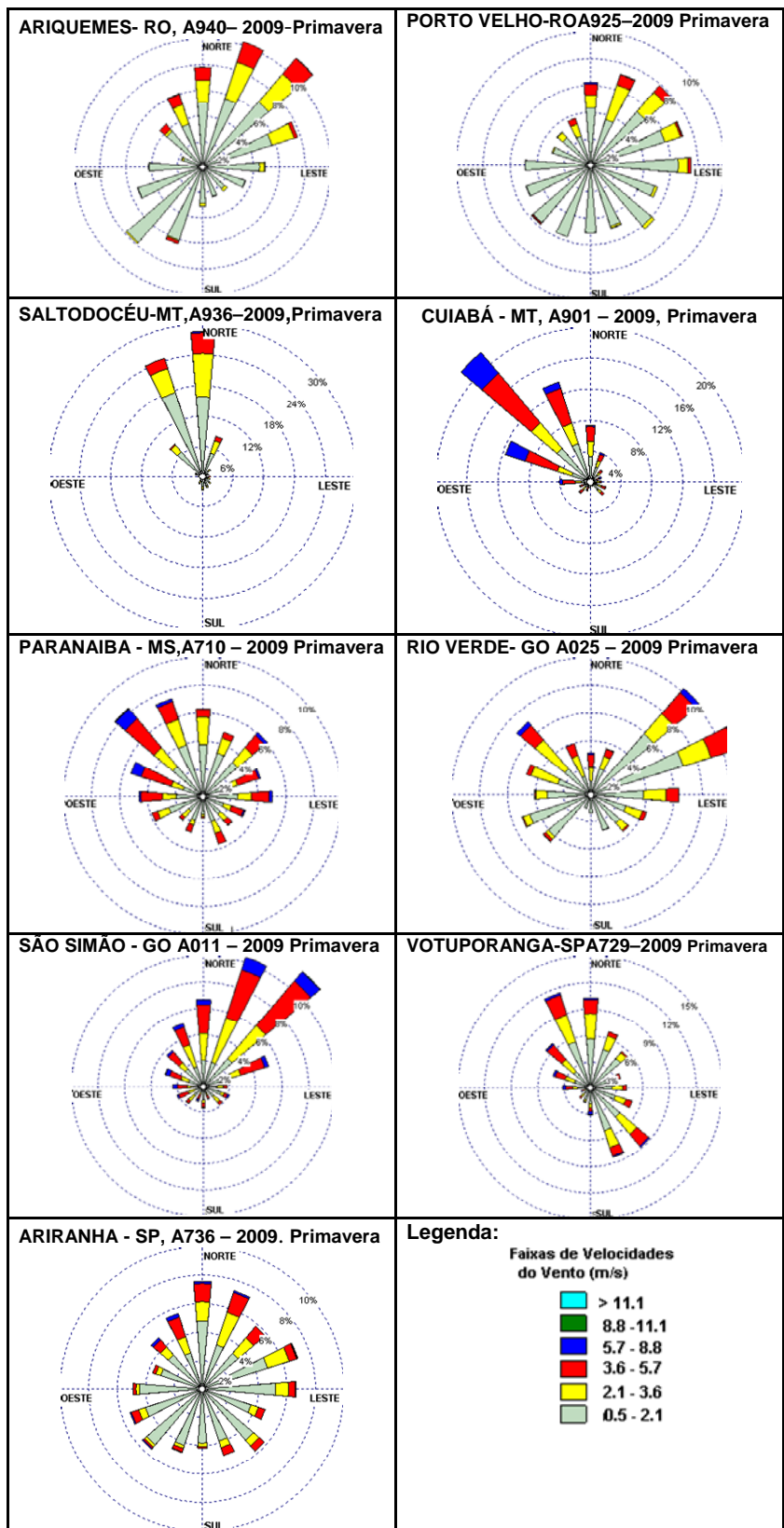
Figura 3.6.3.1-16 – Rosa dos Ventos da Primavera de 2009, ao Longo da AII da Linha de Transmissão. Fonte: (INMET, 2009)
