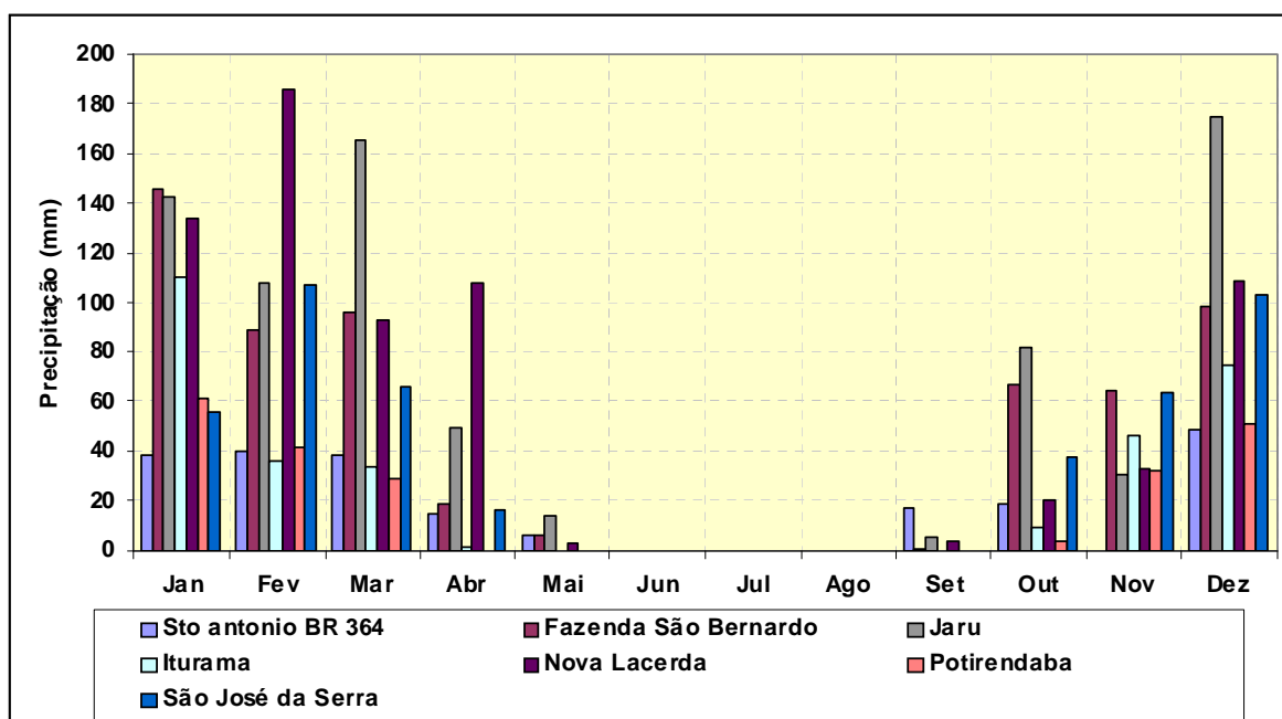
Figura 3.6.3.1-6 – Histograma Comparativo de Precipitações Mínimas Mensais
