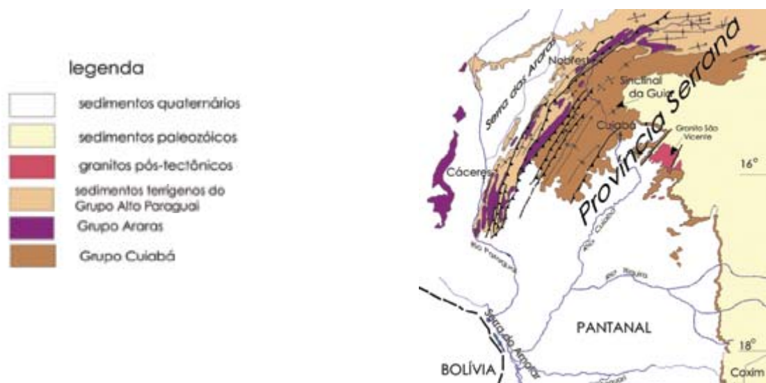
Figura 3.6.3.2-5 – Faixa de dobramentos Paraguai
