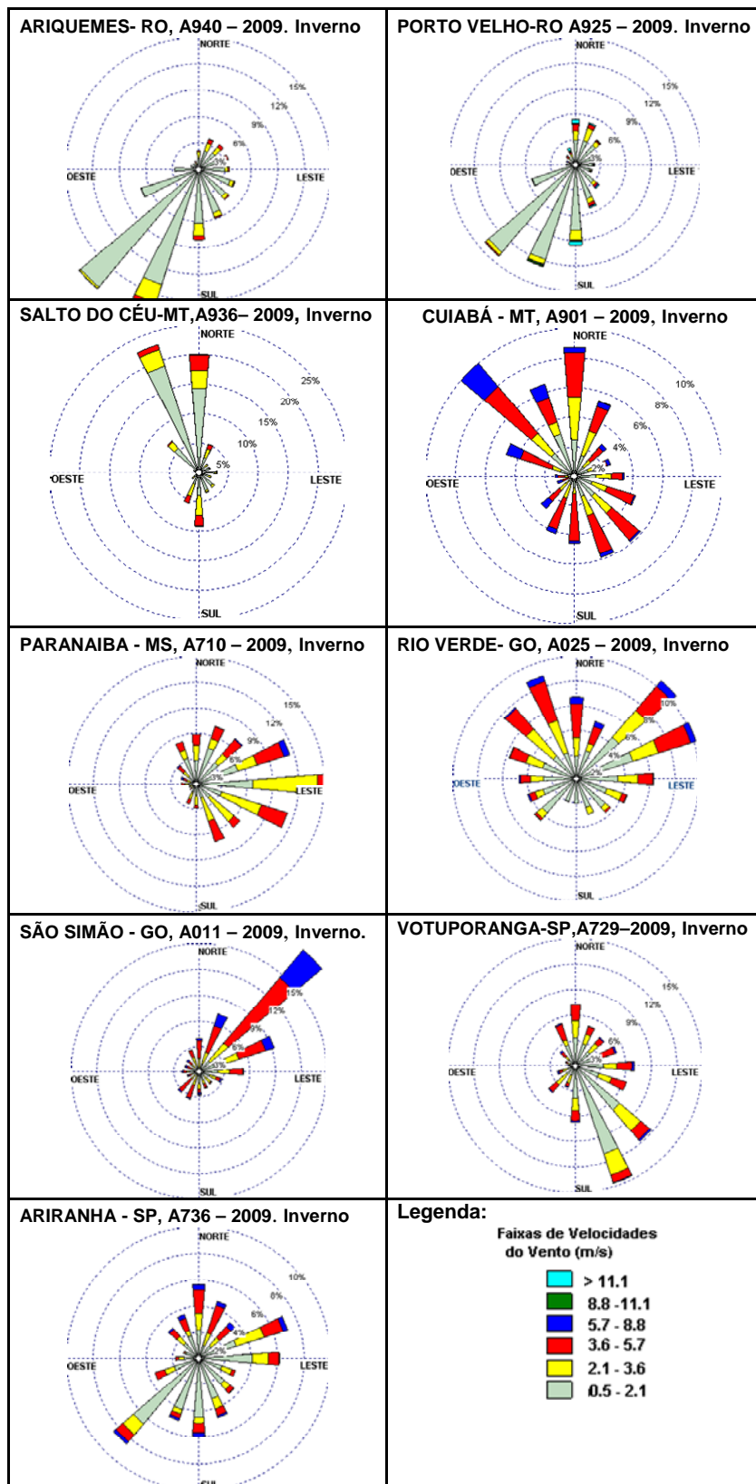
Figura 3.6.3.1-15 – Rosa dos Ventos do Inverno de 2009, ao Longo da AII da Linha de Transmissão. Fonte: (INMET, 2009)
