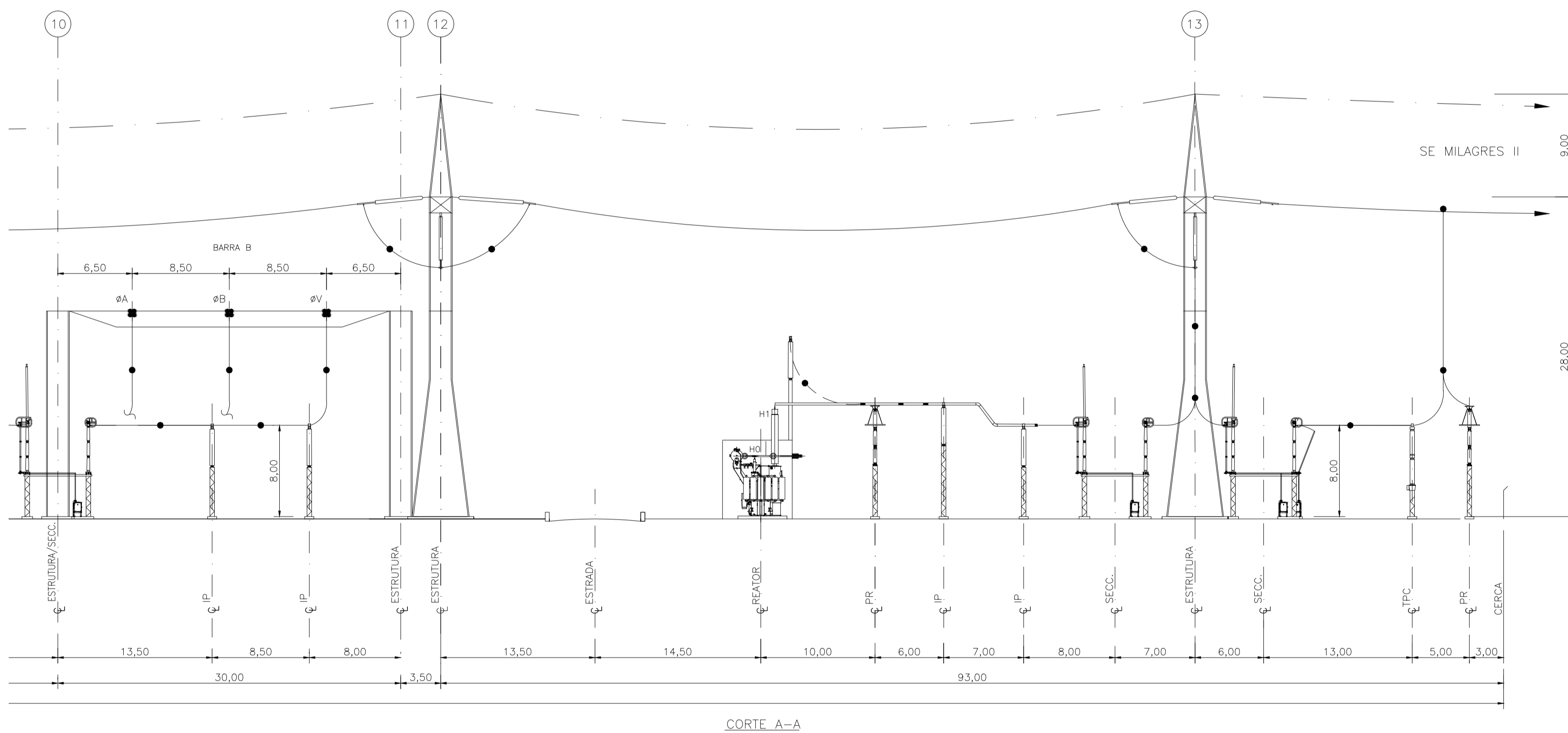
CORTE A-A
