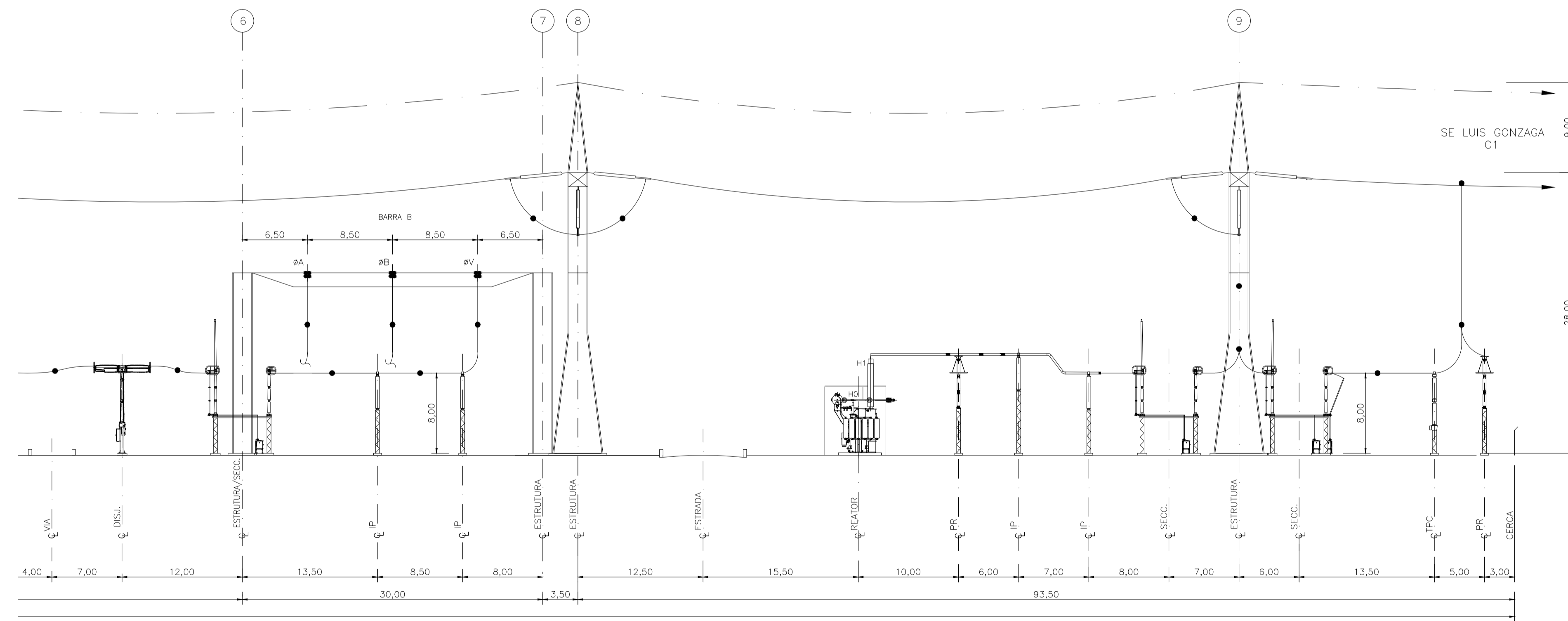
CORTE A-A
