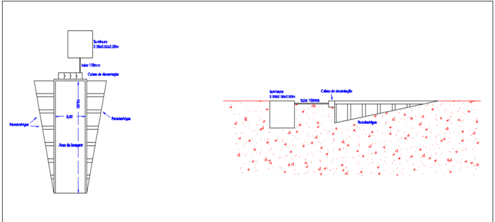
Ilustração 1 - Sistema de separação de resíduos na lavagem do caminhão betoneira.
