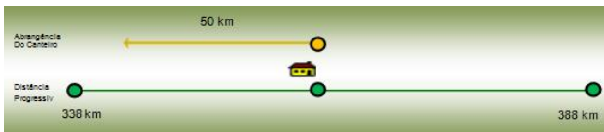
Ilustração 1 - Plano de Ataque e Abrangência para o Canteiro de São João do Piauí 05, para o trecho entre as SEs São João do Piauí – Milagres II
