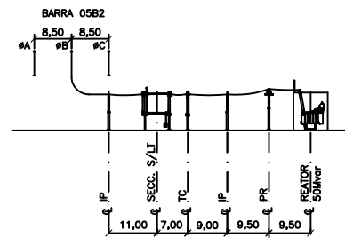
CORTE B-B ESC.: 1:750
