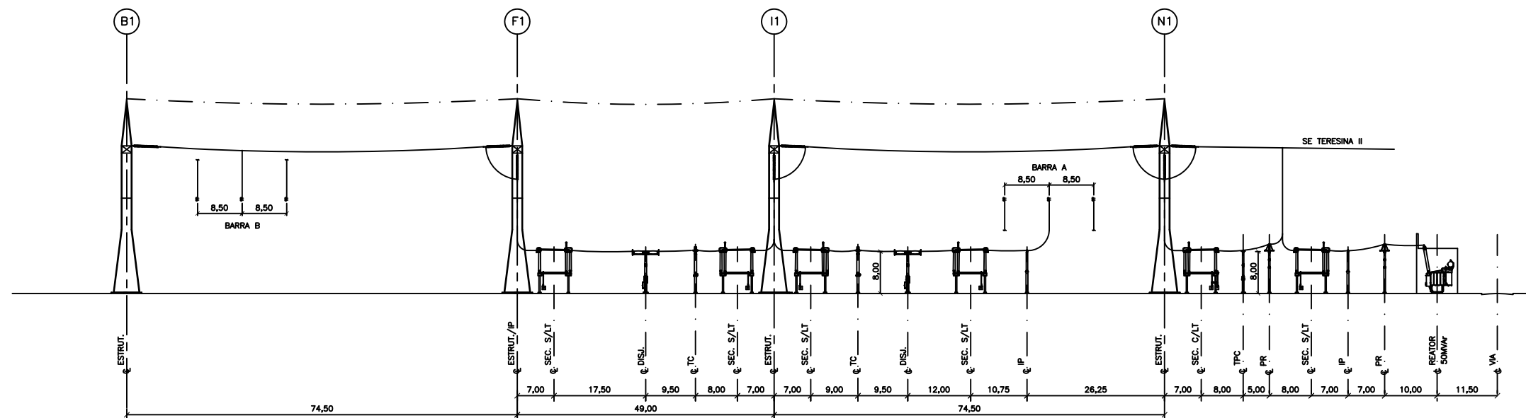
CORTE A-A ESC.: 1:500
