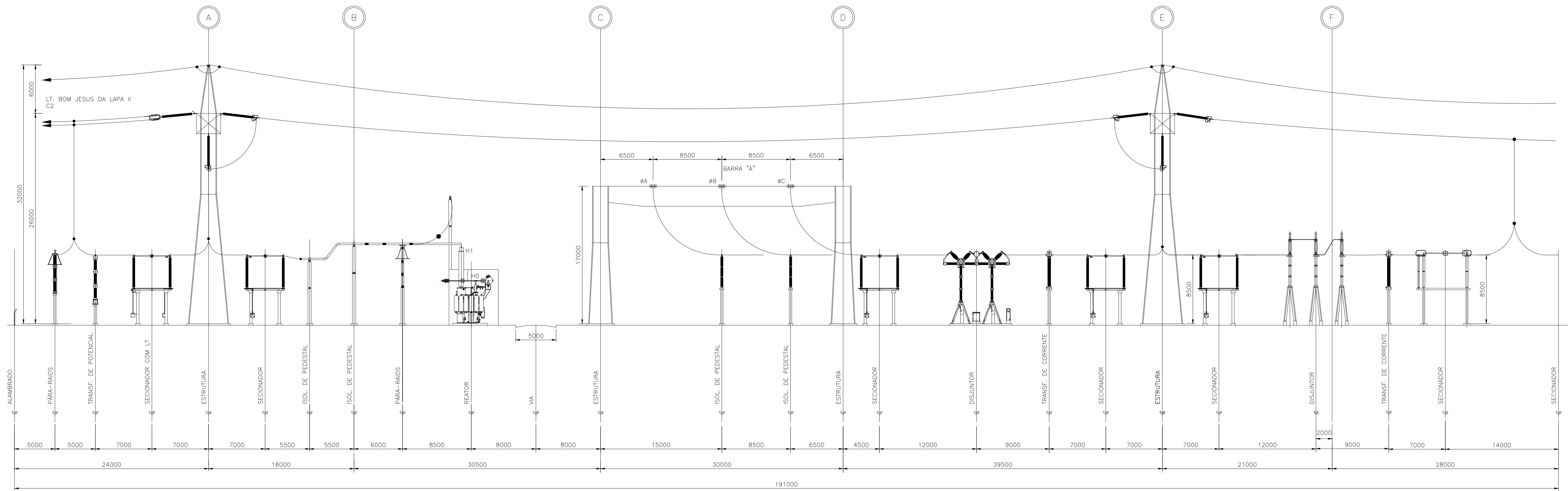
CORTE A-A
