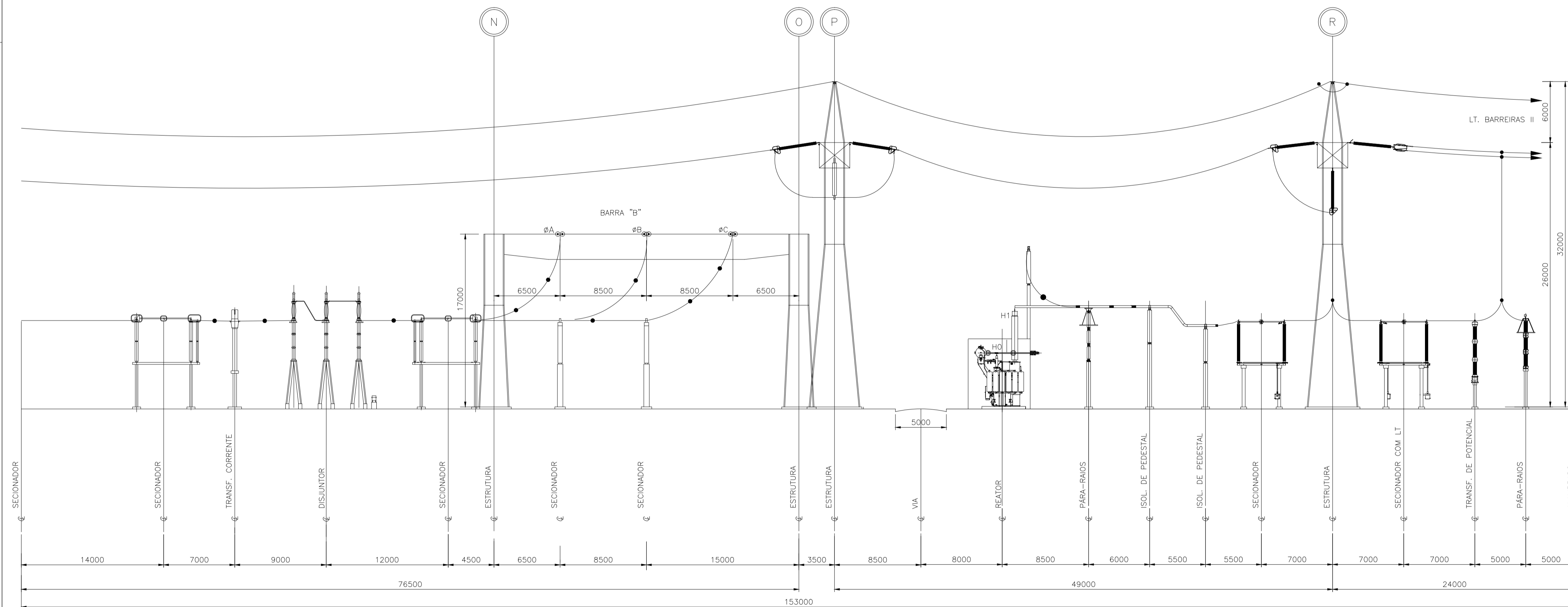
CORTE A-A
