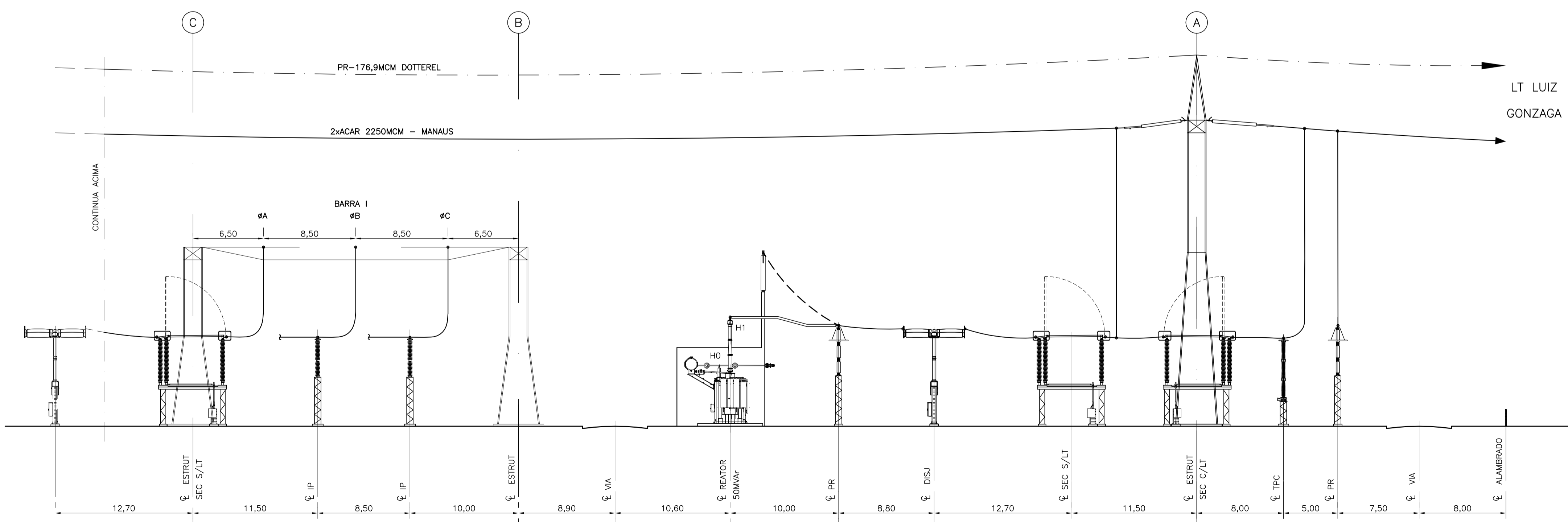
CORTE E-E ESC.: 1:250
