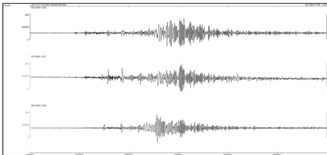
Figura 07: Registro do telessismo na estação XIN 01 ocorrido em Queen Charlotte Islands Region.
