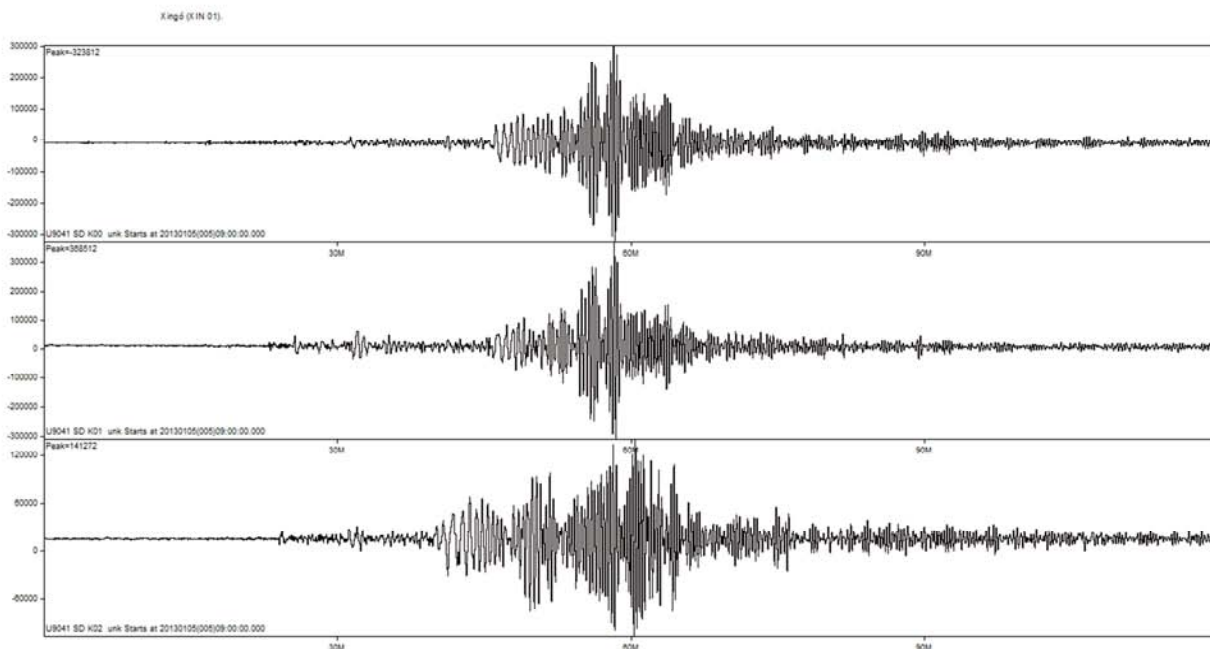
Figura 10: Registro de evento regional ocorrido em Pedra Preta no Estado do Rio Grande do Norte com magnitude de 3,6.
