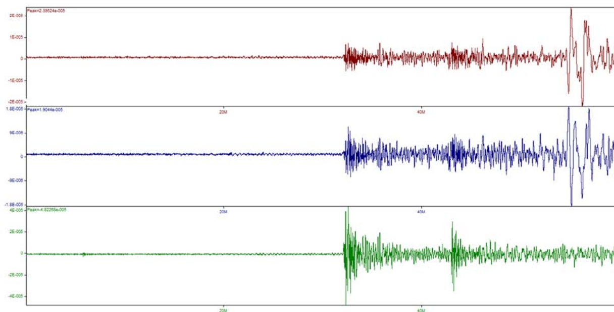
Figura 13: Registro do evento telessismo ocorrido na Ilhas Santa Cruz com magnitude 8,0 m_b , no dia 06.02.13 às 01:32:01 (UTC).
