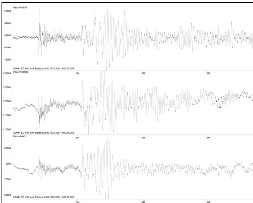
Figura 06: Registro de evento regional artificial na estação XIN 01. Explosão distante cerca de 155 km registrado em 03.11.2012.
