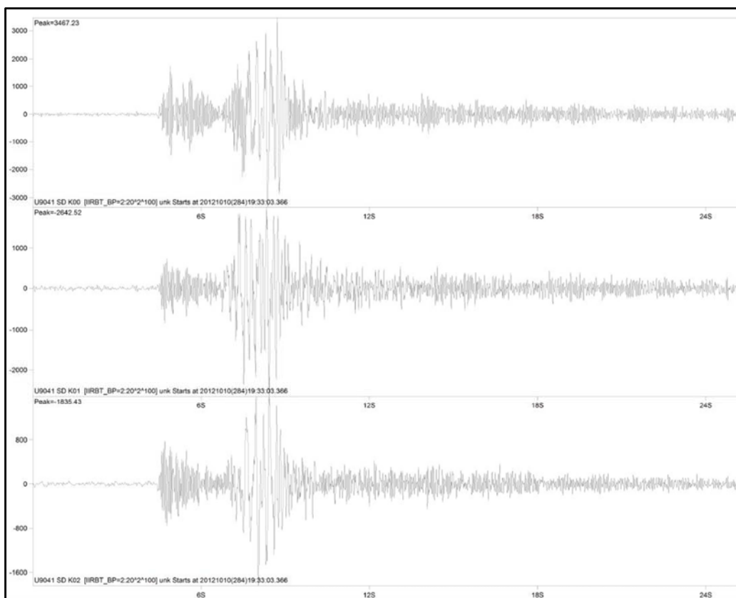
Figura 04: Registro de evento local artificial na estação XIN 01. Explosão distante cerca de 21,57 km registrado em 10.10.2012.
