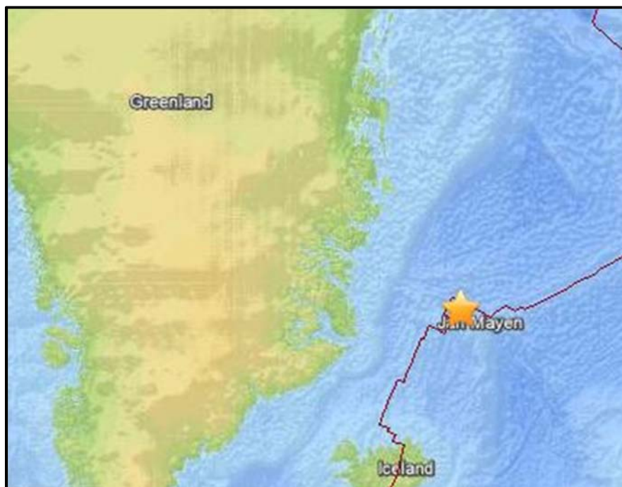
Figura 19: Sismo registrado em Jan Mayen Island com magnitude 6,8 m , pela estação XIN 01 (Fonte: USGS).
