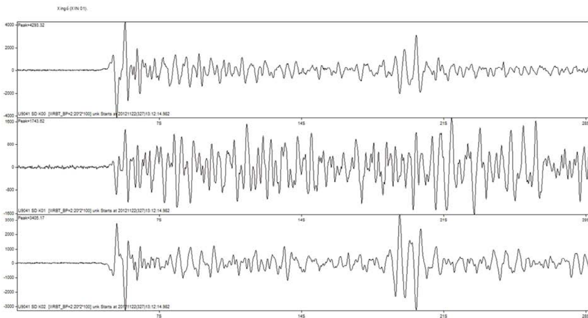
Figura 09: Registro de telessismo SOUTHEASTERN ALASCA com magnitude 7,5 MW.
