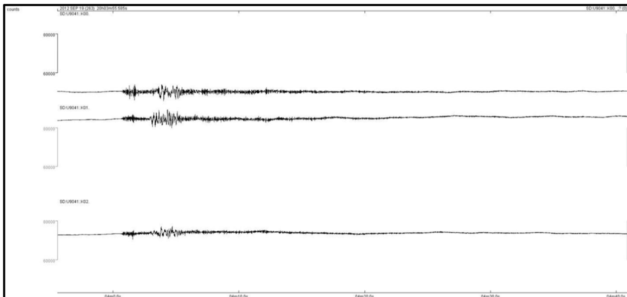
Figura 03: Registro de evento local artificial na estação XIN 01, explosão distante cerca de 21,47 km, ambos registrados em 19.09.2012.
