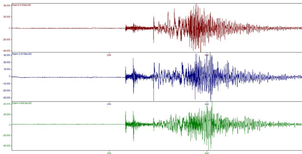
Figura 14: Registro do evento telessismo ocorrido na Colômbia com magnitude 6,9 m_b , no dia 09.02.13 às 14:23:12 (UTC).
