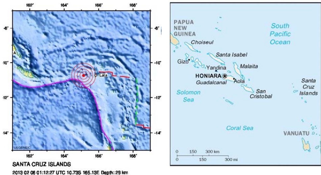
Figura 26: Sismo registrado na Ilha de Santa Cruz no Oceano Pacífico com magnitude 8,0_m pela estação XIN 01 (Fonte: USGS).
