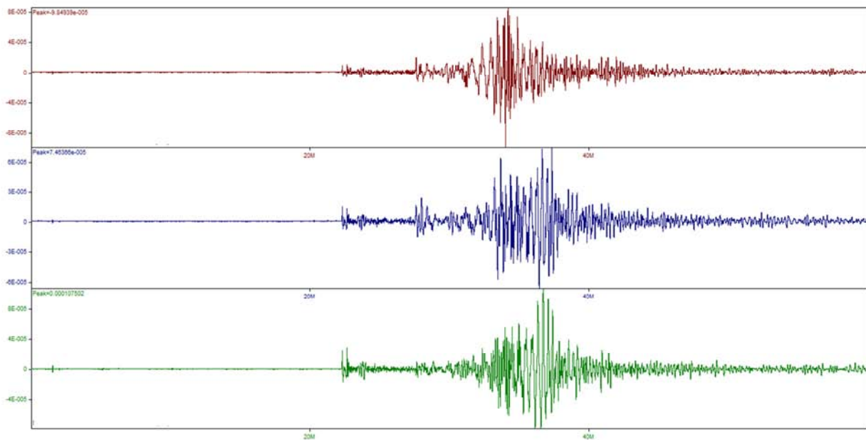
Figura 12: Registro do evento teleseismo ocorrido no deserto do Atacama / Chile com magnitude 6,7 m_b , no dia 30.01.13 às 20:22:10 (UTC).
