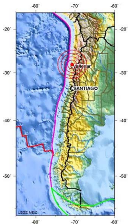
Figura 24: Sismo registrado no deserto do Atacama / Chile com magnitude 6,7m_b pela estação XIN 01 (Fonte: USGS).
