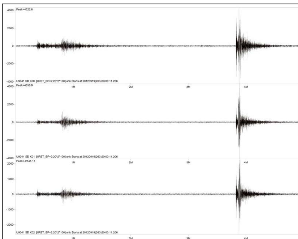
Figura 02: Registro do evento sismográfico ocorrido em São Caetano/PE pela estação XIN 01, com magnitude de 2,2 m_b .
