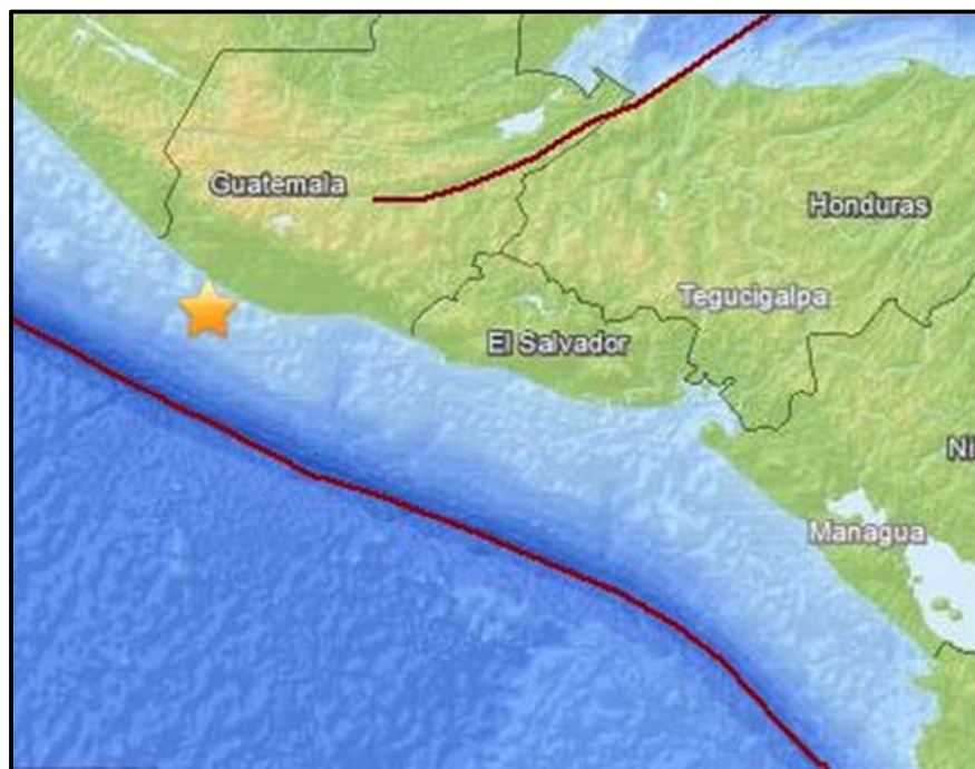
Figura 21: Sismo registrado na região offshore de Guatemala com magnitude 7,4 m_b , pela estação XIN 01 (Fonte: USGS).
