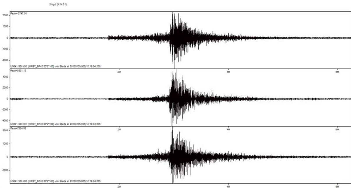
Figura 11: Registro de evento local artificial ocorrido em 09.01.13 às 19:33:54.
