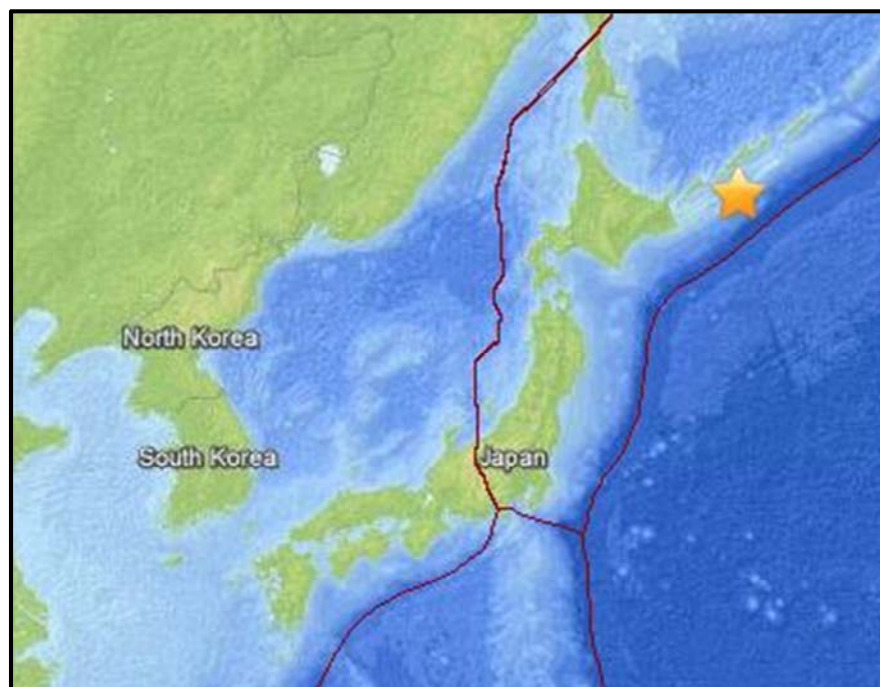
Figura 22: Sismo registrado em Kuril Islands com magnitude 6,4 m_b , pela estação XIN 01 (Fonte: USGS).
