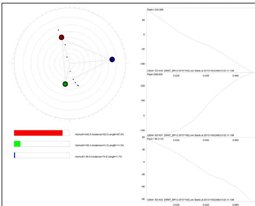
Figura 15: Cálculo da direção do evento regional artificial a partir da estação XIN 01.
