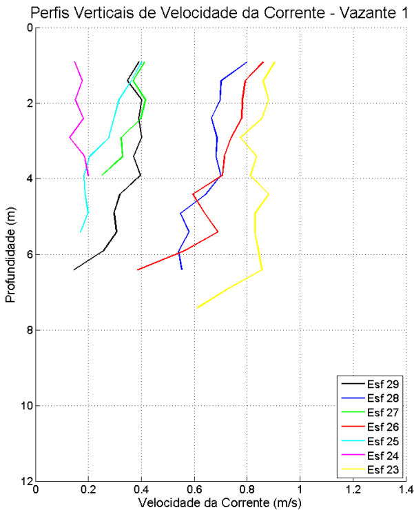
Figura 25: Perfis verticais de velocidade da corrente em período de maré vazante, para cada estação amostral. Campanha 1 – Vazante 1 – data: 09/02/2016.
