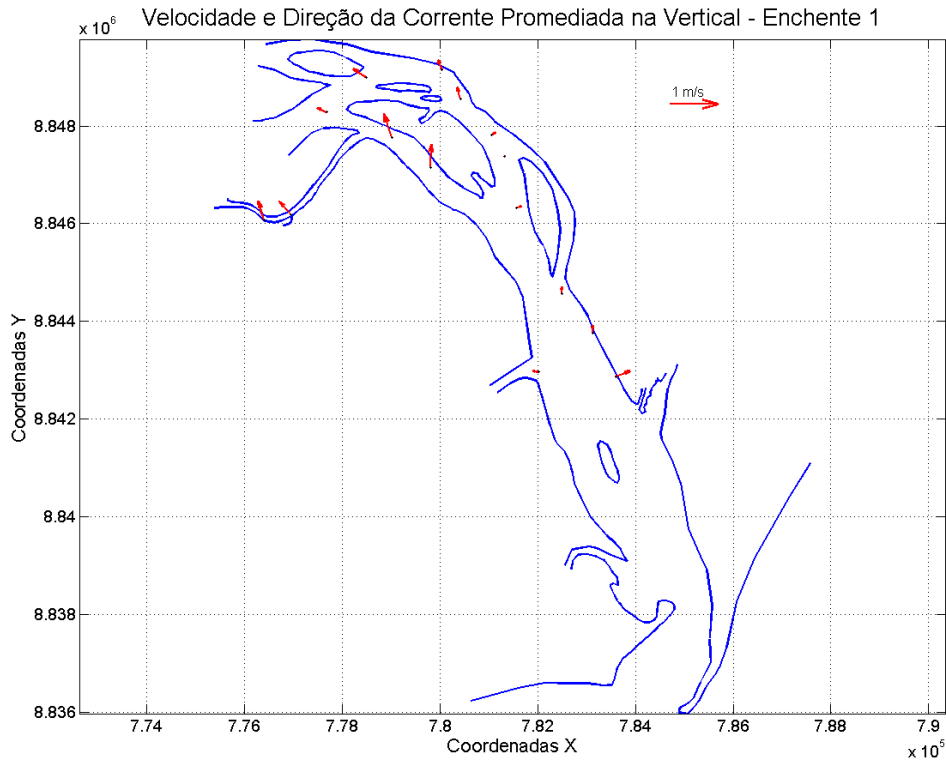
Figura 56: Velocidade e direção da corrente promediada na vertical, em cada estação amostral. Campanha 2 – Enchente 1 – data: 21/02/2016.
