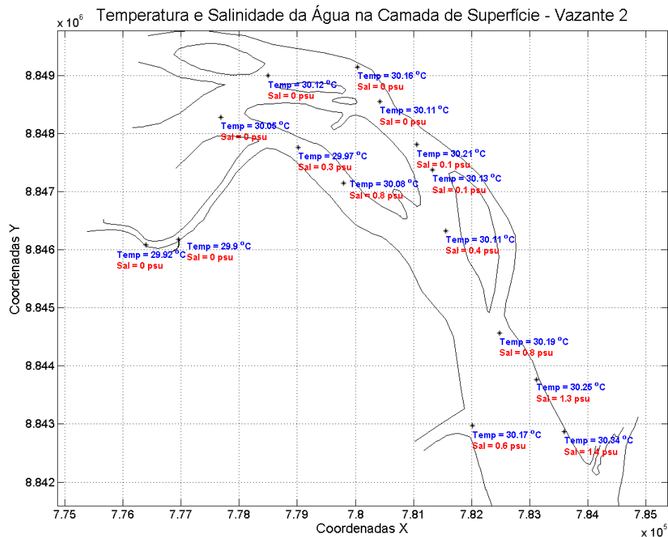
Figura 78: Temperatura e salinidade da água na camada de superfície. Campanha 2 – Vazante 2 – data: 22/02/2016. Resolução CONAMA 357/2005 (I - águas doces: águas com salinidade igual ou inferior a 0,5 ‰).
