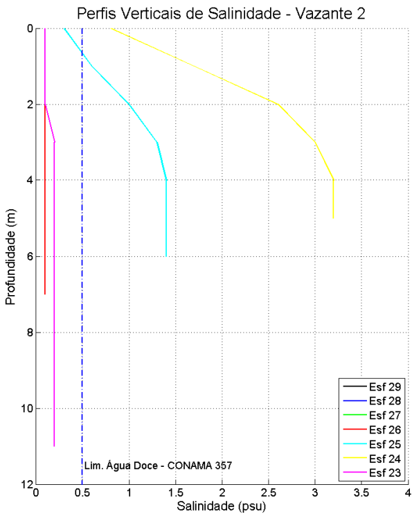
Figura 43: Perfis verticais de salinidade da água em período de maré vazante, para cada estação amostral. Campanha 1 – Vazante 2 – data: 10/02/2016. Resolução CONAMA 357/2005 (I - águas doces: águas com salinidade igual ou inferior a 0,5 ‰).
