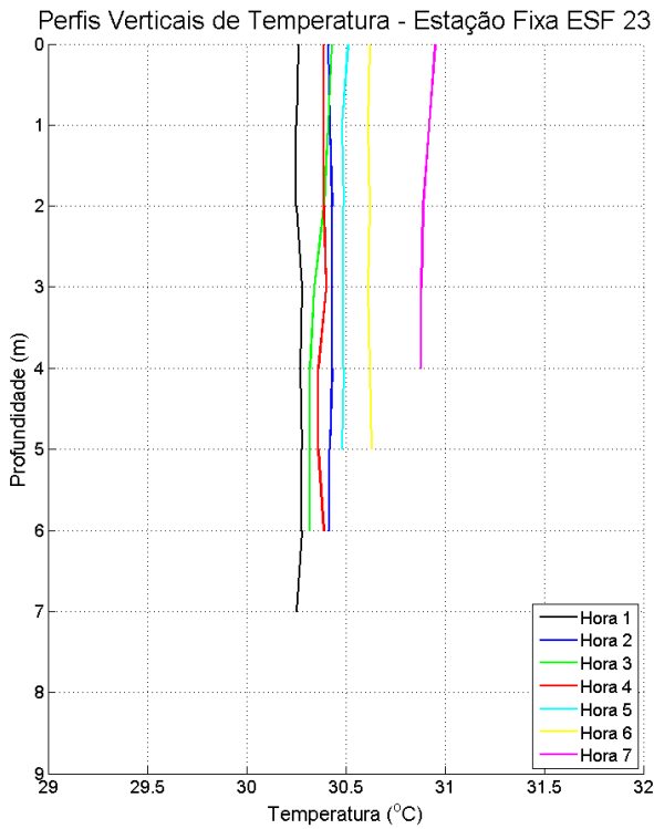
Figura 97: Perfis verticais de temperatura para a estação fixa ESF_23. Campanha 2 – 12 horas – data: 24/02/2016.
