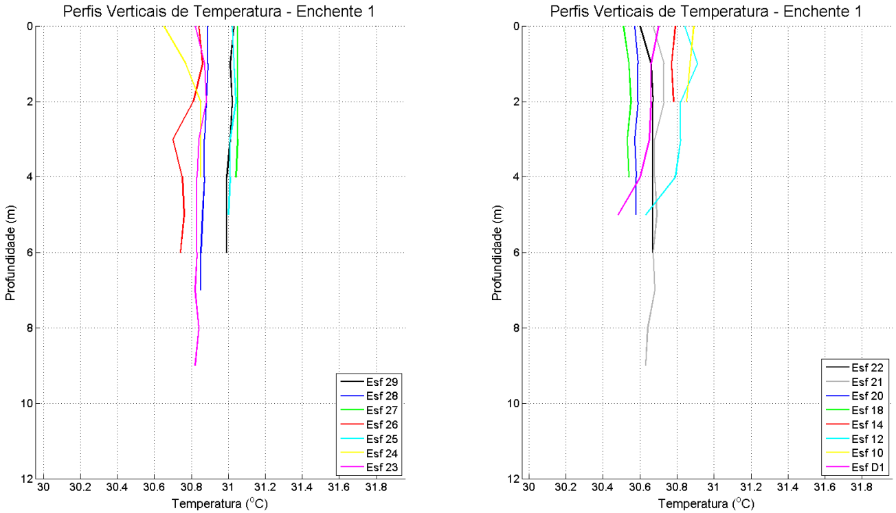
Figura 32: Perfis verticais de temperatura da água em período de maré enchente, para cada estação amostral. Campanha 1 – Enchente 1 – data: 09/02/2016.
