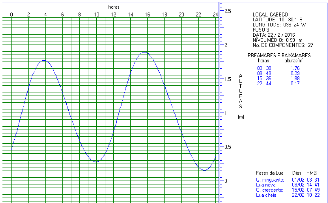
Figura 19. Previsão de maré para o dia 22/02/2016 (campanha 2), para a localidade de Cabeço, localizada na foz do Rio São Francisco.
