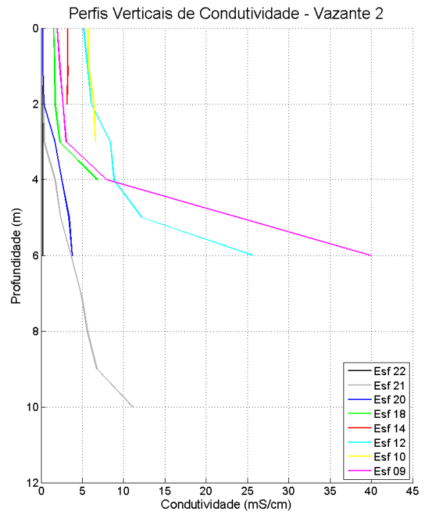
Figura 39: Perfis verticais de condutividade da água em período de maré vazante, para cada estação amostral. Campanha 1 – Vazante 2 – data: 10/02/2016.
