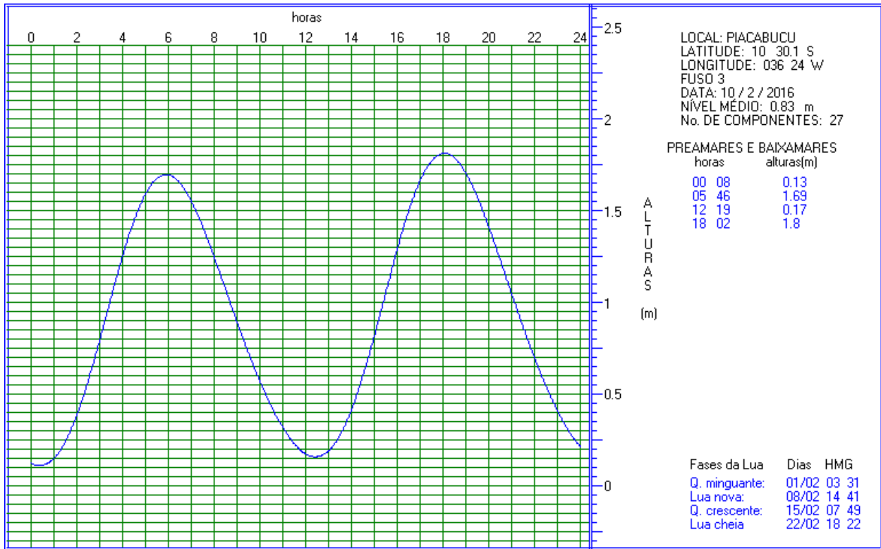
Figura 10. Previsão de maré para o dia 10/02/2016 (campanha 1), para a localidade de Piaçabuçu, localizada na margem esquerda do Rio São Francisco.
