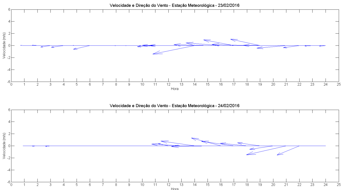
Figura 103: Diagrama stick plot dos dados de ventos medidos no dia 23/02/2016 (painel superior) e 24/02/2016 (painel inferior).
