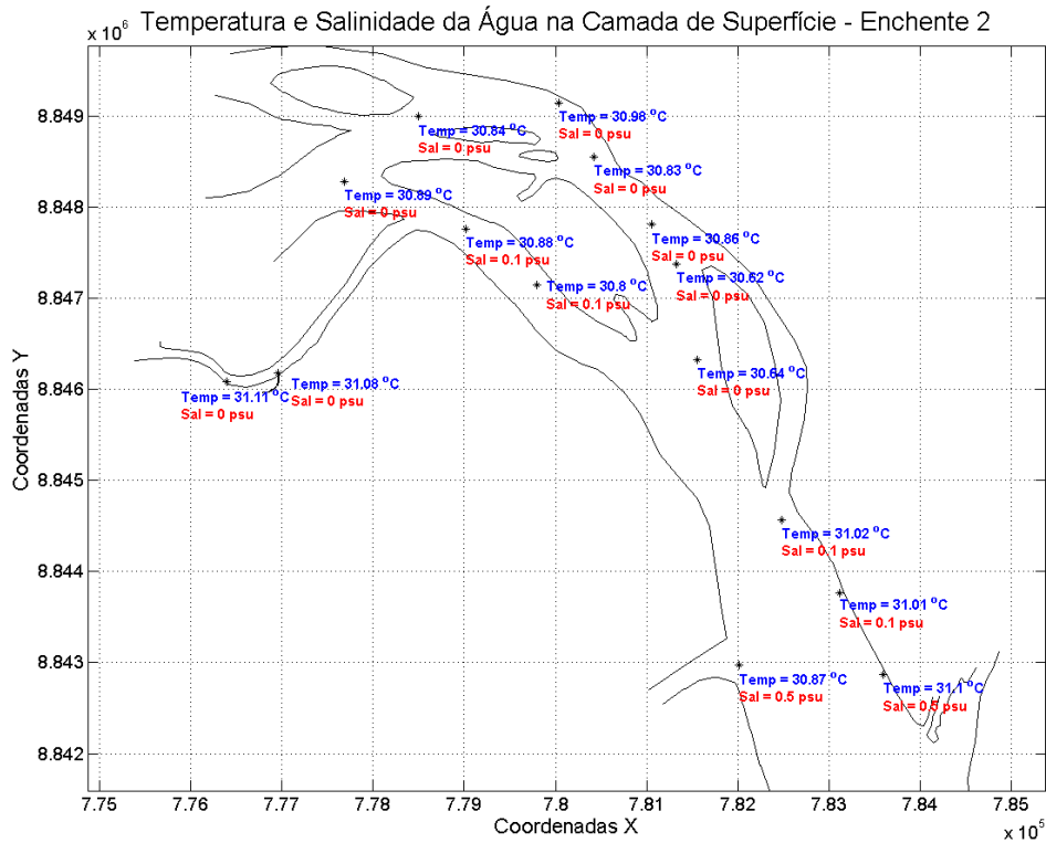
Figura 48: Temperatura e salinidade da água na camada de superfície. Campanha 1 – Enchente 2 – data: 10/02/2016 . Resolução CONAMA 357/2005 (I - águas doces: águas com salinidade igual ou inferior a 0,5 ‰).
