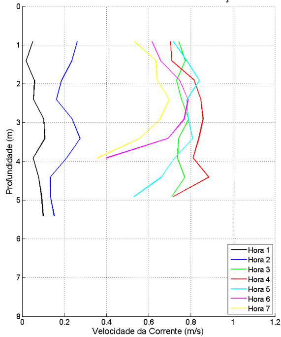
Figura 95: Perfis verticais de velocidade da corrente para a estação fixa ESF_23. Campanha 2 – 12 horas – data: 24/02/2016.
