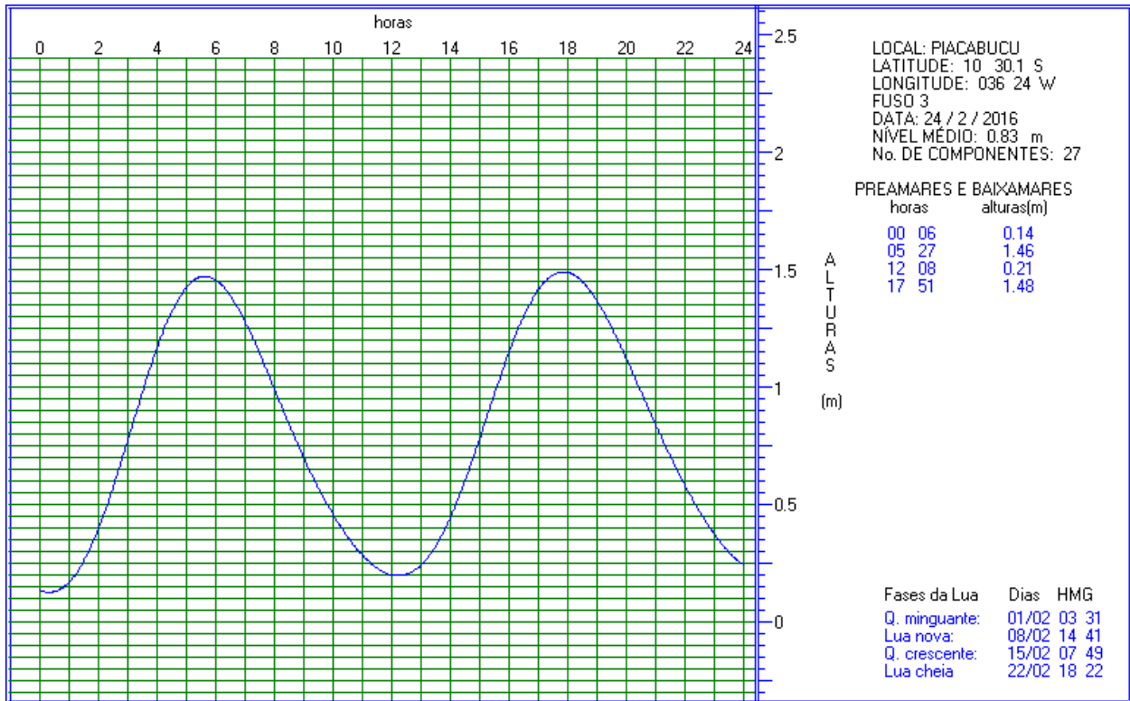
Figura 22: Previsão de maré para o dia 24/02/2016 (campanha 2), para a localidade de Piaçabuçu, localizada na margem esquerda do Rio São Francisco.
