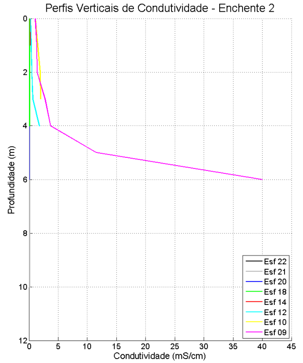
Figura 38: Perfis verticais de condutividade da água em período de maré enchente, para cada estação amostral. Campanha 1 – Enchente 2 – data: 10/02/2016 .
