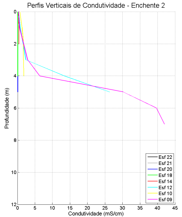
Figura 66: Perfis verticais de condutividade da água em período de maré enchente, para cada estação amostral. Campanha 2 – Enchente 2 – data: 22/02/2016.
