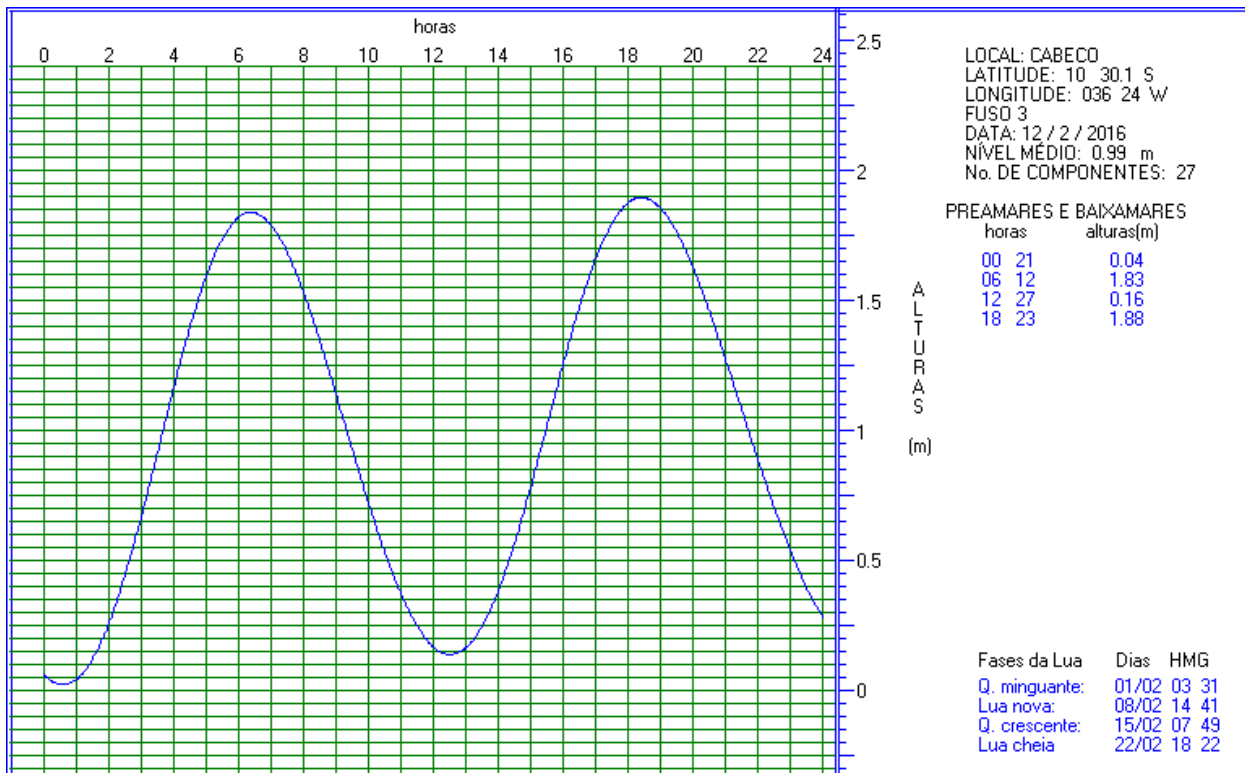
Figura 15. Previsão de maré para o dia 12/02/2016 (campanha 1), para a localidade de Cabeço, localizada na foz do Rio São Francisco.
