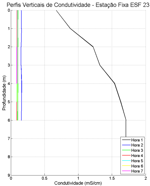
Figura 98: Perfis verticais de condutividade para a estação fixa ESF_23. Campanha 2 – 12 horas – data: 24/02/2016.
