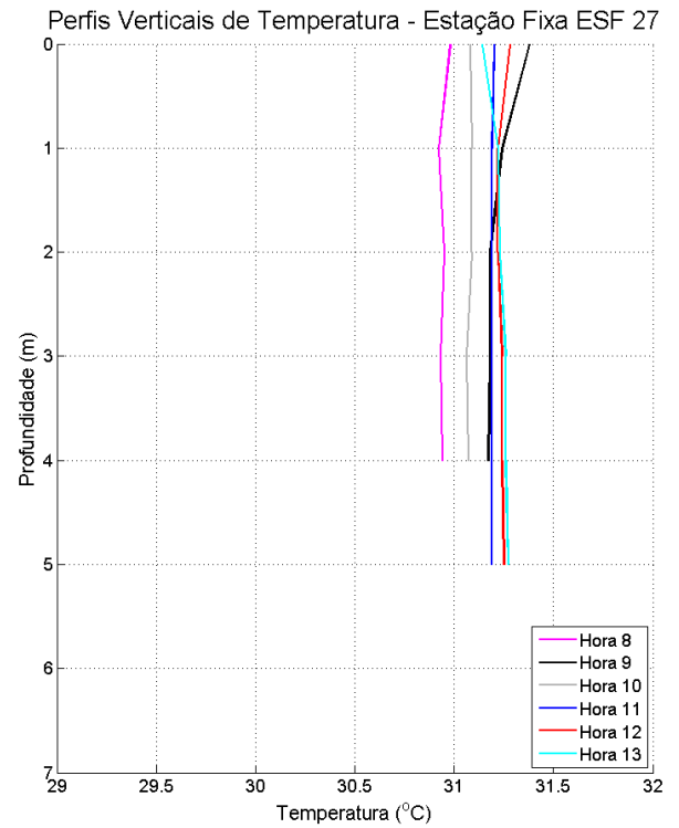
Figura 82: Perfis verticais de temperatura para a estação fixa ESF_27. Campanha 1 – 12 horas – data: 11/02/2016.
