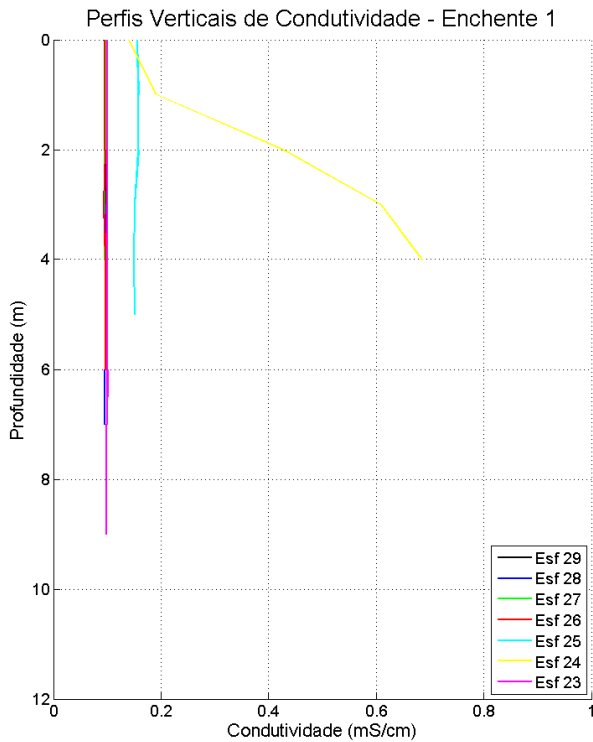
Figura 36: Perfis verticais de condutividade da água em período de maré enchente, para cada estação amostral. Campanha 1 – Enchente 1 – data: 09/02/2016.
