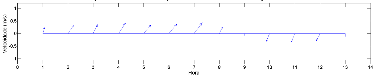
Figura 91: Diagrama “stick plot” das correntes em superfície (painel superior) e fundo (painel inferior), para a estação fixa ESF_27. Campanha 2 – 12 horas – data: 23/02/2016.
