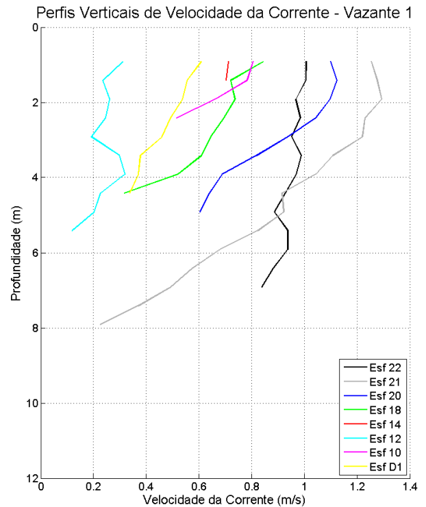
Figura 25: Perfis verticais de velocidade da corrente em período de maré vazante, para cada estação amostral. Campanha 1 – Vazante 1 – data: 09/02/2016.
