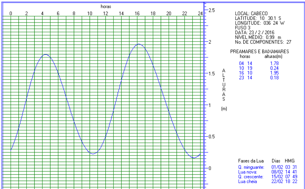
Figura 21. Previsão de maré para o dia 23/02/2016 (campanha 2), para a localidade de Cabeço, localizada na foz do Rio São Francisco.
