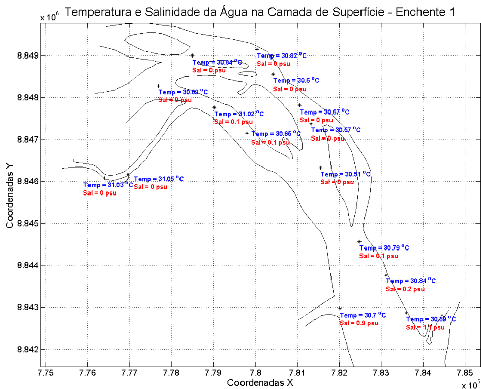
Figura 44: Temperatura e salinidade da água na camada de superfície. Campanha 1 – Enchente 1 – data: 09/02/2016. Resolução CONAMA 357/2005 (I - águas doces: águas com salinidade igual ou inferior a 0,5 ‰).
