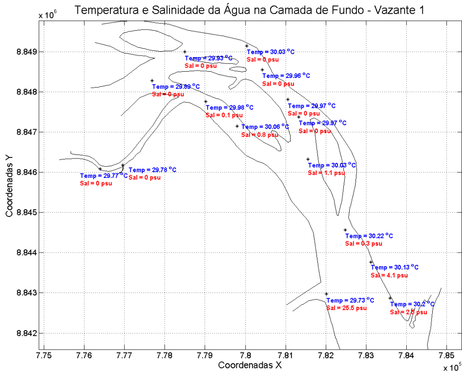
Figura 75: Temperatura e salinidade da água na camada de fundo. Campanha 2 – Vazante 1 – data: 21/02/2016. Resolução CONAMA 357/2005 (I - águas doces: águas com salinidade igual ou inferior a 0,5 ‰).
