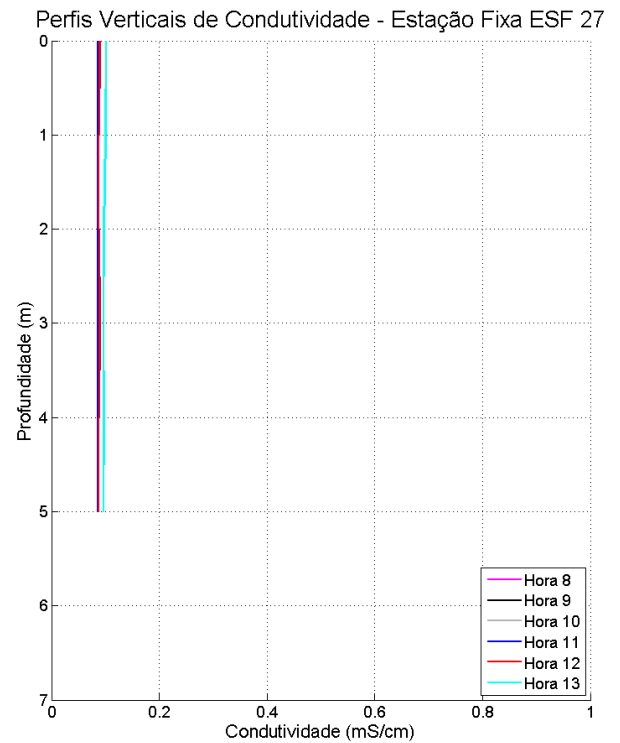
Figura 83: Perfis verticais de condutividade para a estação fixa ESF_27. Campanha 1 – 12 horas – data: 11/02/2016.
