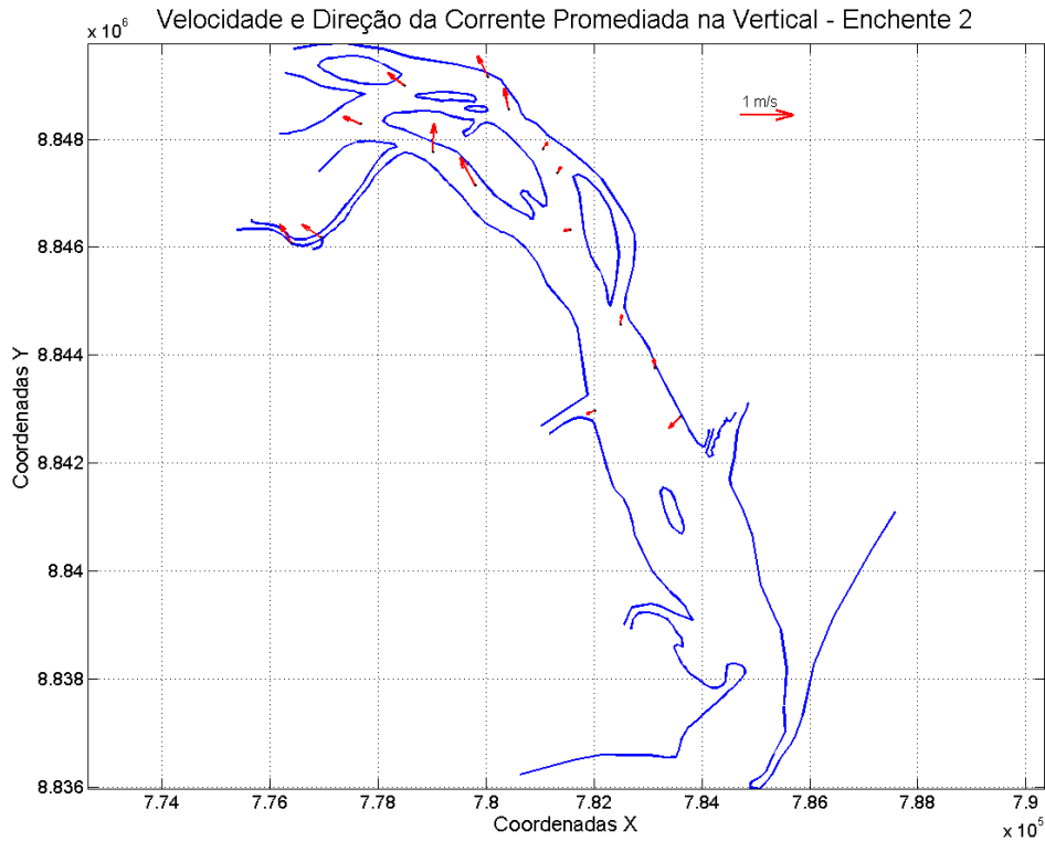
Figura 58: Velocidade e direção da corrente promediada na vertical, em cada estação amostral. Campanha 2 – Enchente 2 – data: 22/02/2016.
