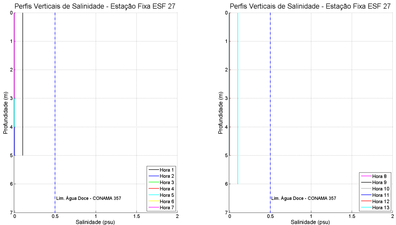
Figura 94: Perfis verticais de salinidade para a estação fixa ESF_27. Campanha 2 – 12 horas – data: 23/02/2016. Resolução CONAMA 357/2005 (I - águas doces: águas com salinidade igual ou inferior a 0,5 ‰).
