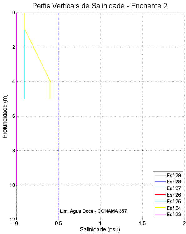
Figura 42: Perfis verticais de salinidade da água em período de maré enchente, para cada estação amostral. Campanha 1 – Enchente 2 – data: 10/02/2016 . Resolução CONAMA 357/2005 (I - águas doces: águas com salinidade igual ou inferior a 0,5 ‰).
