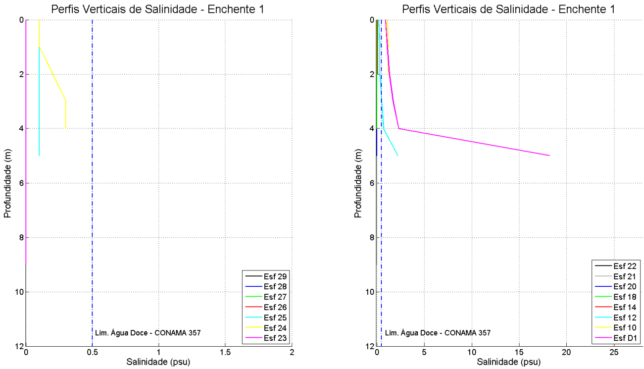
Figura 40: Perfis verticais de salinidade da água em período de maré enchente, para cada estação amostral. Campanha 1 – Enchente 1 – data: 09/02/2016. Resolução CONAMA 357/2005 (I - águas doces: águas com salinidade igual ou inferior a 0,5 ‰).
