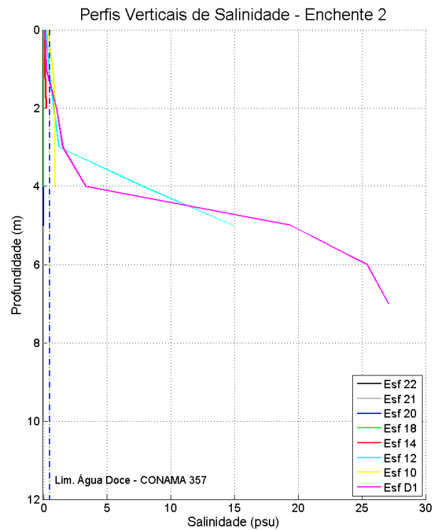
Figura 70: Perfis verticais de salinidade da água em período de maré enchente, para cada estação amostral. Campanha 2 – Enchente 2 – data: 22/02/2016. Resolução CONAMA 357/2005 (I - águas doces: águas com salinidade igual ou inferior a 0,5 ‰).
