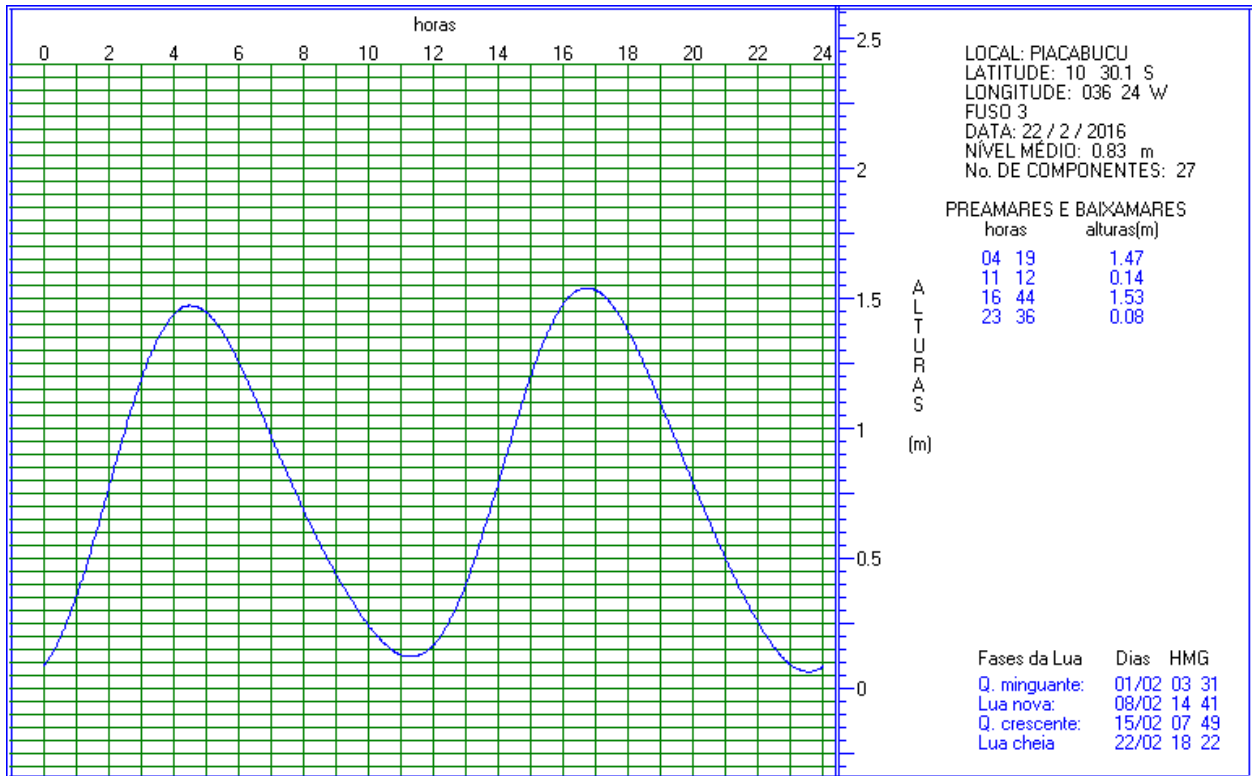
Figura 18. Previsão de maré para o dia 22/02/2016 (campanha 2), para a localidade de Piaçabuçu, localizada na margem esquerda do Rio São Francisco.
