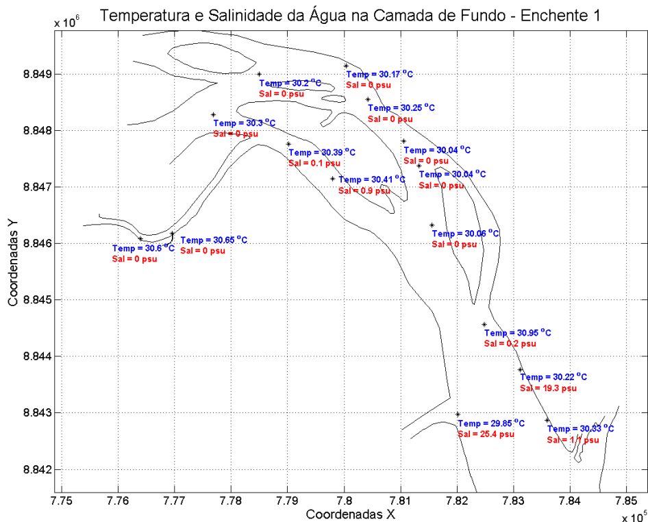
Figura 73: Temperatura e salinidade da água na camada de fundo. Campanha 2 – Enchente 1 – data: 21/02/2016. Resolução CONAMA 357/2005 (I - águas doces: águas com salinidade igual ou inferior a 0,5 ‰).
