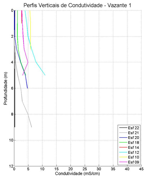
Figura 37: Perfis verticais de condutividade da água em período de maré vazante, para cada estação amostral. Campanha 1 – Vazante 1 – data: 09/02/2016.
