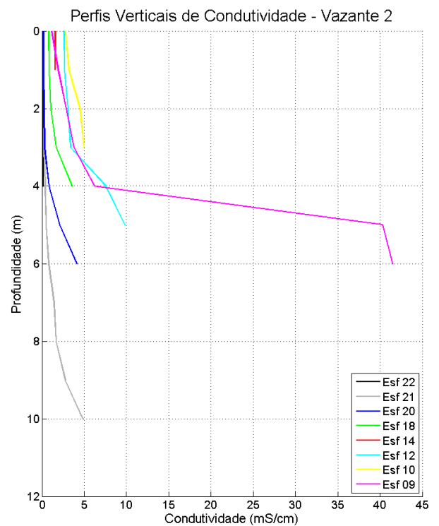
Figura 67: Perfis verticais de condutividade da água em período de maré vazante, para cada estação amostral. Campanha 2 – Vazante 2 – data: 22/02/2016.
