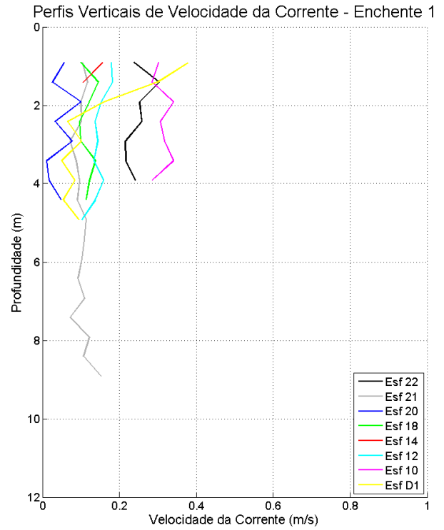
Figura 52: Perfis verticais de velocidade da corrente em período de maré enchente, para cada estação amostral. Campanha 2 – Enchente 1 – data: 21/02/2016.
