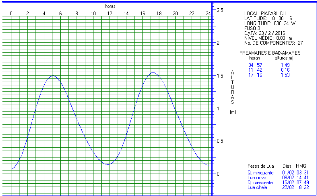
Figura 20. Previsão de maré para o dia 23/02/2016 (campanha 2), para a localidade de Piaçabuçu, localizada na margem esquerda do Rio São Francisco.
