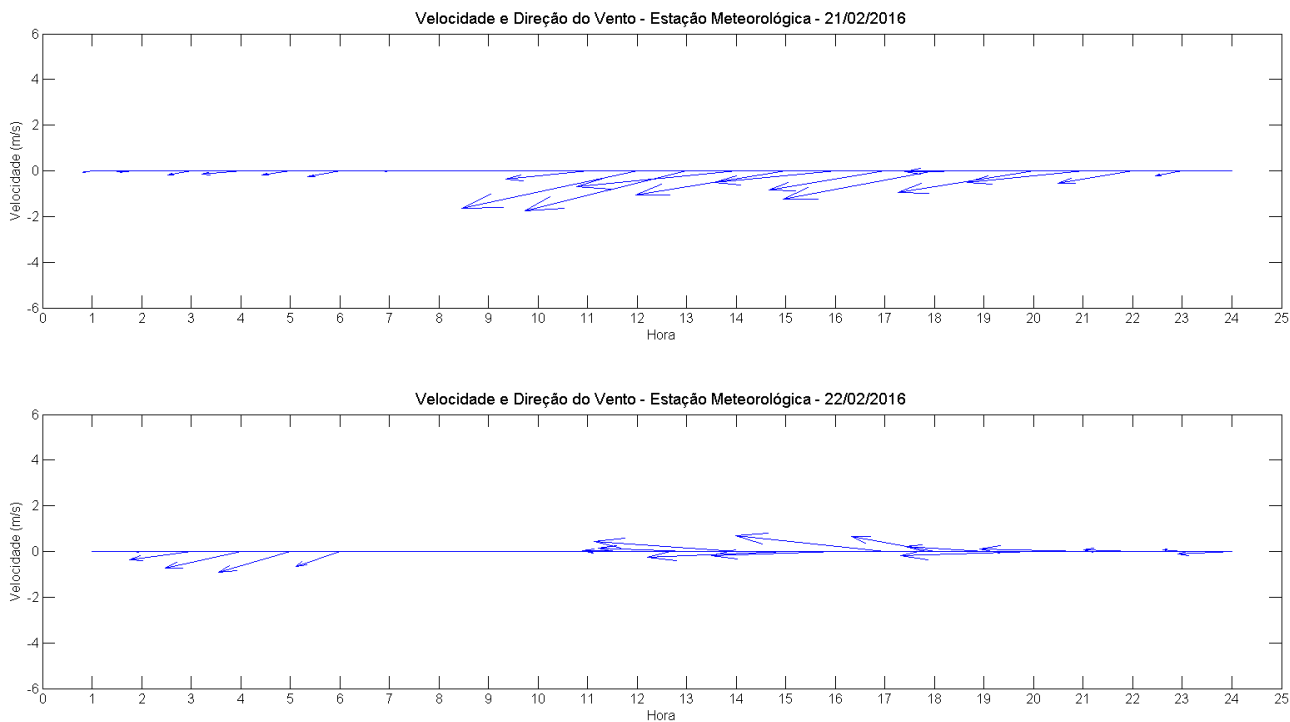
Figura 102: Diagrama stick plot dos dados de ventos medidos no dia 21/02/2016 (painel superior) e 22/02/2016 (painel inferior).
