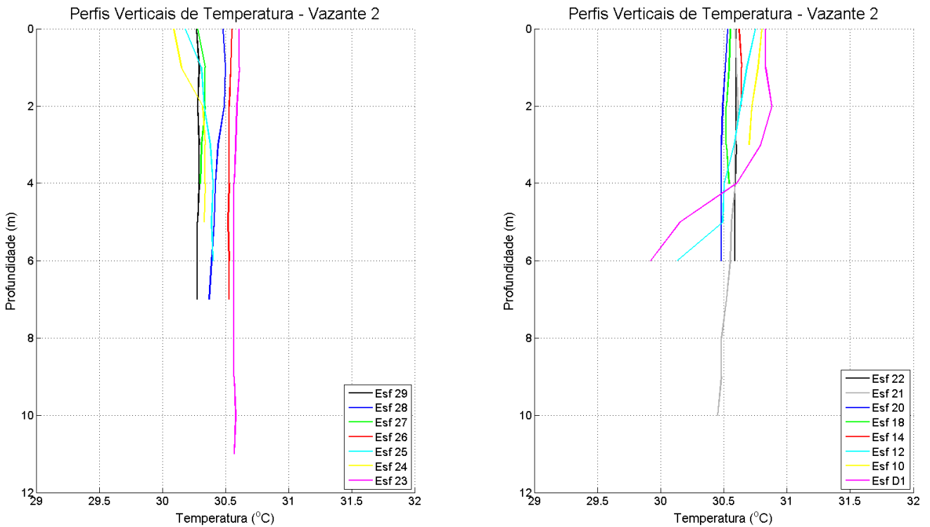
Figura 35: Perfis verticais de temperatura da água em período de maré vazante, para cada estação amostral. Campanha 1 – Vazante 2 – data: 10/02/2016.
