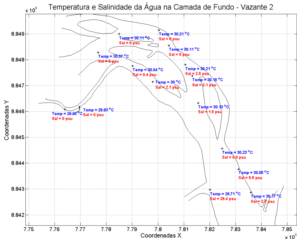
Figura 79: Temperatura e salinidade da água na camada de fundo. Campanha 2 – Vazante 2 – data: 22/02/2016. Resolução CONAMA 357/2005 (I - águas doces: águas com salinidade igual ou inferior a 0,5 ‰).
