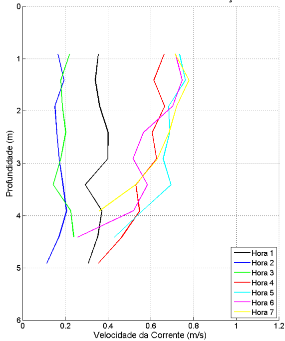
Figura 80: Perfis verticais de velocidade da corrente para a estação fixa ESF_27. Campanha 1 – 12 horas – data: 11/02/2016.
