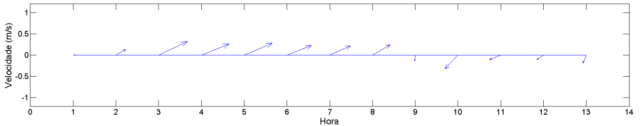
Varição na Velocidade e Direção da Corrente em Superfície - Estação Fixa ESF 23
