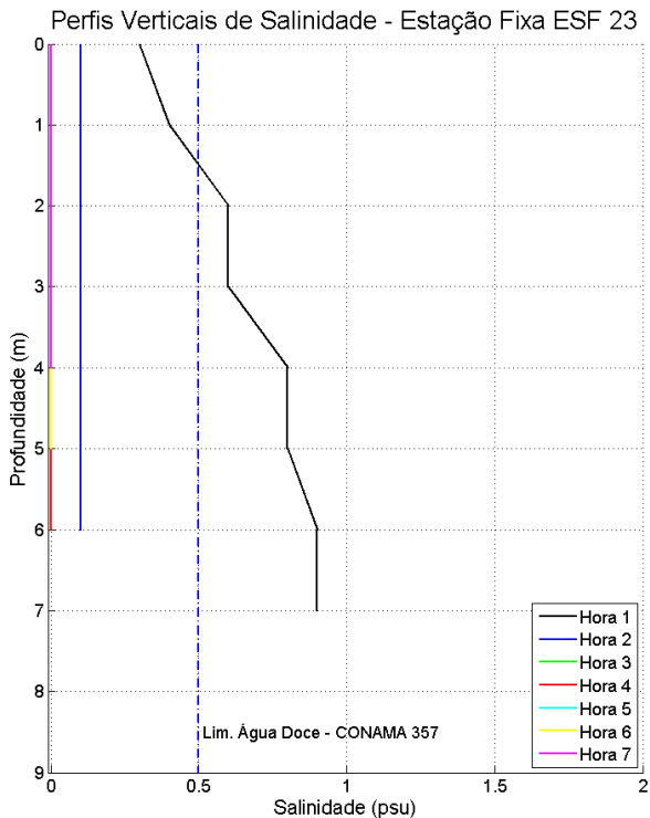
Figura 99: Perfis verticais de salinidade para a estação fixa ESF_23. Campanha 2 – 12 horas – data: 24/02/2016. Resolução CONAMA 357/2005 (I - águas doces: águas com salinidade igual ou inferior a 0,5 ‰).
