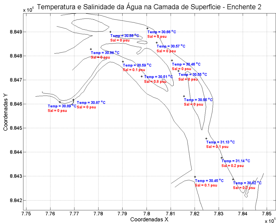
Figura 76: Temperatura e salinidade da água na camada de superfície. Campanha 2 – Enchente 2 – data: 22/02/2016. Resolução CONAMA 357/2005 (I - águas doces: águas com salinidade igual ou inferior a 0,5 ‰).
