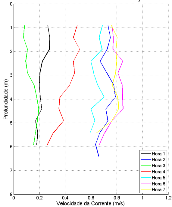
Figura 85: Perfis verticais de velocidade da corrente para a estação fixa ESF_23. Campanha 1 – 12 horas – data: 12/02/2016.
