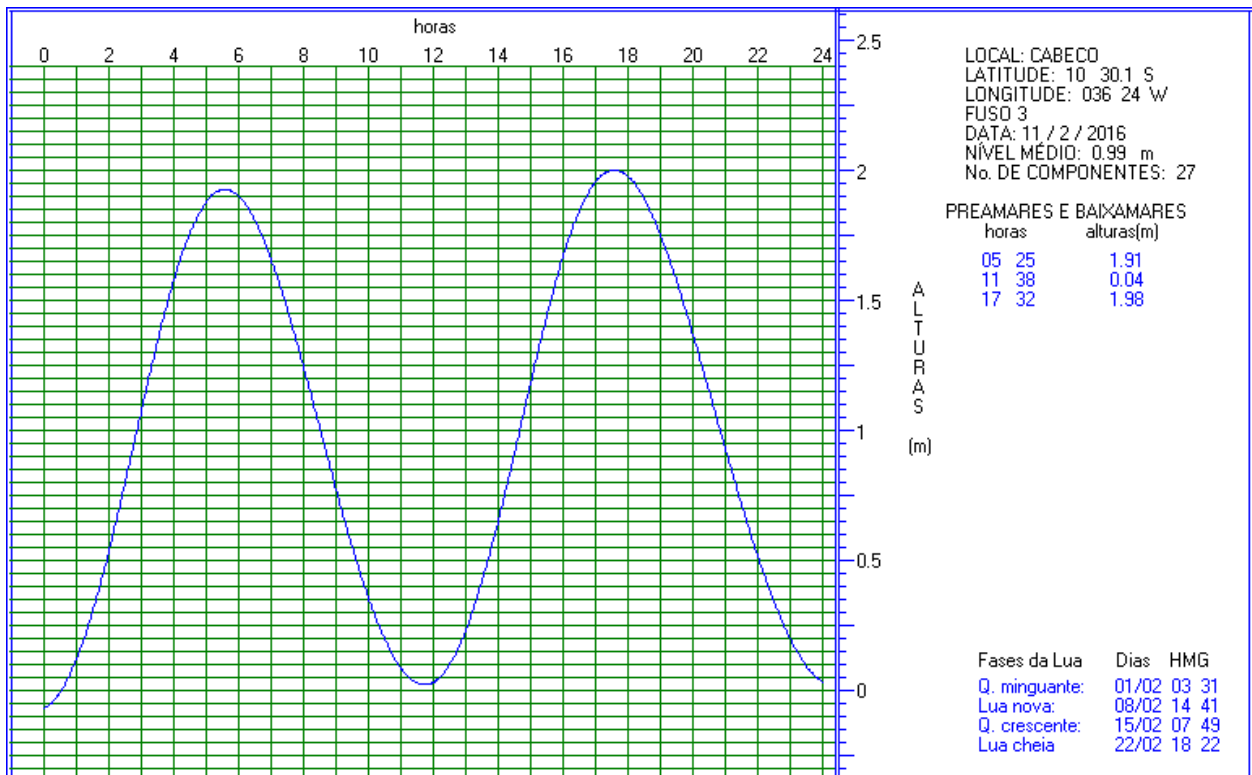
Figura 13. Previsão de maré para o dia 11/02/2016 (campanha 1), para a localidade de Cabeço, localizada na foz do Rio São Francisco.
