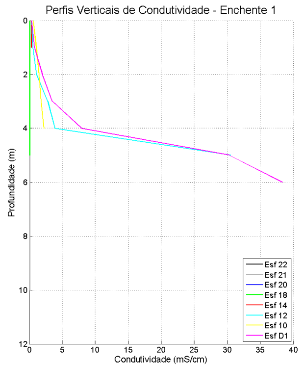
Figura 64: Perfis verticais de condutividade da água em período de maré enchente, para cada estação amostral. Campanha 2 – Enchente 1 – data: 21/02/2016.
