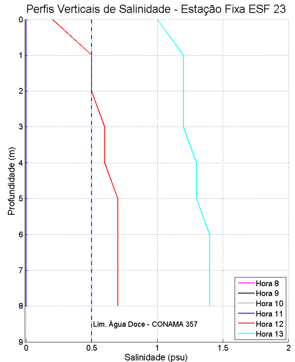
Figura 99: Perfis verticais de salinidade para a estação fixa ESF_23. Campanha 2 – 12 horas – data: 24/02/2016. Resolução CONAMA 357/2005 (I - águas doces: águas com salinidade igual ou inferior a 0,5 ‰).
