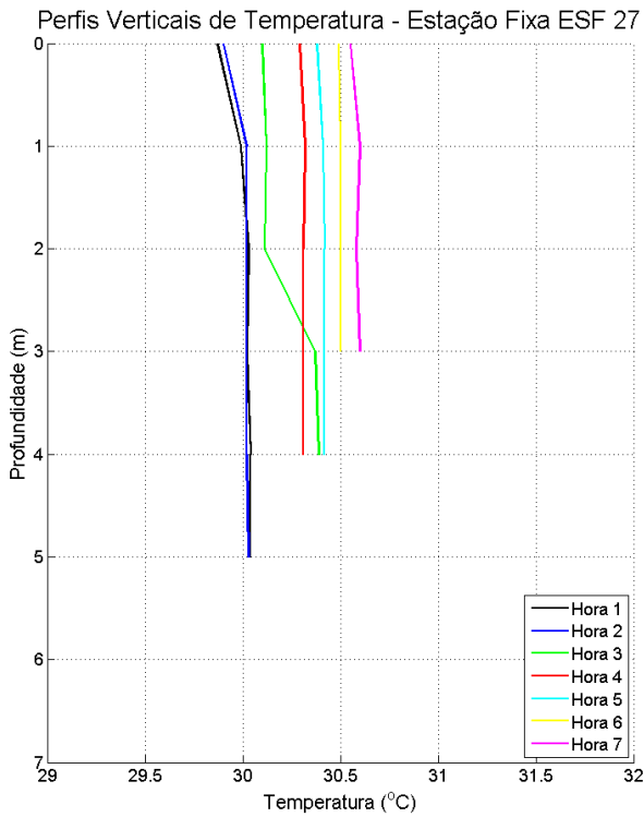
Figura 92: Perfis verticais de temperatura para a estação fixa ESF_27. Campanha 2 – 12 horas – data: 23/02/2016.
