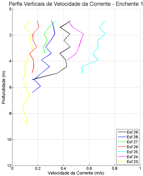
Figura 24: Perfis verticais de velocidade da corrente em período de maré enchente, para cada estação amostral. Campanha 1 – Enchente 1 – data: 09/02/2016.
