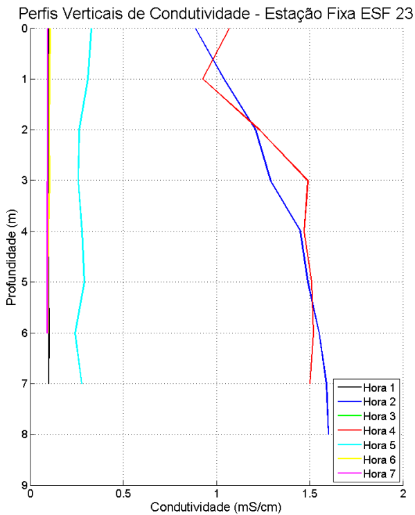
Figura 88: Perfis verticais de condutividade para a estação fixa ESF_23. Campanha 1 – 12 horas – data: 12/02/2016.
