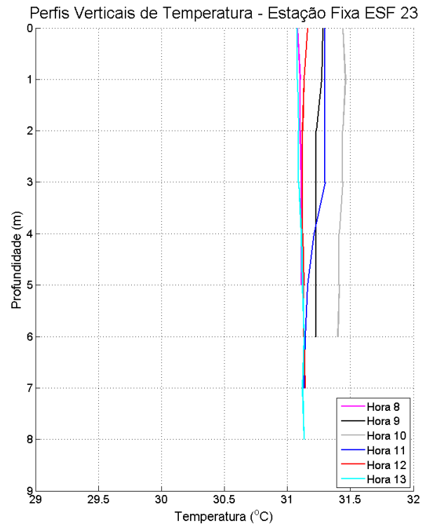
Figura 87: Perfis verticais de temperatura para a estação fixa ESF_23. Campanha 1 – 12 horas – data: 12/02/2016.
