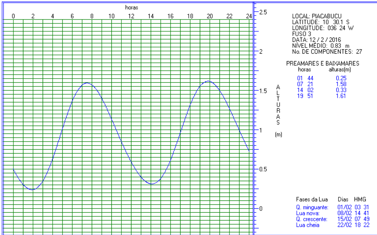
Figura 14. Previsão de maré para o dia 12/02/2016 (campanha 1), para a localidade de Piaçabuçu, localizada na margem esquerda do Rio São Francisco.
