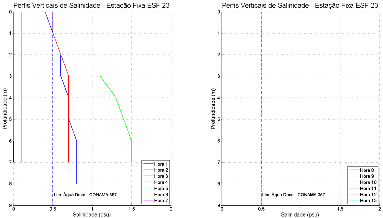
Figura 89: Perfis verticais de salinidade para a estação fixa ESF_23. Campanha 1 – 12 horas – data: 12/02/2016. Resolução CONAMA 357/2005 (I - águas doces: águas com salinidade igual ou inferior a 0,5 ‰).
