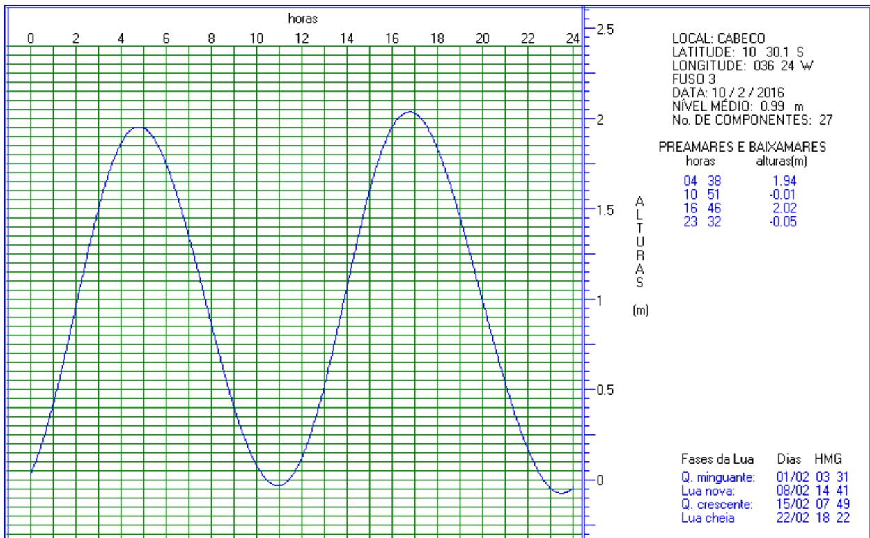
Figura 11. Previsão de maré para o dia 10/02/2016 (campanha 1), para a localidade de Cabeço, localizada na foz do Rio São Francisco.
