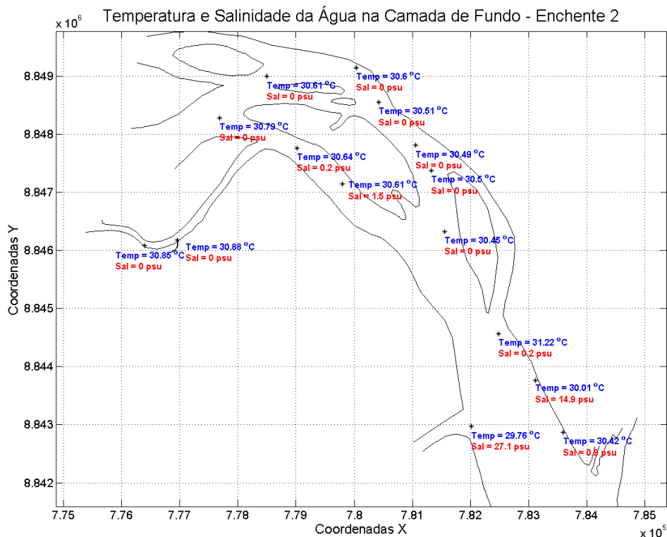
Figura 77: Temperatura e salinidade da água na camada de fundo. Campanha 2 – Enchente 2 – data: 22/02/2016. Resolução CONAMA 357/2005 (I - águas doces: águas com salinidade igual ou inferior a 0,5 ‰).
