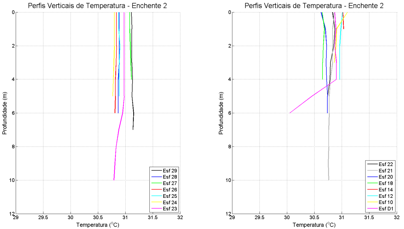
Figura 34: Perfis verticais de temperatura da água em período de maré enchente, para cada estação amostral. Campanha 1 – Enchente 2 – data: 10/02/2016 .
