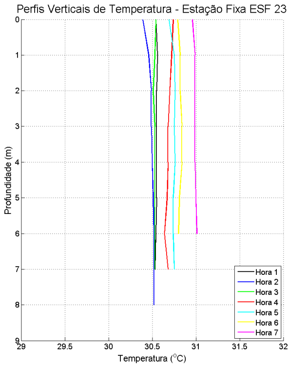
Figura 87: Perfis verticais de temperatura para a estação fixa ESF_23. Campanha 1 – 12 horas – data: 12/02/2016.
