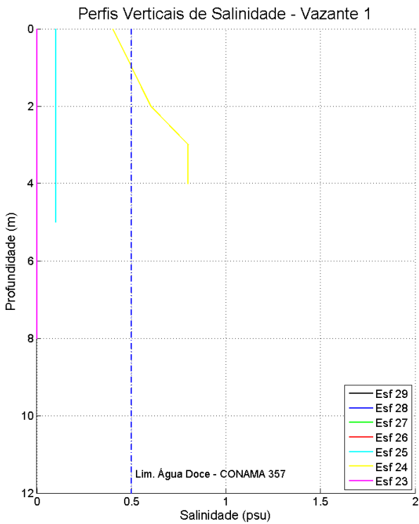
Figura 69: Perfis verticais de salinidade da água em período de maré vazante, para cada estação amostral. Campanha 2 – Vazante 1 – data: 21/02/2016. Resolução CONAMA 357/2005 (I - águas doces: águas com salinidade igual ou inferior a 0,5 ‰).
