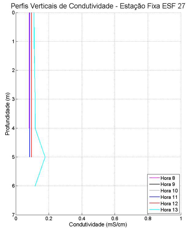
Figura 93: Perfis verticais de condutividade para a estação fixa ESF_27. Campanha 2 – 12 horas – data: 23/02/2016.
