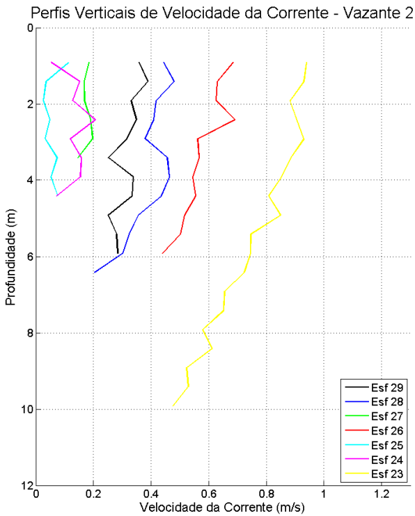
Figura 27: Perfis verticais de velocidade da corrente em período de maré vazante, para cada estação amostral. Campanha 1 – Vazante 2 – data: 10/02/2016.
