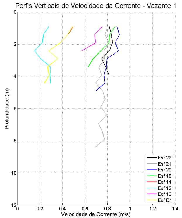
Figura 53: Perfis verticais de velocidade da corrente em período de maré vazante, para cada estação amostral. Campanha 2 – Vazante 1 – data: 21/02/2016.
