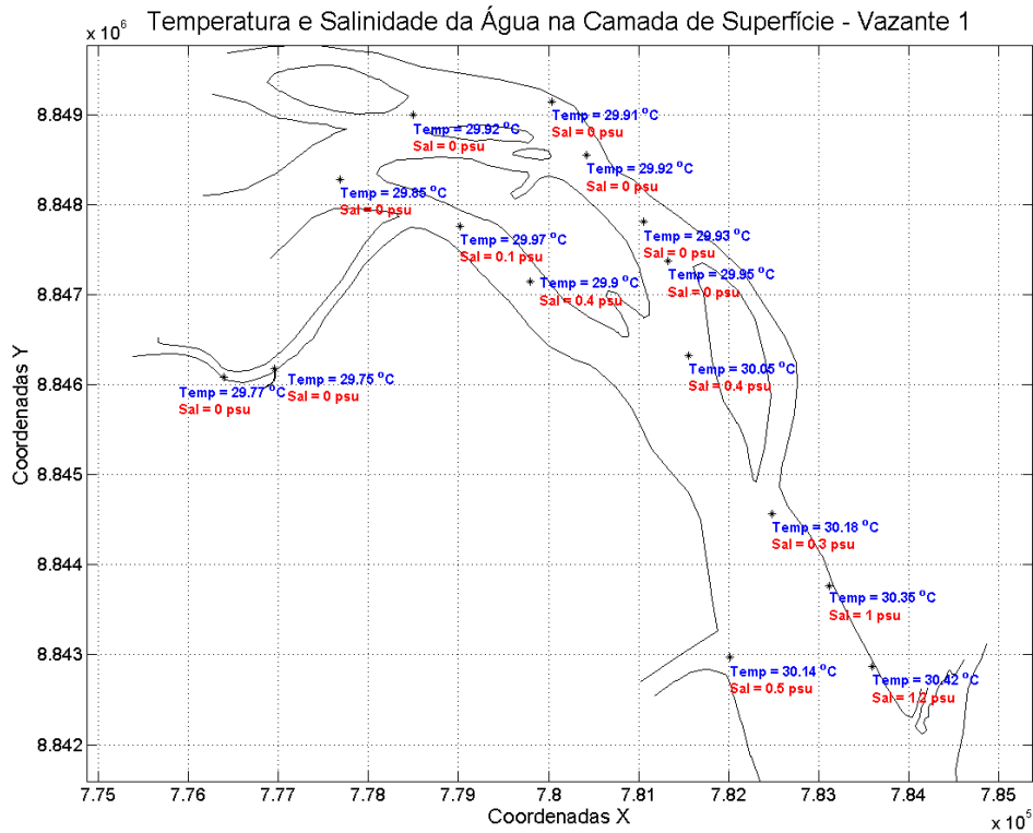
Figura 74: Temperatura e salinidade da água na camada de superfície. Campanha 2 – Vazante 1 – data: 21/02/2016. Resolução CONAMA 357/2005 (I - águas doces: águas com salinidade igual ou inferior a 0,5 ‰).
