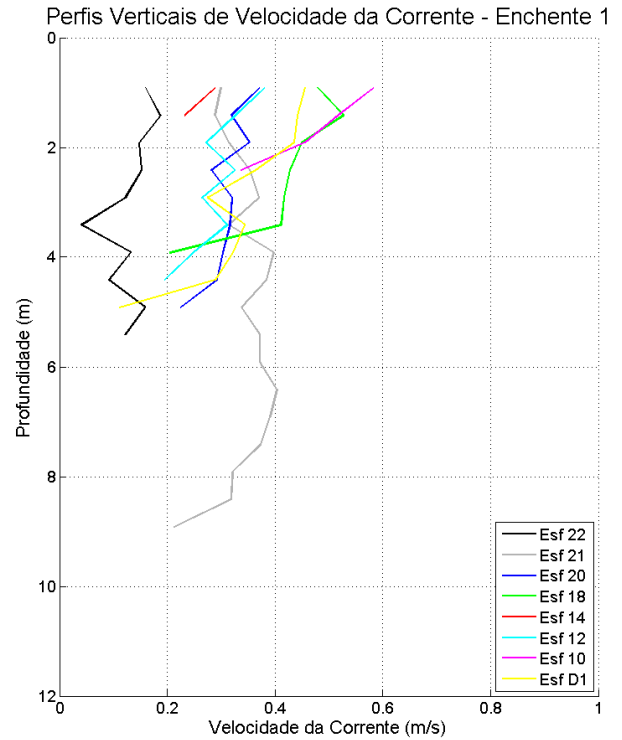
Figura 24: Perfis verticais de velocidade da corrente em período de maré enchente, para cada estação amostral. Campanha 1 – Enchente 1 – data: 09/02/2016.
