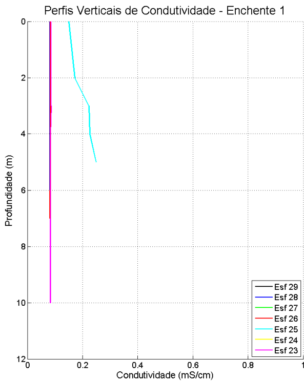
Figura 64: Perfis verticais de condutividade da água em período de maré enchente, para cada estação amostral. Campanha 2 – Enchente 1 – data: 21/02/2016.
