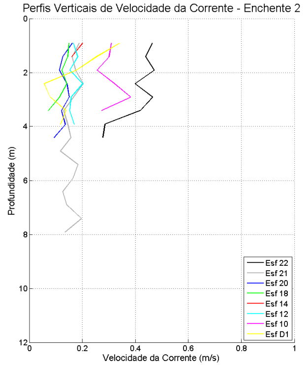
Figura 54: Perfis verticais de velocidade da corrente em período de maré enchente, para cada estação amostral. Campanha 2 – Enchente 2 – data: 22/02/2016.
