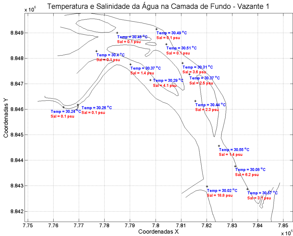
Figura 47: Temperatura e salinidade da água na camada de fundo. Campanha 1 – Vazante 1 – data: 09/02/2016. Resolução CONAMA 357/2005 (I - águas doces: águas com salinidade igual ou inferior a 0,5 ‰).
