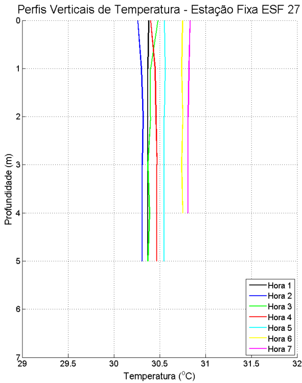
Figura 82: Perfis verticais de temperatura para a estação fixa ESF_27. Campanha 1 – 12 horas – data: 11/02/2016.
