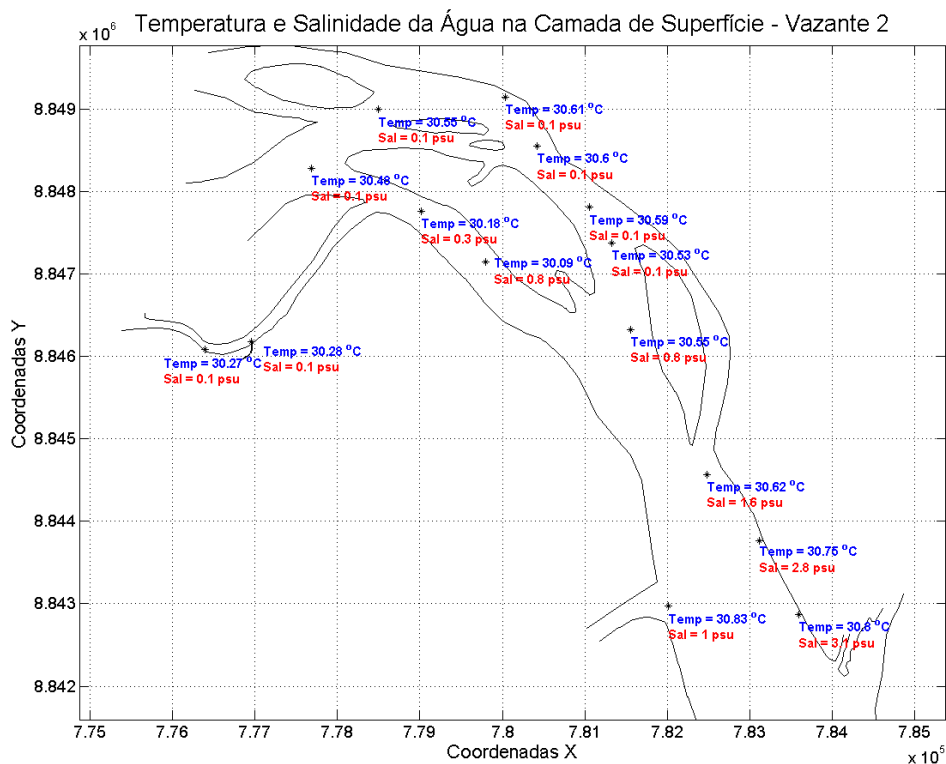
Figura 50: Temperatura e salinidade da água na camada de superfície. Campanha 1 – Vazante 2 – data: 10/02/2016. Resolução CONAMA 357/2005 (I - águas doces: águas com salinidade igual ou inferior a 0,5 ‰).
