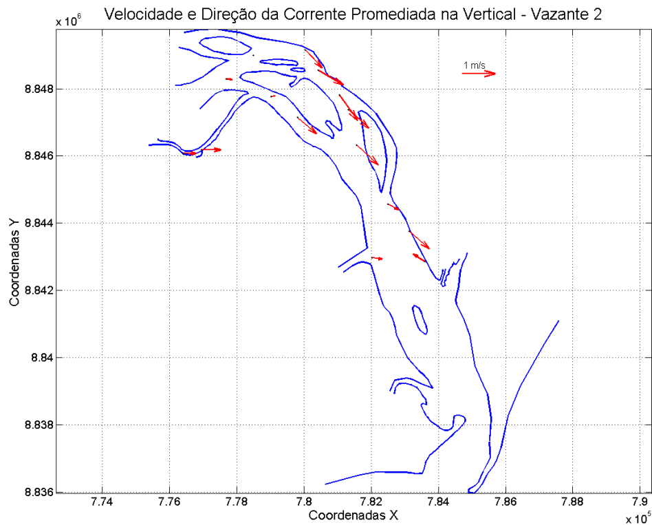
Figura 31: Velocidade e direção da corrente promediada na vertical, em cada estação amostral. Campanha 1 – Vazante 2 – data: 10/02/2016.
