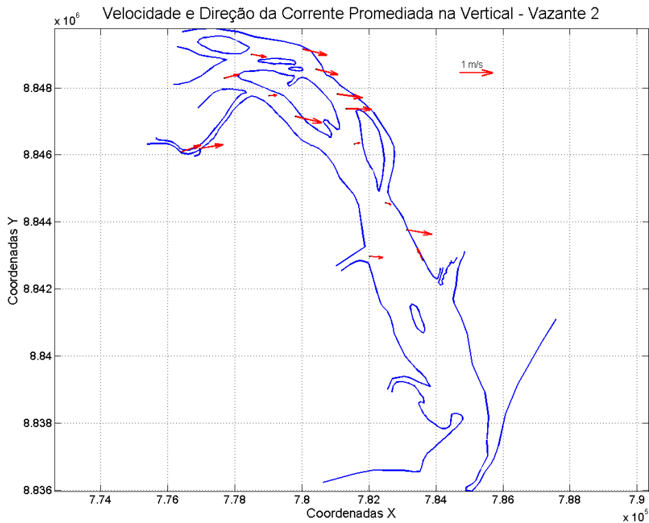
Figura 59: Velocidade e direção da corrente promediada na vertical, em cada estação amostral. Campanha 2 – Vazante 2 – data: 22/02/2016.
