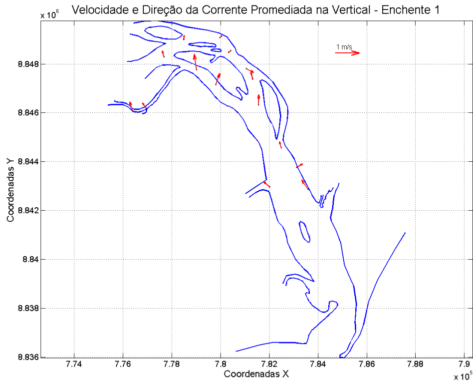
Figura 28: Velocidade e direção da corrente promediada na vertical, em cada estação amostral. Campanha 1 – Enchente 1 – data: 09/02/2016.
