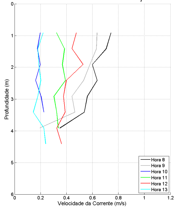
Figura 80: Perfis verticais de velocidade da corrente para a estação fixa ESF_27. Campanha 1 – 12 horas – data: 11/02/2016.
