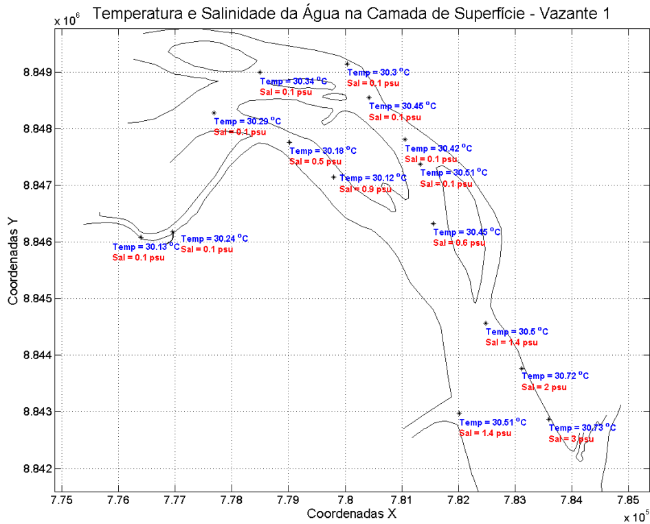
Figura 46: Temperatura e salinidade da água na camada de superfície. Campanha 1 – Vazante 1 – data: 09/02/2016. Resolução CONAMA 357/2005 (I - águas doces: águas com salinidade igual ou inferior a 0,5 ‰).
