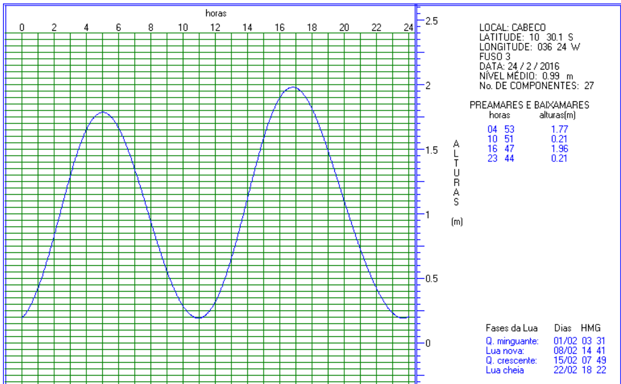
Figura 23. Previsão de maré para o dia 24/02/2016 (campanha 2), para a localidade de Cabeço, localizada na foz do Rio São Francisco.
