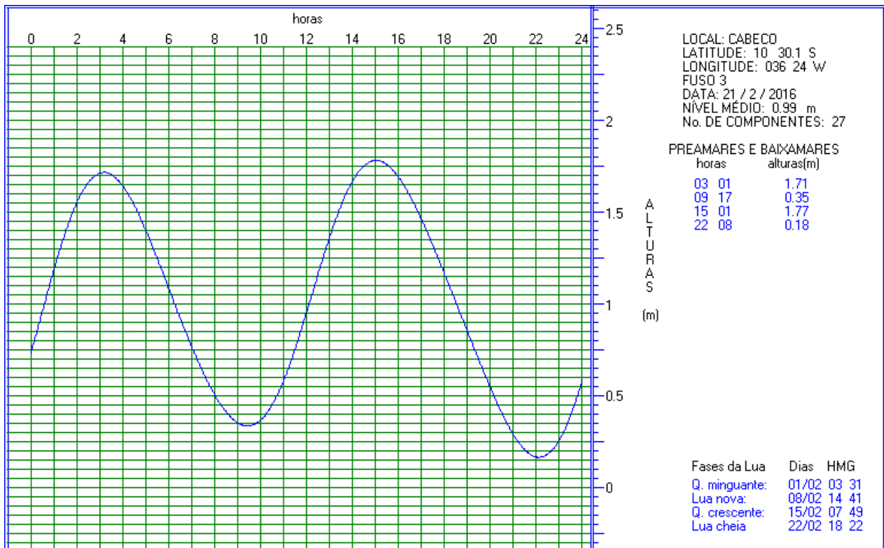
Figura 17. Previsão de maré para o dia 21/02/2016 (campanha 1), para a localidade de Cabeço, localizada na foz do Rio São Francisco.
