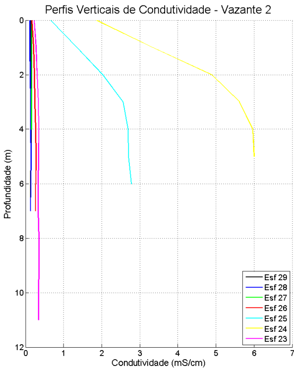
Figura 39: Perfis verticais de condutividade da água em período de maré vazante, para cada estação amostral. Campanha 1 – Vazante 2 – data: 10/02/2016.
