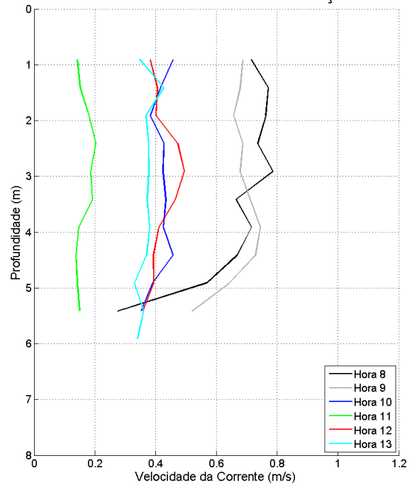
Figura 85: Perfis verticais de velocidade da corrente para a estação fixa ESF_23. Campanha 1 – 12 horas – data: 12/02/2016.
