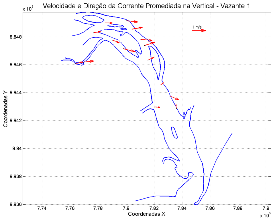
Figura 57: Velocidade e direção da corrente promediada na vertical, em cada estação amostral. Campanha 2 – Vazante 1 – data: 21/02/2016.
