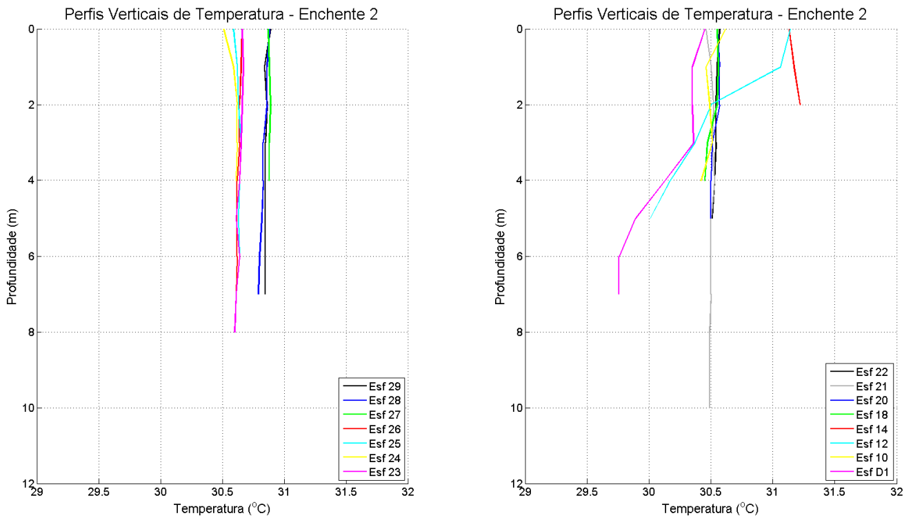
Figura 62: Perfis verticais de temperatura da água em período de maré enchente, para cada estação amostral. Campanha 2 – Enchente 2 – data: 22/02/2016.
