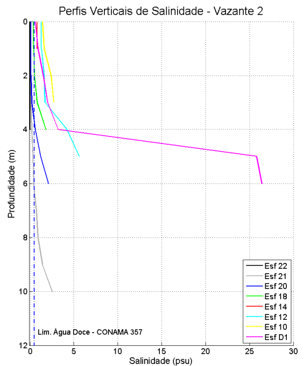
Figura 71: Perfis verticais de salinidade da água em período de maré vazante, para cada estação amostral. Campanha 2 – Vazante 2 – data: 22/02/2016. Resolução CONAMA 357/2005 (I - águas doces: águas com salinidade igual ou inferior a 0,5 ‰).
