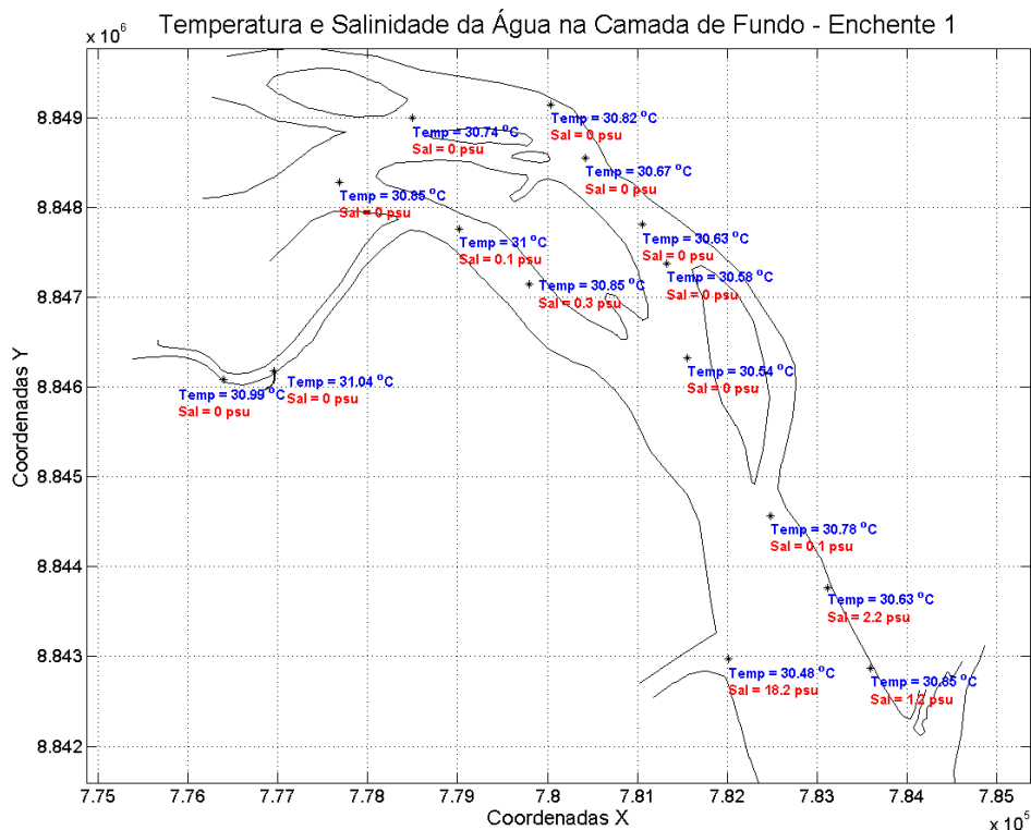
Figura 45: Temperatura e salinidade da água na camada de fundo. Campanha 1 – Enchente 1 – data: 09/02/2016. Resolução CONAMA 357/2005 (I - águas doces: águas com salinidade igual ou inferior a 0,5 ‰).
