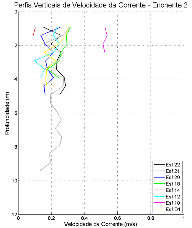
Figura 26: Perfis verticais de velocidade da corrente em período de maré enchente, para cada estação amostral. Campanha 1 – Enchente 2 – data: 10/02/2016.
