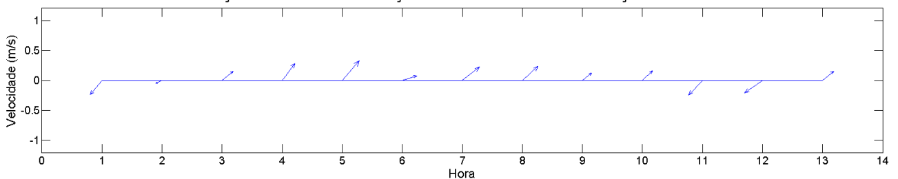
Figura 81: Diagrama “stick plot” das correntes em superfície (painel superior) e fundo (painel inferior), para a estação fixa ESF_27. Campanha 1 – 12 horas – data: 11/02/2016.
