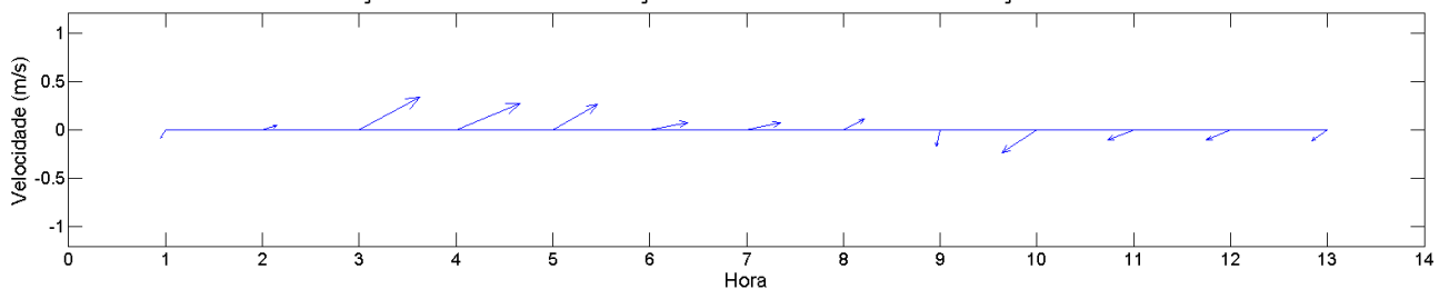
Figura 96: Diagrama “stick plot” das correntes em superfície (painel superior) e fundo (painel inferior), para a estação fixa ESF_23. Campanha 2 – 12 horas – data: 24/02/2016.
