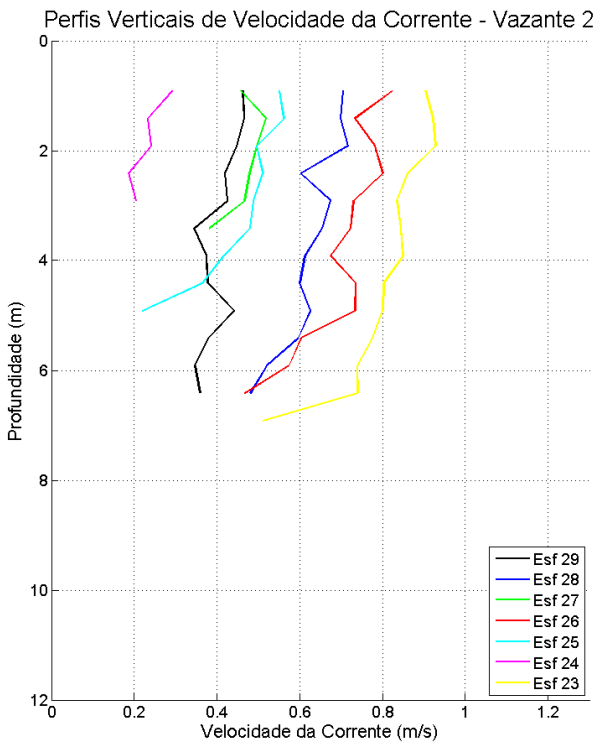
Figura 55: Perfis verticais de velocidade da corrente em período de maré vazante, para cada estação amostral. Campanha 2 – Vazante 2 – data: 22/02/2016.
