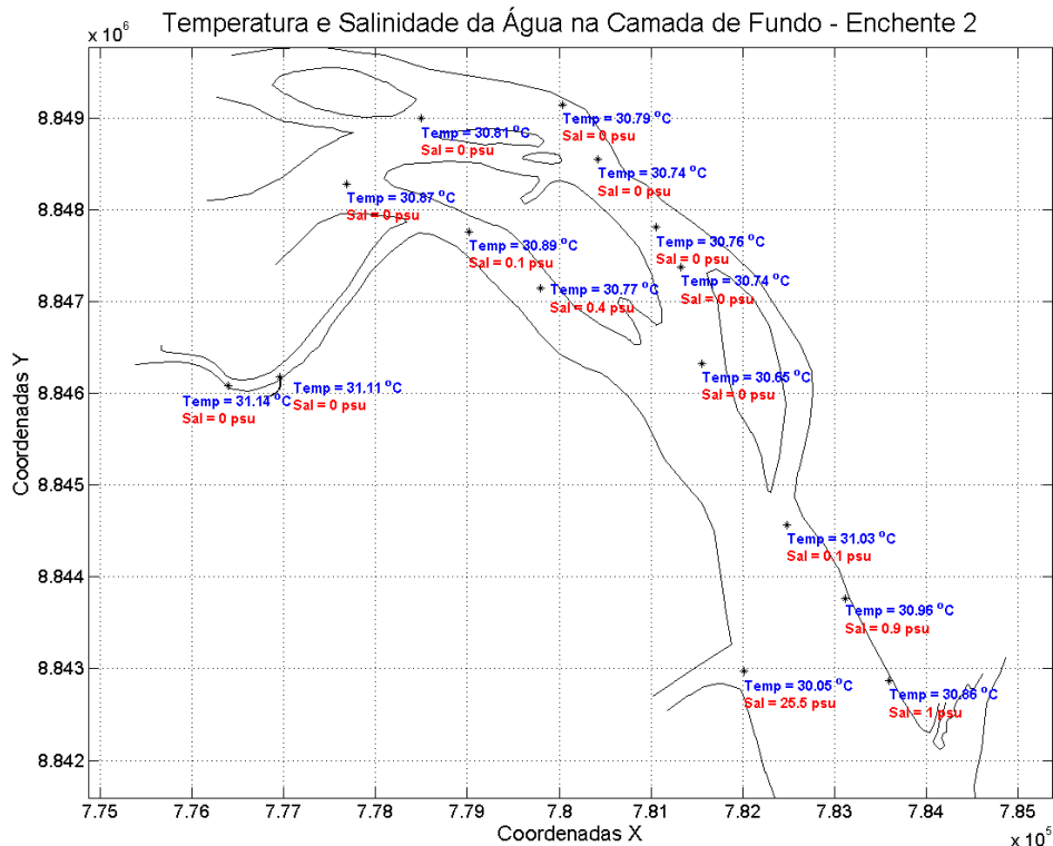
Figura 49: Temperatura e salinidade da água na camada de fundo. Campanha 1 – Enchente 2 – data: 10/02/2016 . Resolução CONAMA 357/2005 (I - águas doces: águas com salinidade igual ou inferior a 0,5 ‰).
