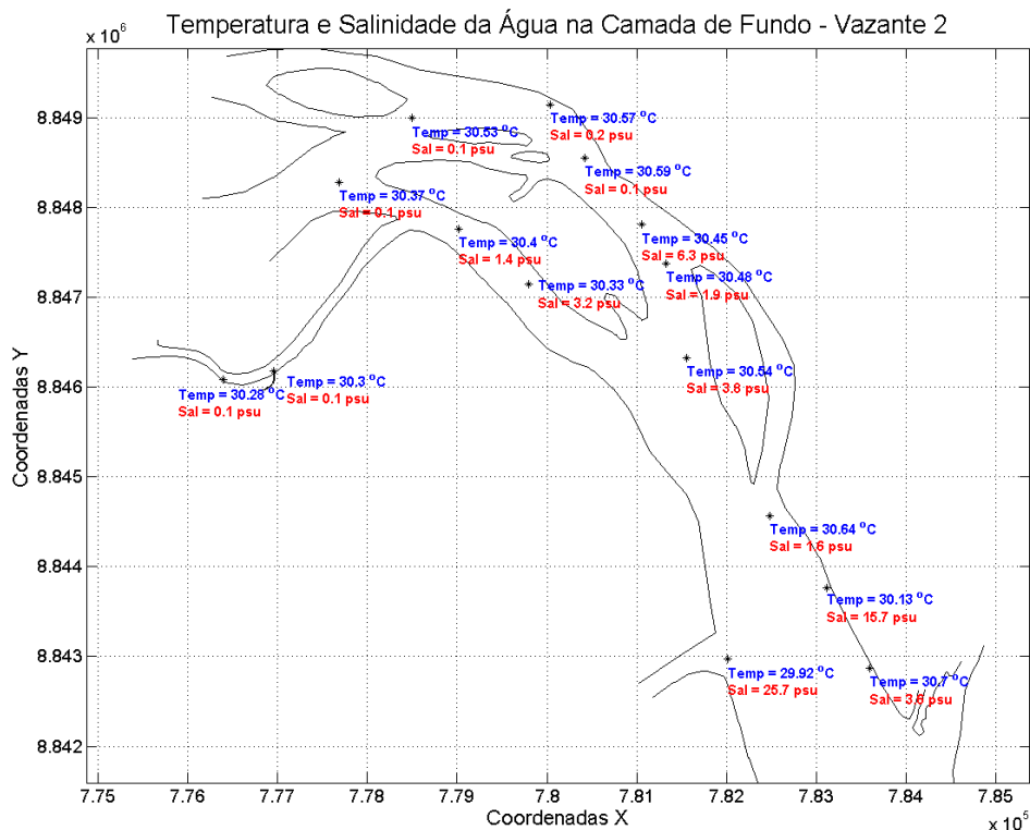
Figura 51: Temperatura e salinidade da água na camada de fundo. Campanha 1 – Vazante 2 – data: 10/02/2016. Resolução CONAMA 357/2005 (I - águas doces: águas com salinidade igual ou inferior a 0,5 ‰).
