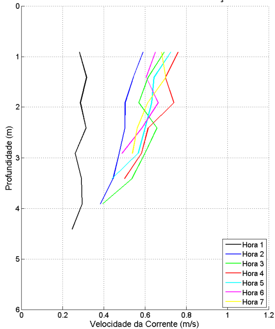
Figura 90: Perfis verticais de velocidade da corrente para a estação fixa ESF_27. Campanha 2 – 12 horas – data: 23/02/2016.
