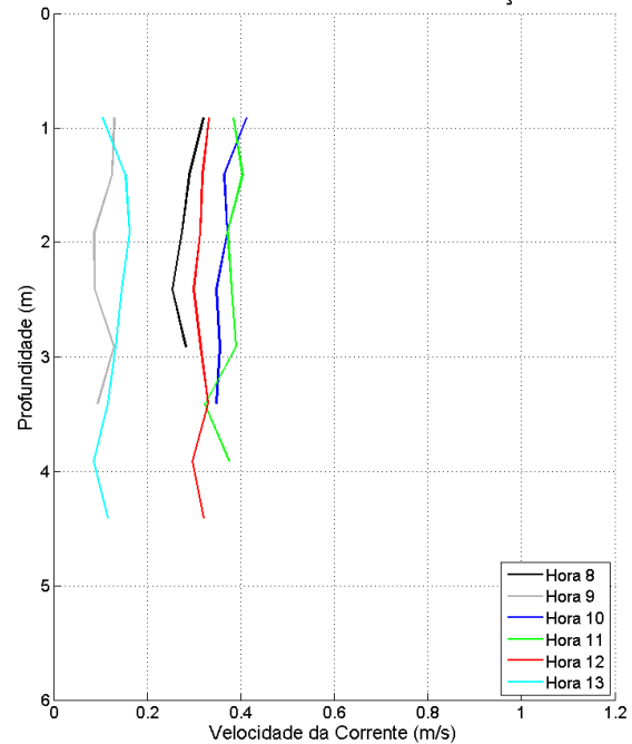
Figura 90: Perfis verticais de velocidade da corrente para a estação fixa ESF_27. Campanha 2 – 12 horas – data: 23/02/2016.
