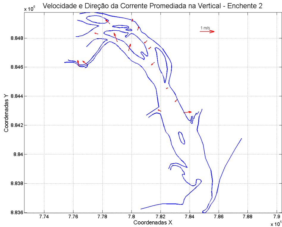
Figura 30: Velocidade e direção da corrente promediada na vertical, em cada estação amostral. Campanha 1 – Enchente 2 – data: 10/02/2016 .
