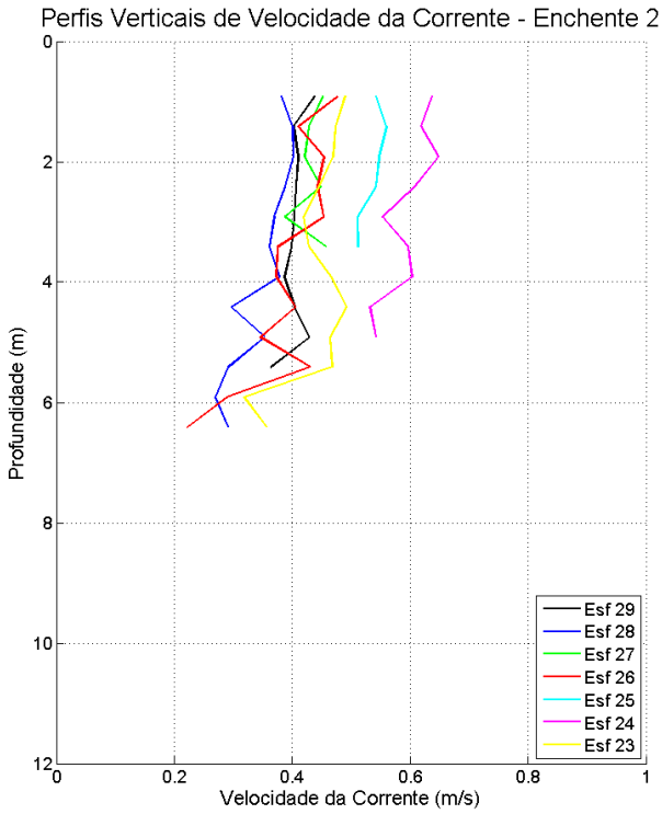
Figura 54: Perfis verticais de velocidade da corrente em período de maré enchente, para cada estação amostral. Campanha 2 – Enchente 2 – data: 22/02/2016.
