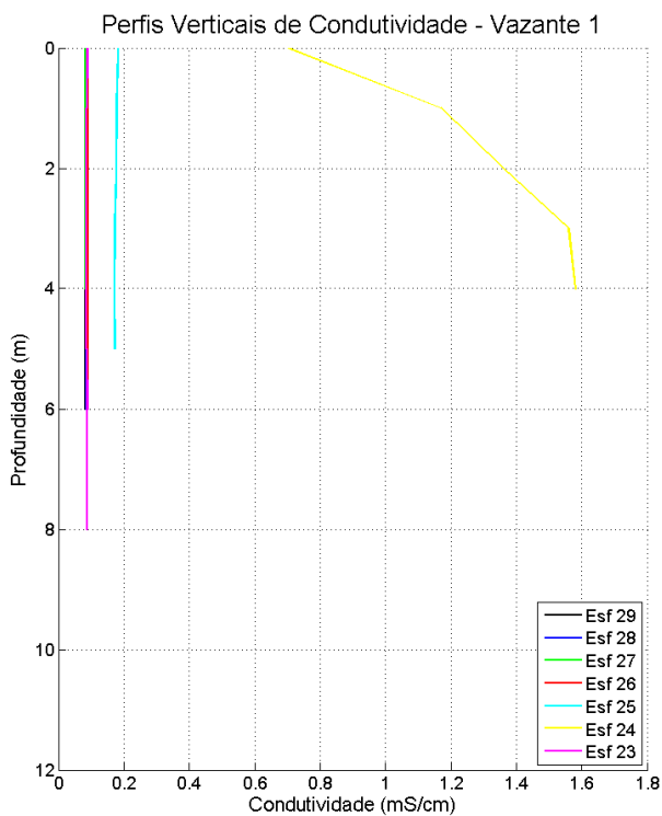
Figura 65: Perfis verticais de condutividade da água em período de maré vazante, para cada estação amostral. Campanha 2 – Vazante 1 – data: 21/02/2016.
