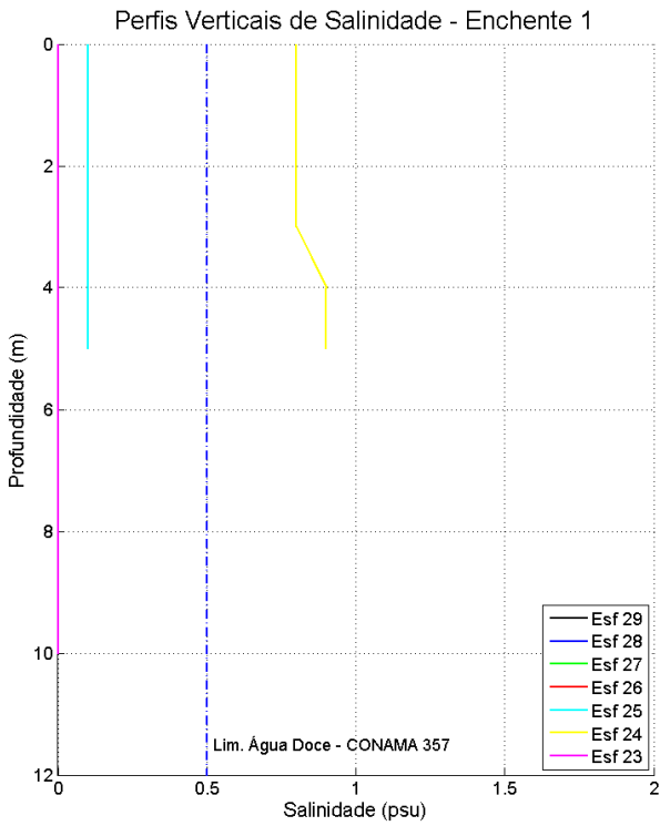
Figura 68: Perfis verticais de salinidade da água em período de maré enchente, para cada estação amostral. Campanha 2 – Enchente 1 – data: 21/02/2016. Resolução CONAMA 357/2005 (I - águas doces: águas com salinidade igual ou inferior a 0,5 ‰).
