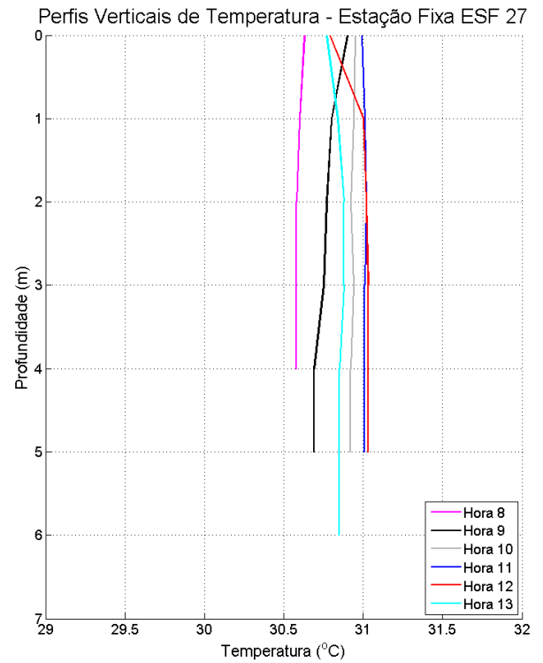
Figura 92: Perfis verticais de temperatura para a estação fixa ESF_27. Campanha 2 – 12 horas – data: 23/02/2016.
