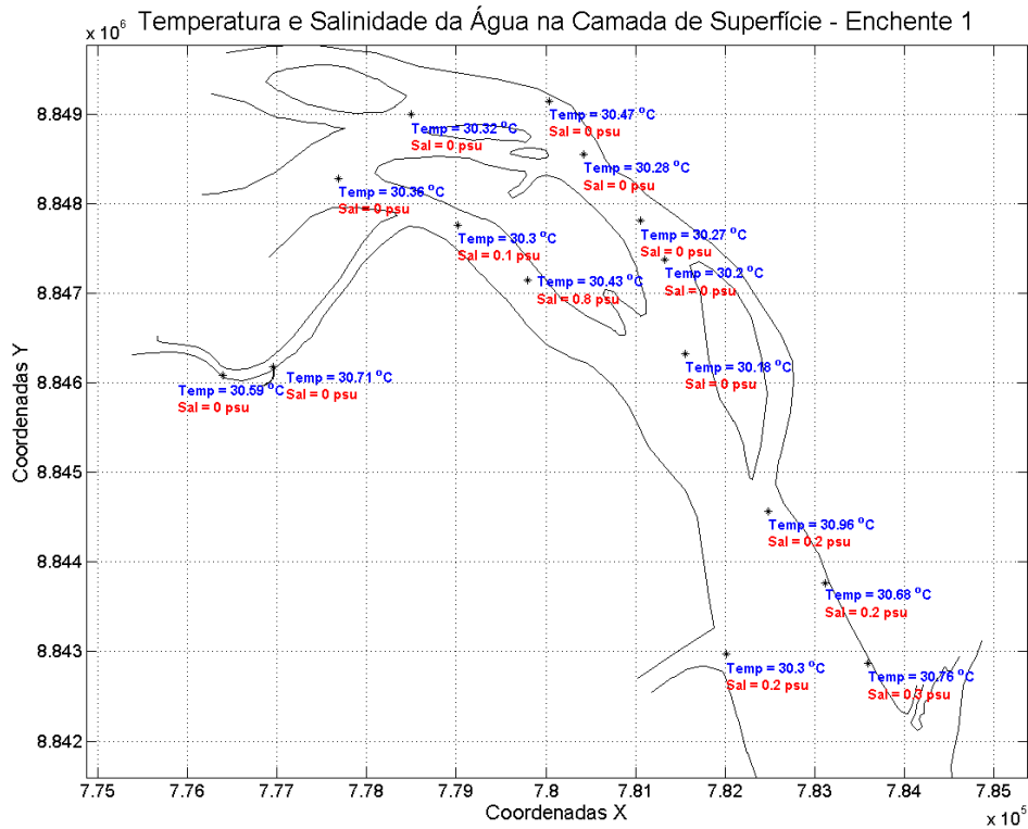
Figura 72: Temperatura e salinidade da água na camada de superfície. Campanha 2 – Enchente 1 – data: 21/02/2016. Resolução CONAMA 357/2005 (I - águas doces: águas com salinidade igual ou inferior a 0,5 ‰).
