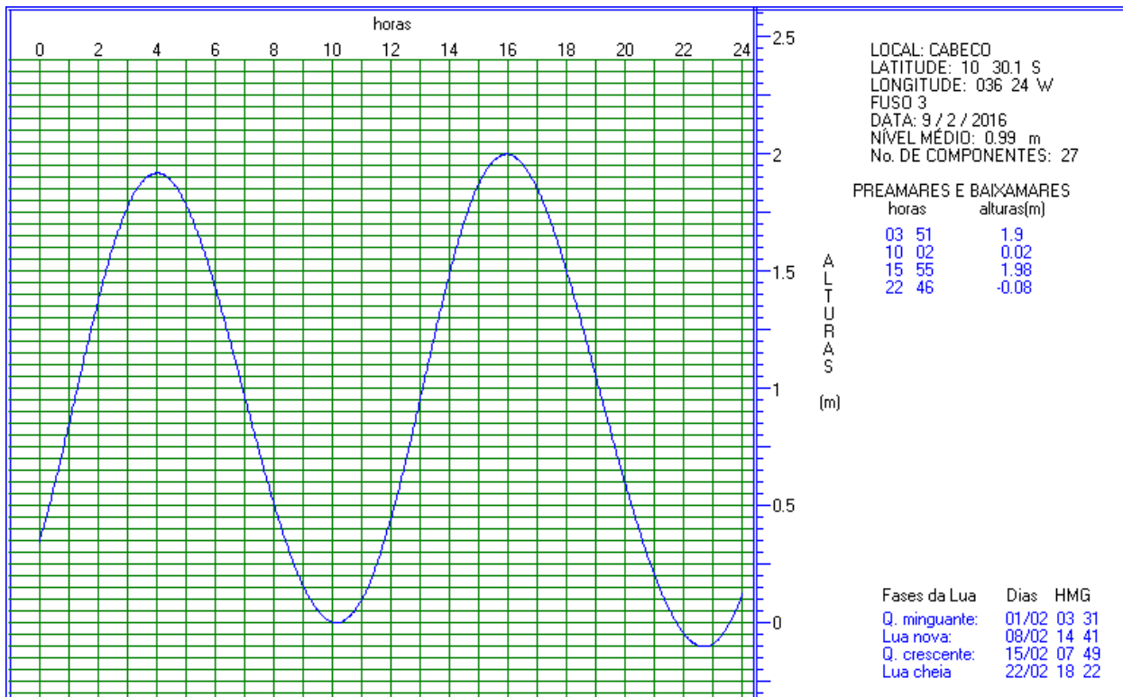
Figura 9. Previsão de maré para o dia 09/02/2016 (campanha 1), para a localidade de Cabeço, localizada na foz do Rio São Francisco.
