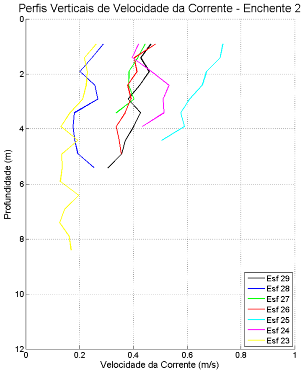
Figura 26: Perfis verticais de velocidade da corrente em período de maré enchente, para cada estação amostral. Campanha 1 – Enchente 2 – data: 10/02/2016.
