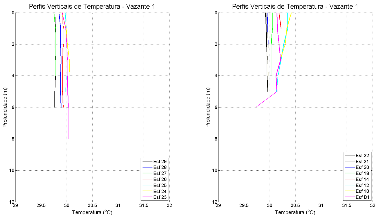
Figura 61: Perfis verticais de temperatura da água em período de maré vazante, para cada estação amostral. Campanha 2 – Vazante 1 – data: 21/02/2016.
