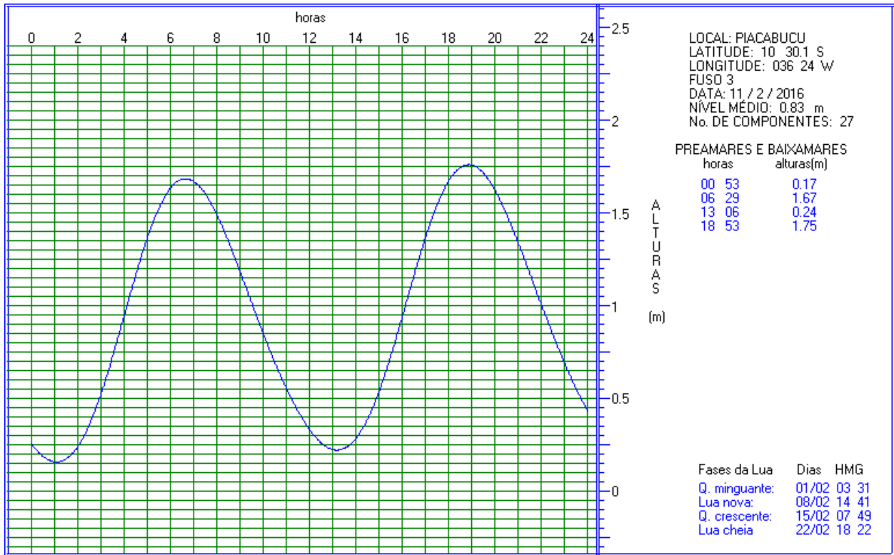
Figura 12. Previsão de maré para o dia 11/02/2016 (campanha 1), para a localidade de Piaçabuçu, localizada na margem esquerda do Rio São Francisco.
