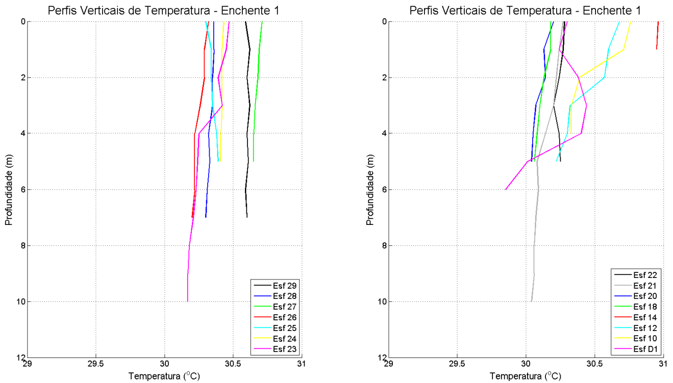
Figura 60: Perfis verticais de temperatura da água em período de maré enchente, para cada estação amostral. Campanha 2 – Enchente 1 – data: 21/02/2016.
