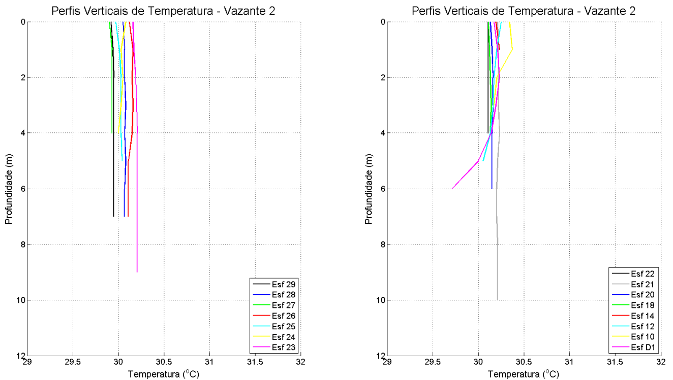
Figura 63: Perfis verticais de temperatura da água em período de maré vazante, para cada estação amostral. Campanha 2 – Vazante 2 – data: 22/02/2016.
