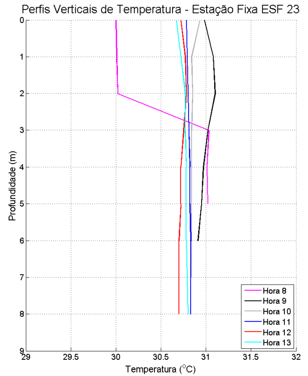
Figura 97: Perfis verticais de temperatura para a estação fixa ESF_23. Campanha 2 – 12 horas – data: 24/02/2016.
