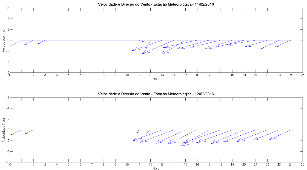
Figura 101: Diagrama “stick plot” dos dados de ventos medidos no dia 11/02/2016 (painel superior) e 12/02/2016 (painel inferior).
