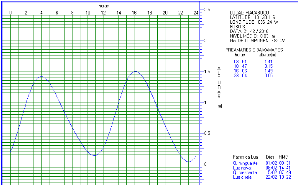
Figura 16. Previsão de maré para o dia 21/02/2016 (campanha 1), para a localidade de Piaçabuçu, localizada na margem esquerda do Rio São Francisco.
