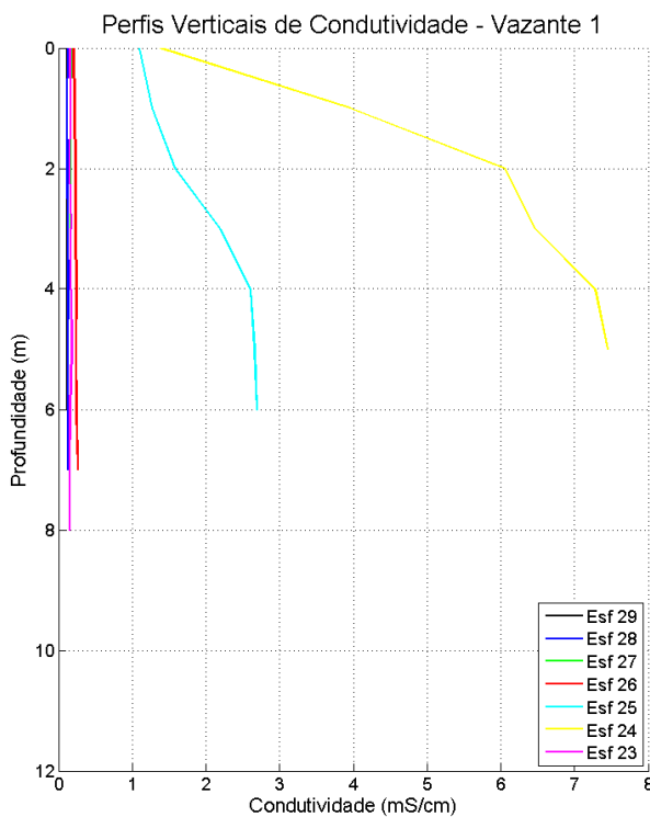
Figura 37: Perfis verticais de condutividade da água em período de maré vazante, para cada estação amostral. Campanha 1 – Vazante 1 – data: 09/02/2016.
