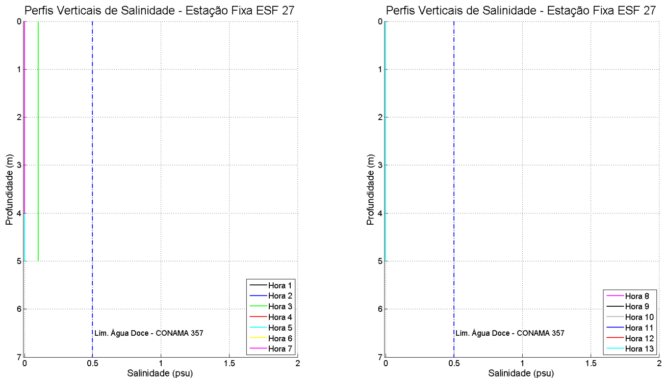
Figura 84: Perfis verticais de salinidade para a estação fixa ESF_27. Campanha 1 – 12 horas – data: 11/02/2016. Resolução CONAMA 357/2005 (I - águas doces: águas com salinidade igual ou inferior a 0,5 ‰).
