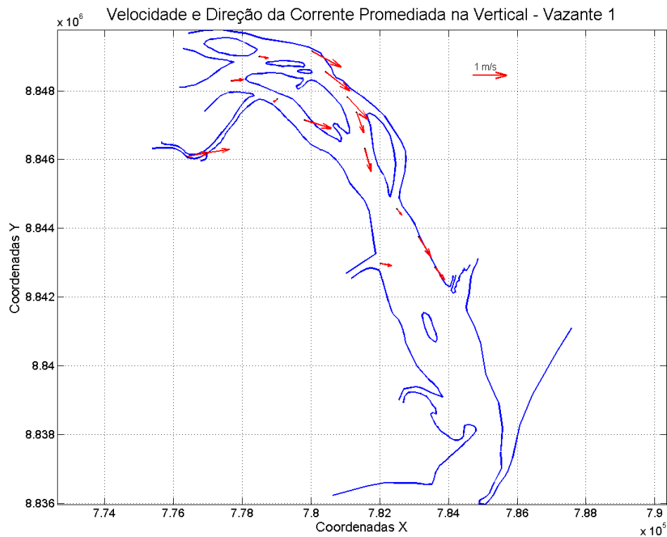
Figura 29: Velocidade e direção da corrente promediada na vertical, em cada estação amostral. Campanha 1 – Vazante 1 – data: 09/02/2016.
