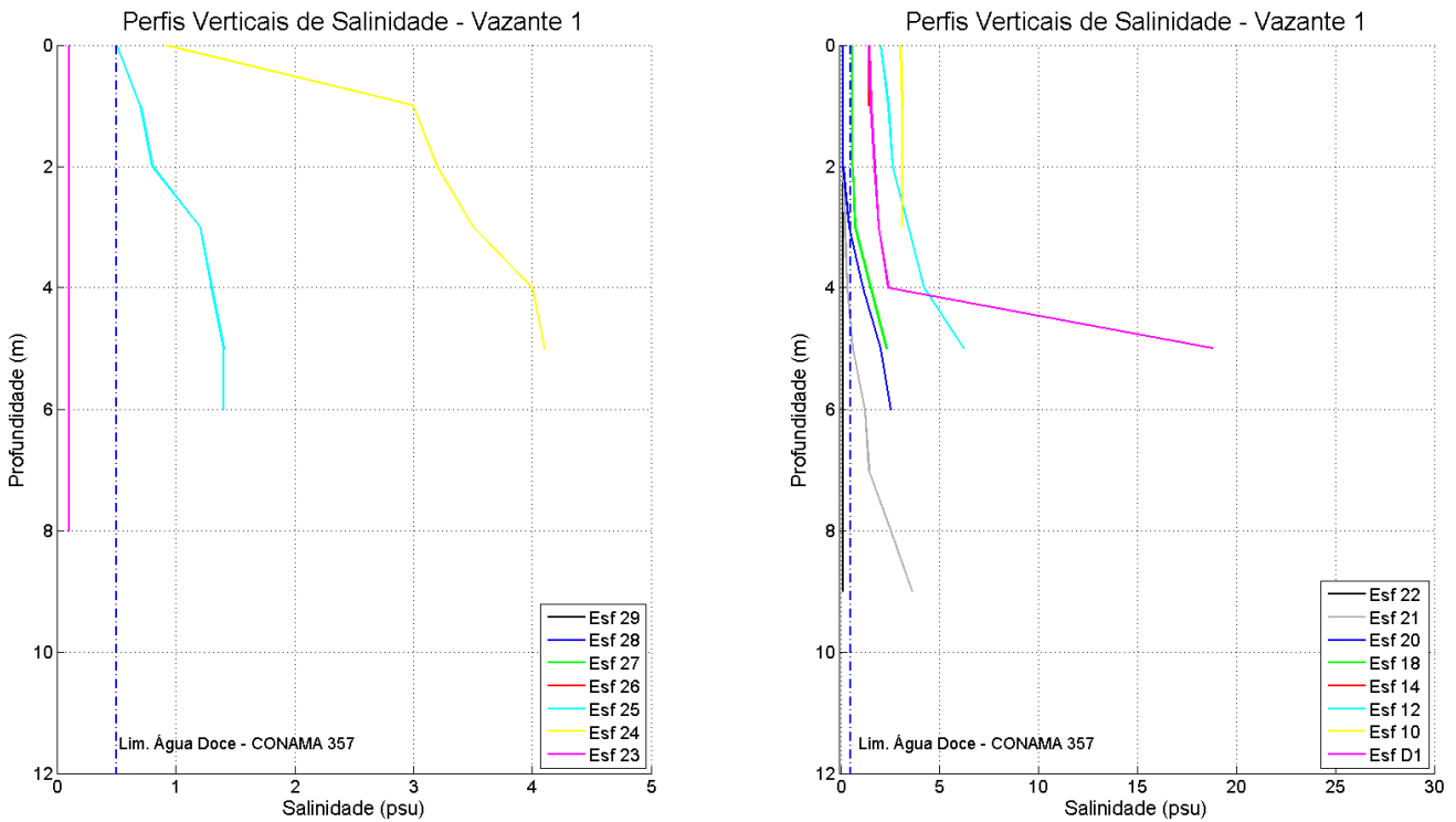
Figura 41: Perfis verticais de salinidade da água em período de maré vazante, para cada estação amostral. Campanha 1 – Vazante 1 – data: 09/02/2016. Resolução CONAMA 357/2005 (I - águas doces: águas com salinidade igual ou inferior a 0,5 ‰).
