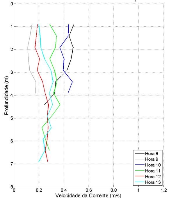
Figura 95: Perfis verticais de velocidade da corrente para a estação fixa ESF_23. Campanha 2 – 12 horas – data: 24/02/2016.
