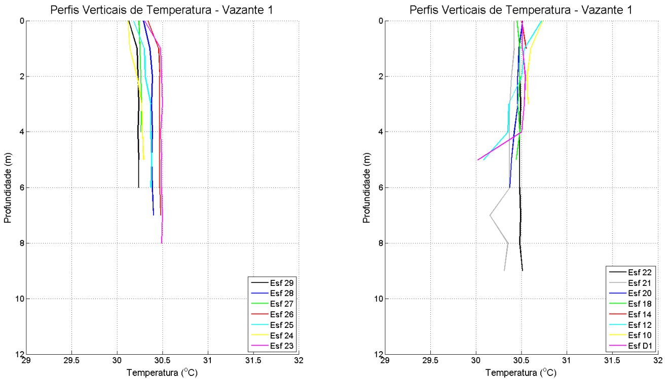
Figura 33: Perfis verticais de temperatura da água em período de maré vazante, para cada estação amostral. Campanha 1 – Vazante 1 – data: 09/02/2016.
