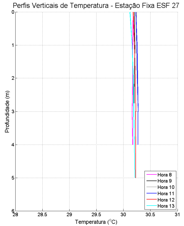
Figura 89: Perfis verticais de temperatura para a estação fixa ESF_27. Campanha 1 – 12 horas – data: 13/01/2016.
