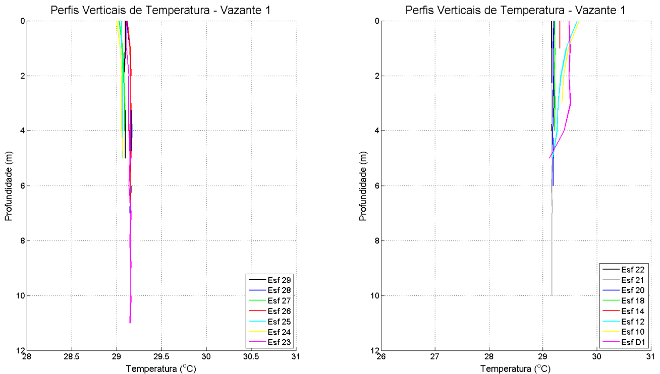
Figura 63: Perfis verticais de temperatura da água em período de maré vazante, para cada estação amostral. Campanha 2 – Vazante 1 – data: 24/01/2016.
