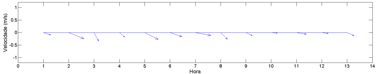
Figura 93: Diagrama stick plot das correntes em superfície (painel superior) e fundo (painel inferior), para a estação fixa ESF_23. Campanha 2 – 12 horas – data: 26/01/2016.
