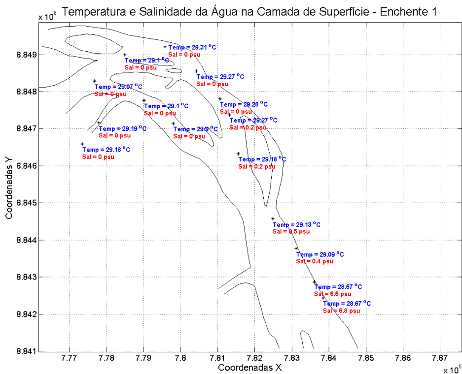
Figura 46: Temperatura e salinidade da água na camada de superfície. Campanha 1 – Enchente 1 – data: 10/01/2016. Resolução CONAMA 357/2005 (I - águas doces: águas com salinidade igual ou inferior a 0,5 ‰)
