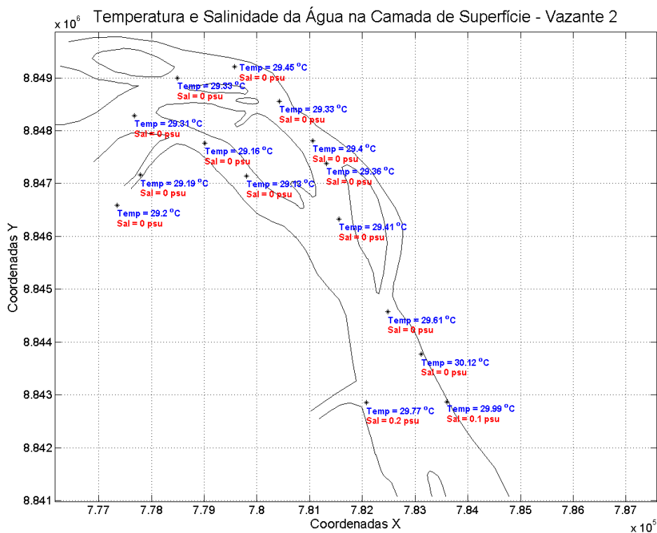
Figura 80: Temperatura e salinidade da água na camada de superfície. Campanha 2 – Vazante 2 – data: 25/01/2016. Resolução CONAMA 357/2005 (I - águas doces: águas com salinidade igual ou inferior a 0,5 ‰)
