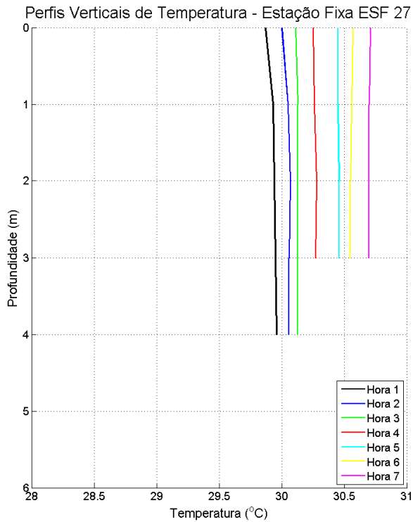
Figura 99: Perfis verticais de temperatura para a estação fixa ESF_27. Campanha 2 – 12 horas – data: 27/01/2016.
