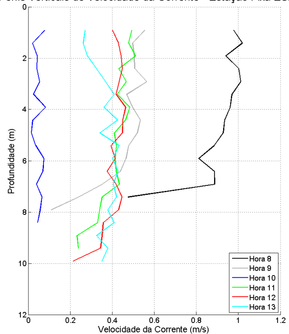
Figura 82: Perfis verticais de velocidade da corrente para a estação fixa ESF_23. Campanha 1 – 12 horas – data: 12/01/2016.
