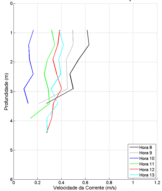
Figura 87: Perfis verticais de velocidade da corrente para a estação fixa ESF_27. Campanha 1 – 12 horas – data: 13/01/2016.
