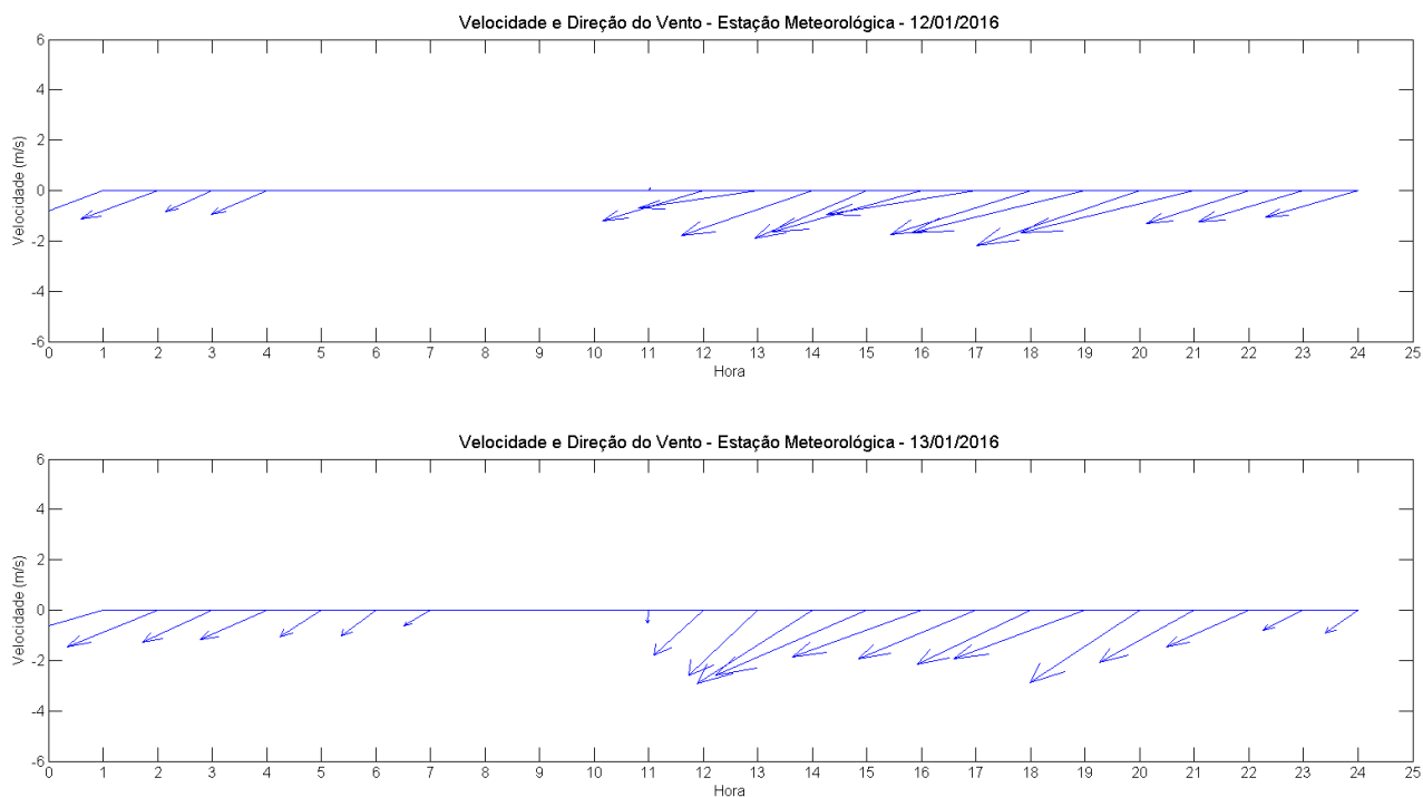
Figura 103: Diagrama stick plot dos dados de ventos medidos no dia 12/01/2016 (painel superior) e 13/01/2016 (painel inferior).
