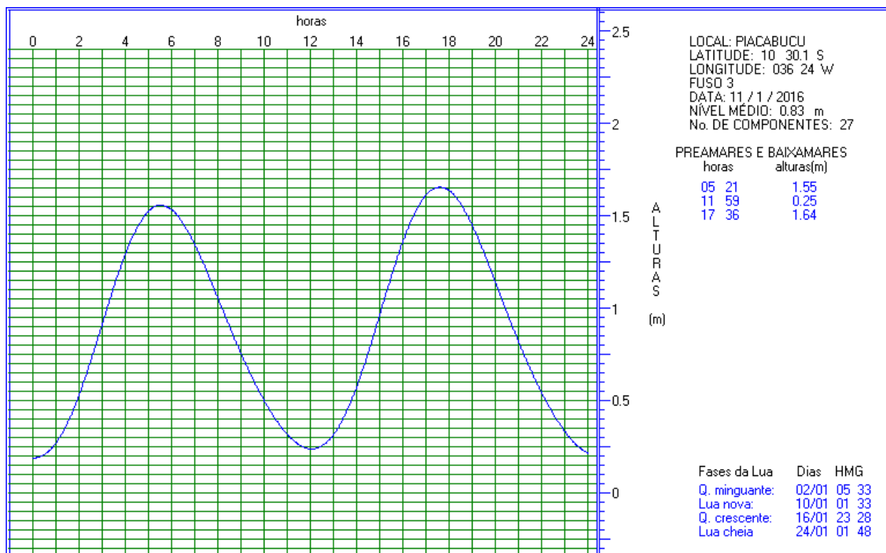
Figura 10. Previsão de maré para o dia 11/01/2016 (campanha 1), para a localidade de Piaçabuçu, localizada na margem do Rio São Francisco.
