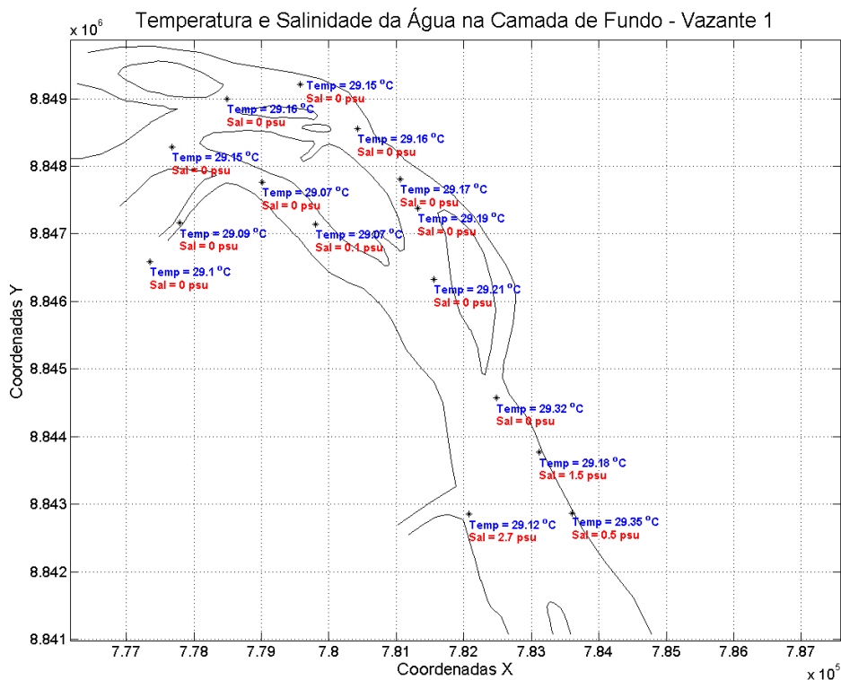
Figura 77: Temperatura e salinidade da água na camada de fundo. Campanha 2 – Vazante 1 – data: 24/01/2016. Resolução CONAMA 357/2005 (I - águas doces: águas com salinidade igual ou inferior a 0,5 ‰)
