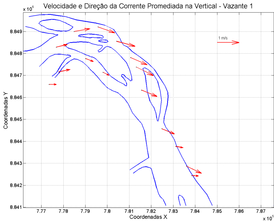
Figura 59: Velocidade e direção da corrente promediada na vertical, em cada estação amostral. Campanha 2 – Vazante 1 – data: 24/01/2016.
