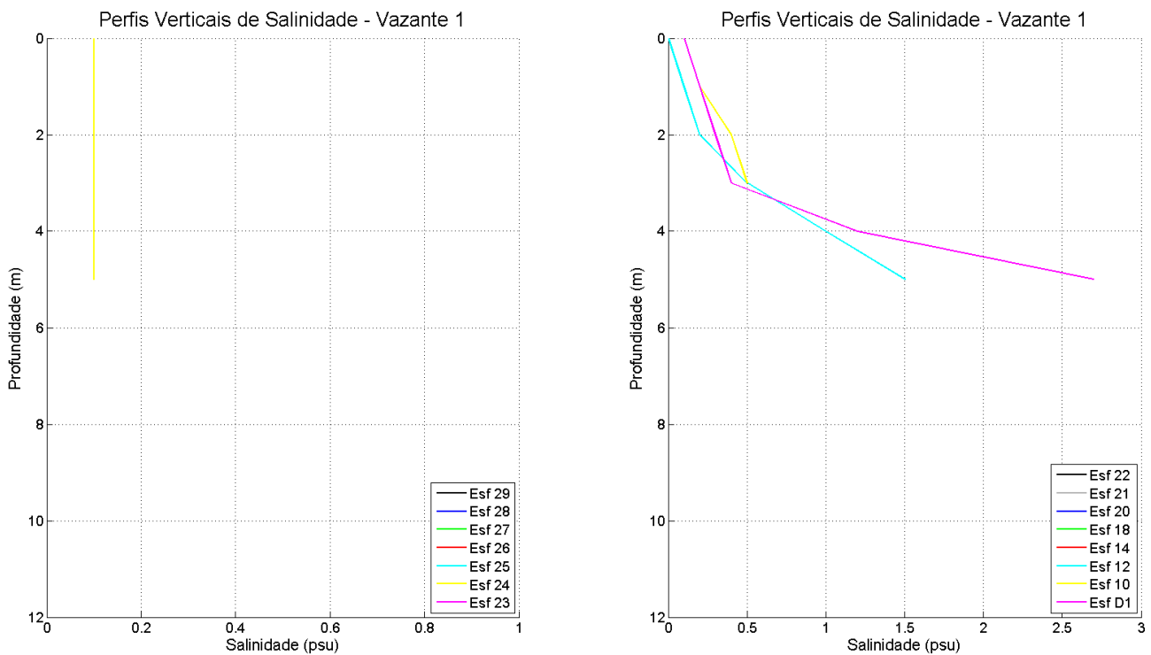
Figura 71: Perfis verticais de salinidade da água em período de maré enchente, para cada estação amostral. Campanha 2 – Vazante 1 – data: 24/01/2016. Resolução CONAMA 357/2005 (I - águas doces: águas com salinidade igual ou inferior a 0,5 ‰)
