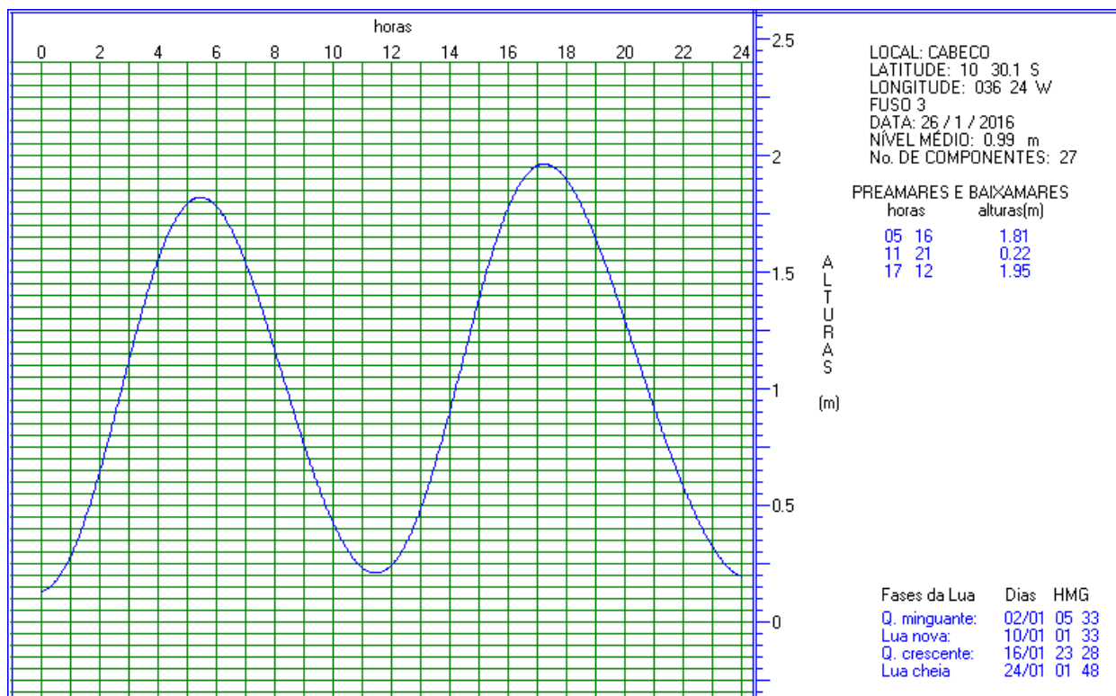
Figura 23. Previsão de maré para o dia 26/01/2016 (campanha 2), para a localidade de Cabeço, localizada na foz do Rio São Francisco.
