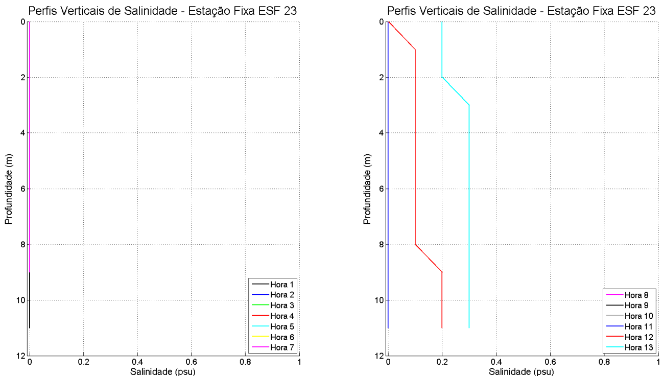
Figura 96: Perfis verticais de salinidade para a estação fixa ESF_23. Campanha 2 – 12 horas – data: 26/01/2016. Resolução CONAMA 357/2005 (I - águas doces: águas com salinidade igual ou inferior a 0,5 ‰)
