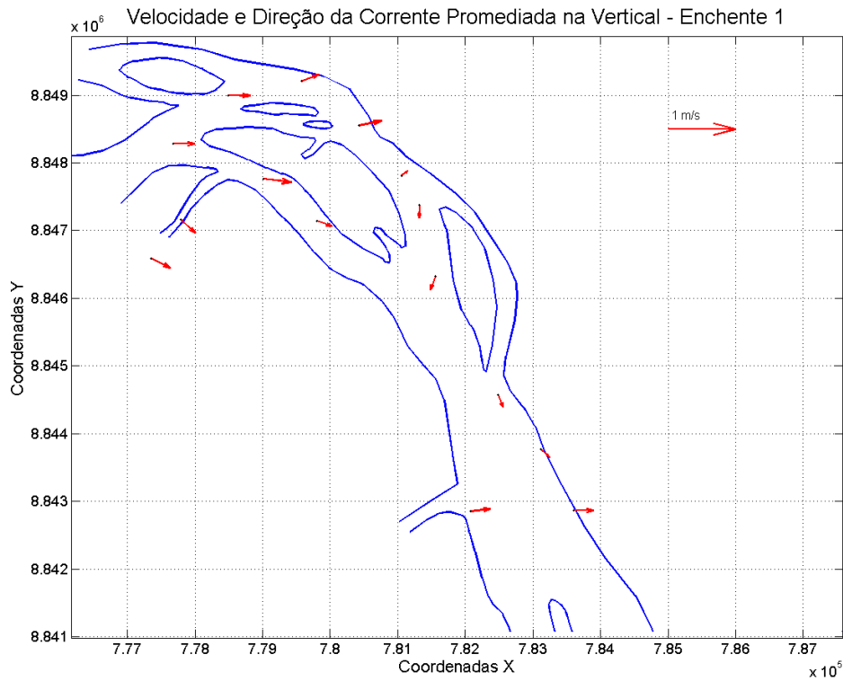
Figura 58: Velocidade e direção da corrente promediada na vertical, em cada estação amostral. Campanha 2 – Enchente 1 – data: 24/01/2016.
