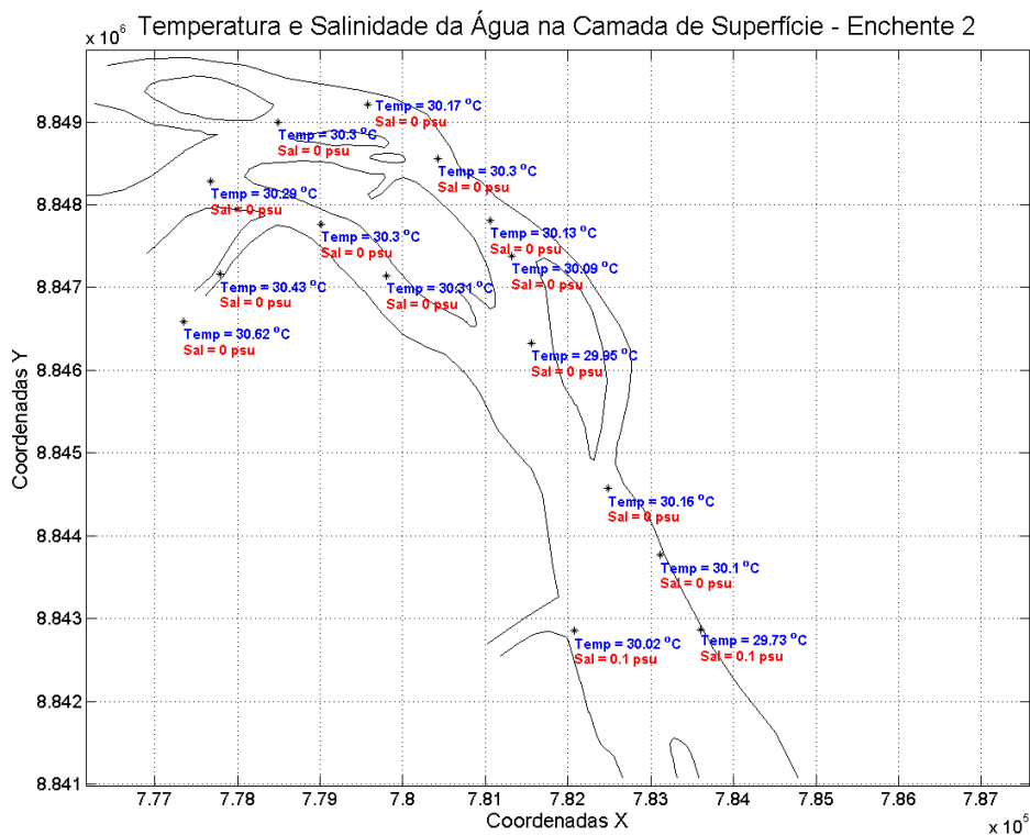
Figura 78: Temperatura e salinidade da água na camada de superfície. Campanha 2 – Enchente 2 – data: 25/01/2016. Resolução CONAMA 357/2005 (I - águas doces: águas com salinidade igual ou inferior a 0,5 ‰)
