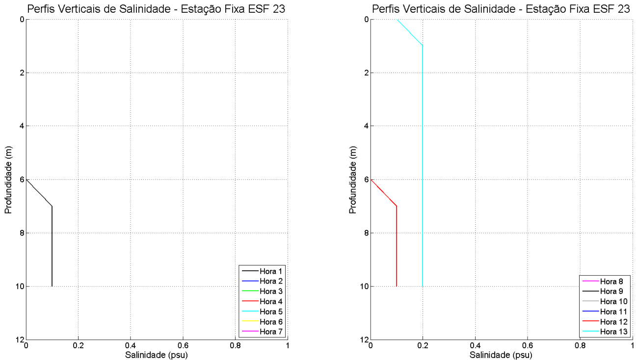
Figura 86: Perfis verticais de salinidade para a estação fixa ESF_23. Campanha 1 – 12 horas – data: 12/01/2016. Resolução CONAMA 357/2005 (I - águas doces: águas com salinidade igual ou inferior a 0,5 ‰)
