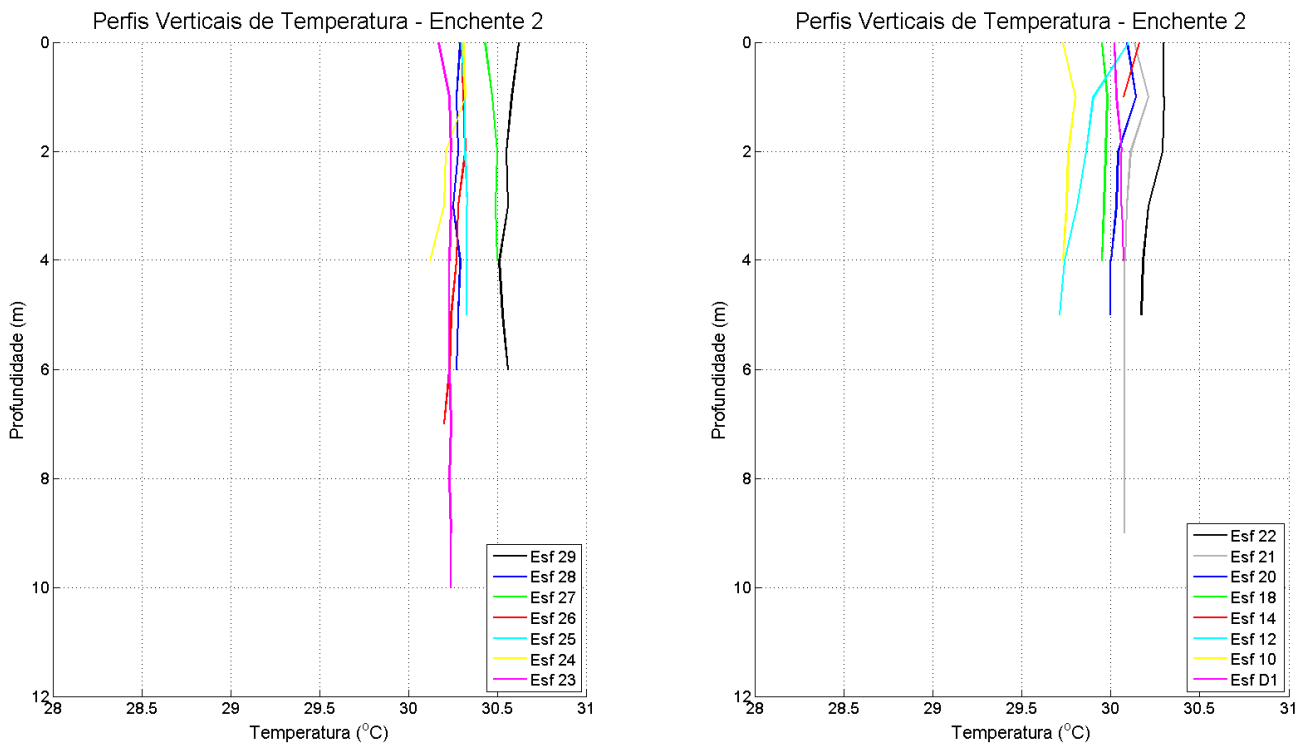
Figura 64: Perfis verticais de temperatura da água em período de maré enchente, para cada estação amostral. Campanha 2 – Enchente 2 – data: 25/01/2016.
