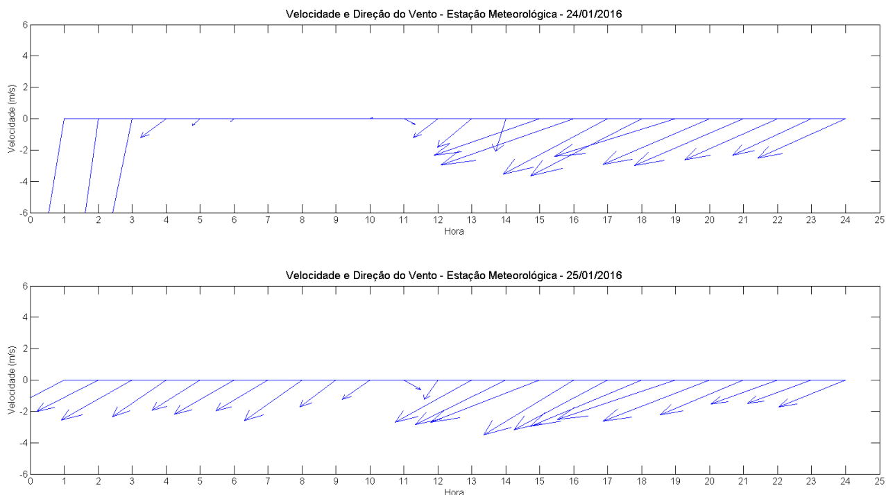
Figura 105: Diagrama stick plot dos dados de ventos medidos no dia 24/01/2016 (painel superior) e 25/01/2016 (painel inferior).
