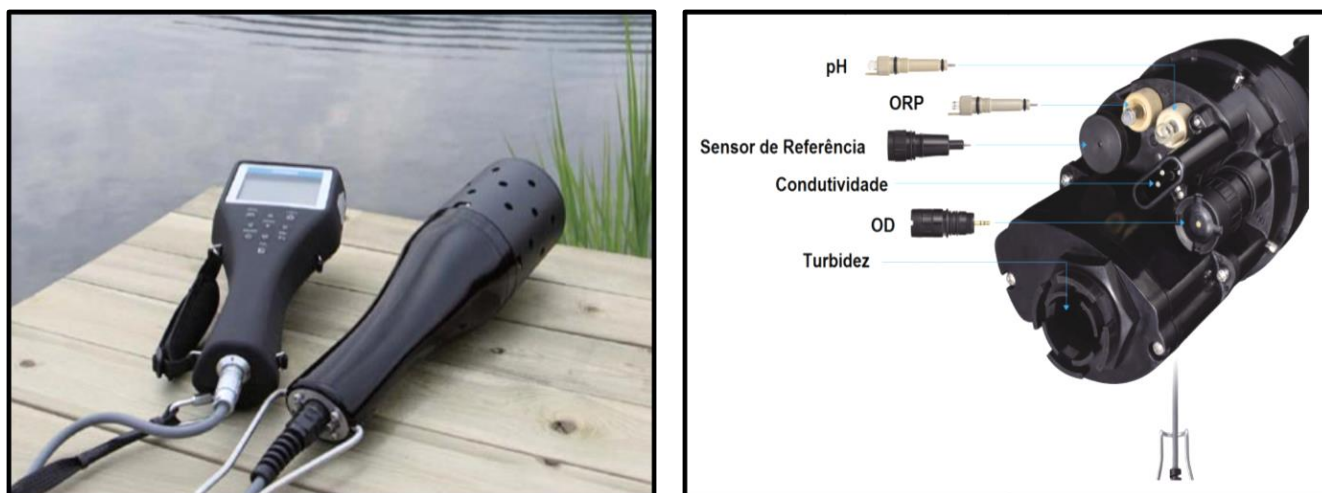
Figura 4. Equipamento utilizado nas medições de temperatura, condutividade e salinidade da água no baixo estuário do Rio São Francisco – sonda multiparâmetro Horiba, série U-50. No painel direito os detalhes dos sensores.
