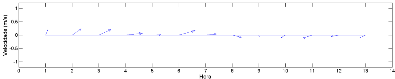
Figura 98: Diagrama stick plot das correntes em superfície (painel superior) e fundo (painel inferior), para a estação fixa ESF_27. Campanha 2 – 12 horas – data: 27/01/2016.
