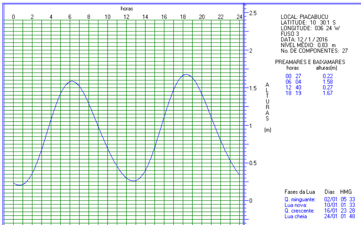
Figura 12. Previsão de maré para o dia 12/01/2016 (campanha 1), para a localidade de Piaçabuçu, localizada na margem do Rio São Francisco.
