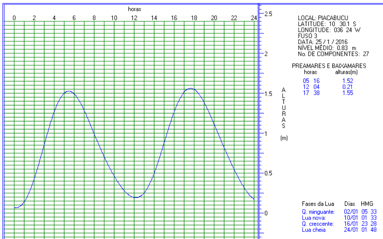
Figura 20. Previsão de maré para o dia 25/01/2016 (campanha 2), para a localidade de Piaçabuçu, localizada na margem do Rio São Francisco.
