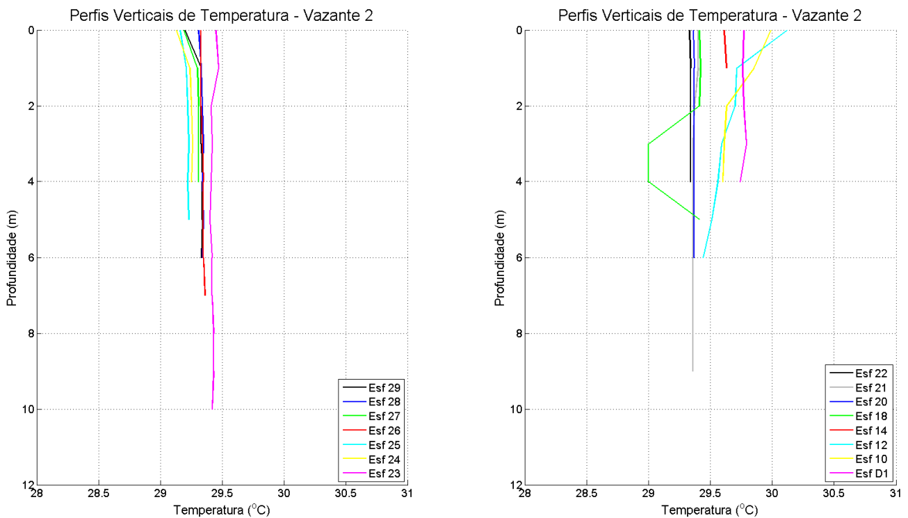
Figura 65: Perfis verticais de temperatura da água em período de maré enchente, para cada estação amostral. Campanha 2 – Vazante 2 – data: 25/01/2016.
