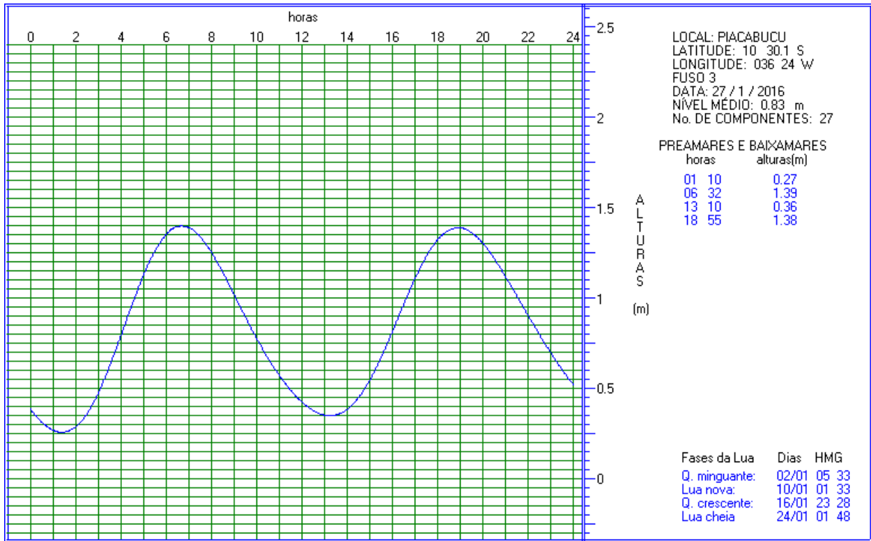
Figura 24: Previsão de maré para o dia 27/01/2016 (campanha 2), para a localidade de Piaçabuçu, localizada na margem do Rio São Francisco.
