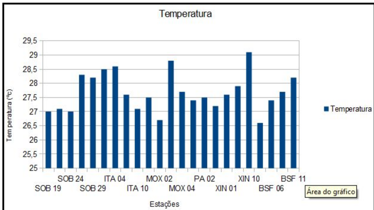
Figura 3: Temperatura da água nas estações de monitoramento. Fonte: Adaptado de Chesf: Correspondência CE-SOC-354/2016.
