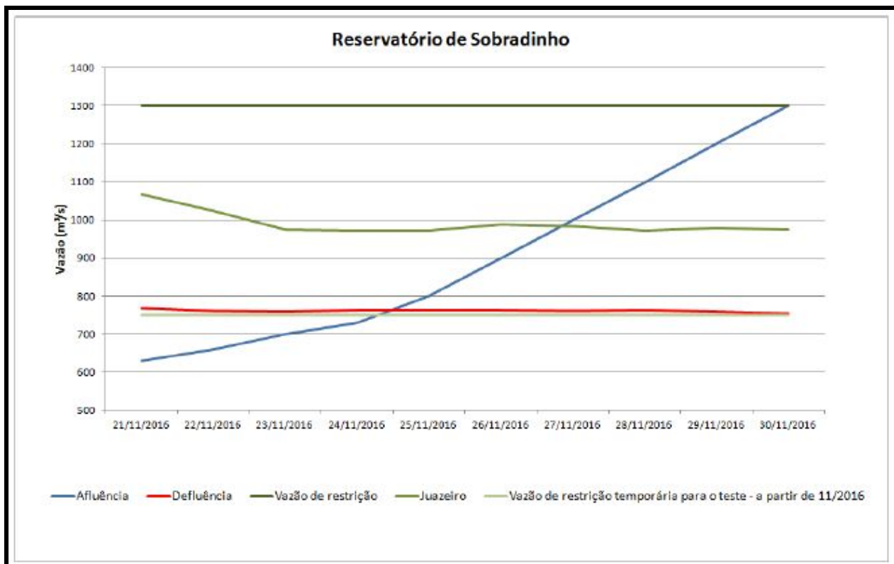
Figura 2: Vazões afluentes ao reservatório de Sobradinho. Fonte: Companhia Hidro Elétrica do São Francisco, Correspondência CE-SOC-354/2016.
