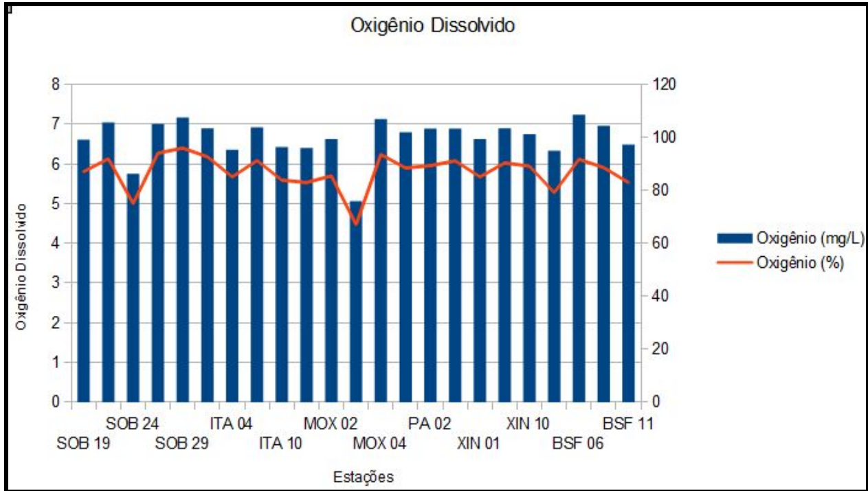
Figura 6: Oxigênio Dissolvido nas estações de monitoramento. Fonte: Correspondência CE-SOC-354/2016.
