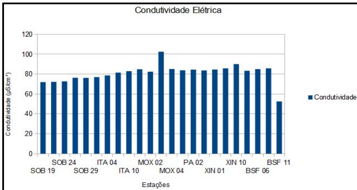
Figura 5: Condutividade elétrica nas estações de monitoramento. Fonte: Correspondência CE-SOC-354/2016.
