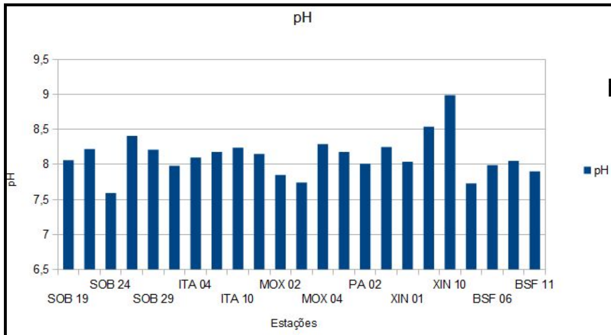
Figura 4: pH nas estações de monitoramento. Fonte: Correspondência CE-SOC-354/2016.
