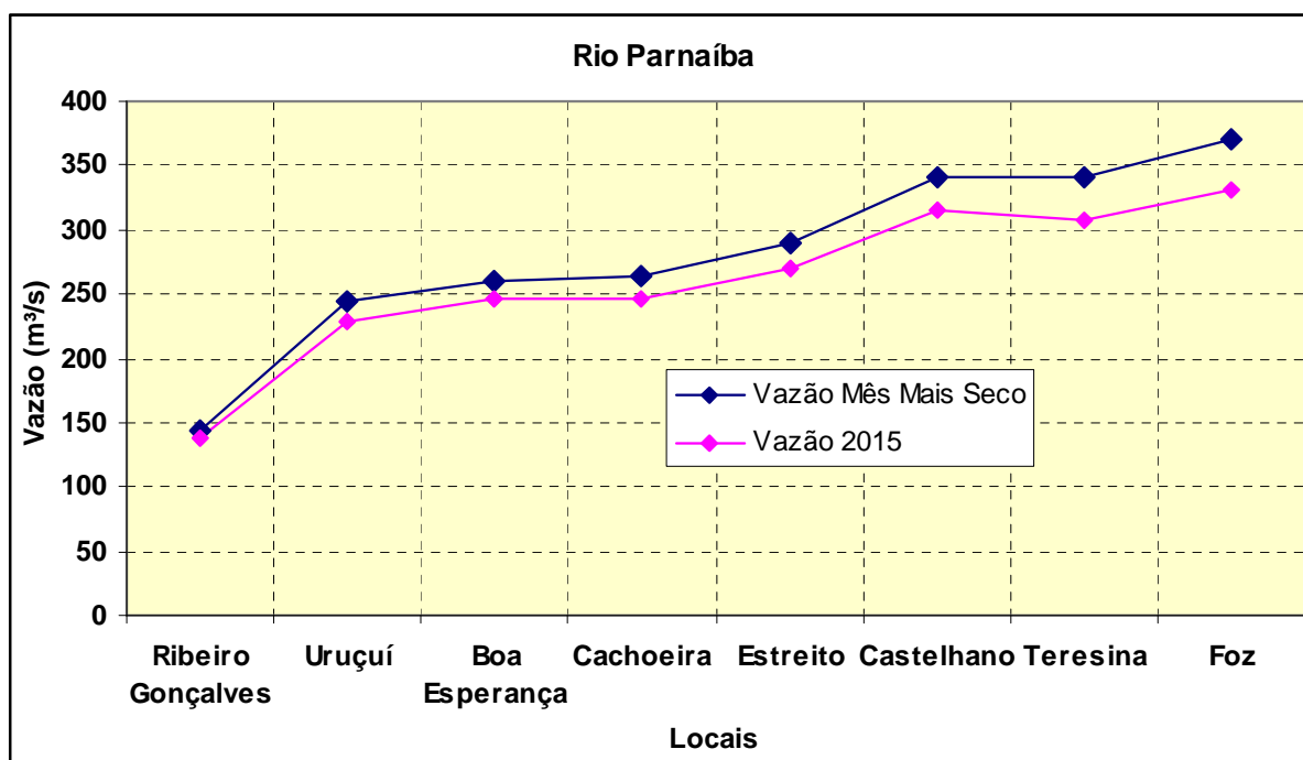
Gráfico 3.3-4 Diagrama esquemático com os aproveitamentos – Vazão Mínima.
