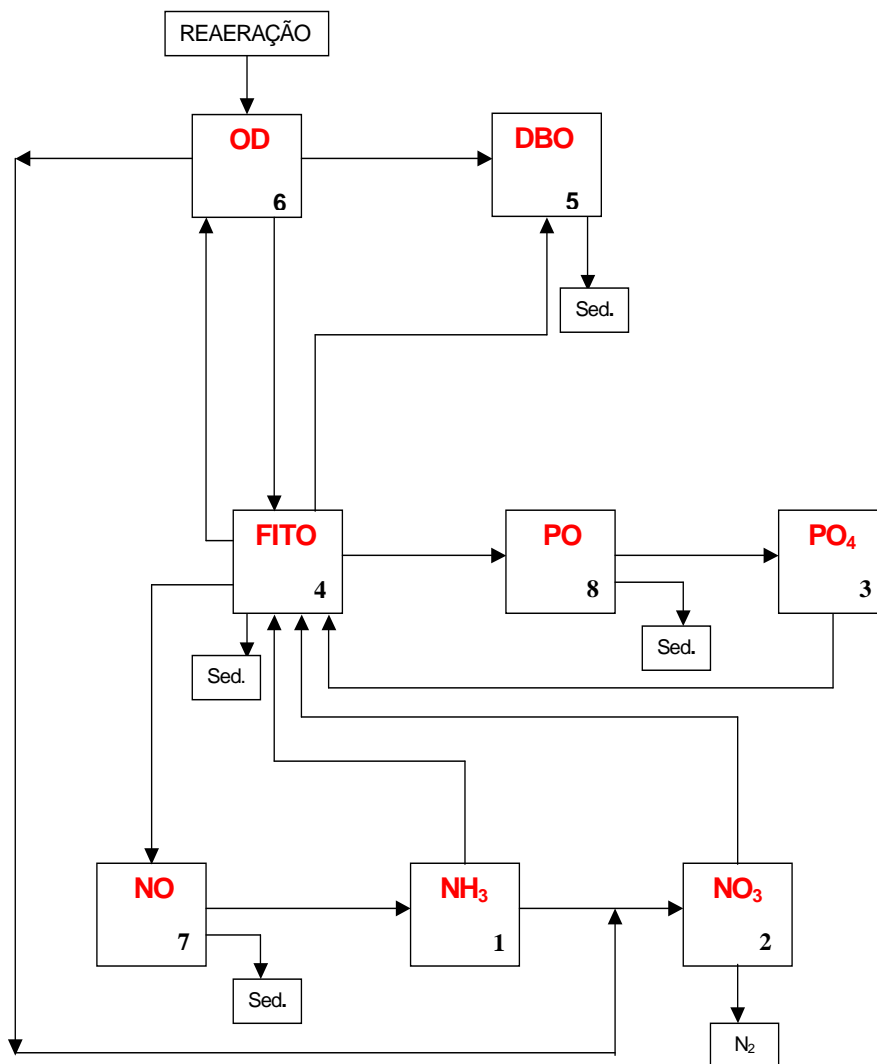
Figura 1.1-2 Estrutura do Módulo EUTRO4 Original
