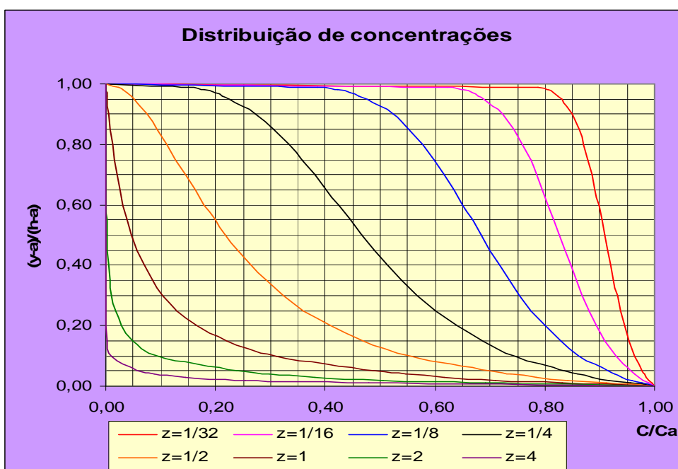
Gráfico 2.6-1 Distribuição de Concentrações ao longo da vertical com a=0,05, h . Fonte: Vanoni, 1977.
