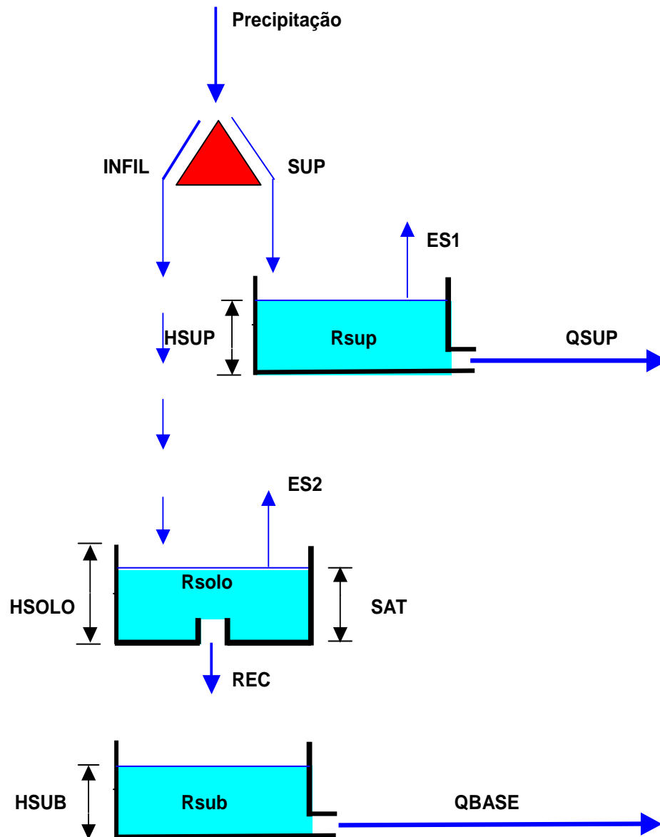
Figura 1.1-1 Representação Esquemática do Modelo de Simulação
