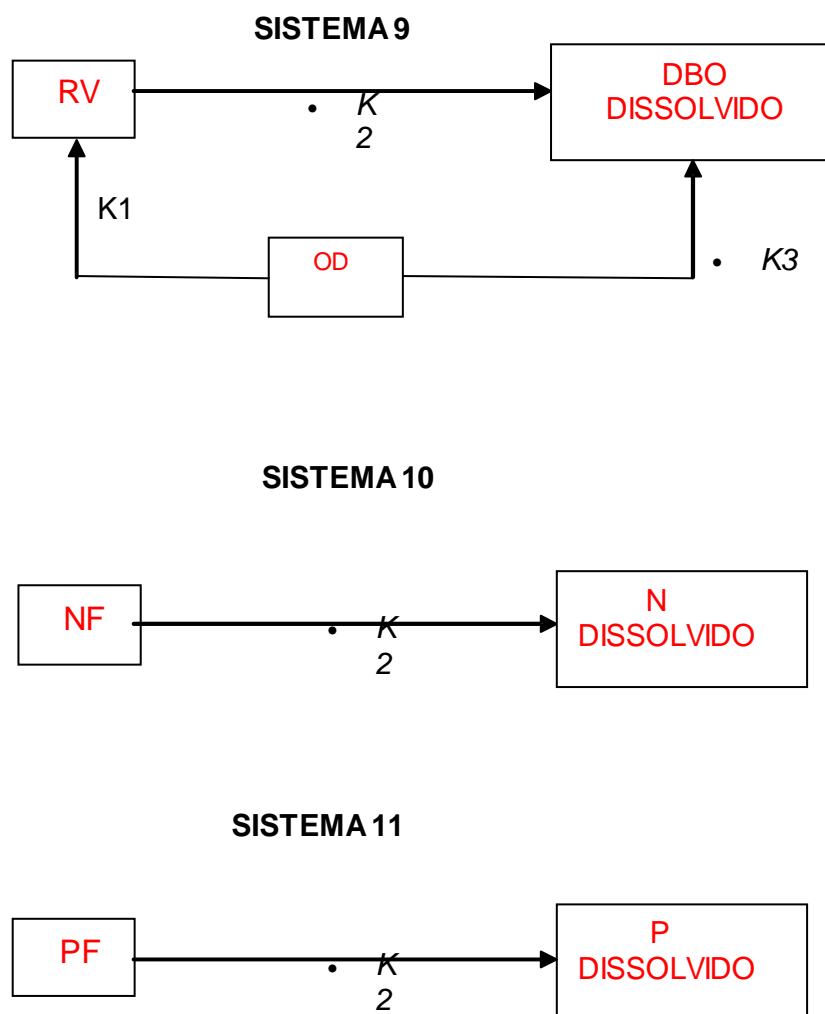
Figura 1.1-4 Representações Cinéticas dos SISTEMAS 9, 10 e 11
