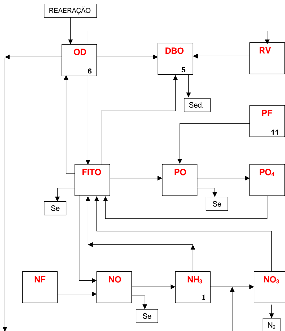
Figura 1.1-3 Estrutura do Módulo EUTRO4 Modificado
