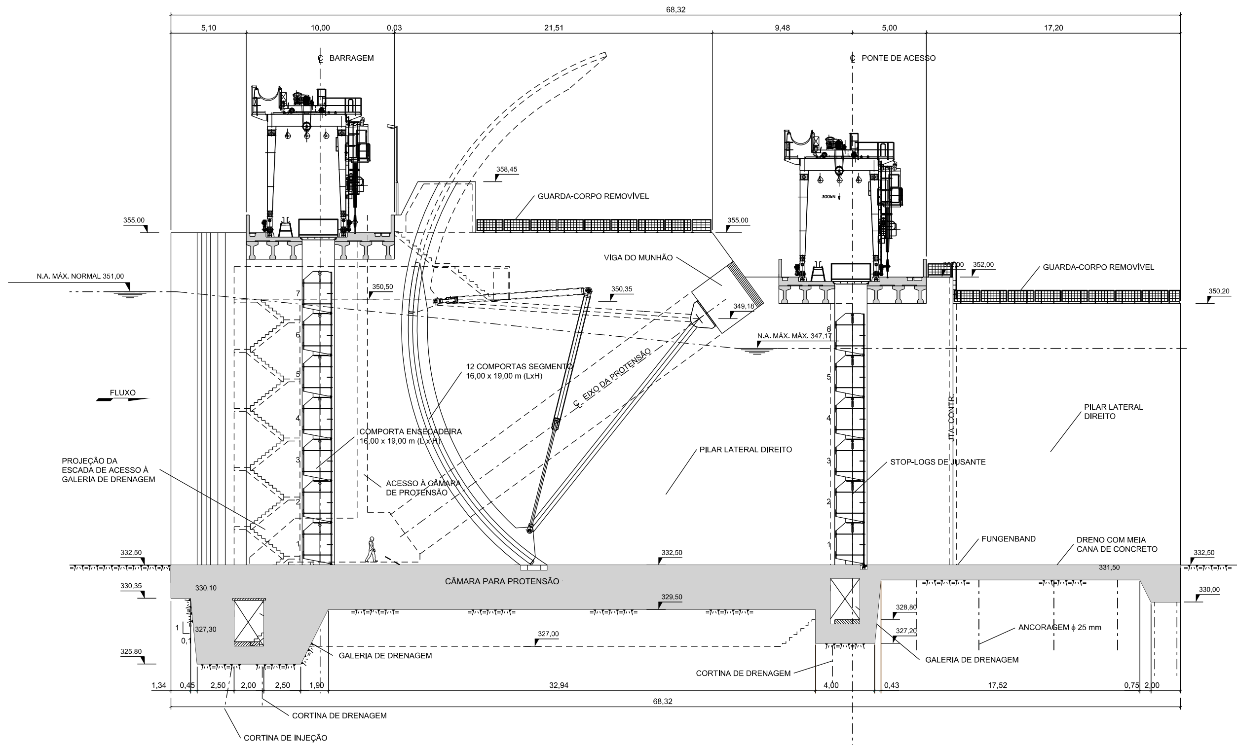
SEÇÃO TÍPICA - PILAR LATERAL DIREITO 1:250
