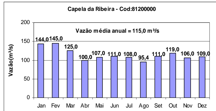
FIGURA 12.1.1/01 – HISTOGRAMAS DAS VAZÕES MÉDIAS MENSAIS AO LONGO DO RIO RIBEIRA
