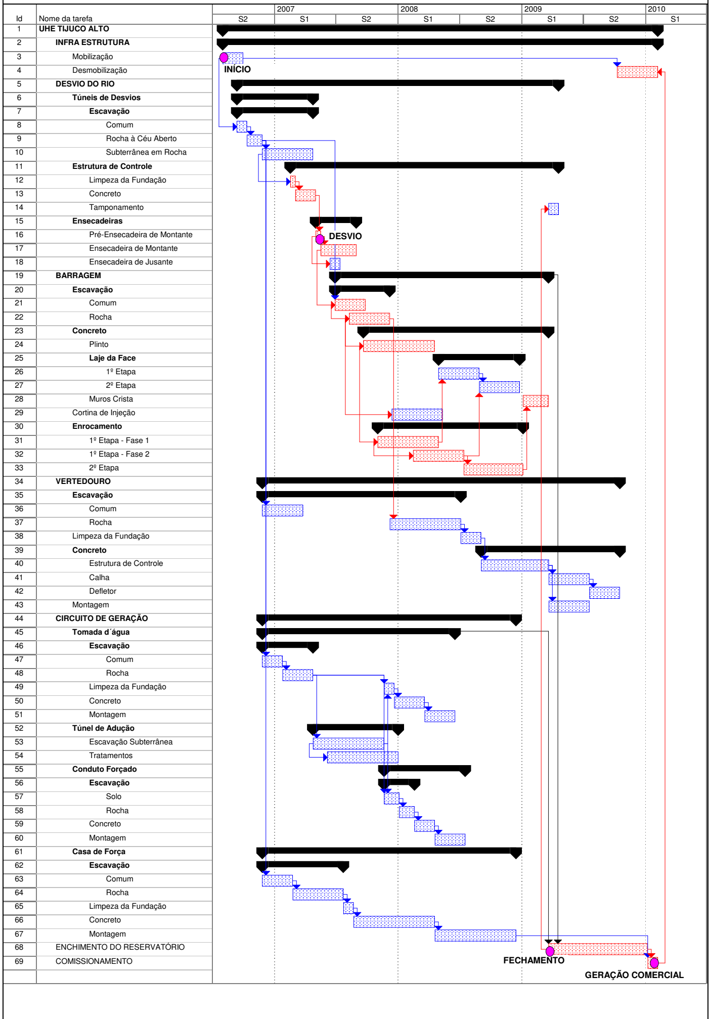
FIGURA 7.17/01 - CRONOGRAMA DE CONSTRUÇÃO
