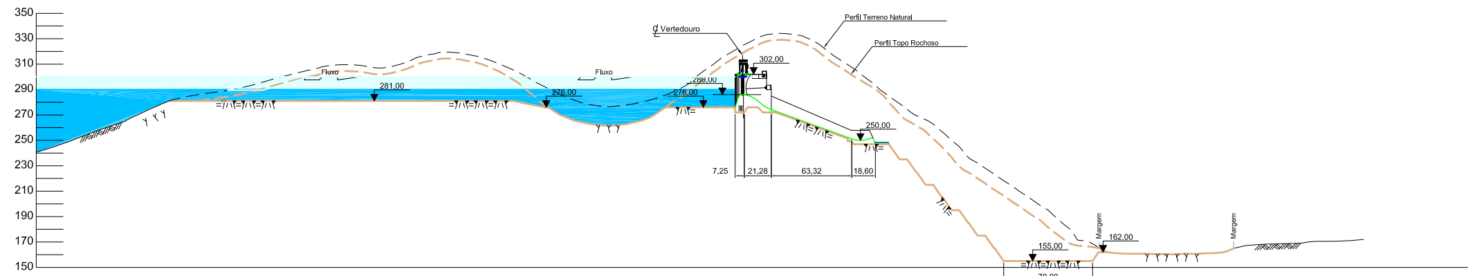
Seção Típica do Vertedouro
