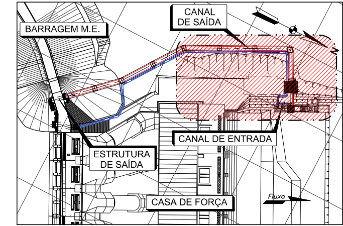
PLANTA CHAVE (Sem escala)
