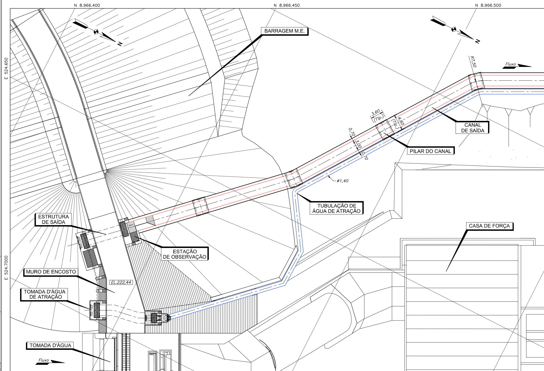
PLANTA
