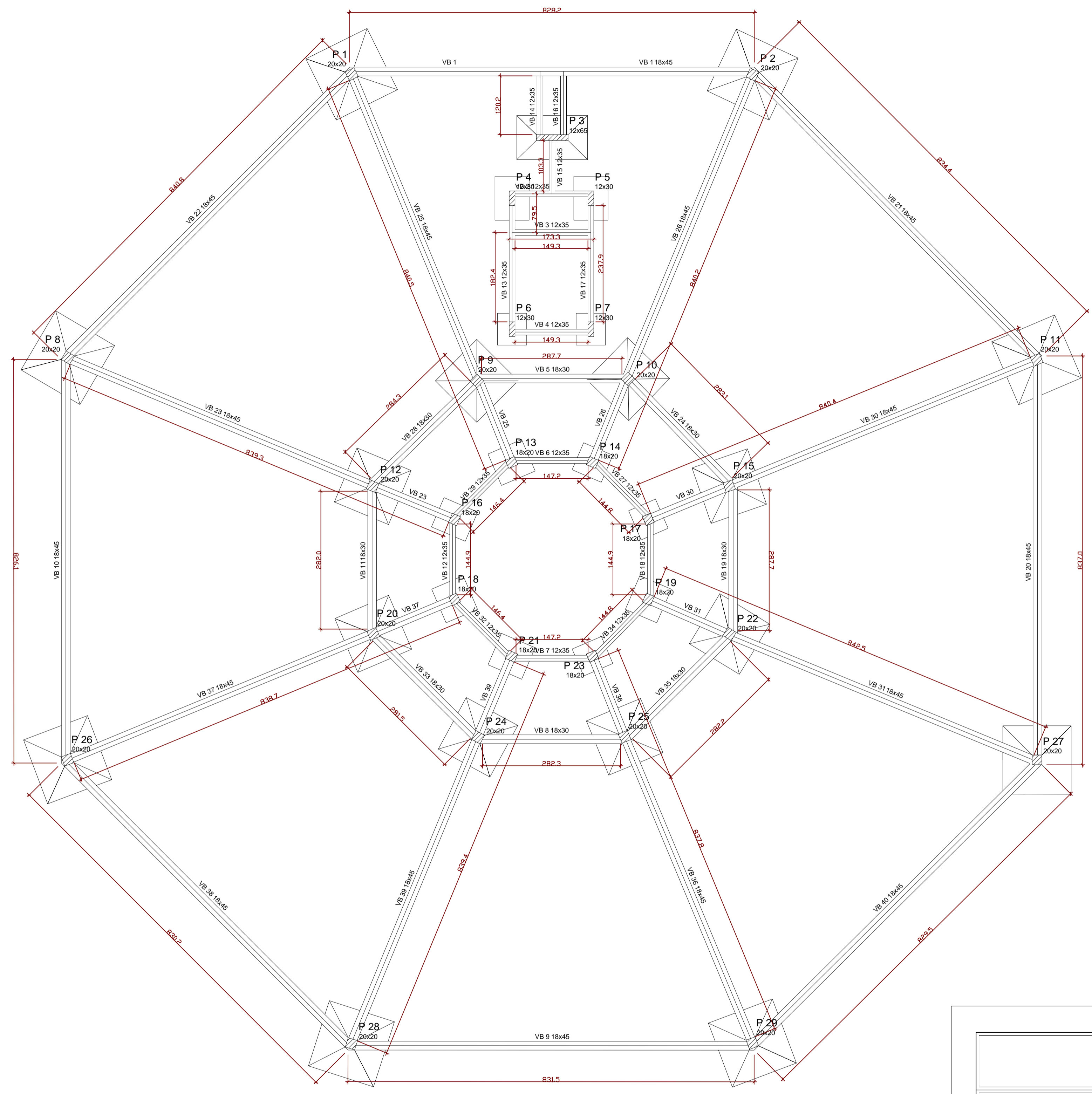
Forma do pavimento terreo escala 1:50
