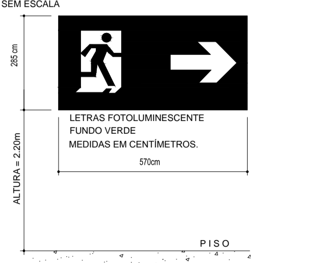
DETALHE 03 - CÓDIGO "13" da NBR 13434-2:2004 PLACA INDICAÇÃO DO SENTIDO (esquerda ou direita) DE UMA SAÍDA DE EMERGÊNCIA (fixada na parede) SEM ESCALA
