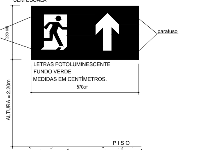
DETALHE 02 - CÓDIGO "14" da NBR 13434-2:2004 PLACA INDICAÇÃO DO SENTIDO (esquerda ou direita) DE UMA SAÍDA DE EMERGÊNCIA (fixada na parede) SEM ESCALA
