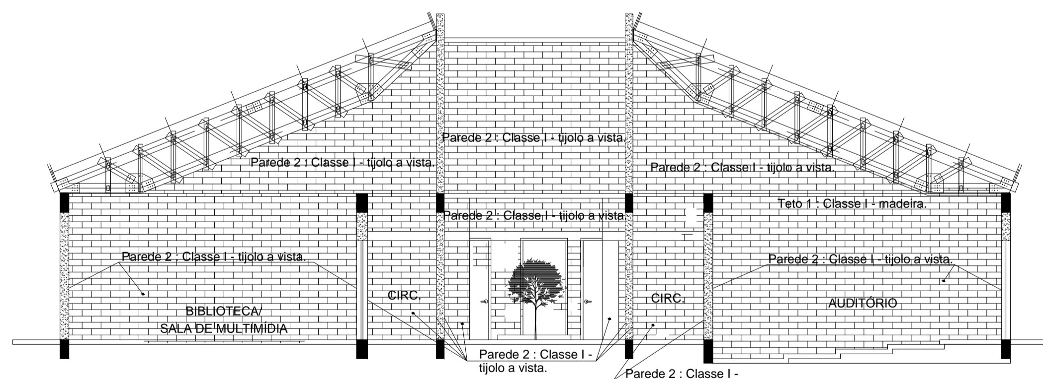
CORTE A-A - CONTROLE DE MATERIAIS DE ACABAMENTO - CMAR ESCALA 1:75
