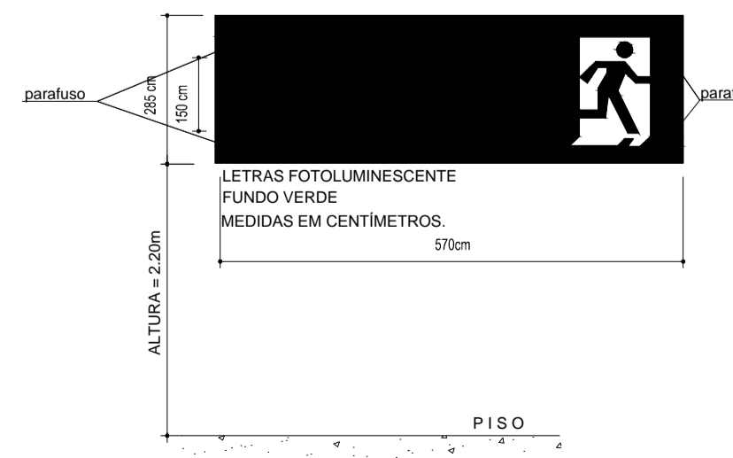
DETALHE 01 - CÓDIGO "17" da NBR 13434-2:2004 PLACA DE SINALIZAÇÃO DE SAÍDA DE EMERGÊNCIA ROTA DE FUGA FINAL (fixadas acima das portas) SEM ESCALA
