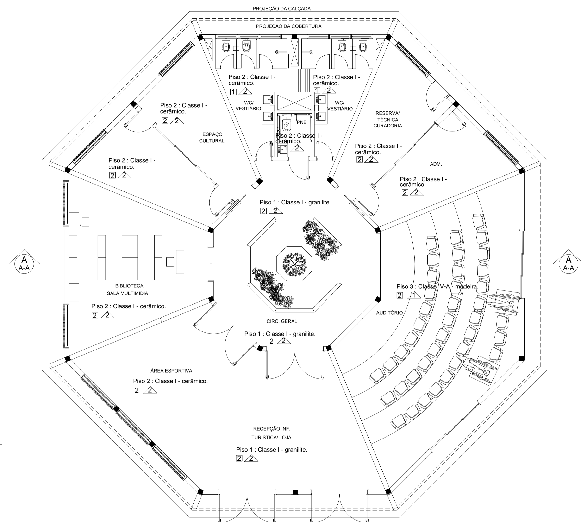
PLANTA BAIXA - CONTROLE DE MATERIAIS DE ACABAMENTO - CMAR ESCALA 1:75
