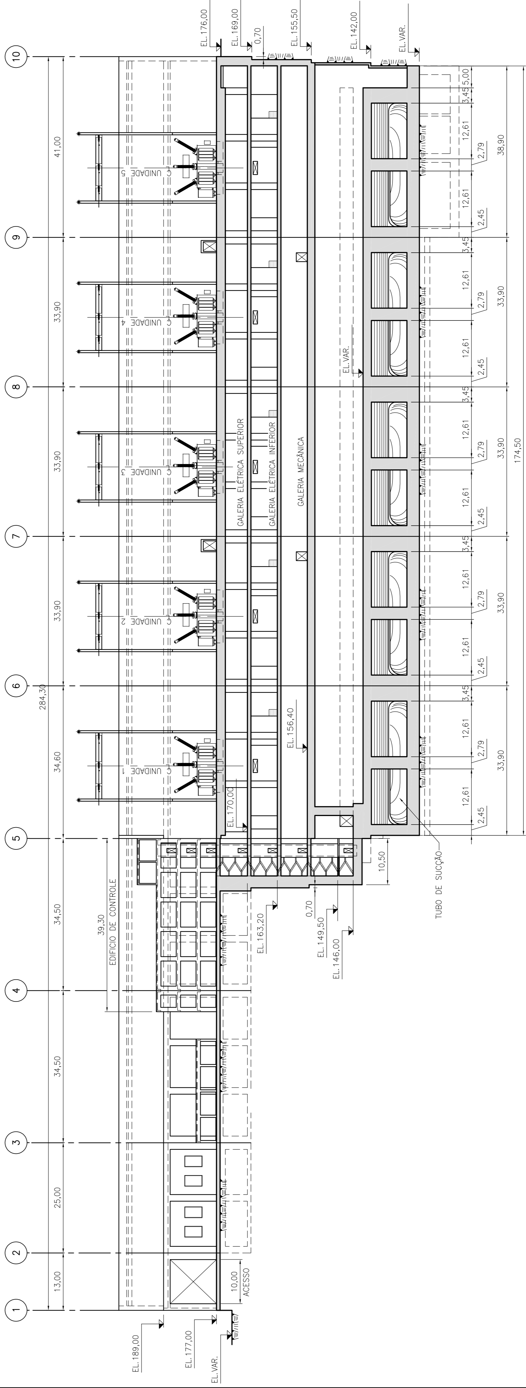
CORTE LONGITUDINAL PELA GALERIAS
