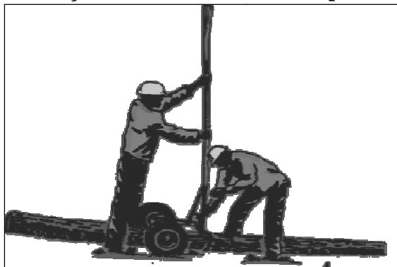
Figura 18 Instalação do carrinho de arraste para remoção de peças de madeira
