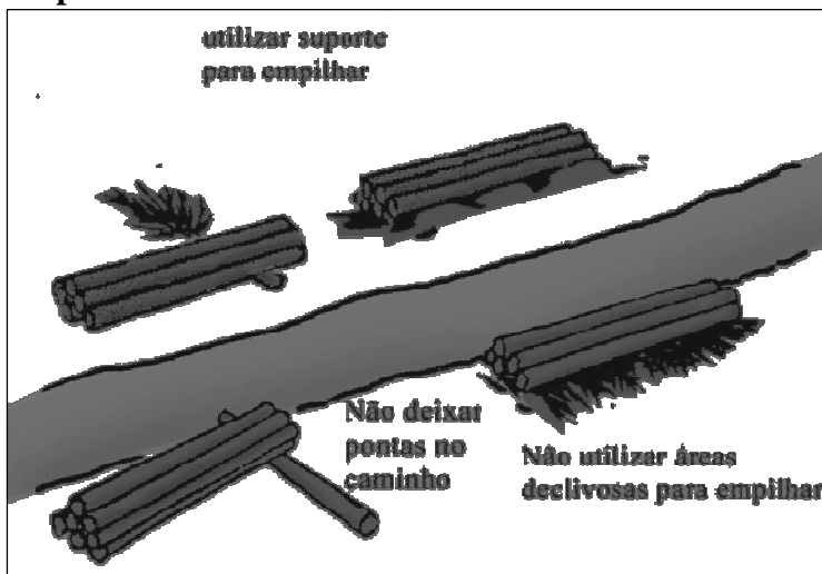
Figura 20 Empilhamento de toras de madeira
