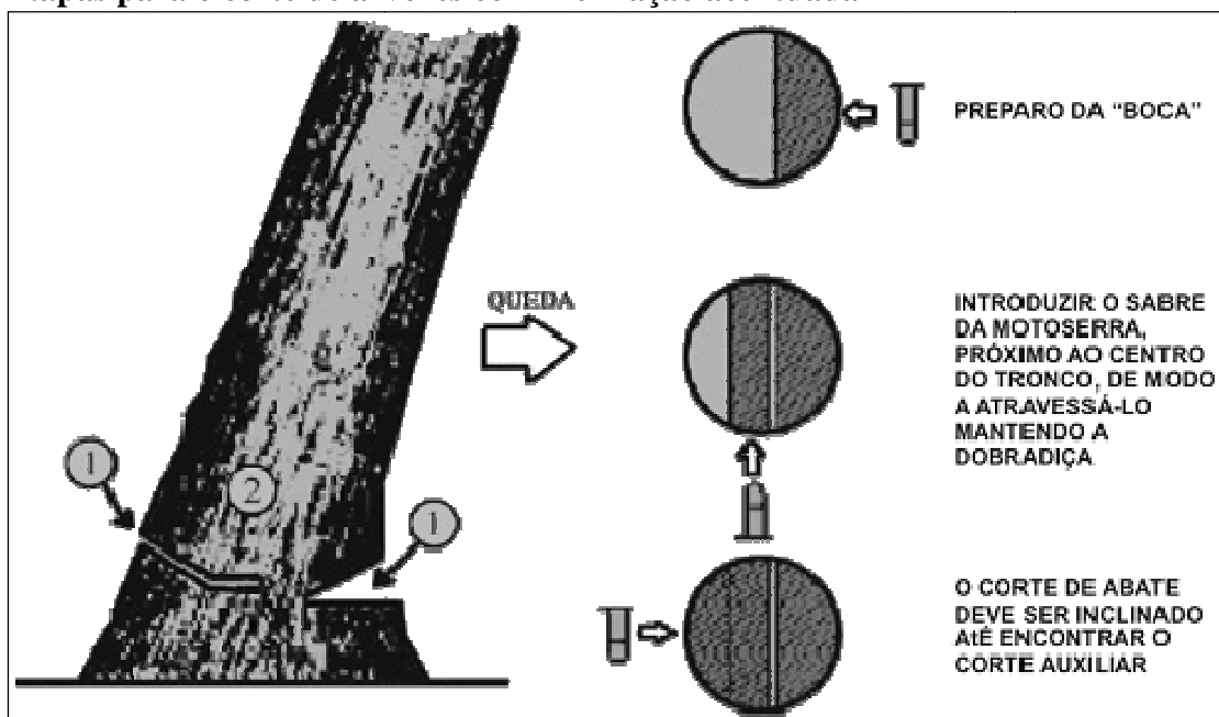
Figura 13 Etapas para o corte de árvores com inclinação acentuada
