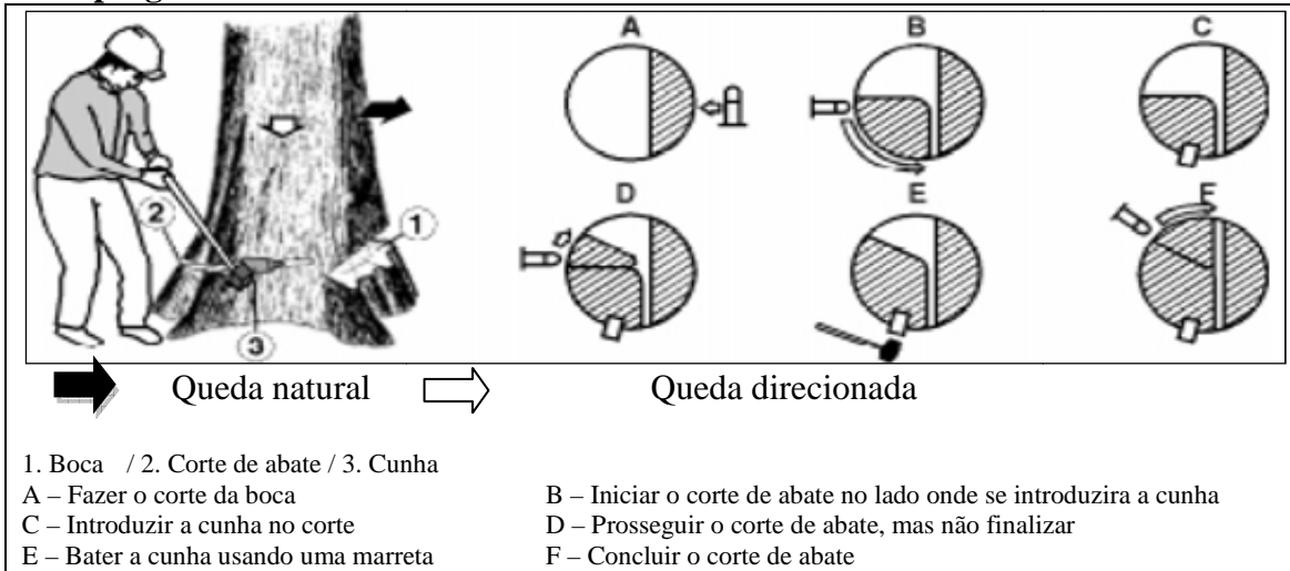
Figura 4 Seqüências de operações de corte para re-direcionamento da queda da árvore com o emprego de cunha
