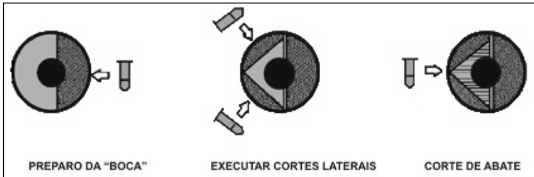
Figura 12 Sequências de operações para o direcionamento da queda de espécies cujo tronco está ocado
