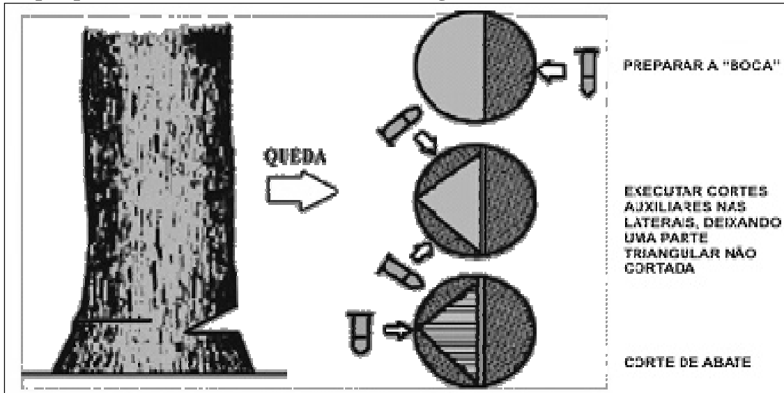
Figura 14 Etapas para o corte de árvores com diâmetro grande
