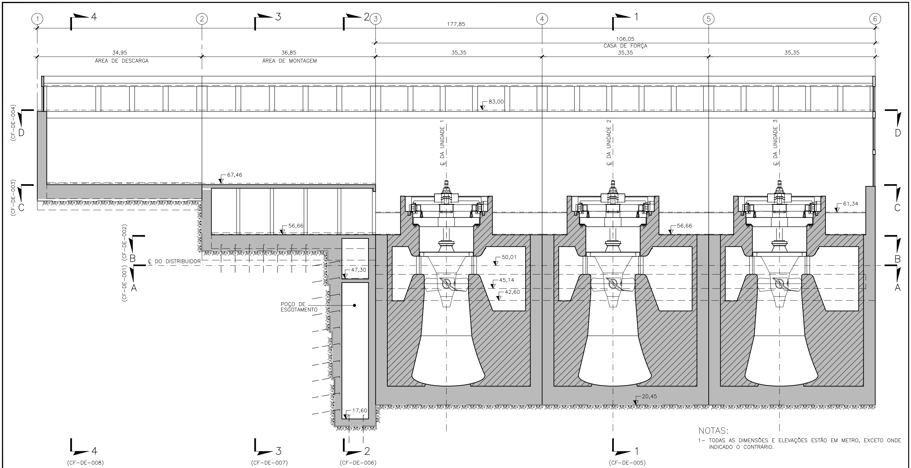
CORTE 5-5
