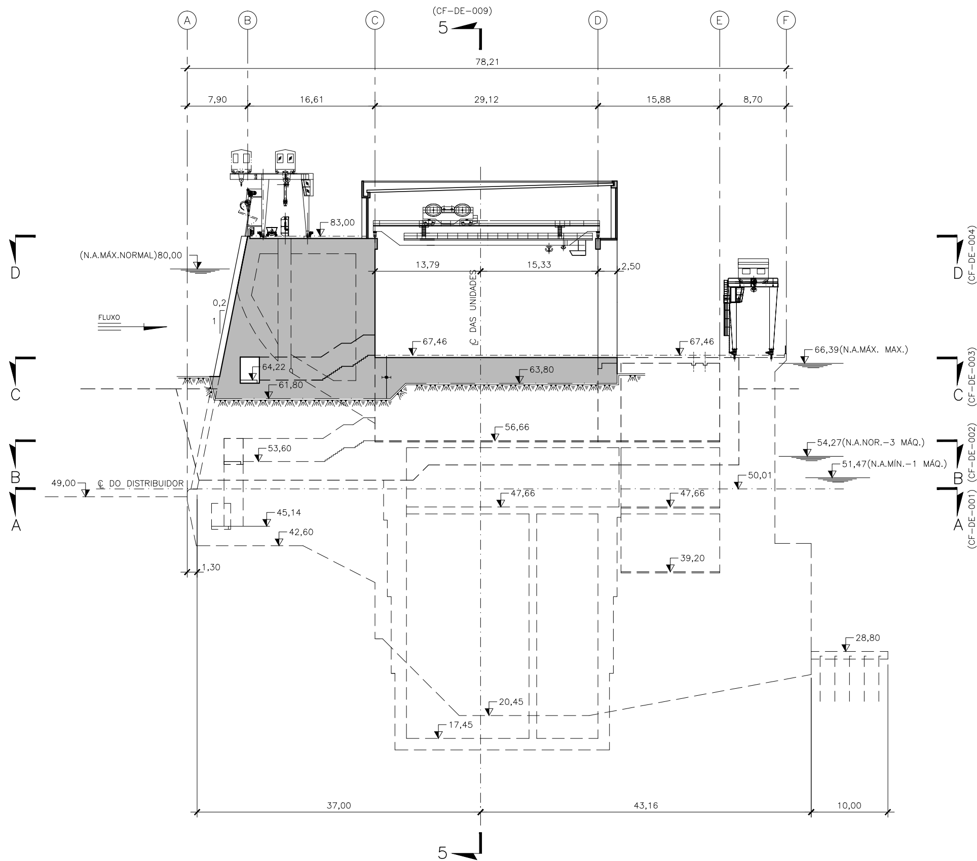
CORTE 4-4 (CF-DE-001/002/003/004)
