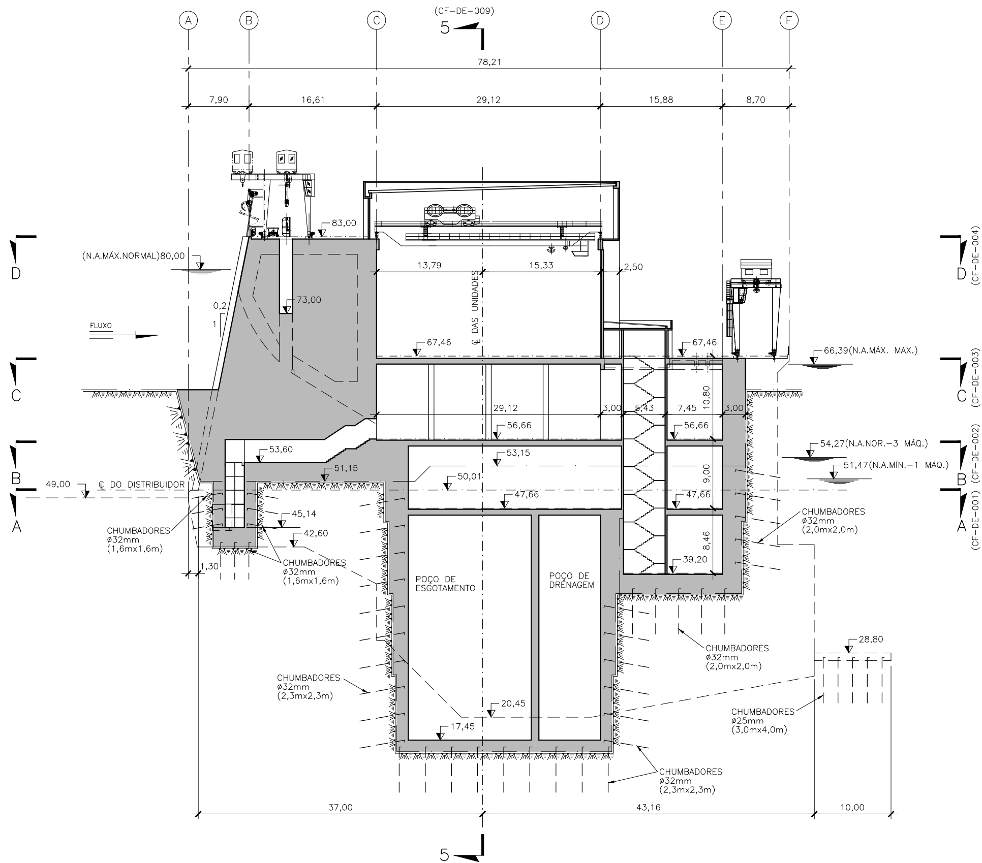
CORTE 2-2 (CF-DE-001/002/003/004)
