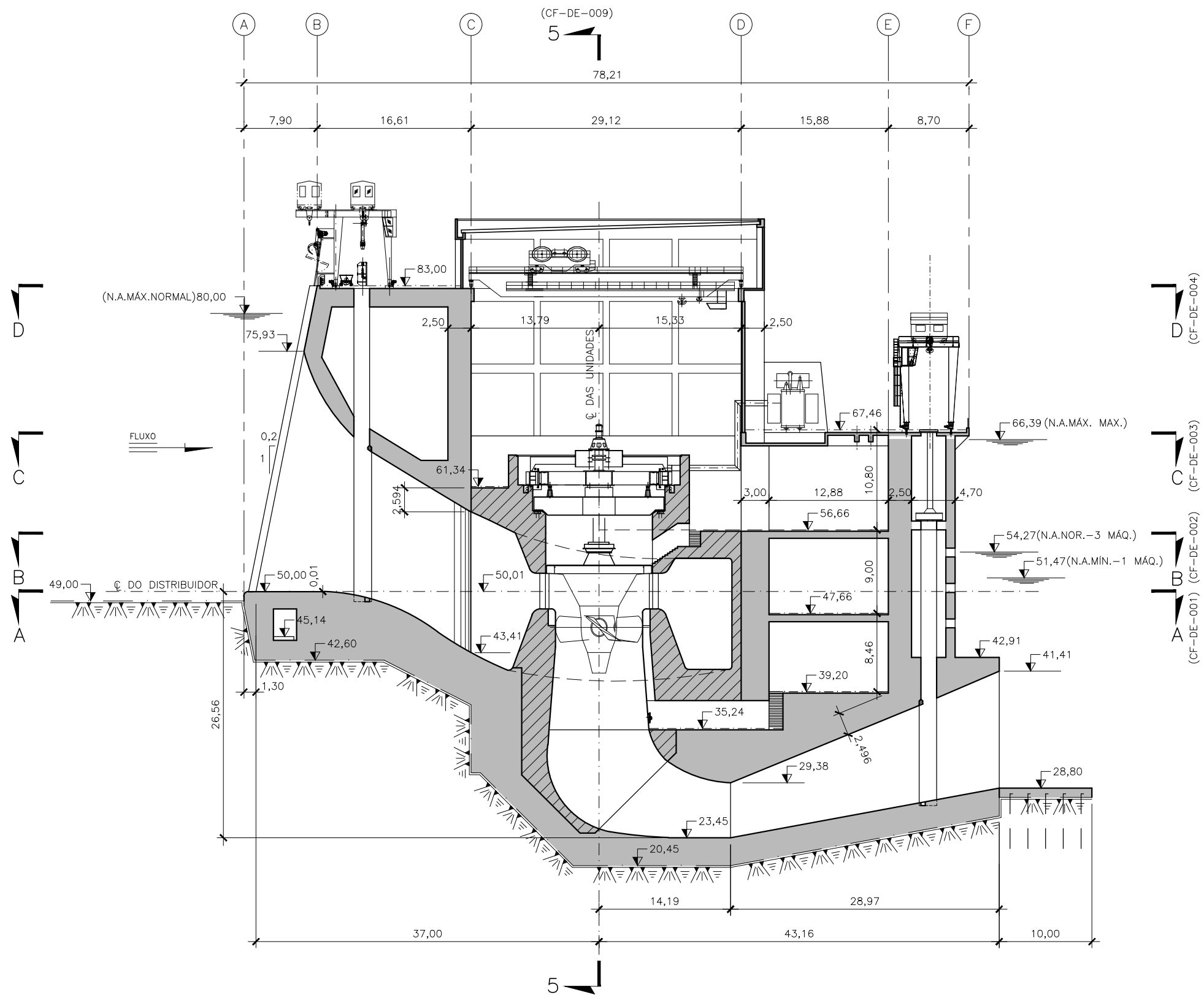
CORTE 1-1 (CF-DE-001/002/003/004)
