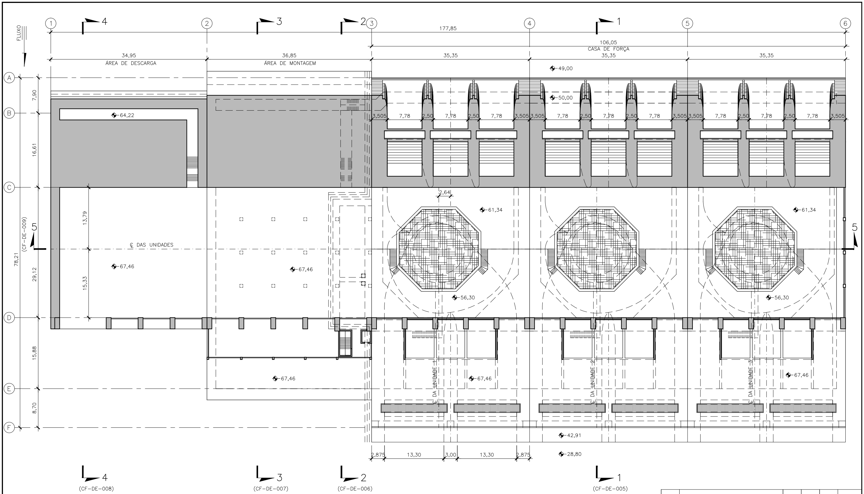
PLANTA C-C
