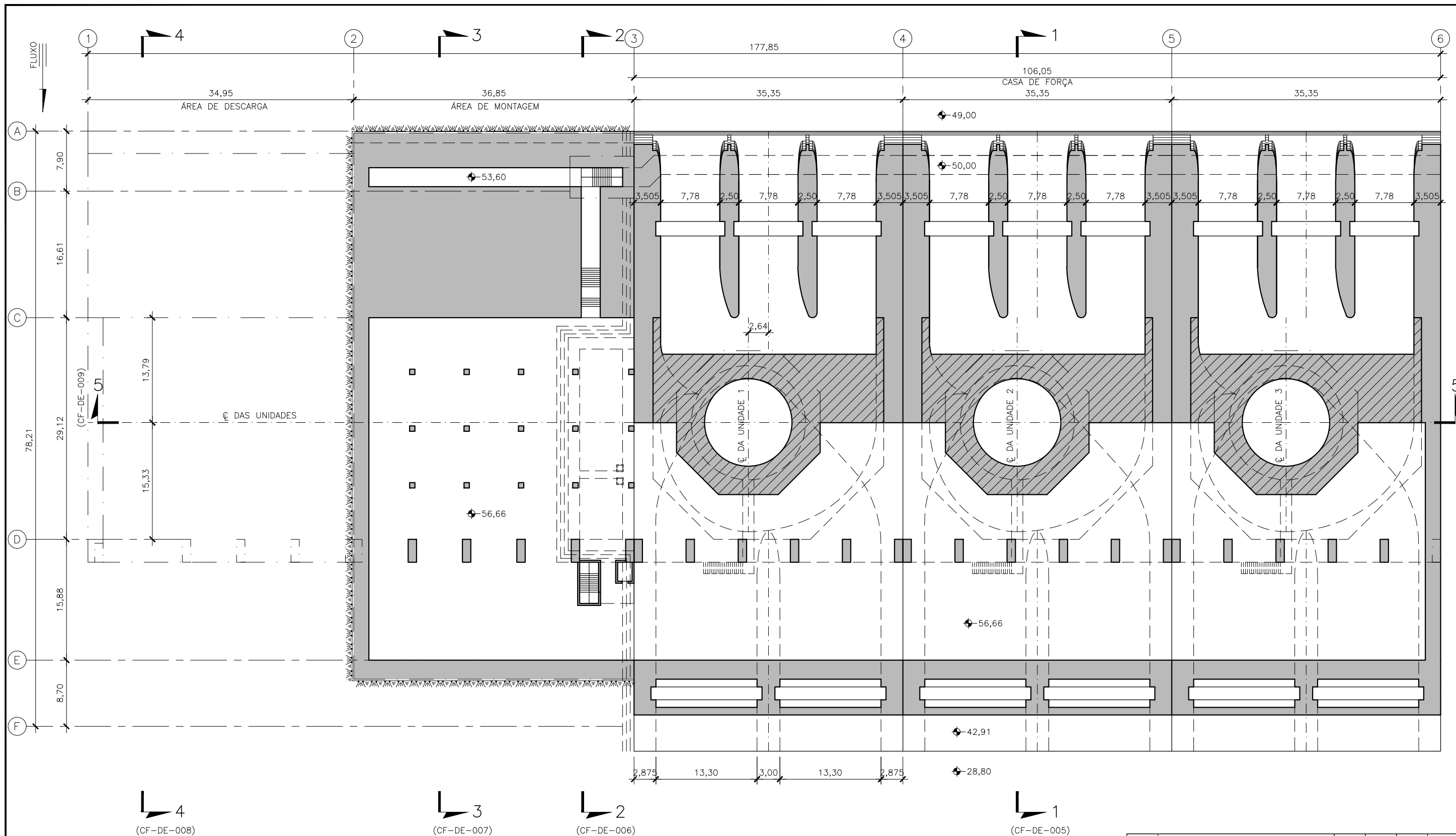
PLANTA B-B
