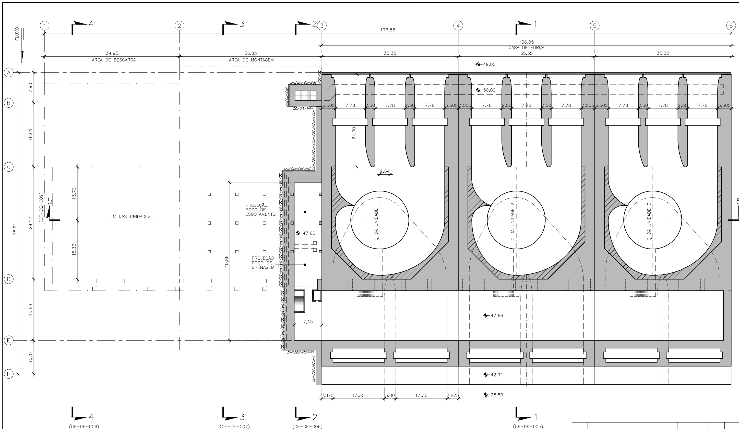
PLANTA A-A
