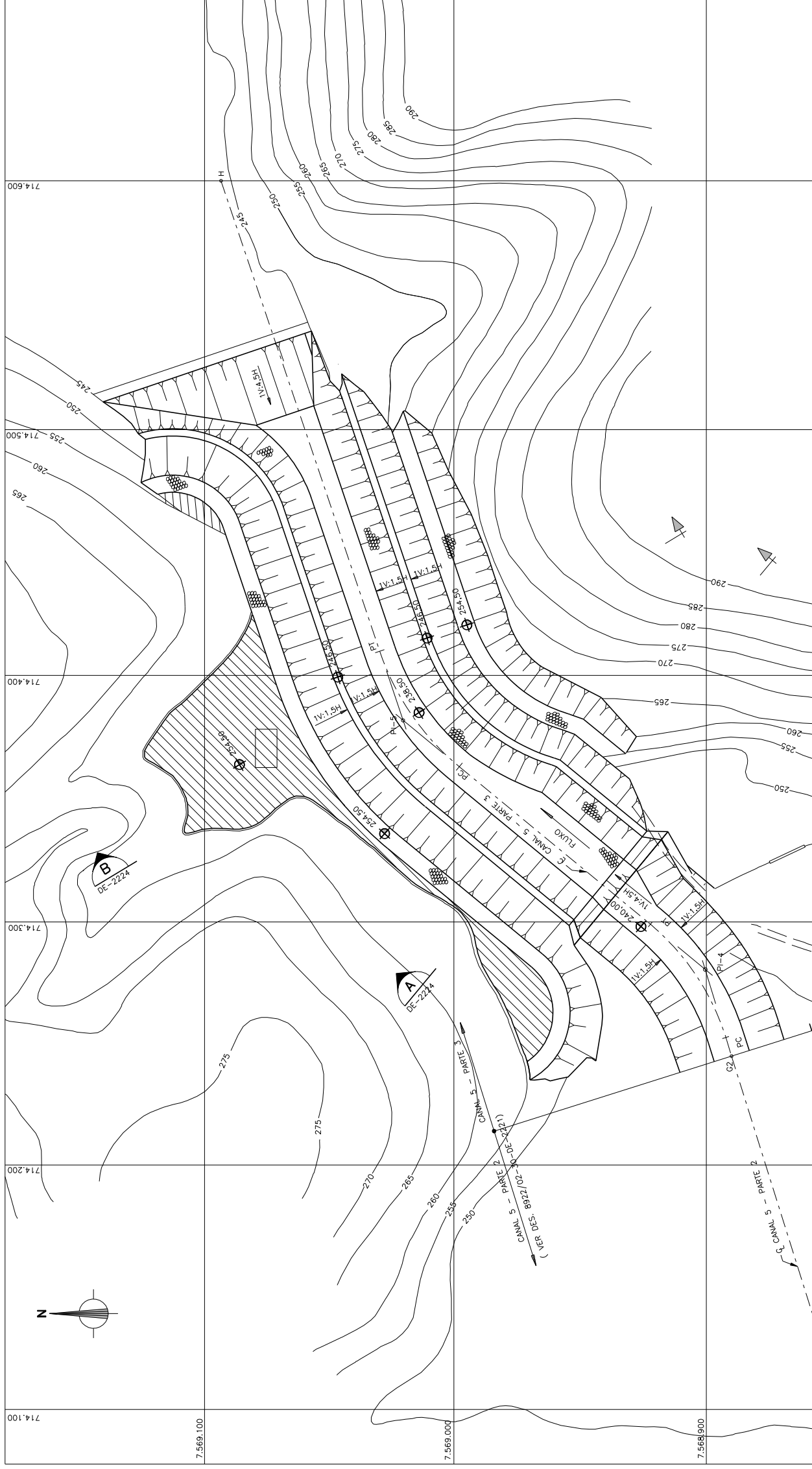
PLANTA 1:1000
