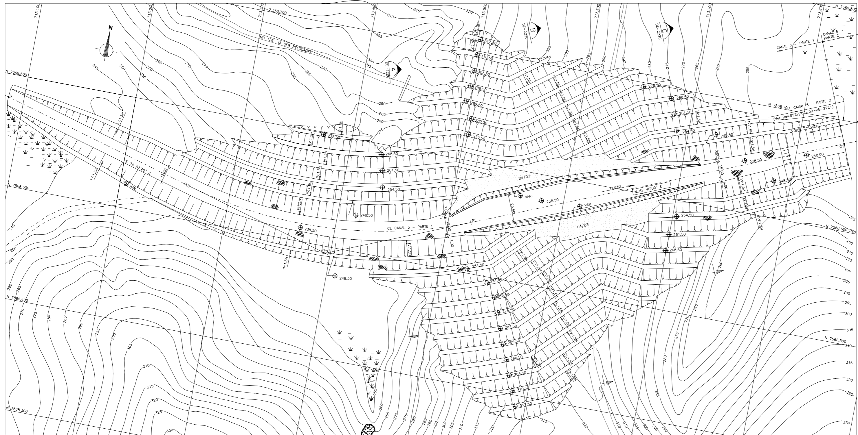
PLANTA 1:1000
