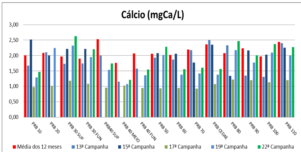
Figura VII-25 - Resultados de Cálcio – Rio Paraíba do Sul
