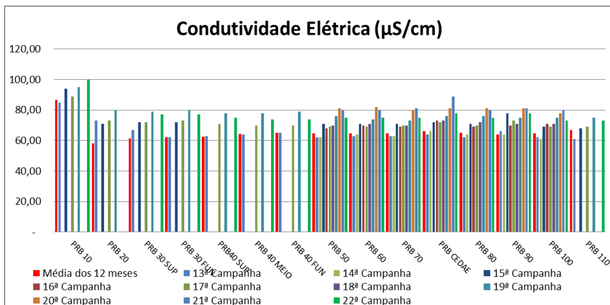
Figura VII-13 - Resultados de Condutividade Elétrica – Rio Paraíba do Sul
