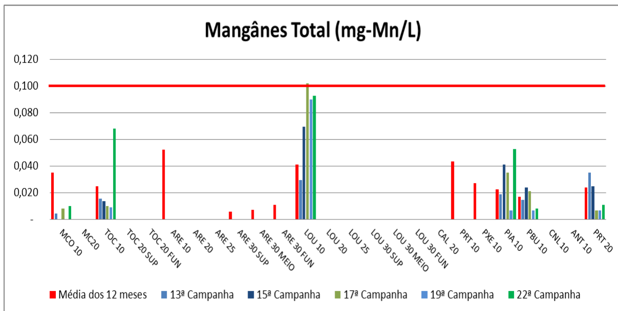
Figura VII-56 - Resultados de Manganês - Tributários
