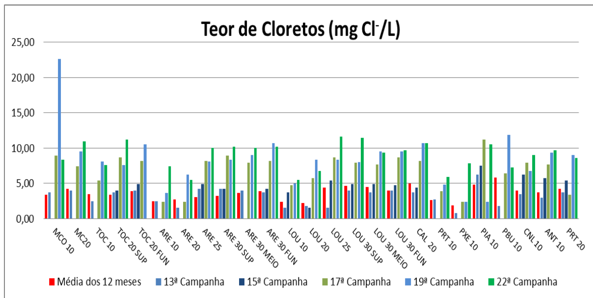
Figura VII-34 - Resultados de Teor de Cloretos - Tributários
