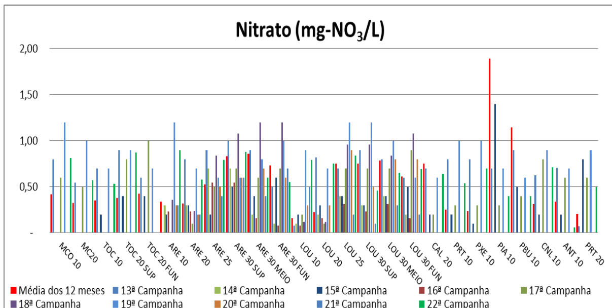
Figura VII-38 - Resultados de Nitrato - Tributários
