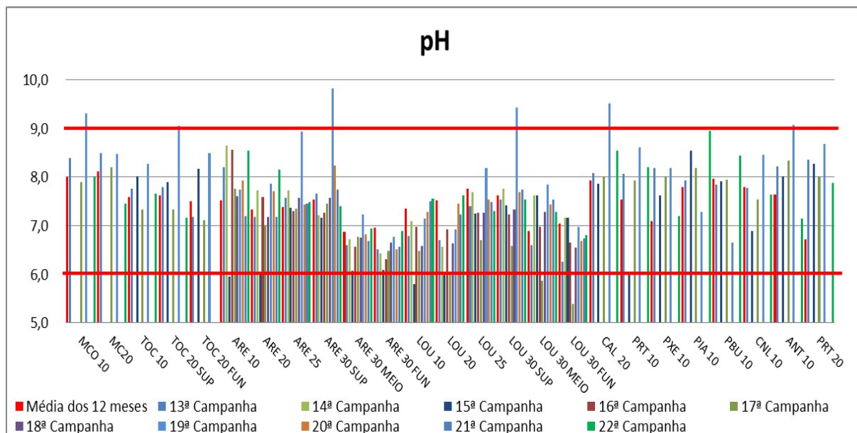
Figura VII-16 - Resultados de pH - Tributários
