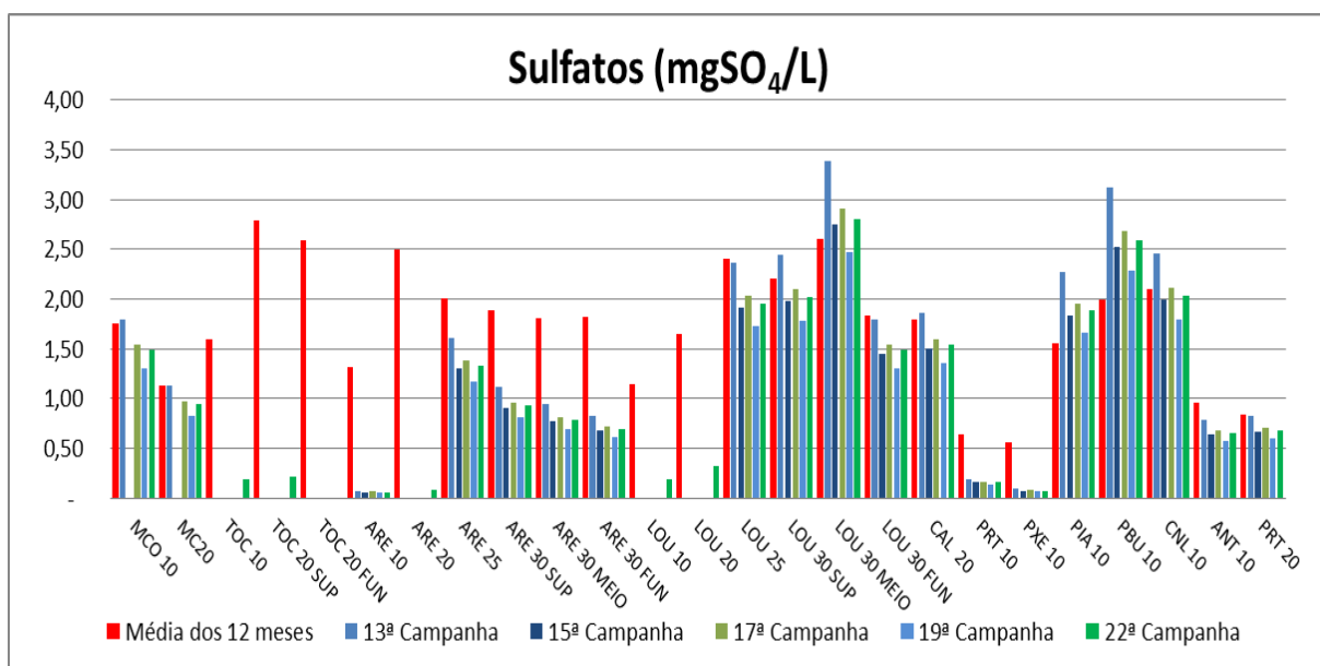
Figura VII-36 - Resultados de Sulfato - Tributários
