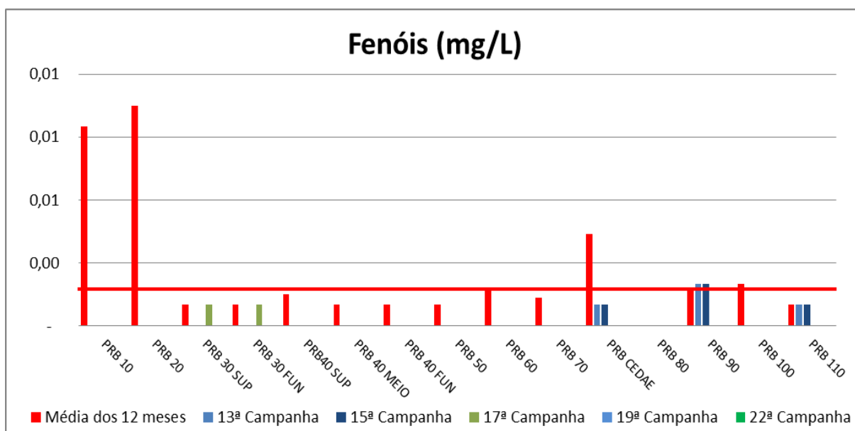
Figura VII-49 - Resultados de Fenóis – Rio Paraíba do Sul
