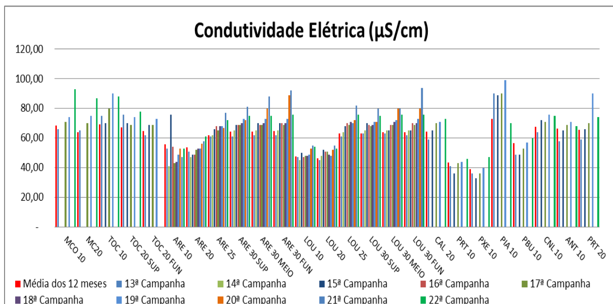
Figura VII-14 - Resultados de Condutividade Elétrica - Tributários
