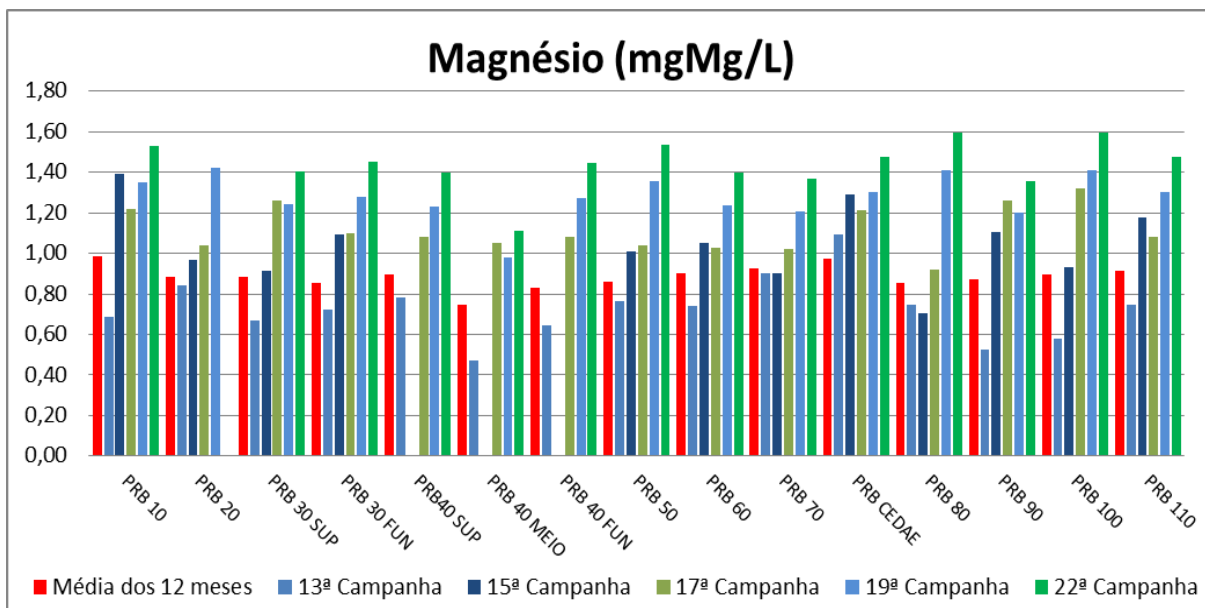
Figura VII-27 - Resultados de Magnésio – Rio Paraíba do Sul
