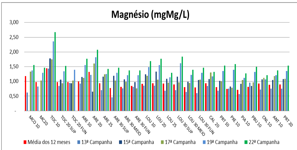
Figura VII-28 - Resultados de Magnésio - Tributários
