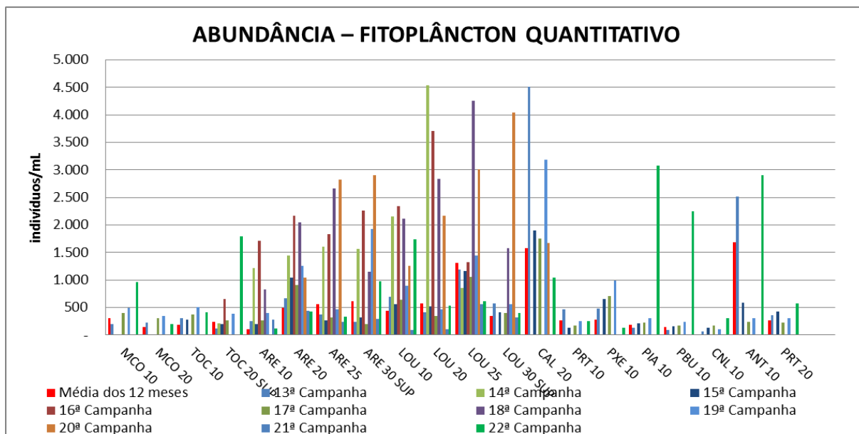
Figura VII-83 – Abundância de Fitoplâncton - Tributários.
