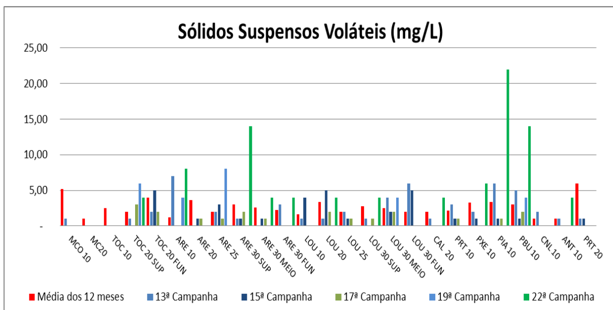
Figura VII-12 - Resultados de Sólidos Suspensos Voláteis - Tributários
