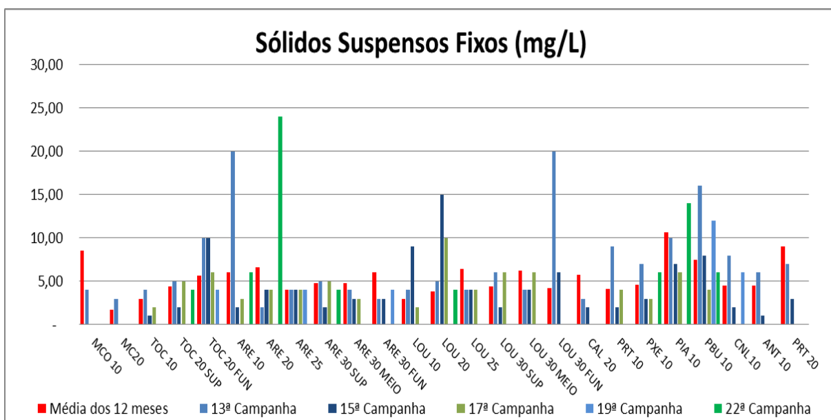
Figura VII-10 - Resultados de Sólidos Suspensos Fixos - Tributários
