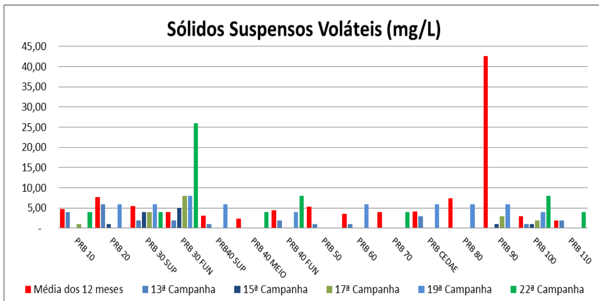
Figura VII-11 - Resultados de Sólidos Suspensos Voláteis – Rio Paraíba do Sul
