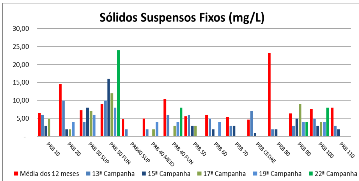
Figura VII-9 - Resultados de Sólidos Suspensos Fixos – Rio Paraíba do Sul
