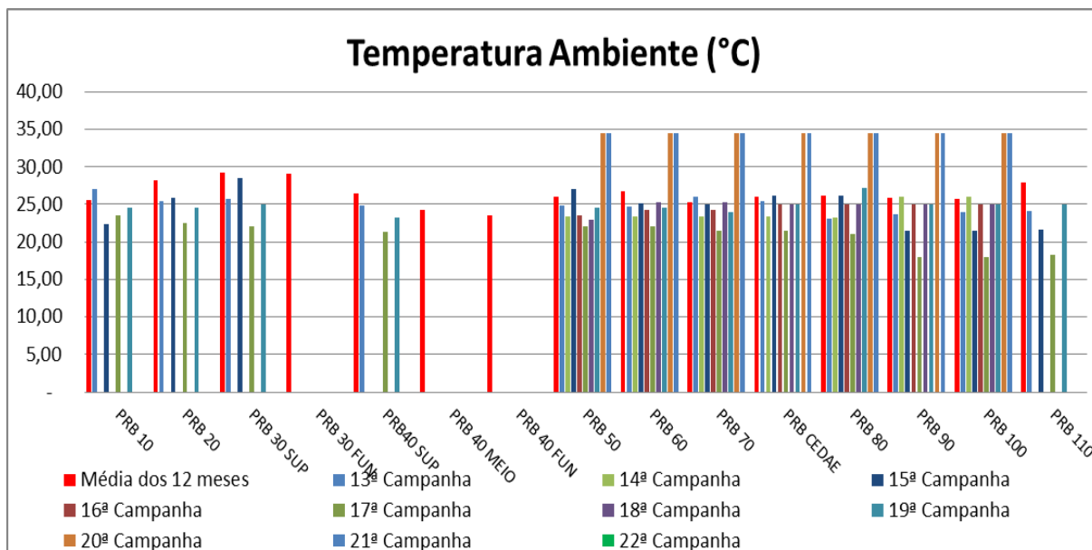
Figura VII-3 - Resultados da Temperatura Ambiente – Rio Paraíba do Sul
