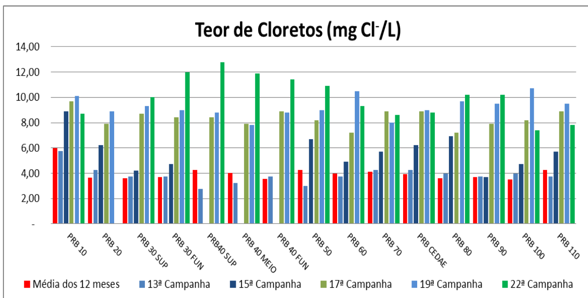
Figura VII-33 - Resultados de Teor de Cloretos – Rio Paraíba do Sul
