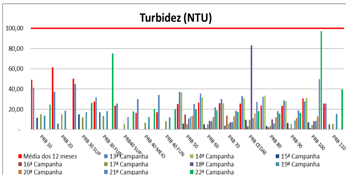
Figura VII-7 - Resultados de Turbidez – Rio Paraíba do Sul
