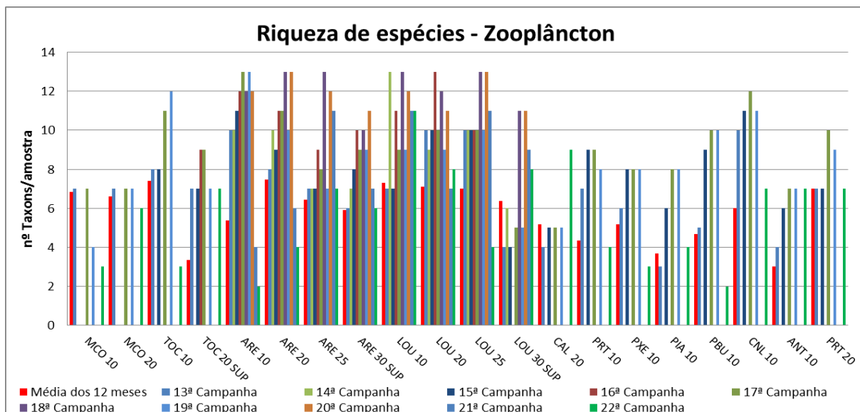
Figura VII-89 – Riqueza de espécies – Zooplâncton - Tributários
