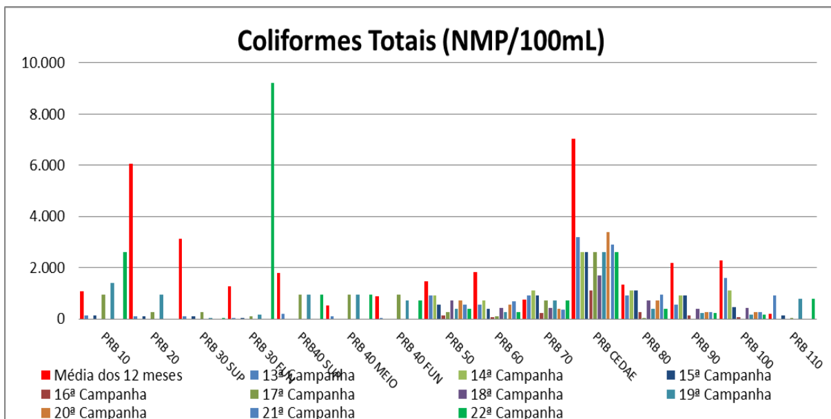
Figura VII-75 - Resultados de Coliformes Totais – Rio Paraíba do Sul
