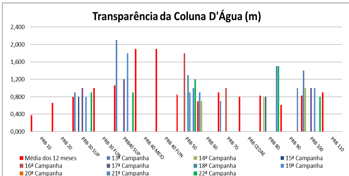
Figura VII-5 - Resultados de Transparência da coluna d'água – Rio Paraíba do Sul
