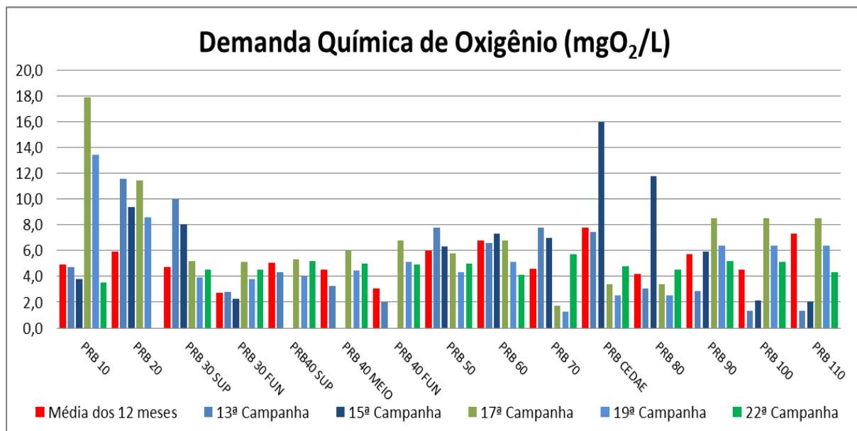
Figura VII-21 - Resultados da Demanda Química de Oxigênio – DQO – Rio Paraíba do Sul
