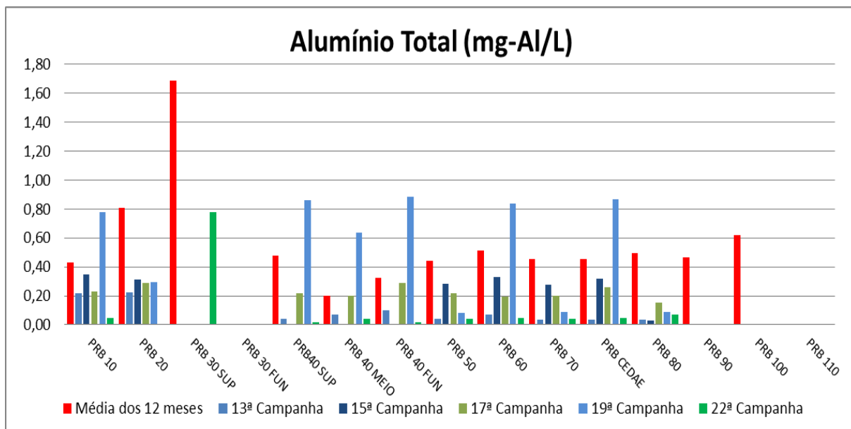
Figura VII-62 - Resultados de Alumínio Total – Rio Paraíba do Sul
