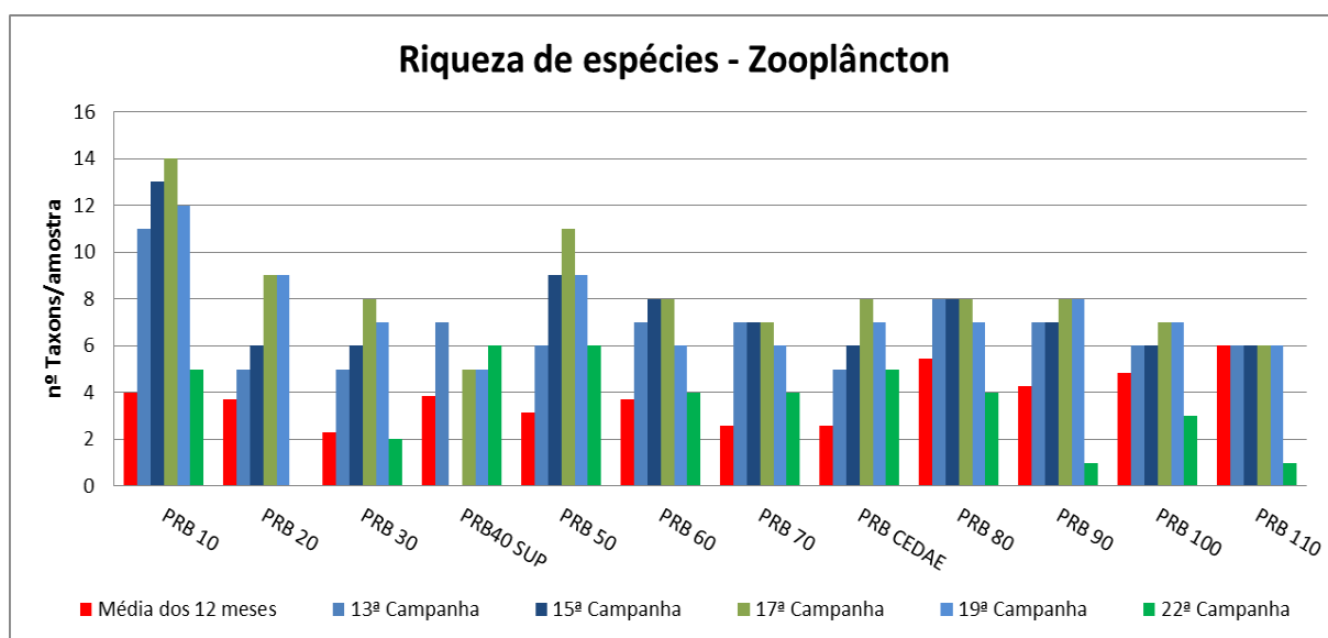
Figura VII-88 – Riqueza de espécies – Zooplâncton – Rio Paraíba do Sul
