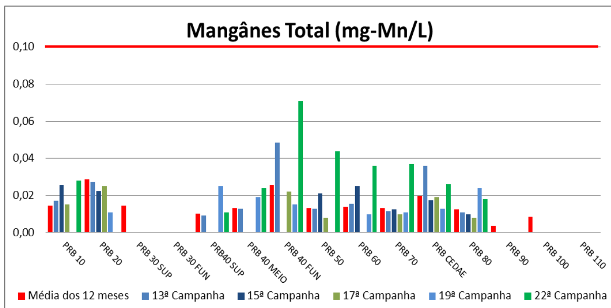
Figura VII-55 - Resultados de Manganês – Rio Paraíba do Sul
