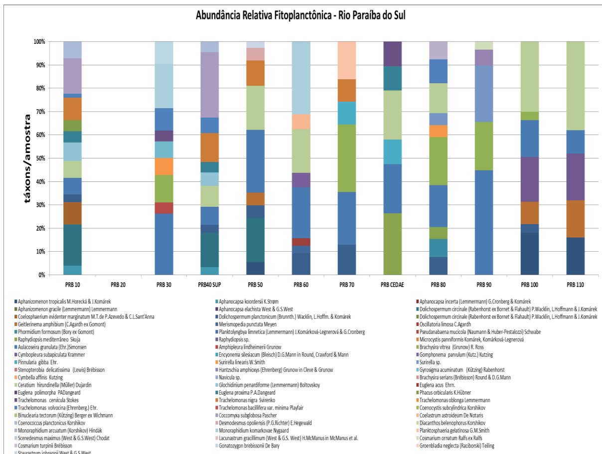
Figura VII-84 – Abundância Relativa Fitoplanctônica – Rio Paraíba do Sul.
