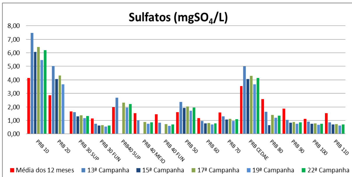
Figura VII-35 - Resultados de Sulfato – Rio Paraíba do Sul
