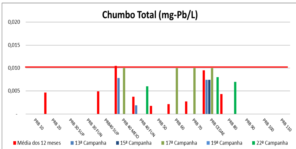
Figura VII-57 - Resultados de Chumbo – Rio Paraíba do Sul
