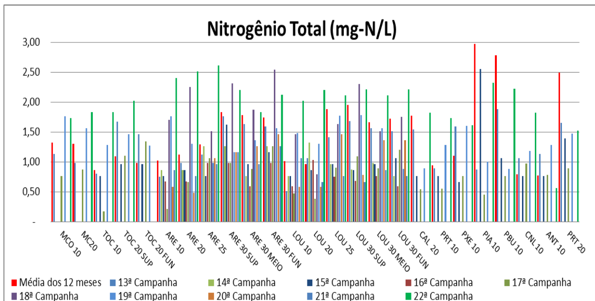
Figura VII-42 - Resultados de Nitrogênio Total - Tributários
