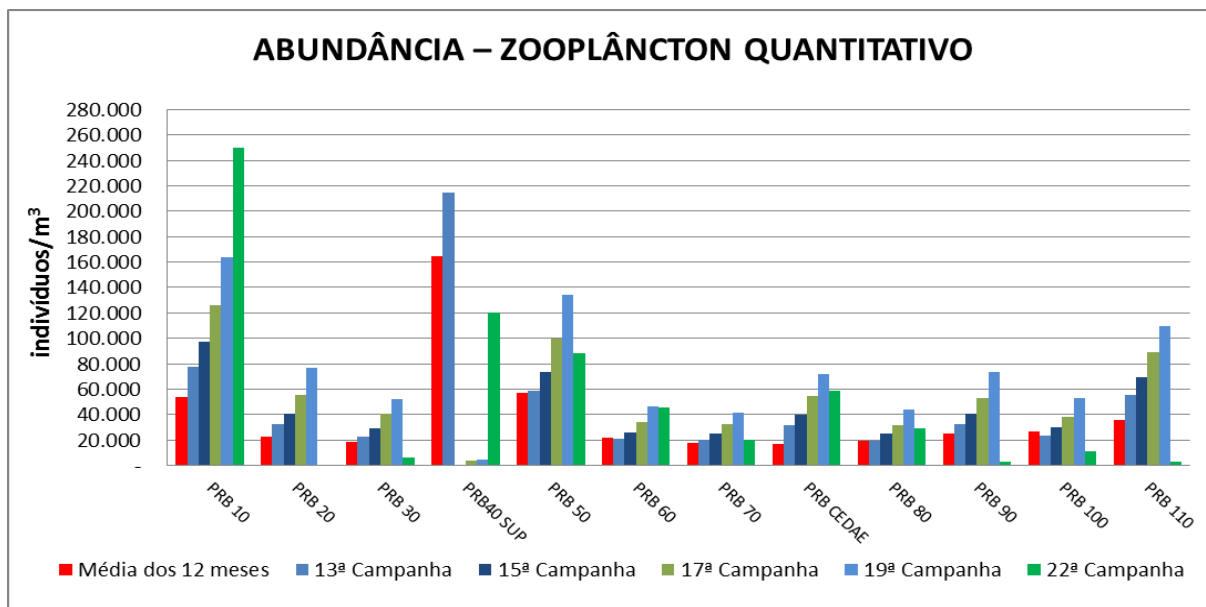
Figura VII-91 – Abundância de Zooplâncton - Rio Paraíba do Sul.
