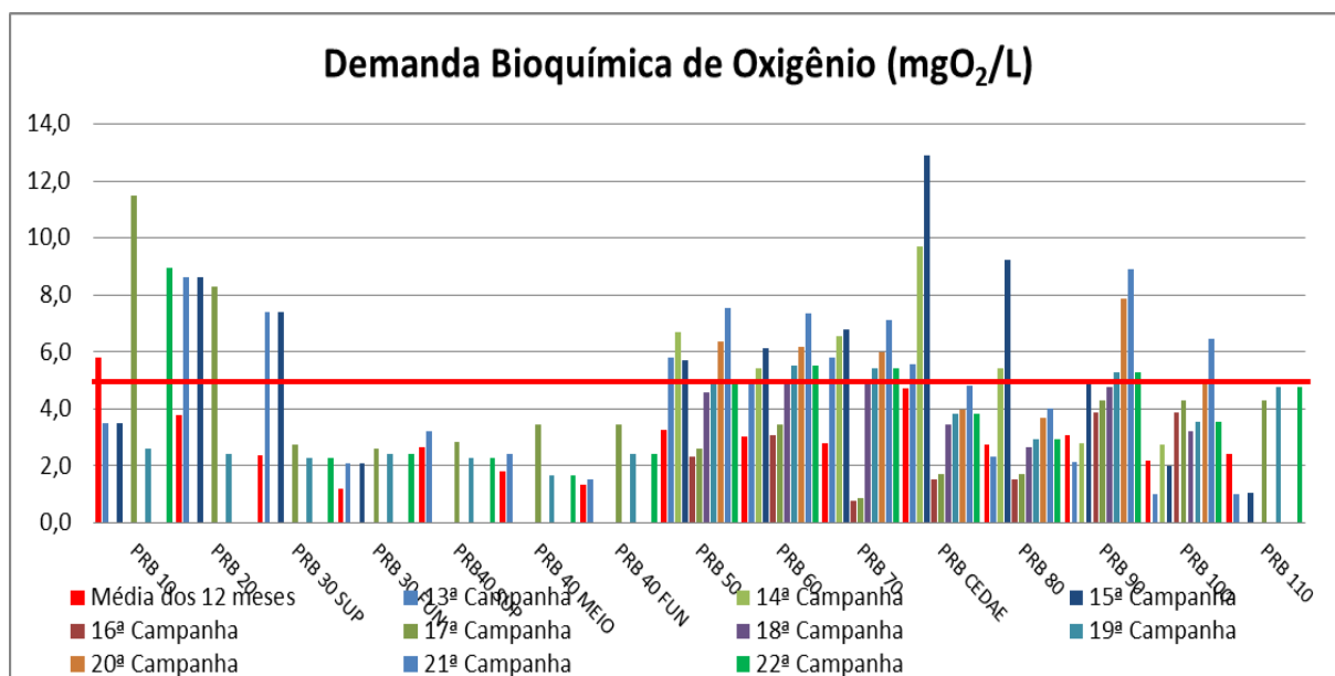
Figura VII-19 - Resultados da Demanda Bioquímica de Oxigênio – DBO – Rio Paraíba do Sul
