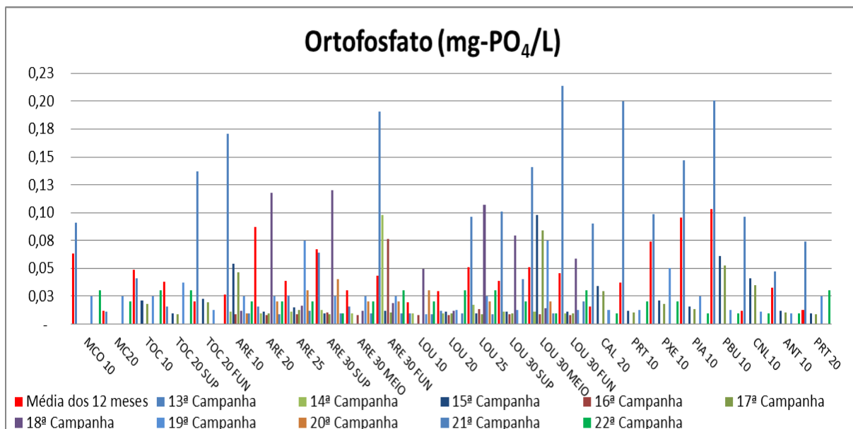
Figura VII-46 - Resultado de Ortofosfato - Tributários
