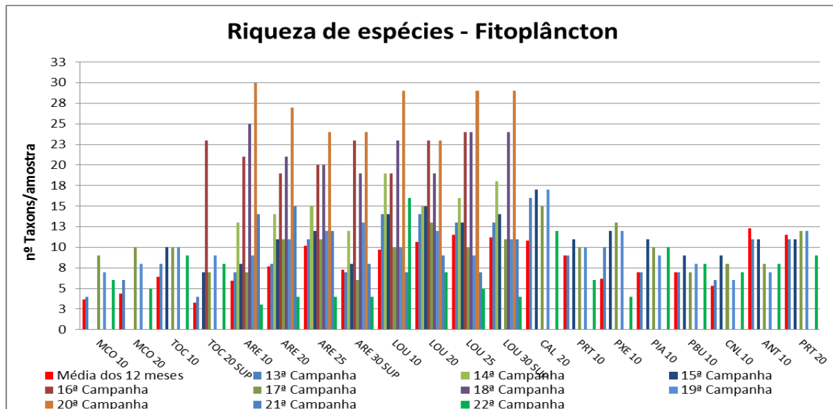
Figura VII-80 – Riqueza de espécies – Fitoplâncton - Tributários
