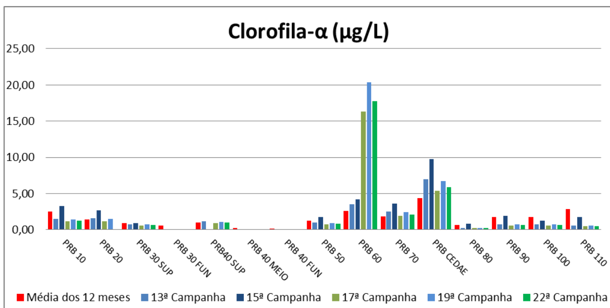
Figura VII-65 - Resultados de Clorofila-a – Rio Paraíba do Sul
