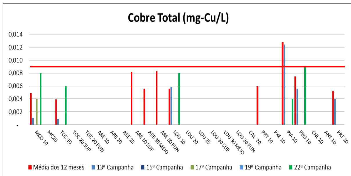
Figura VII-61 - Resultados de Cobre - Tributários
