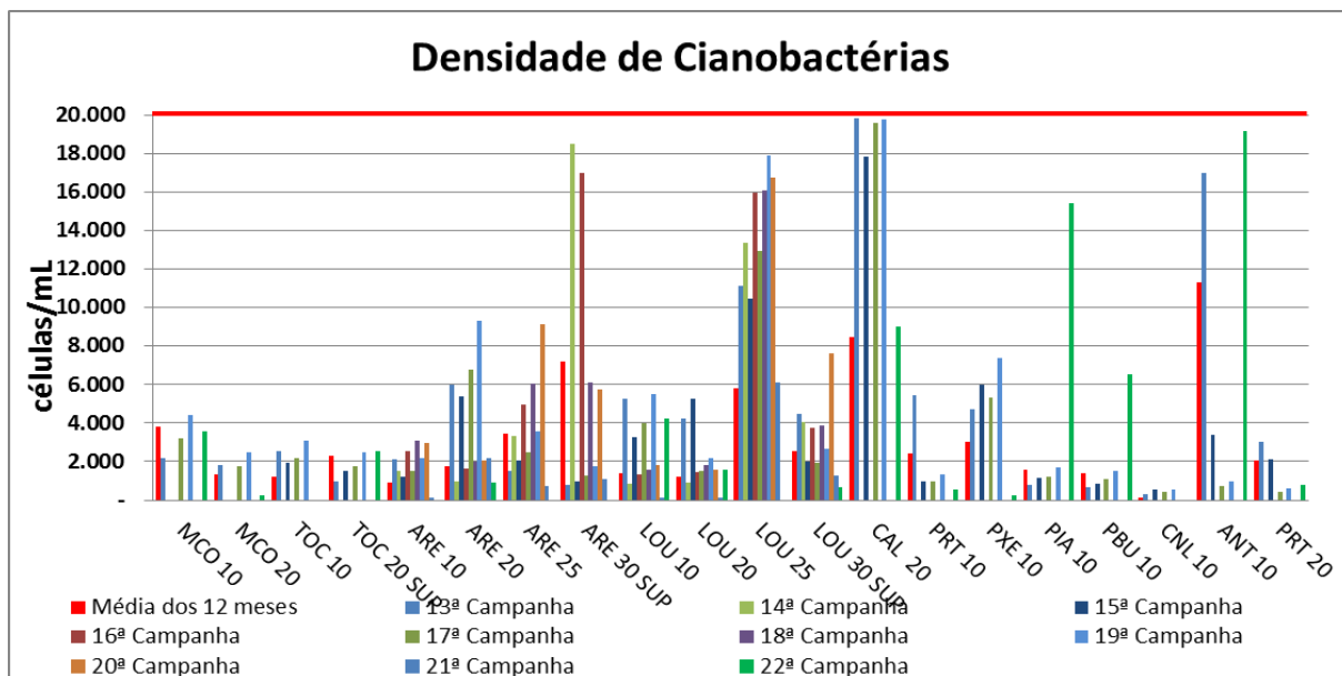
Figura VII-87 – Densidade de Cianobactérias - Tributários.
