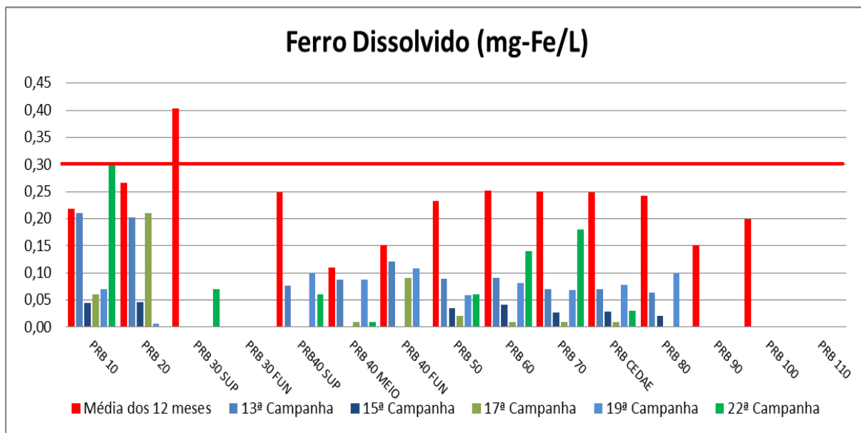
Figura VII-53 - Resultados de Ferro Dissolvido – Rio Paraíba do Sul
