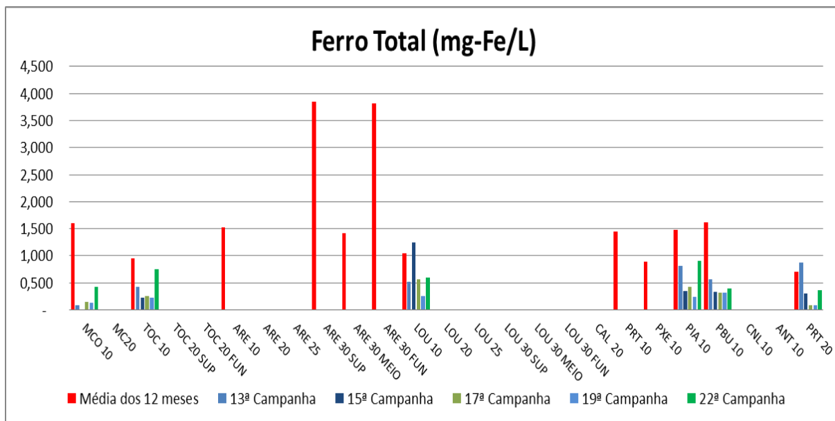
Figura VII-52 - Resultados de Ferro Total - Tributários
