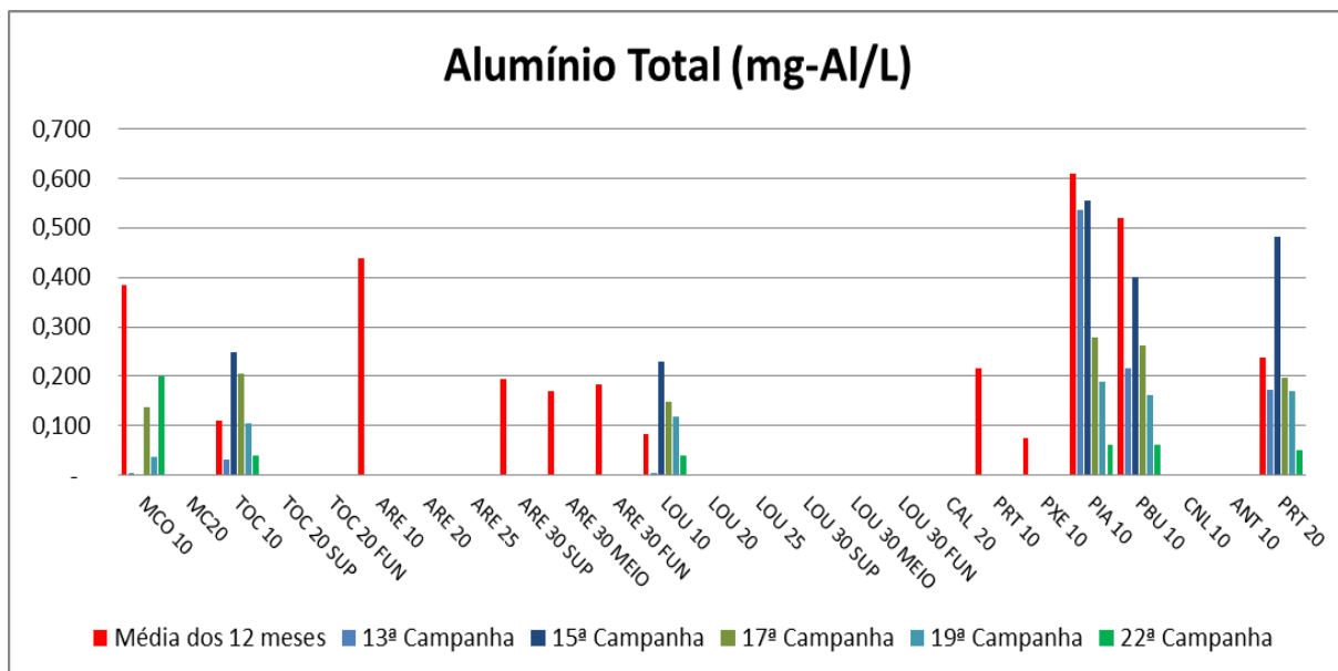
Figura VII-63 - Resultados de Alumínio Total - Tributários
