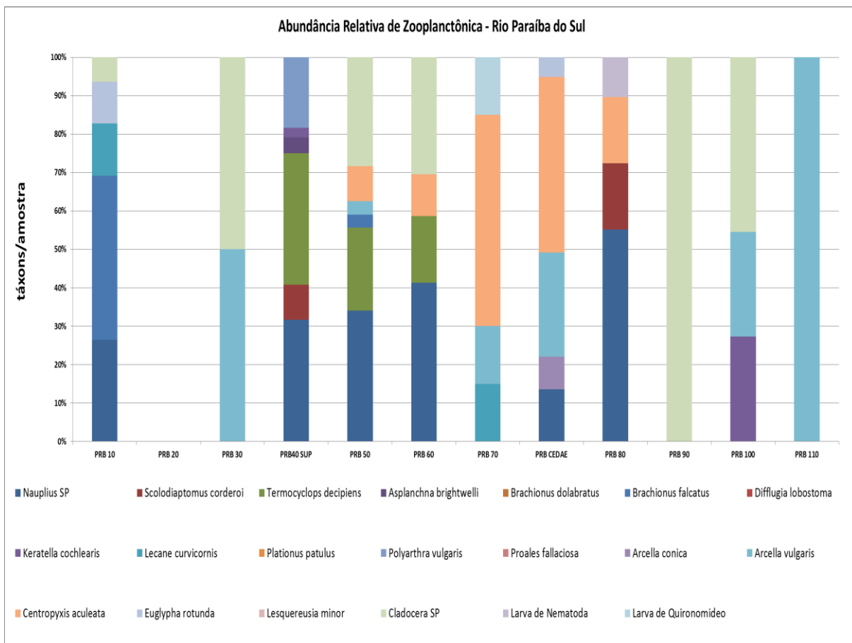
Figura VII-93 – Abundância Relativa de Zooplânctônica – Rio Paraíba do Sul.
