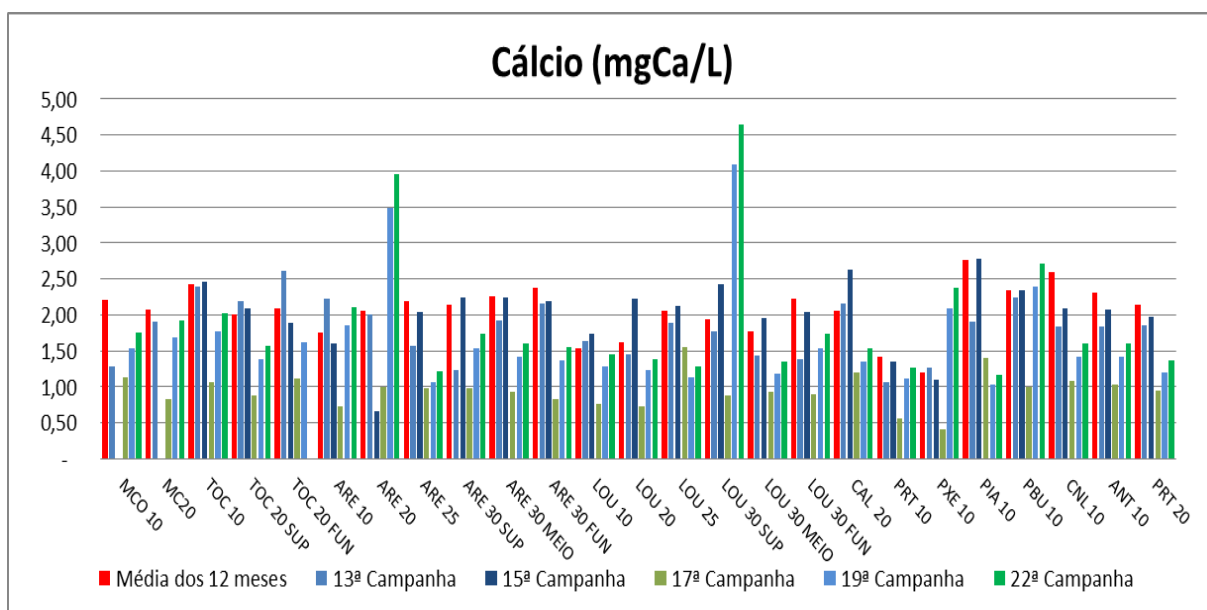
Figura VII-26 - Resultados de Cálcio - Tributários
