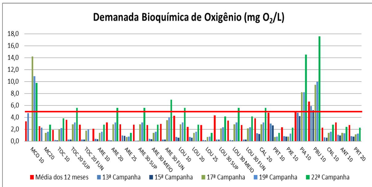
Figura VII-20 - Resultados da Demanda Bioquímica de Oxigênio – DBO - Tributários
