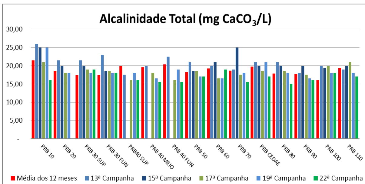
Figura VII-23 - Resultados da Alcalinidade Total – Rio Paraíba do Sul
