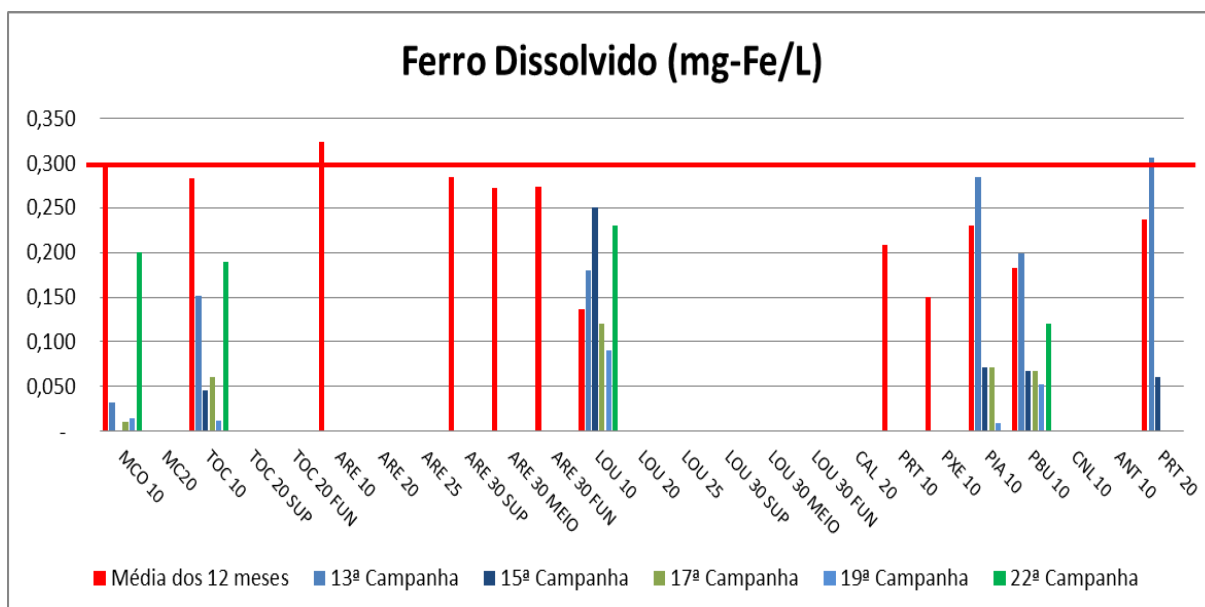
Figura VII-54 - Resultados de Ferro Dissolvido - Tributários
