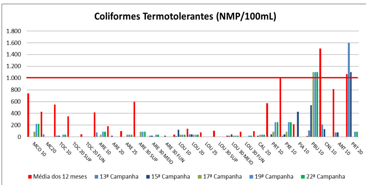
Figura VII-78 - Resultados de Coliformes Termotolerantes - Tributários
