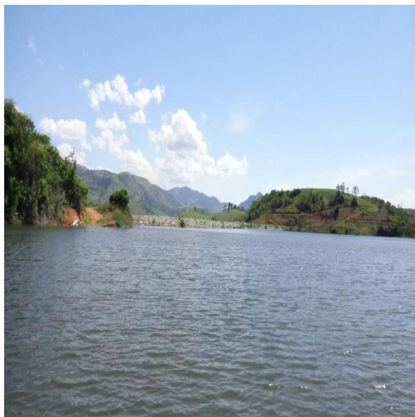
Figura IV-24 – Estação CAL 20, reservatório de Calçado.
