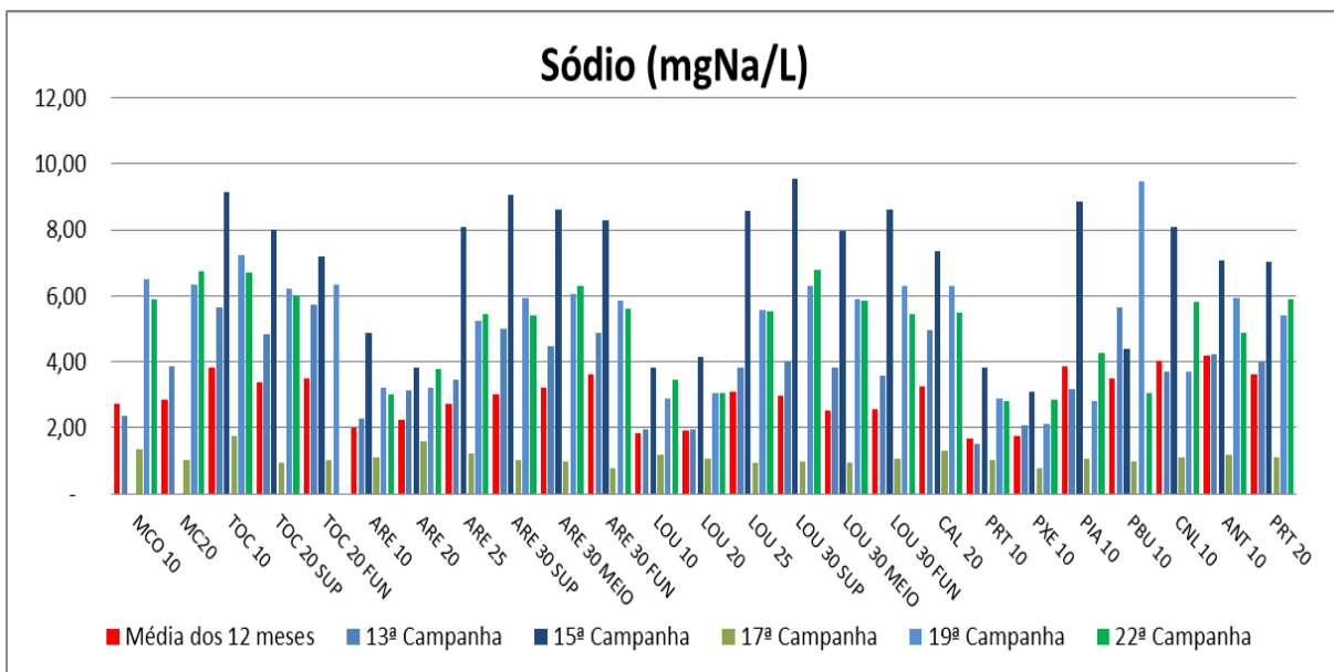
Figura VII-30 - Resultados de Sódio - Tributários
