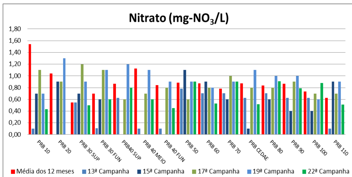
Figura VII-37 - Resultados de Nitrato – Rio Paraíba do Sul
