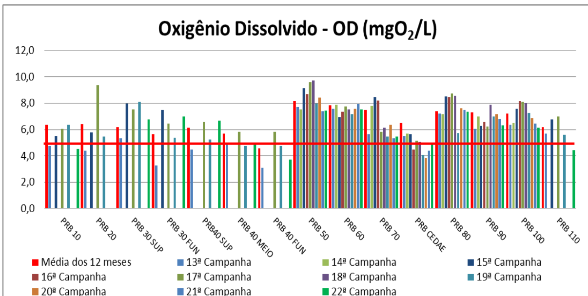
Figura VII-17 - Resultados de OD – Rio Paraíba do Sul
