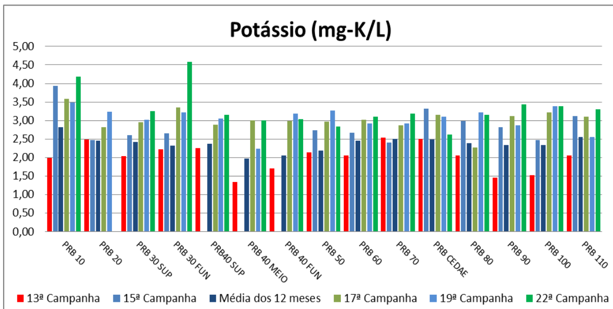
Figura VII-31 - Resultados de Potássio – Rio Paraíba do Sul
