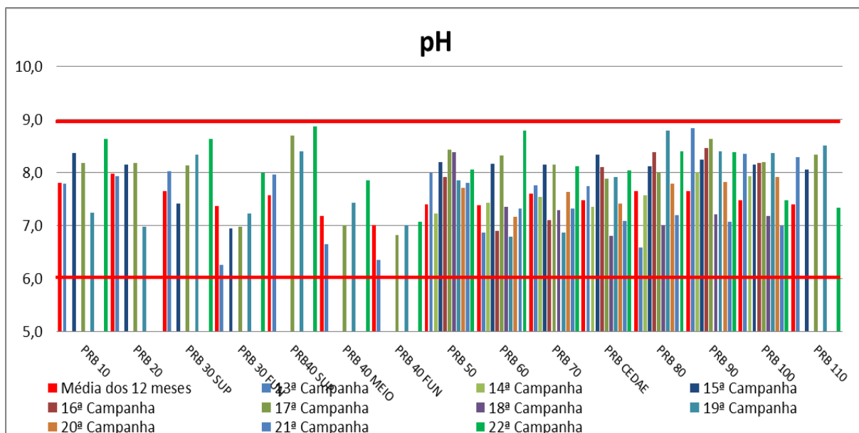
Figura VII-15 - Resultados de pH – Rio Paraíba do Sul
