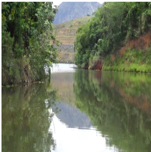
Figura IV-15 – Estação TOC 20 reservatório Tocaia.
