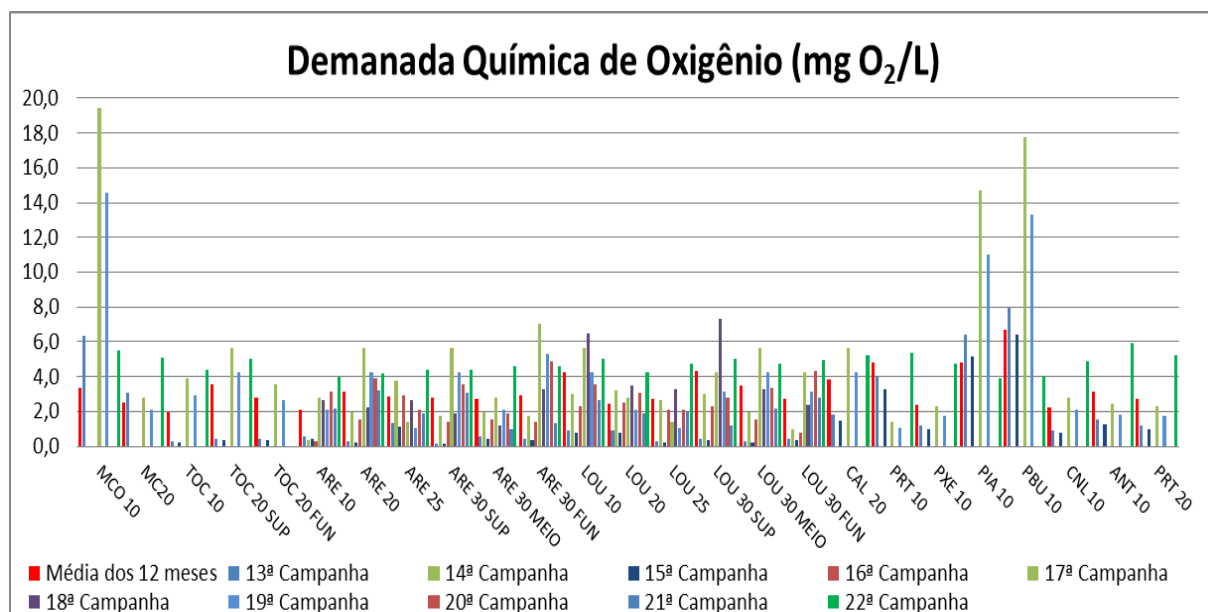
Figura VII-22 - Resultados da Demanda Química de Oxigênio – DQO - Tributários
