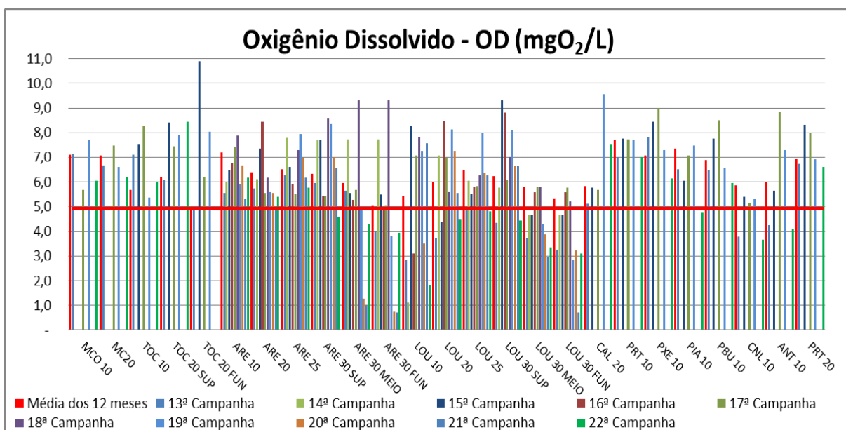
Figura VII-18 - Resultados de OD - Tributários
