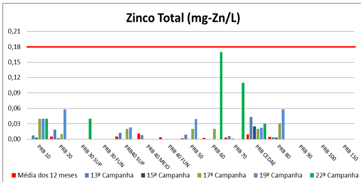
Figura VII-58 - Resultados de Zinco – Rio Paraíba do Sul
