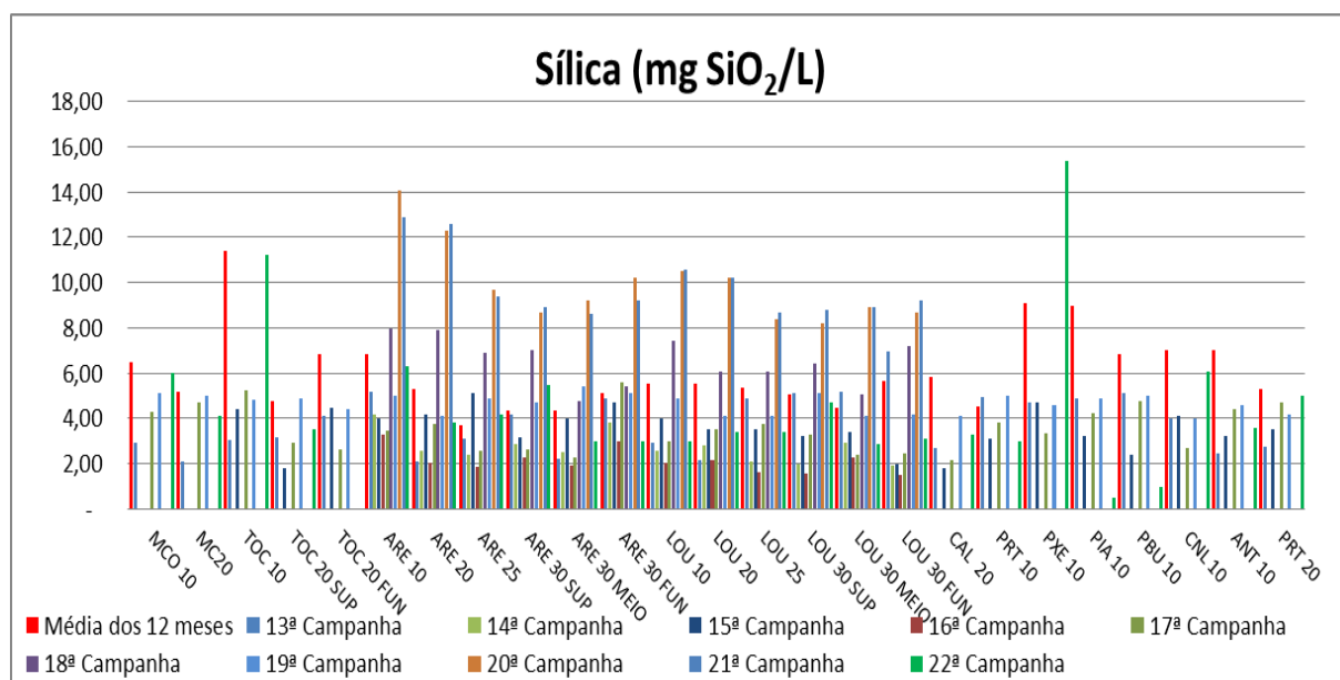
Figura VII-48 - Resultados de Sílica - Tributários
