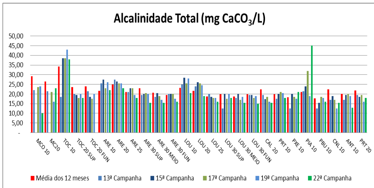
Figura VII-24 - Resultados da Alcalinidade Total - Tributários
