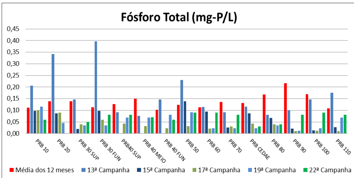
Figura VII-43 - Resultado de Fósforo Total – Rio Paraíba do Sul
