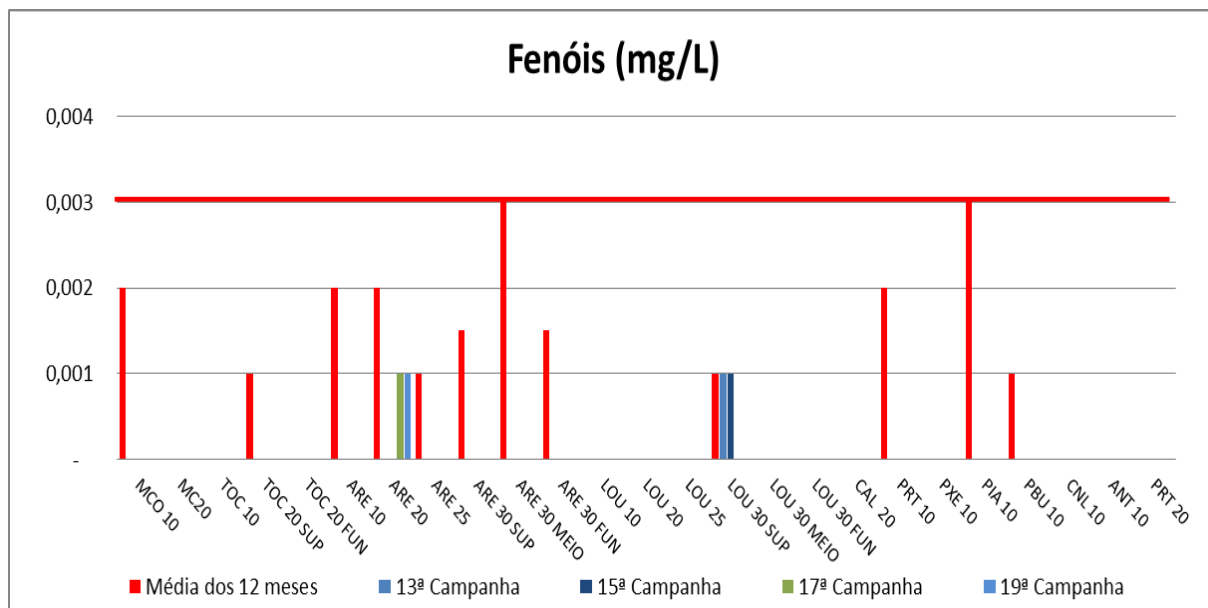
Figura VII-50 - Resultados de Fenóis - Tributários
