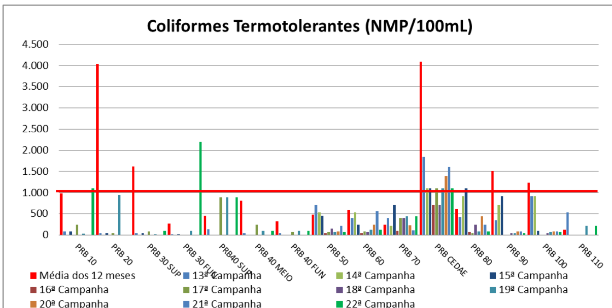
Figura VII-77 - Resultados de Coliformes Termotolerantes – Rio Paraíba do Sul
