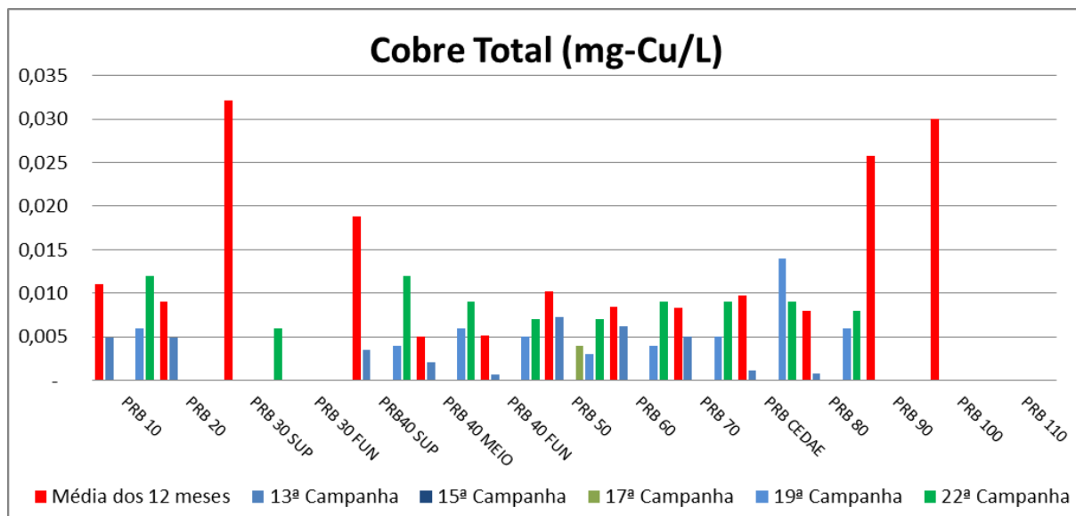
Figura VII-60 - Resultados de Cobre – Rio Paraíba do Sul
