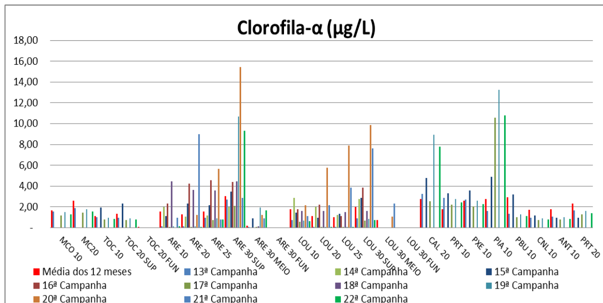
Figura VII-66 - Resultados de Clorofila-a - Tributários
