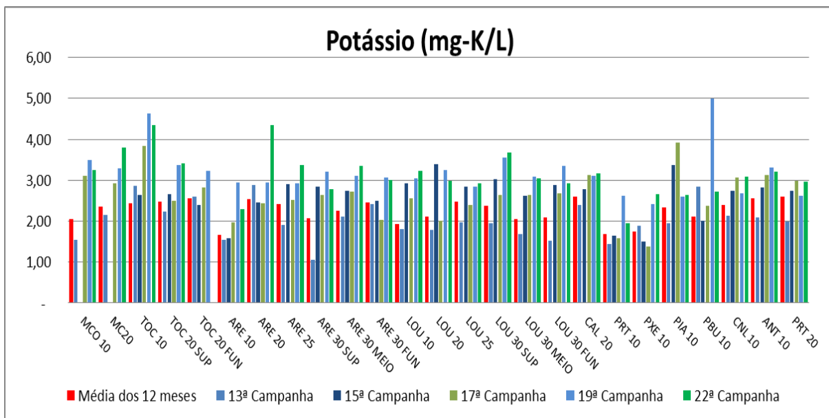
Figura VII-32 - Resultados de Potássio - Tributários
