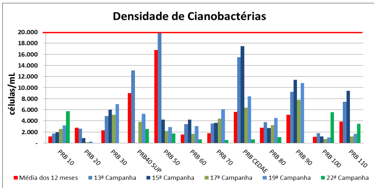
Figura VII-86 – Densidade de Cianobactérias – Rio Paraíba do Sul.
