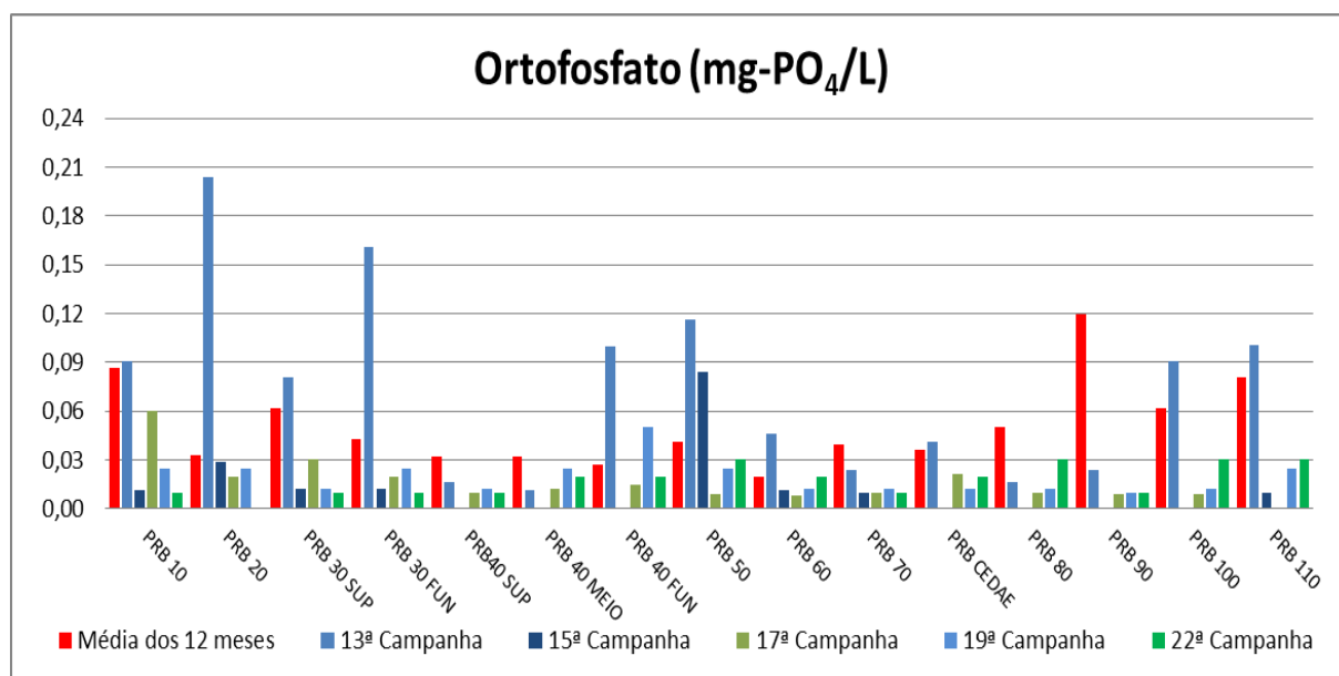
Figura VII-45 - Resultado de Ortofosfato – Rio Paraíba do Sul
