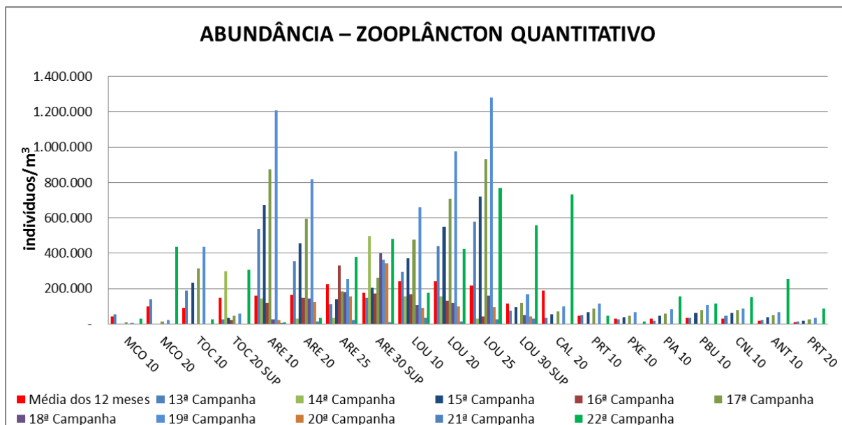
Figura VII-92 – Abundância de Zooplâncton - Tributários.
