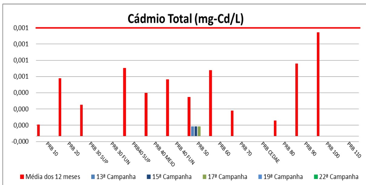
Figura VII-64 - Resultados de Cádmio Total – Rio Paraíba do Sul
