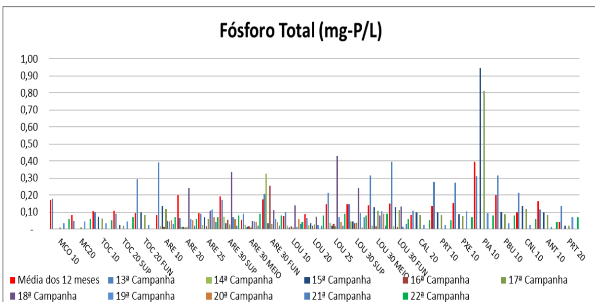
Figura VII-44 - Resultado de Fósforo Total - Tributários
