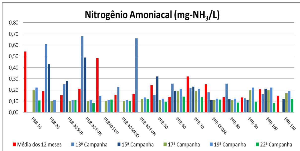
Figura VII-39 - Resultados de Nitrogênio Amoniacal – Rio Paraíba do Sul
