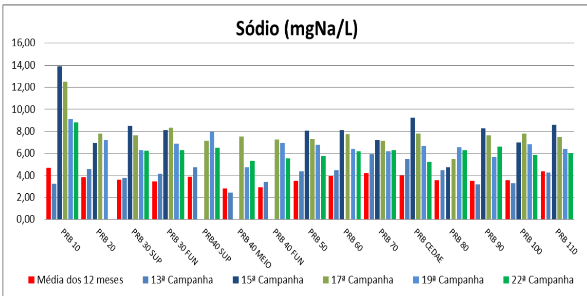
Figura VII-29 - Resultados de Sódio – Rio Paraíba do Sul
