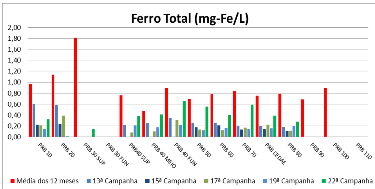
Figura VII-51 - Resultados de Ferro Total – Rio Paraíba do Sul
