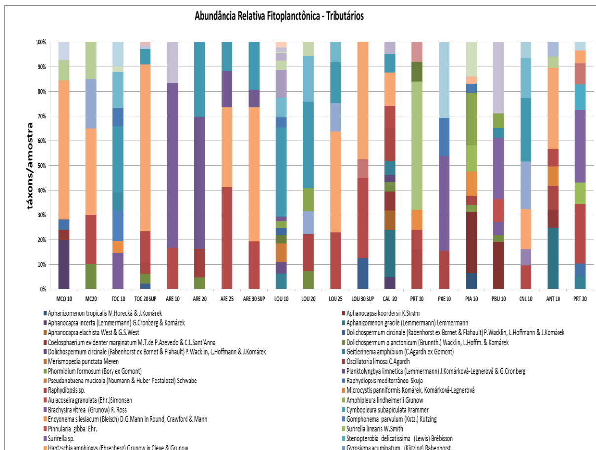
Figura VII-85 – Abundância Relativa Fitoplanctônica - Tributários.
