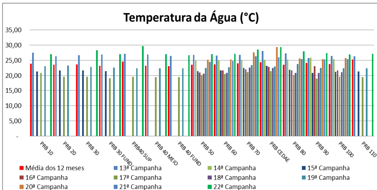
Figura VII-1 - Resultados da Temperatura da Água – Paraíba do Sul
