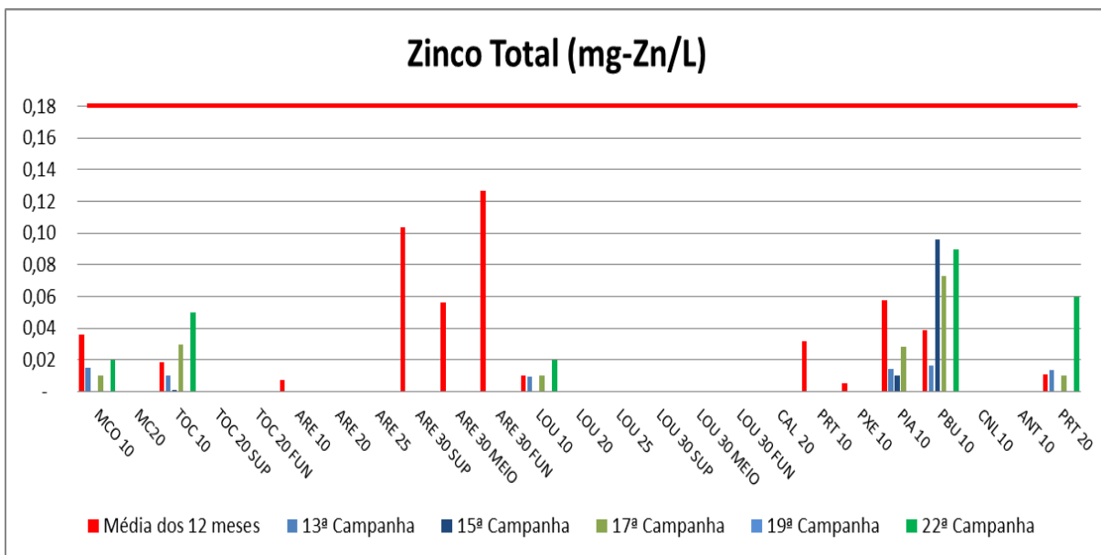
Figura VII-59 - Resultados de Zinco - Tributários
