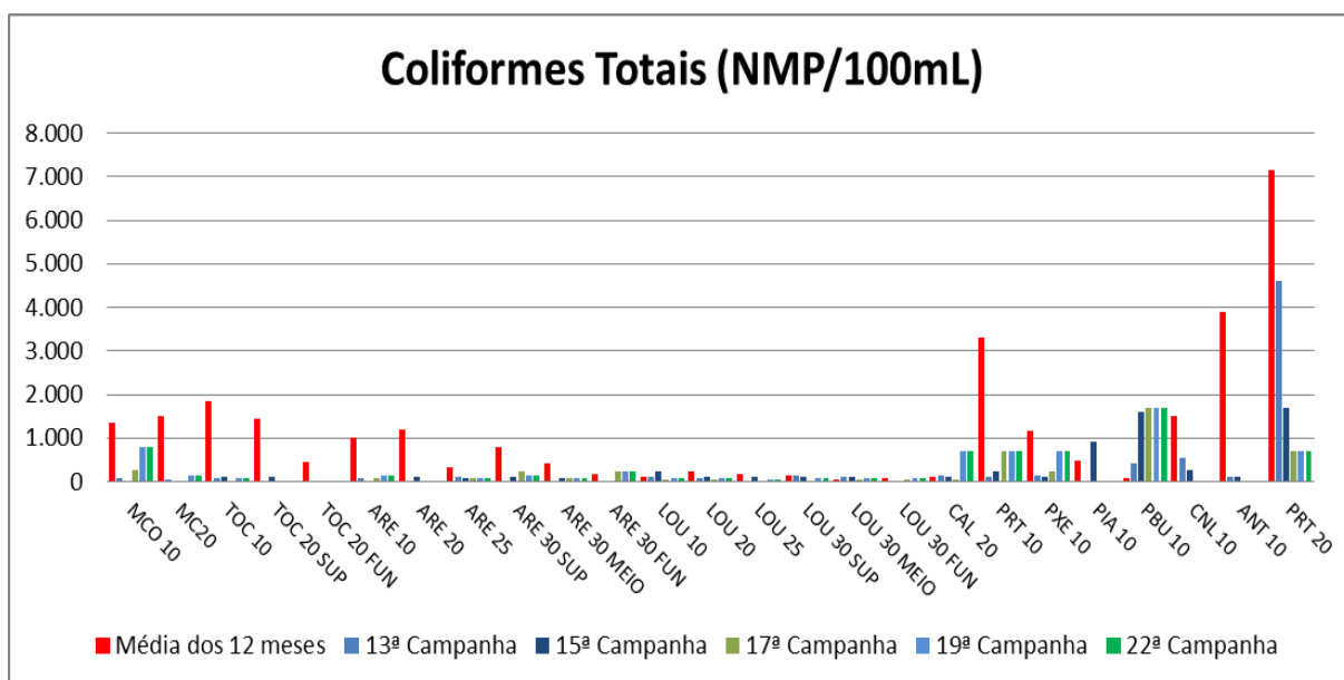
Figura VII-76 - Resultados de Coliformes Totais - Tributários
