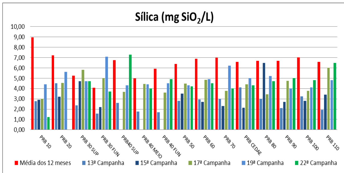
Figura VII-47 - Resultados de Sílica – Rio Paraíba do Sul
