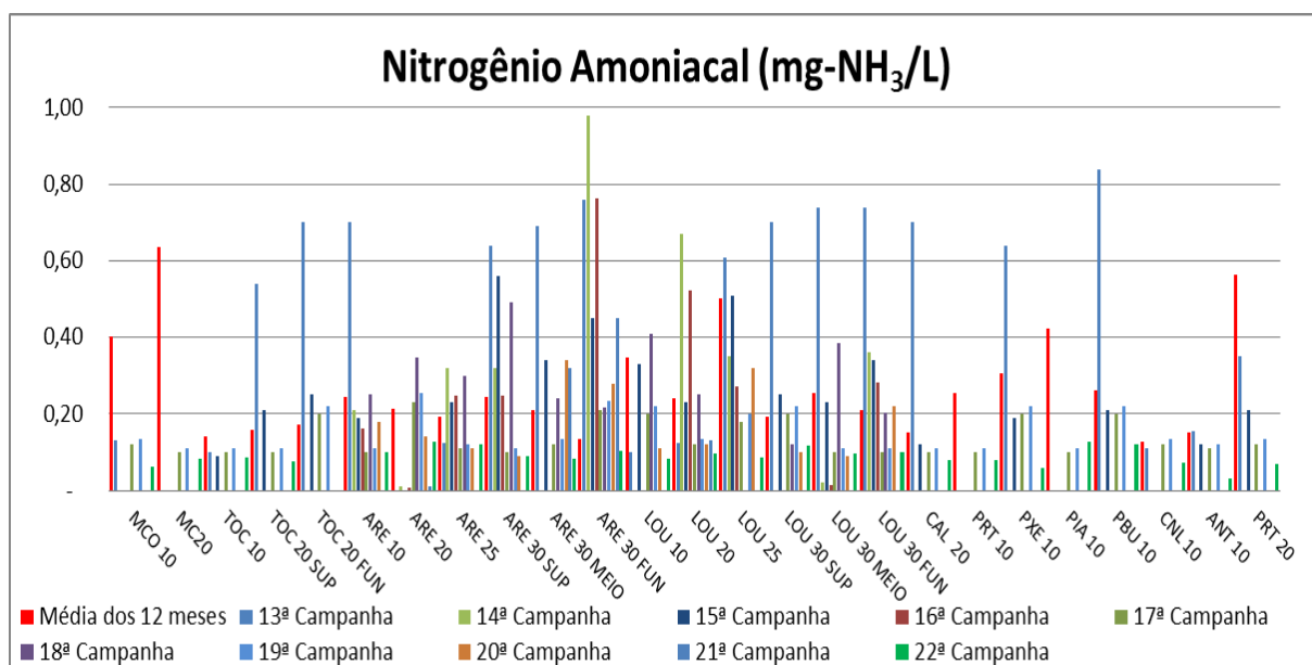
Figura VII-40 - Resultados de Nitrogênio Amoniacal - Tributários
