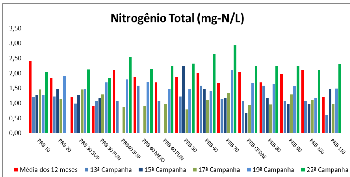
Figura VII-41 - Resultados de Nitrogênio Total – Rio Paraíba do Sul
