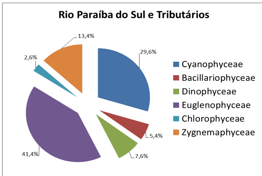
Figura VII-31 – Porcentagem de contribuição, em número de táxons de Fitoplâncton nos Tributários (Circuito do Lourical).
