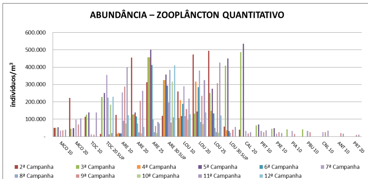
Figura VII-37 – Abundância de Zooplâncton - Tributários.
