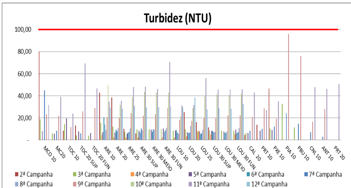
Figura VII-8 - Resultados de Turbidez - Tributários
