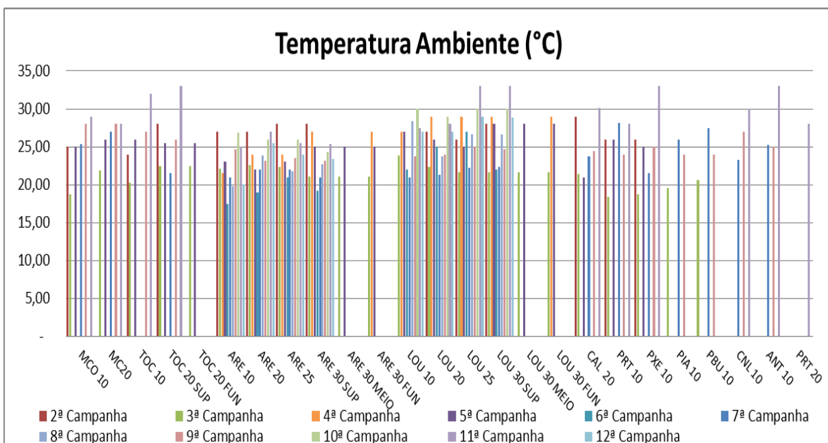
Figura VII-4 - Resultados da Temperatura Ambiente - Tributários
