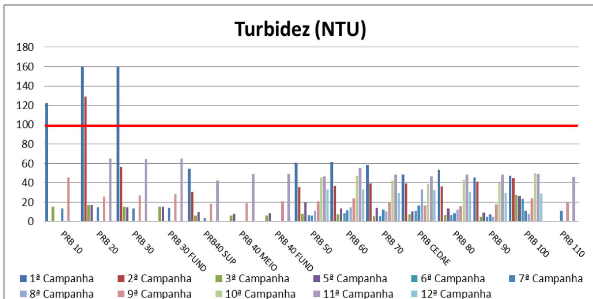
Figura VII-7 - Resultados de Turbidez - Resolução ANA nº 354, de 11 de Março de 2013.
