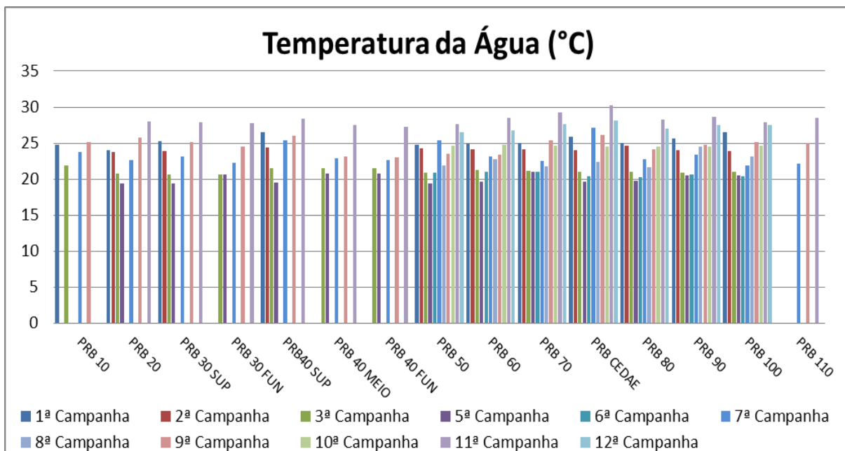
Figura VII-1 - Resultados da Temperatura da Água - Resolução ANA nº 713, de 11 de Junho de 2013.
