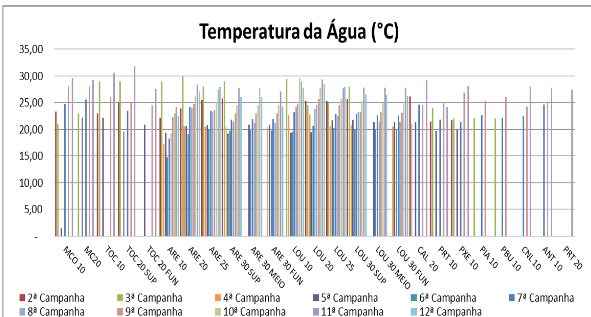
Figura VII-2 - Resultados da Temperatura da Água - Tributários
