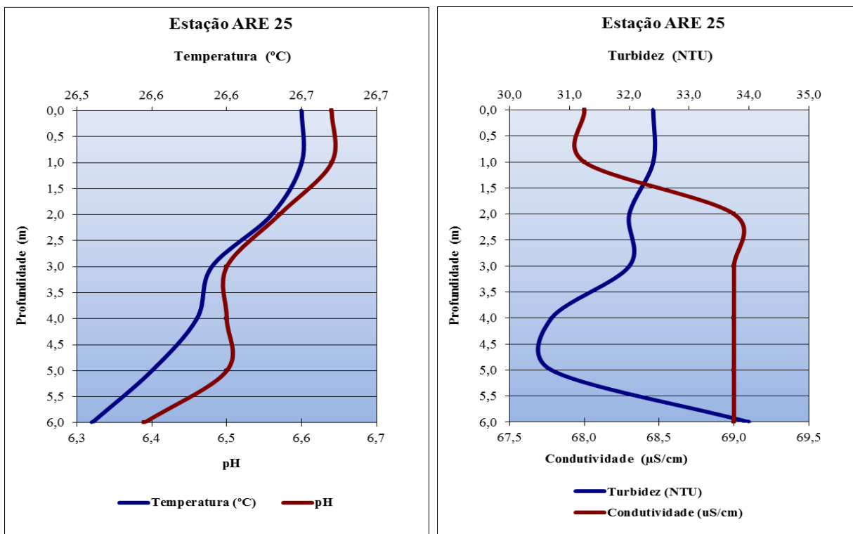
Figura VII-24 - Perfis ponto ARE 25
