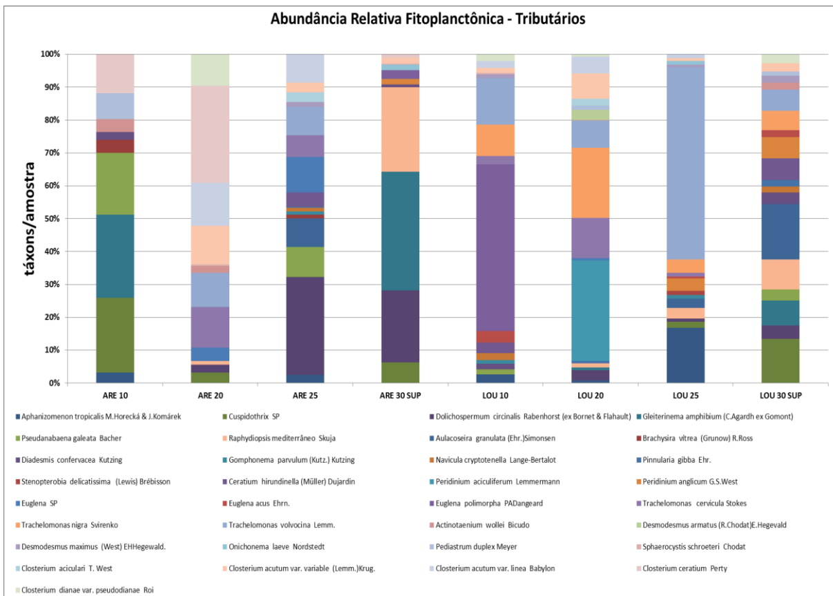
Figura VII-33 – Abundância Relativa Fitoplancônica - Tributários.
