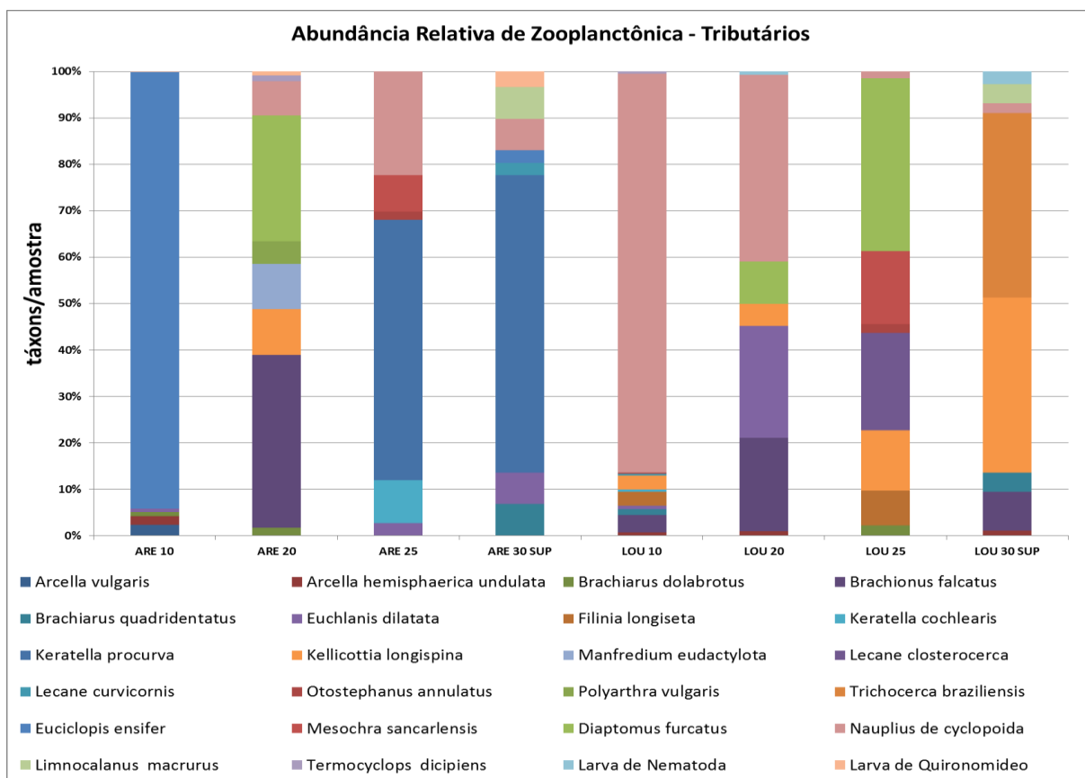
Figura VII-38 – Abundância Relativa de Zooplânctônica - Tributários.
