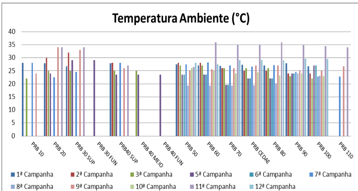
Figura VII-3 - Resultados da Temperatura da Ambiente - Resolução ANA nº 713, de 11 de Junho de 2013.
