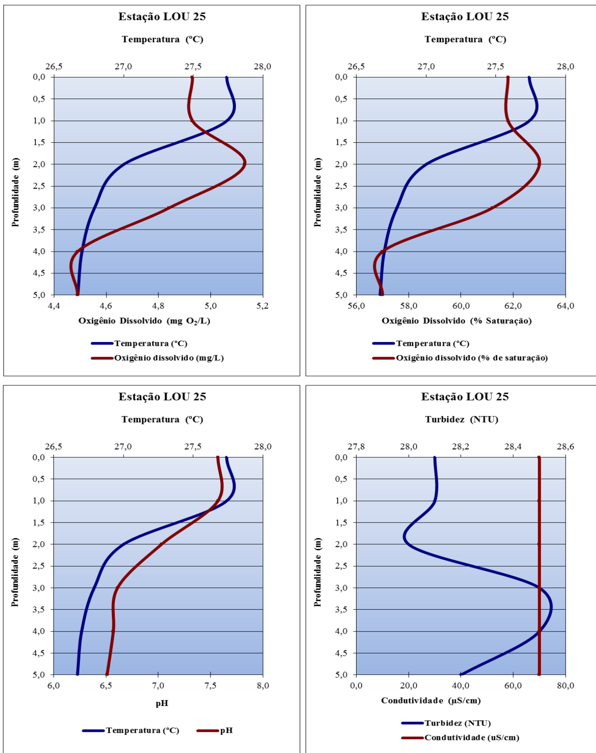
Figura VII-27 - Perfis ponto LOU 25
