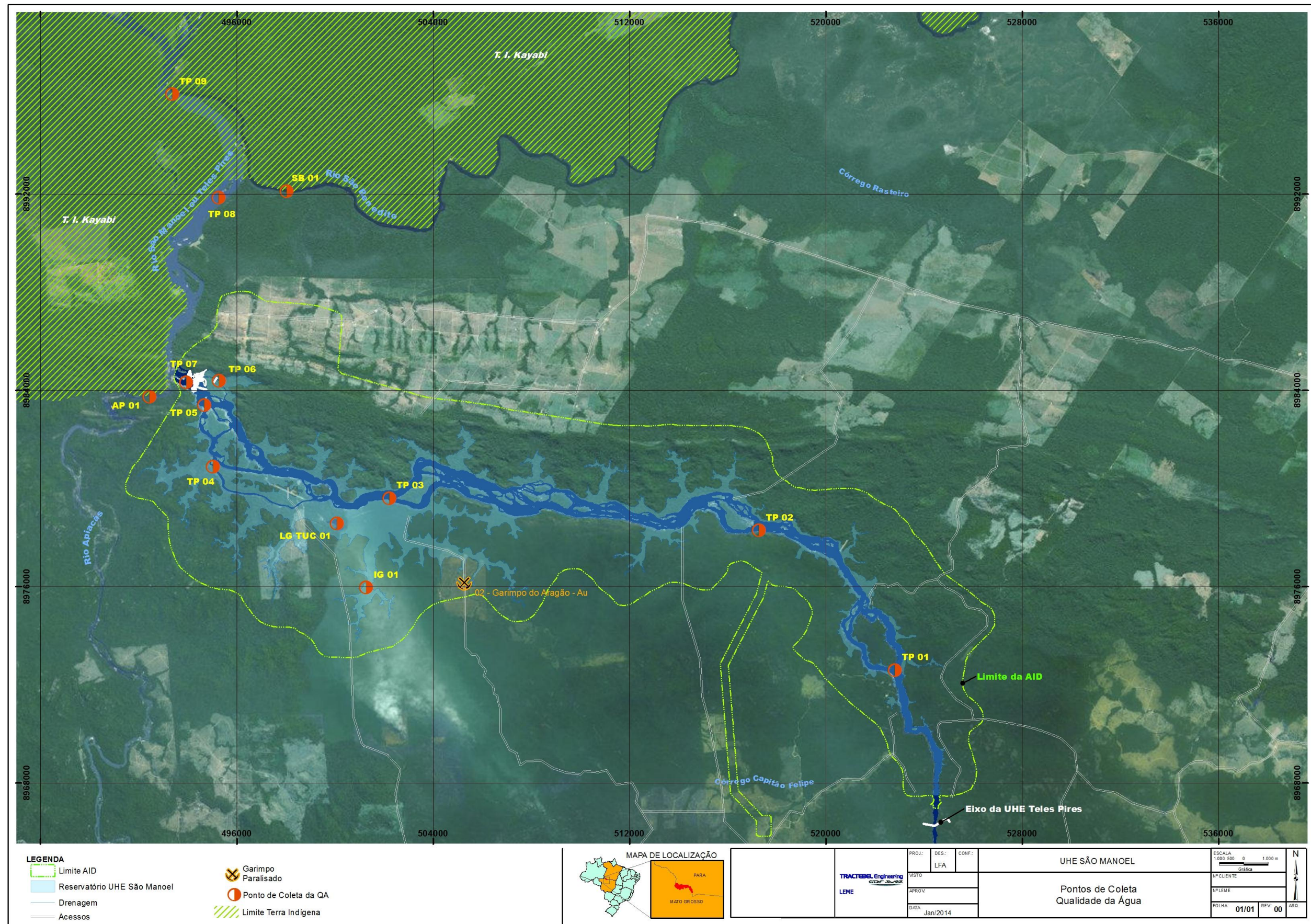
Figura 11 - 1 – Malha amostral do Programa de Monitoramento Limnológico e da Qualidade de Água da UHE São Manoel.
