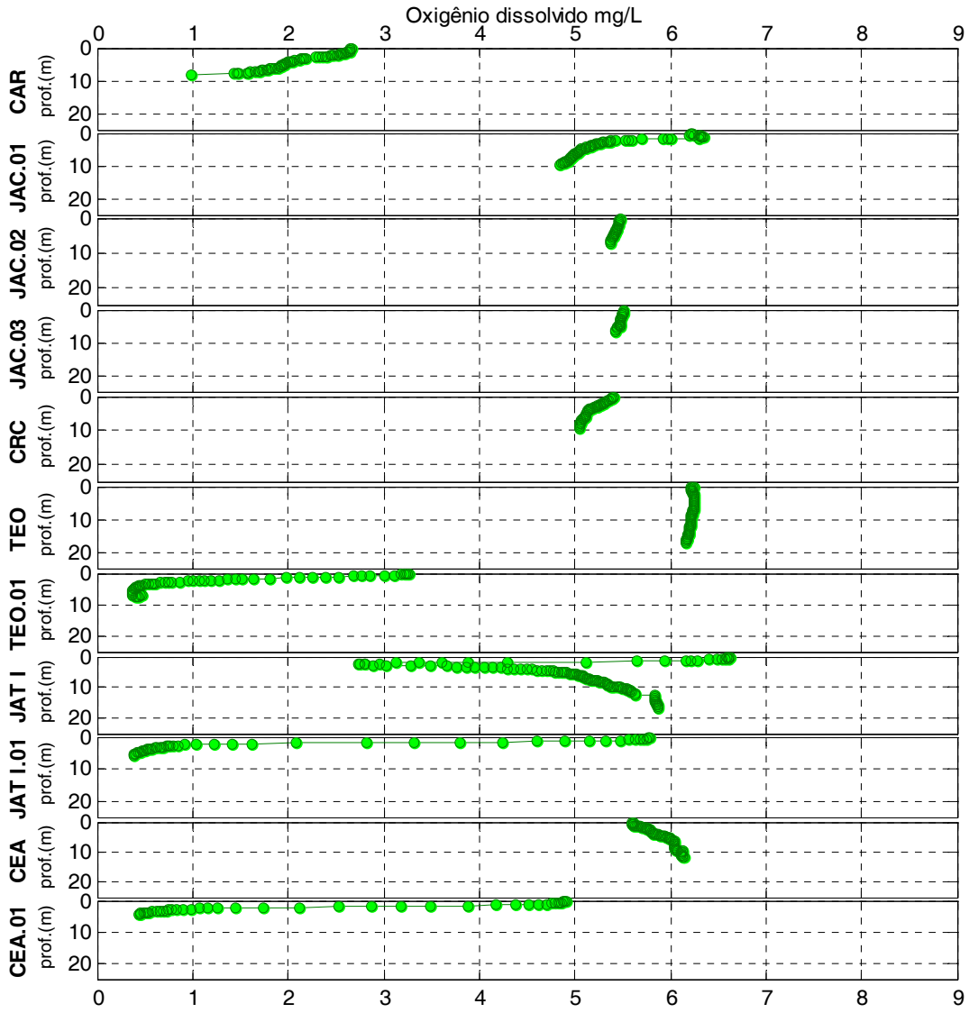
Figura 2-19 - Perfis de oxigênio dissolvido nos tributários em maio de 2012 (águas altas).
