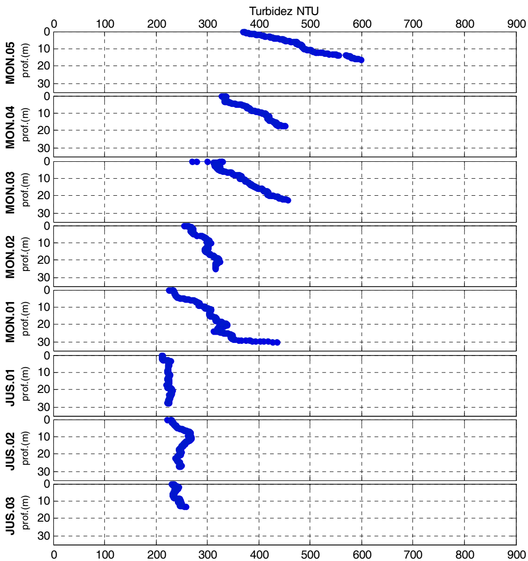
Figura 2-9 - Perfis de turbidez no rio Madeira em maio de 2012 (águas altas).
