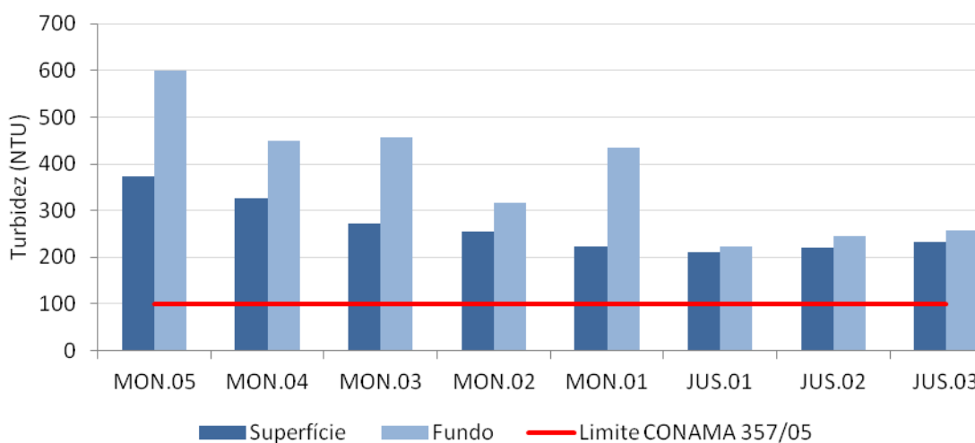
Figura 2-8 - Valores de turbidez no rio Madeira em maio de 2012 (águas altas).
