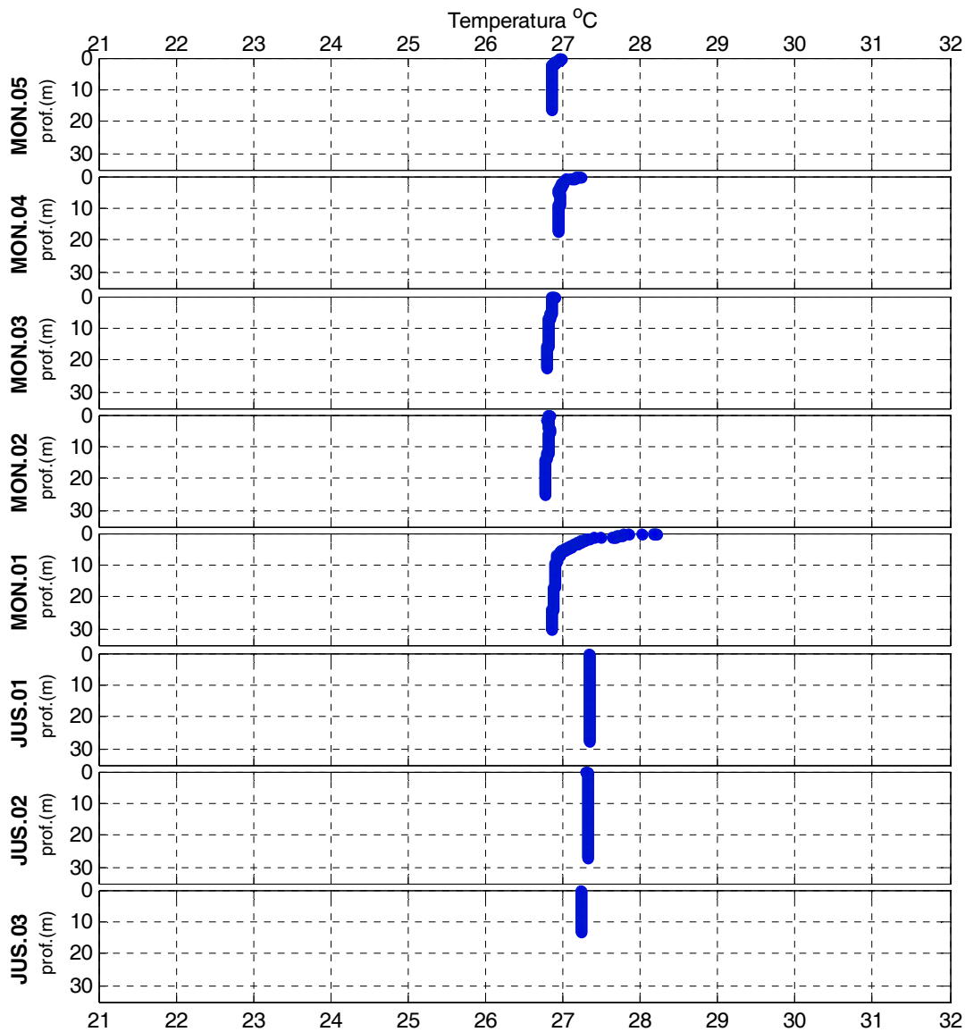
Figura 2-5 - Perfis de temperatura no rio Madeira em maio de 2012 (águas altas).
