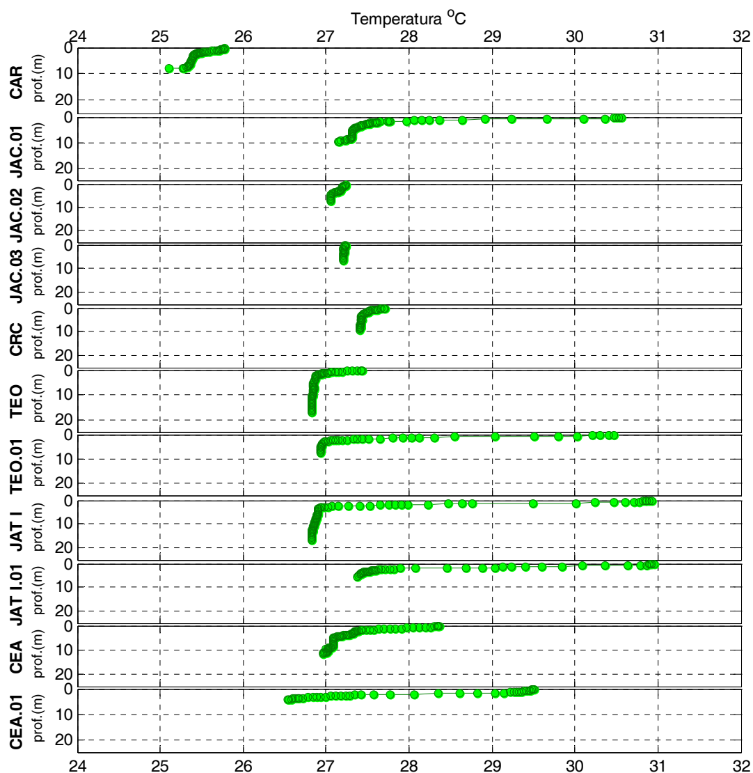
Figura 2-7 - Perfis de temperatura nos tributários em maio de 2012 (águas altas).
