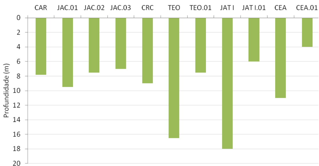
Figura 2-2 - Profundidade da coluna d'água nos tributários em maio de 2012 (águas altas).
