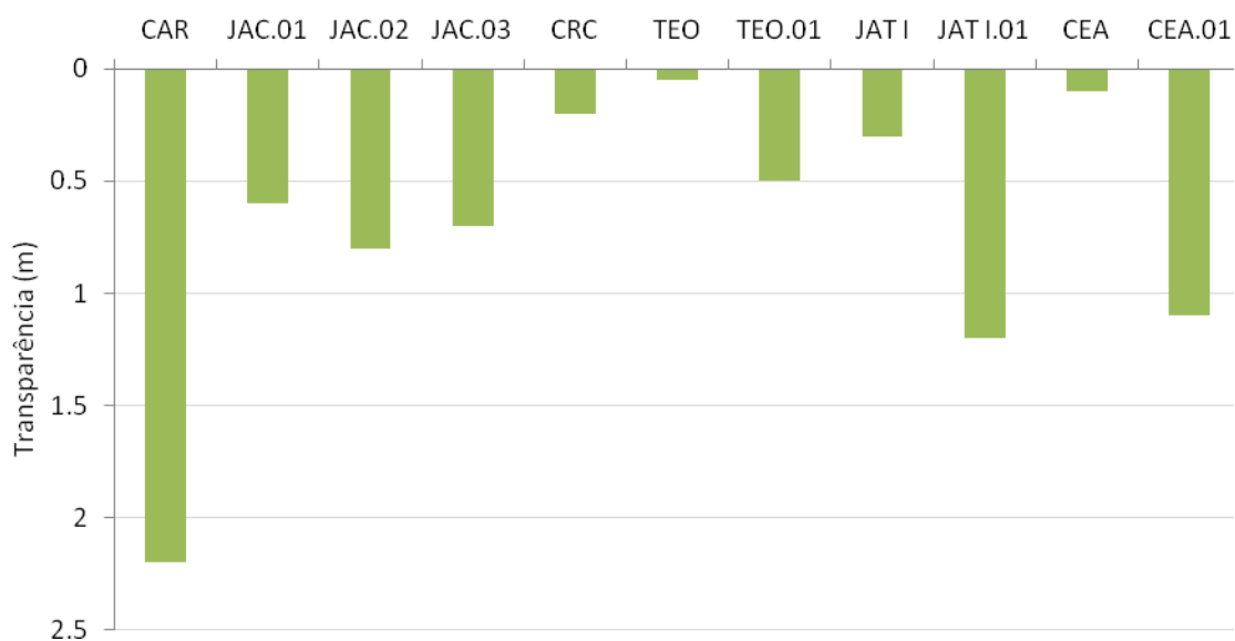
Figura 2-3 - Transparência da coluna d'água nos tributários em maio de 2012 (águas altas).
