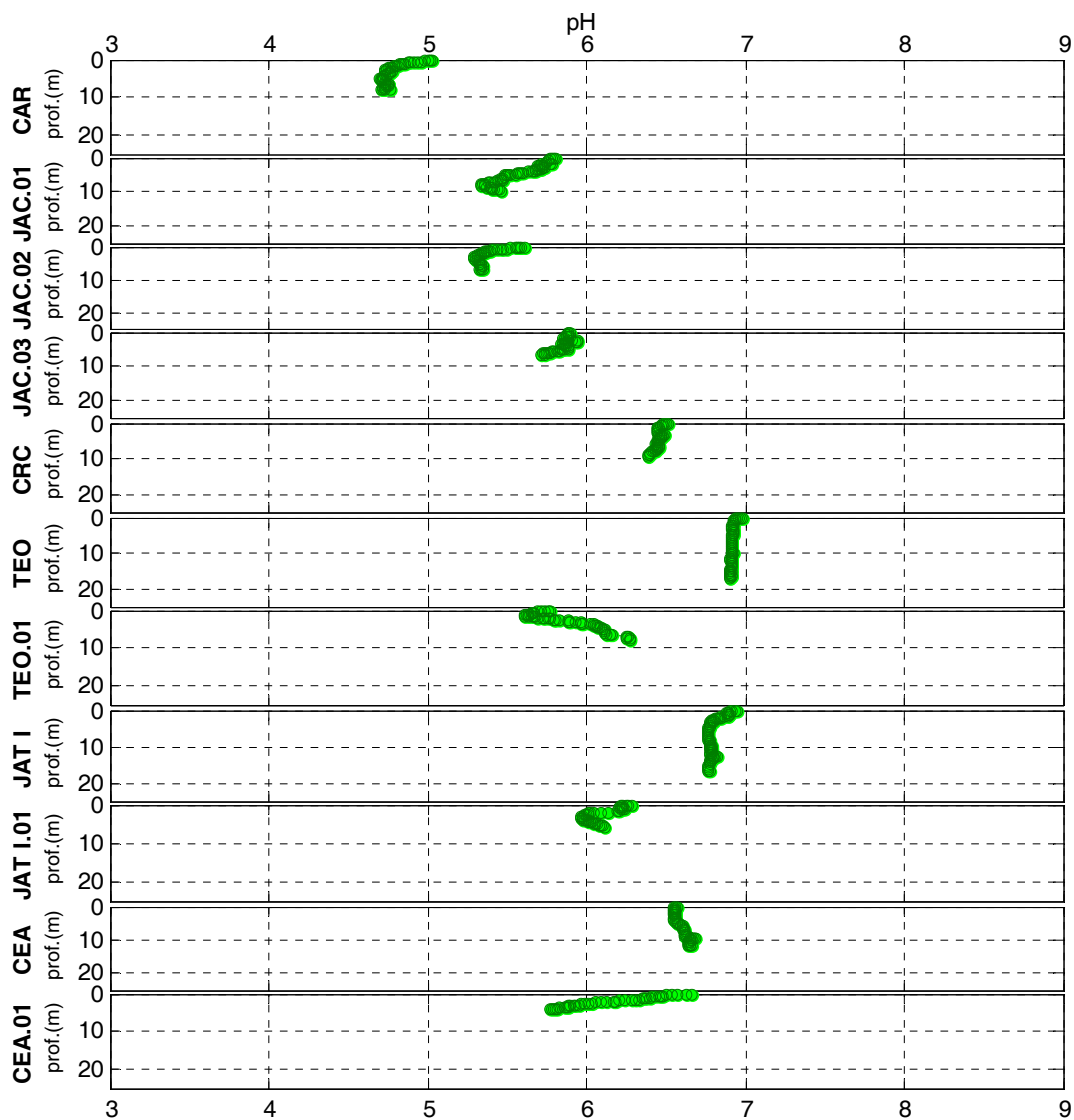
Figura 2-15 - Perfis de pH nos tributários em maio de 2012 (águas altas).
