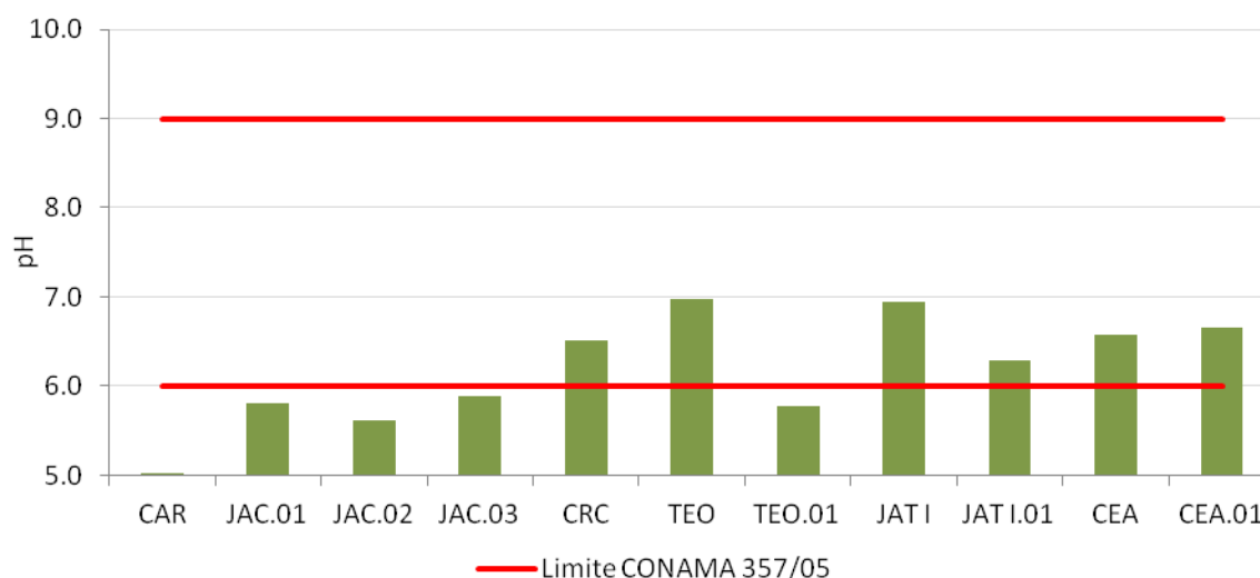
Figura 2-14 - Valores de pH nos tributários em maio de 2012 (águas altas).
