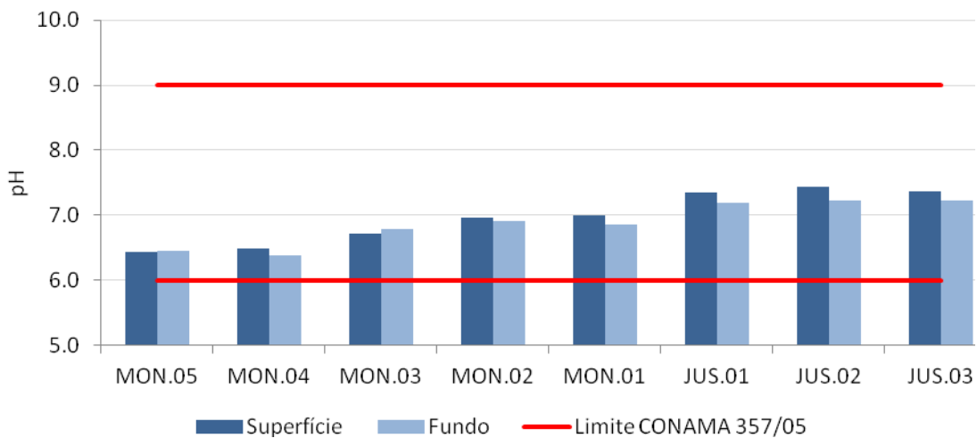
Figura 2-12 - Valores de pH no rio Madeira em maio de 2012 (águas altas).
