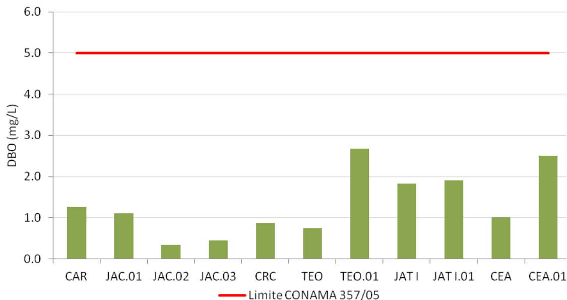
Figura 2-21 - Demanda bioquímica de oxigênio (DBO 5 ) nos tributários em maio de 2012 (águas altas).
