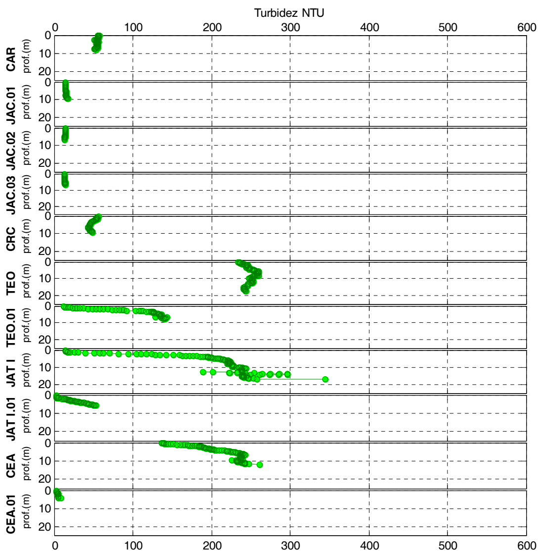
Figura 2-11 - Perfis de turbidez nos tributários em maio de 2012 (águas altas).
