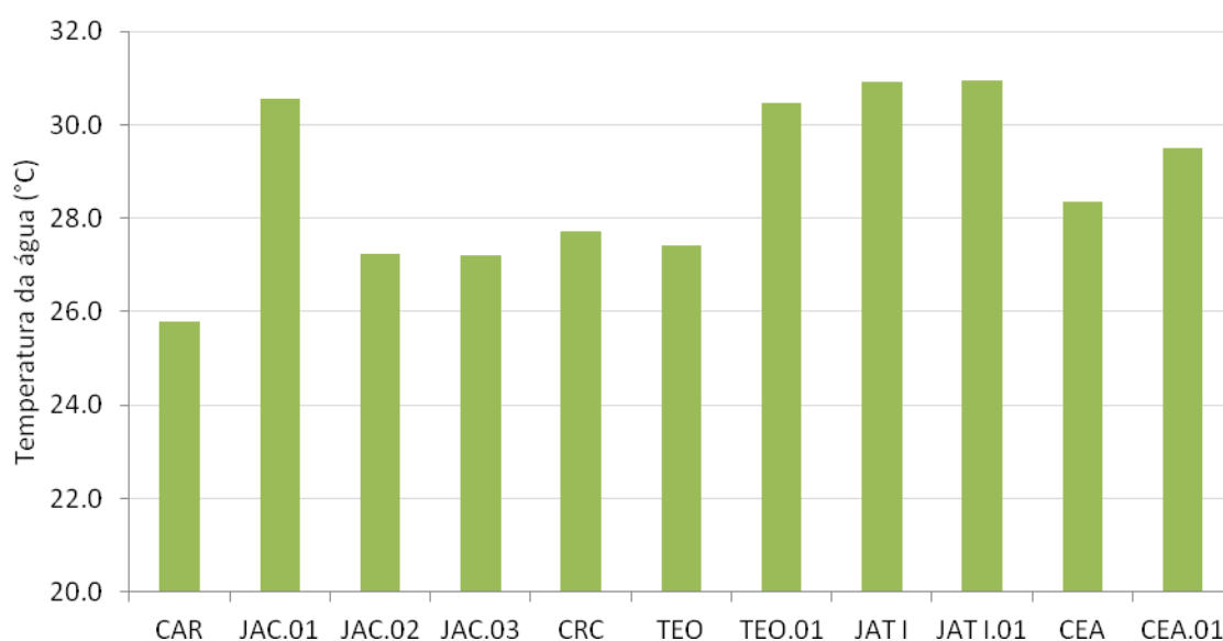
Figura 2-6 - Temperatura da água nos tributários em maio de 2012 (águas altas).
