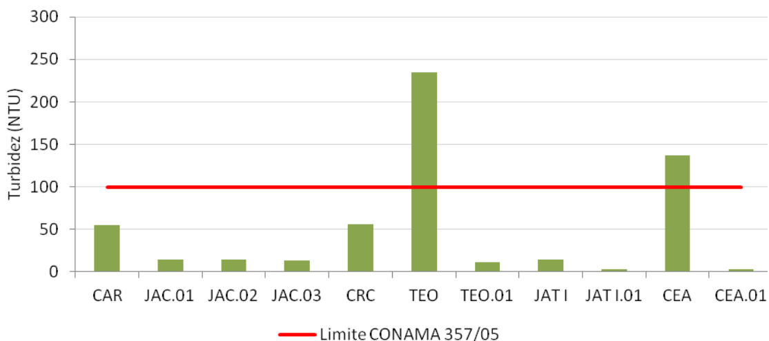
Figura 2-10 - Valores de turbidez nos tributários em maio de 2012 (águas altas).
