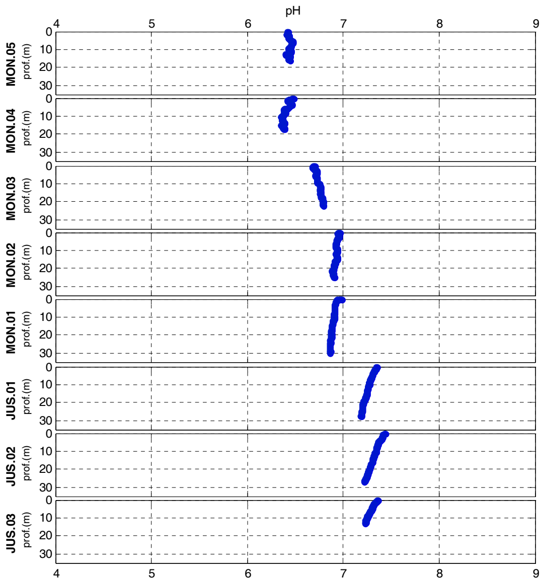
Figura 2-13 - Perfis de pH nos rio Madeira em maio de 2012 (águas altas).
