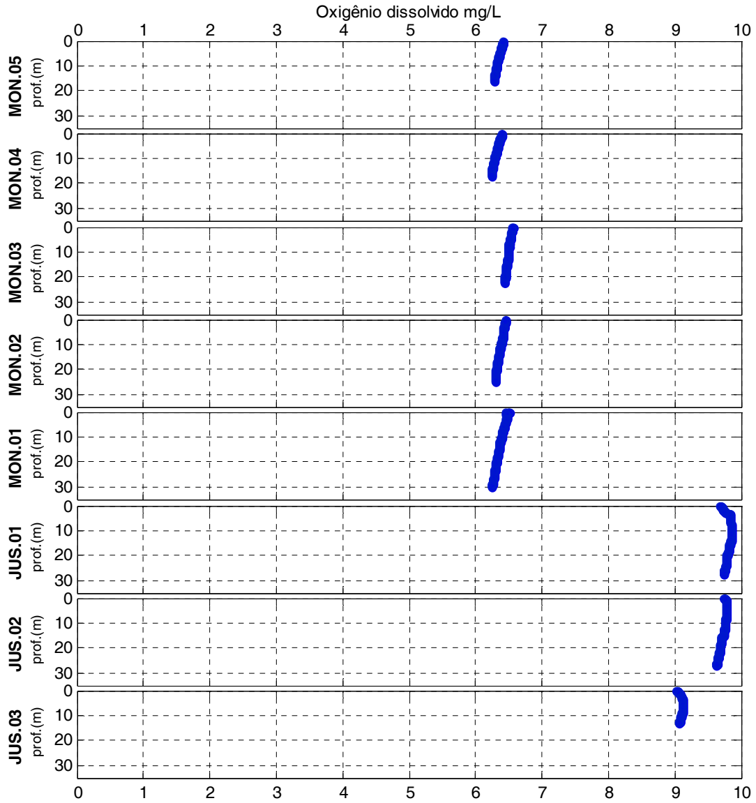
Figura 2-17 - Perfis de concentração de oxigênio dissolvido no rio Madeira em maio de 2012 (águas altas).
