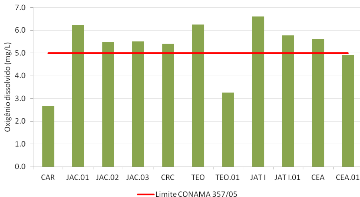
Figura 2-18 - Concentrações de oxigênio dissolvido nos tributários em maio de 2012 (águas altas).
