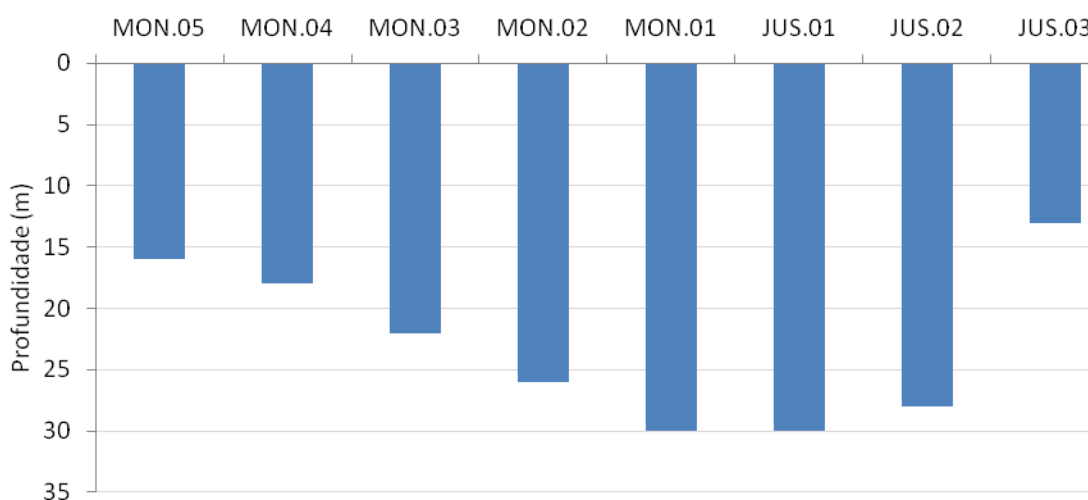
Figura 2-1 - Profundidade da coluna d'água no rio Madeira em maio de 2012 (águas altas).
