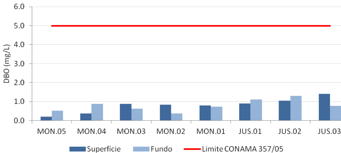
Figura 2-20 - Demanda bioquímica de oxigênio (DBO) nos rio Madeira em maio de 2012 (águas altas).
