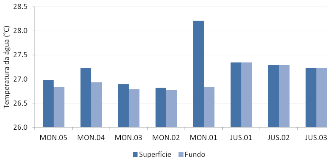
Figura 2-4 - Temperatura da água no rio Madeira em maio de 2012 (águas altas).
