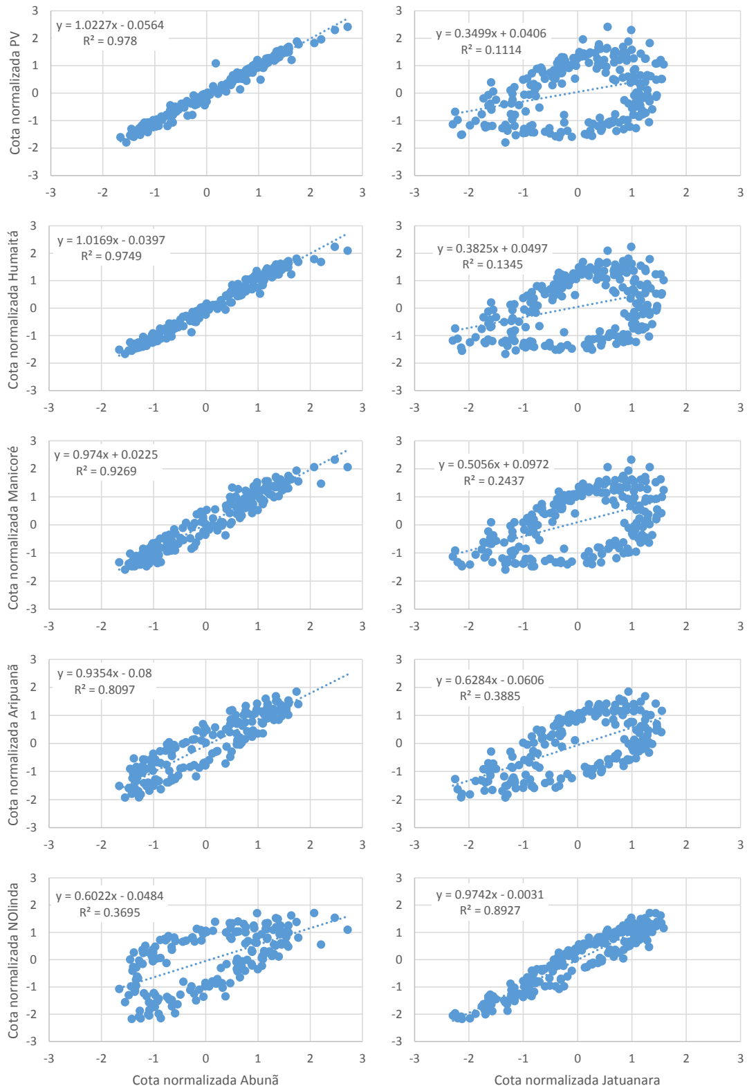
Figura 5. Gráficos de dispersão entre as cotas mensuradas nas estações hidrológicas de Porto Velho, Humaitá, Manicoré, Aripuanã e Nova Olinda do Norte (na ordem superior – inferior) com as cotas mensuradas em Abunã (esquerda) e Jatuarana-AM (direita). As cotas foram padronizadas e normalizadas (média=0, desvio-padrão=1) e referem-se ao período de janeiro/1996 a dezembro/2014.
