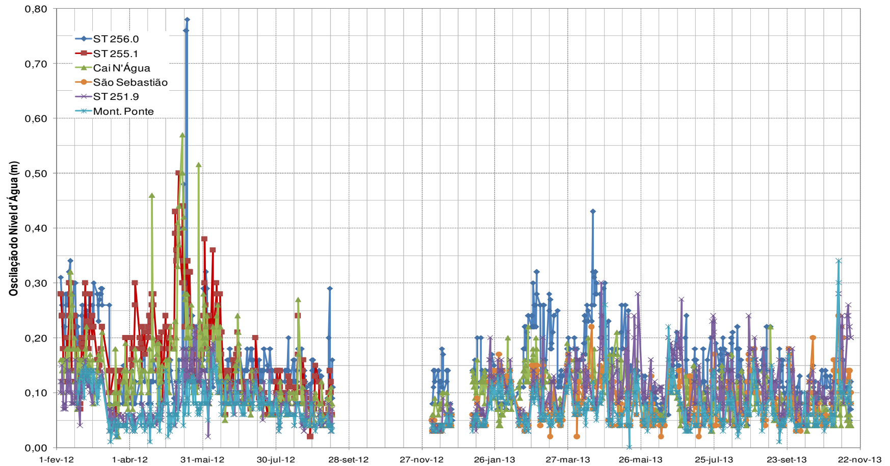
Figura 3. Oscilação mais freqüente do nível d'água nos locais de monitoramento a jusante da UHE Santo Antônio – 04/02/12 a 14/11/13
