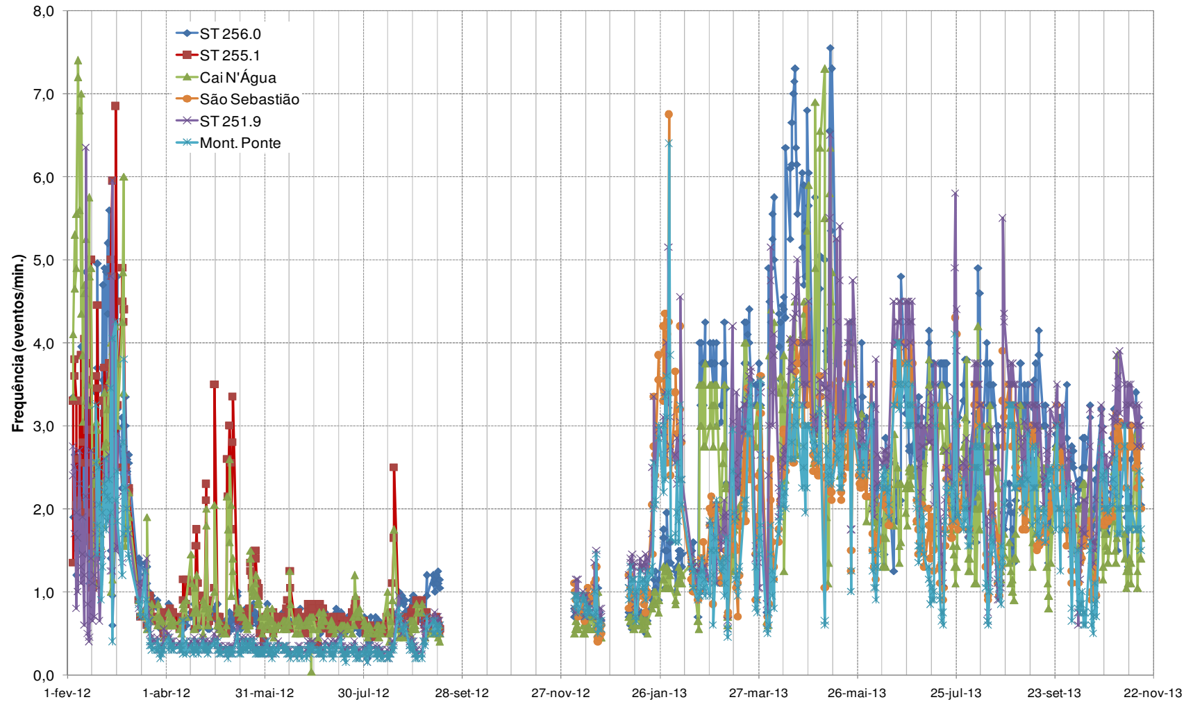
Figura 7. Frequência da oscilação do nível d'água nos locais de monitoramento a jusante da UHE Santo Antônio
