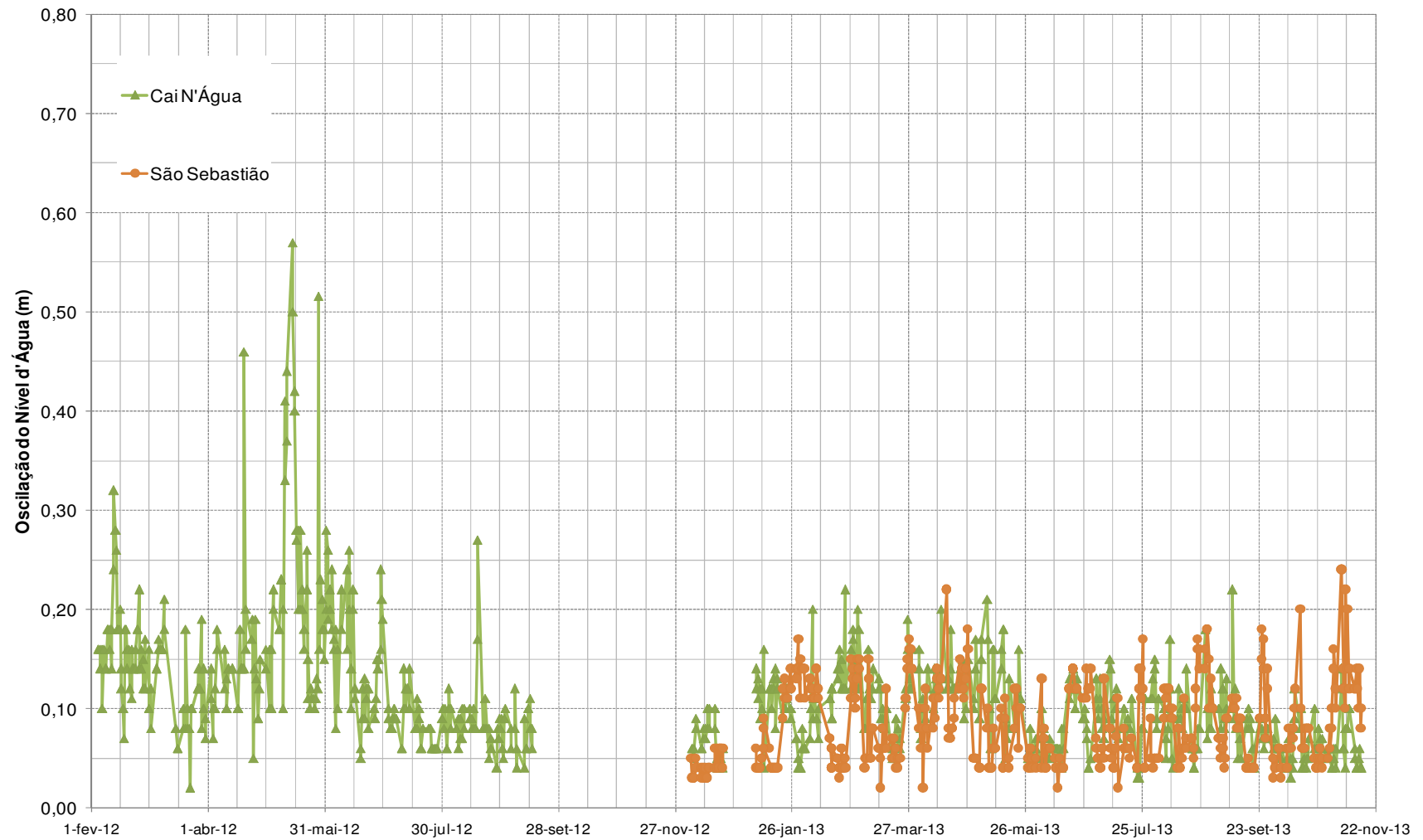
Figura 5. Oscilação mais freqüente do nível d'água – Cai n'água e São Sebastião
