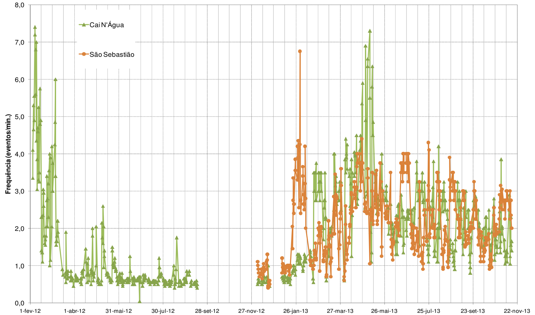
Figura 9. Frequência da oscilação do nível d'água – Cai n'água e São Sebastião
