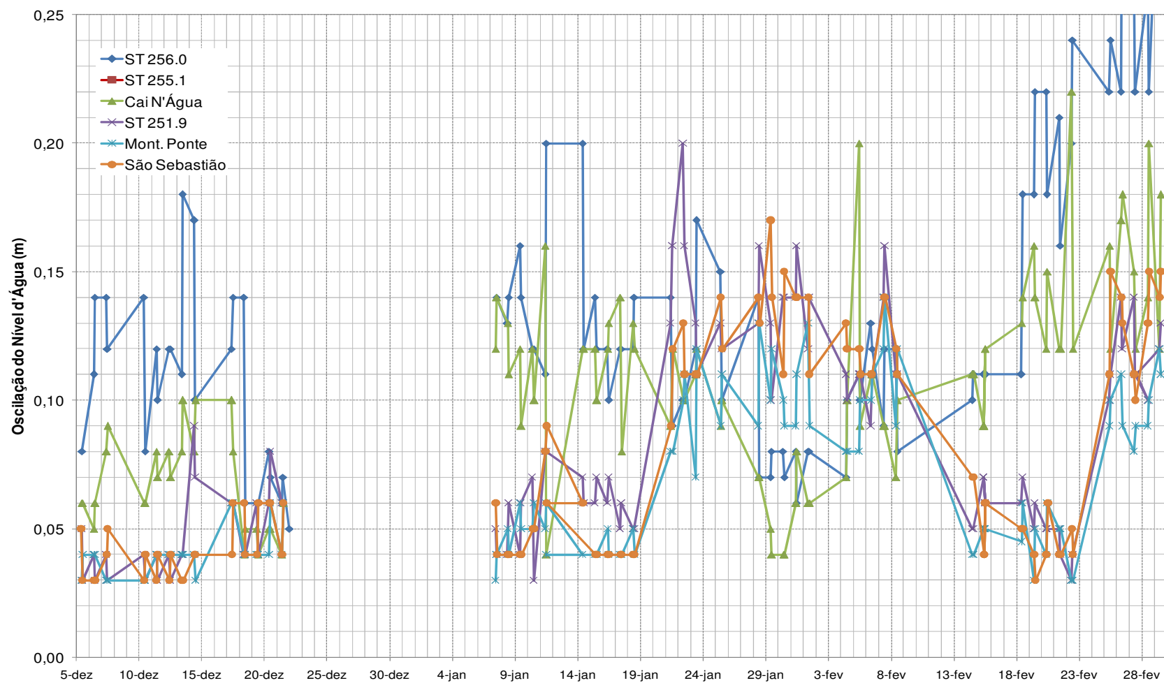
Figura 4. Oscilação mais freqüente do nível d'água nos locais de monitoramento a jusante da UHE Santo Antônio no Período de 05/12/12 a 01/03/13
