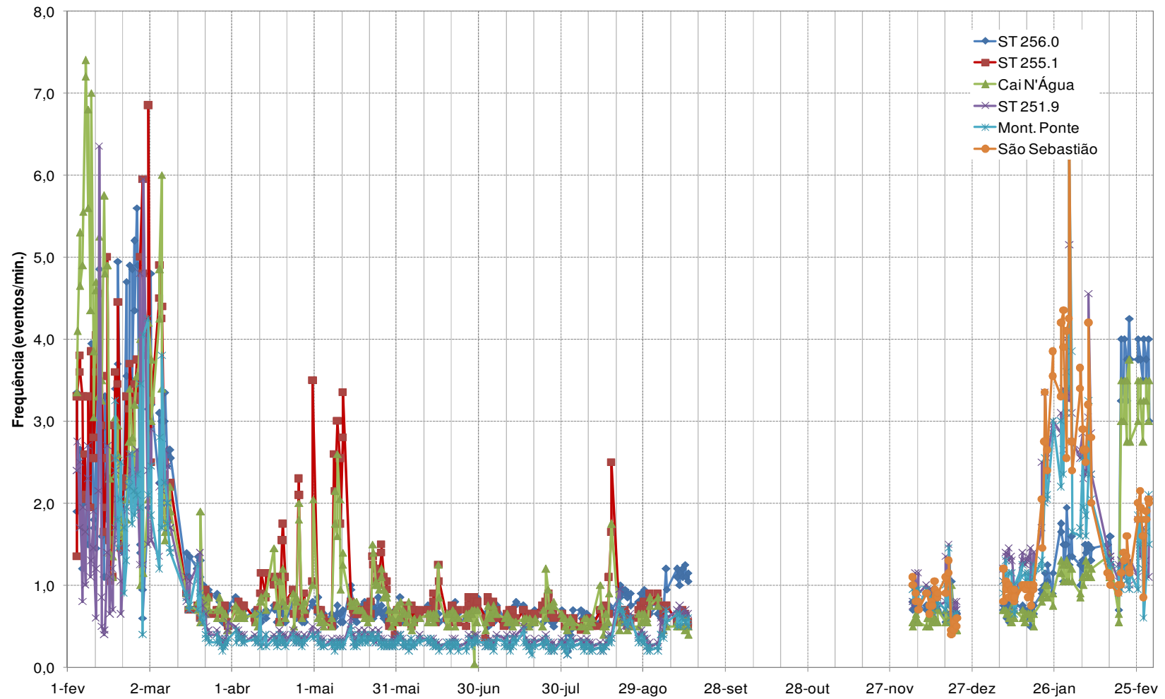
Figura 5. Frequência da oscilação do nível d'água nos locais de monitoramento a jusante da UHE Santo Antônio
