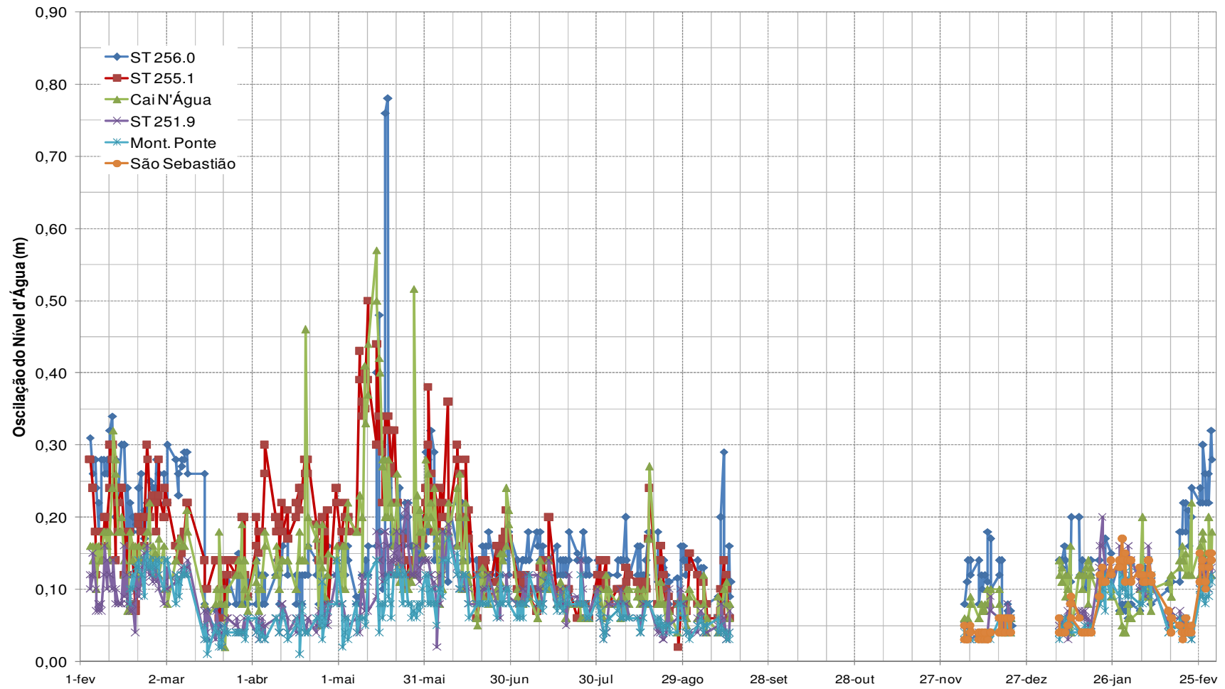
Figura 3. Oscilação mais freqüente do nível d'água nos locais de monitoramento a jusante da UHE Santo Antônio
